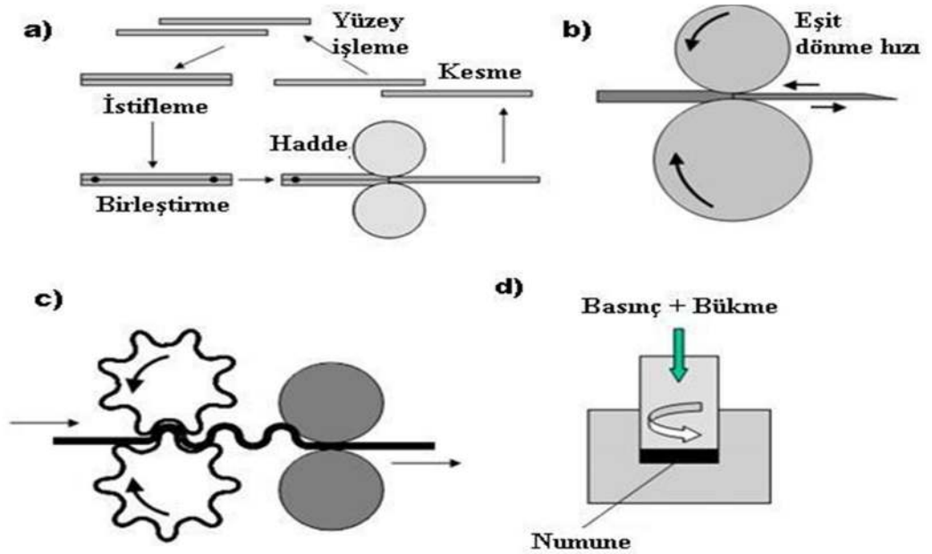
Şekil 1.1. APD yöntemleri a) Biriktirmeli haddeli birleştirme b) Asimetrik haddeleme c) Sürekli kıvrırma ve sertleştirme d) Yüksek basınçta bükme (Verlinden 2006)
