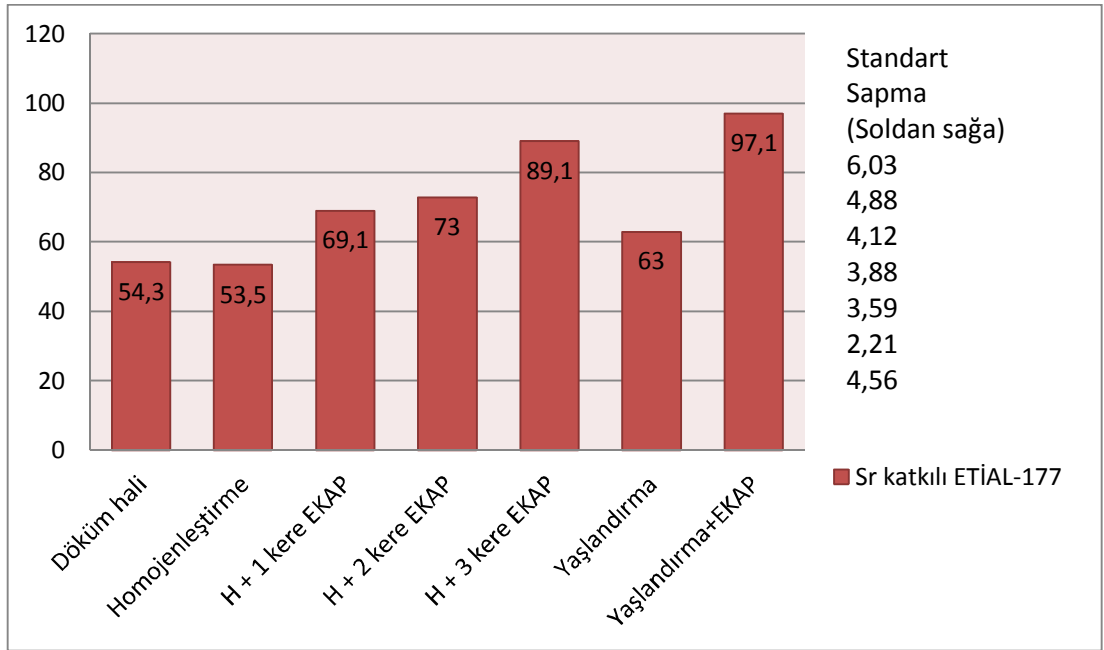
Şekil 4.2. % 0,02 Sr katkılı ETİAL-177 sertlik değerleri grafiği
