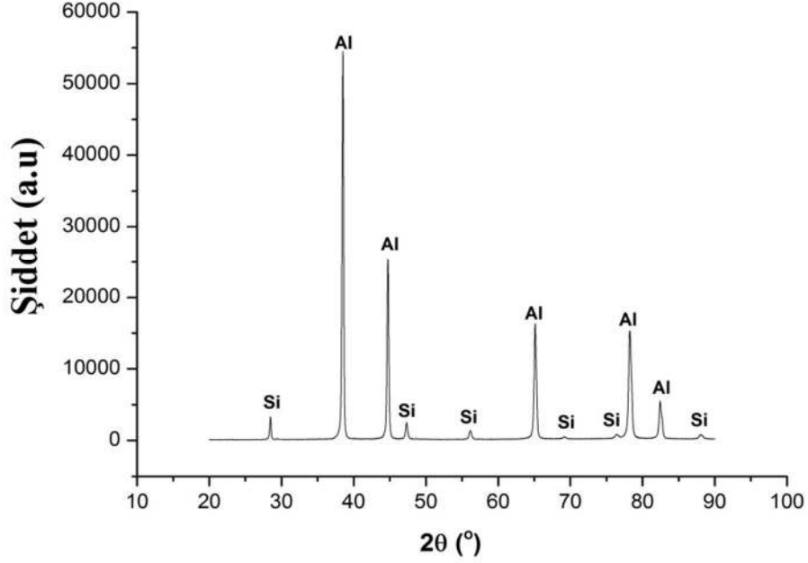
Şekil 7.66. Al-5Ti-1B 1 kere EKAP işlemlili katkılı ETİAL-177 XRD analiz grafiği
