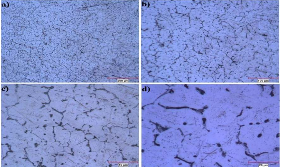
Şekil 7.36. % 5 Al-5Ti-1B EAP işlemsiz katkı ETİAL-220 hali mikro yapı fotoğrafları a) 100x b) 200x c) 500x d) 1000x
