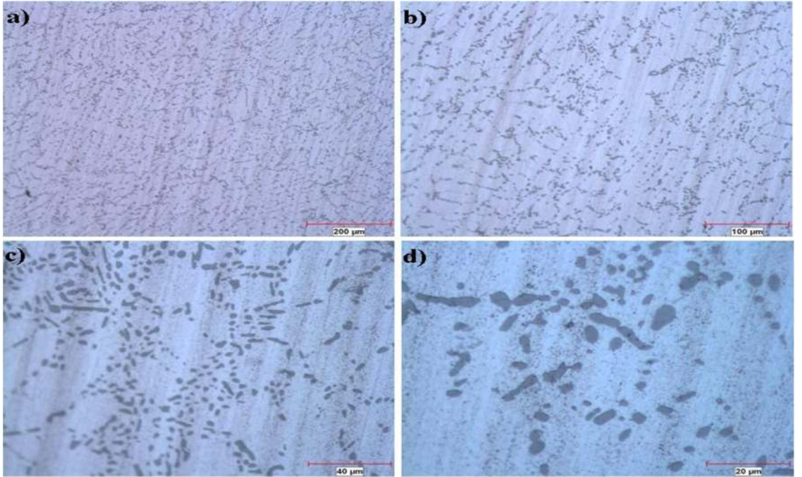
Şekil 7.18. % 0,2 Al-5Ti-1B 1 kere EAPK işlemli katkılı ETİAL-177 2 kere sıcak EAPK hali mikro yapı fotoğrafları a) 100x b) 200x c) 500x d) 1000x
