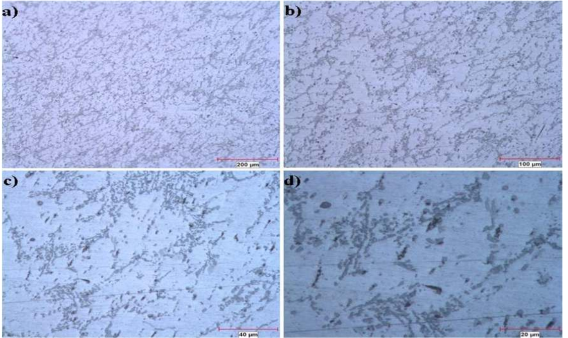
Şekil 7.26. % 5 Al-5Ti-1B 2 kere EKAP işlemli katkılı ETİAL-177 sıcak EKAP hali mikro yapı fotoğrafları a) 100x b) 200x c) 500x d) 1000x
