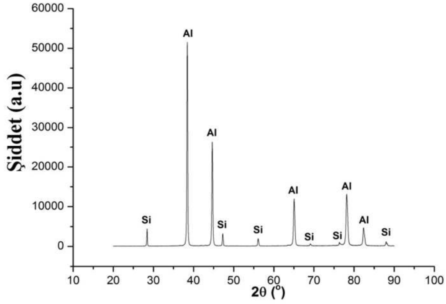
Şekil 7.59. ETİAL-177 yaşlandırma sonrası EKAP işlemleri numune XRD analiz grafiği
