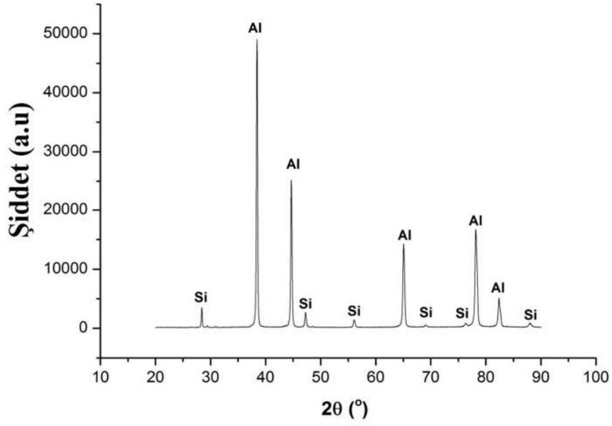
Şekil 7.65. Al-5Ti-1B EKAP işlemsiz katkılı ETİAL-177 XRD analiz grafiği
