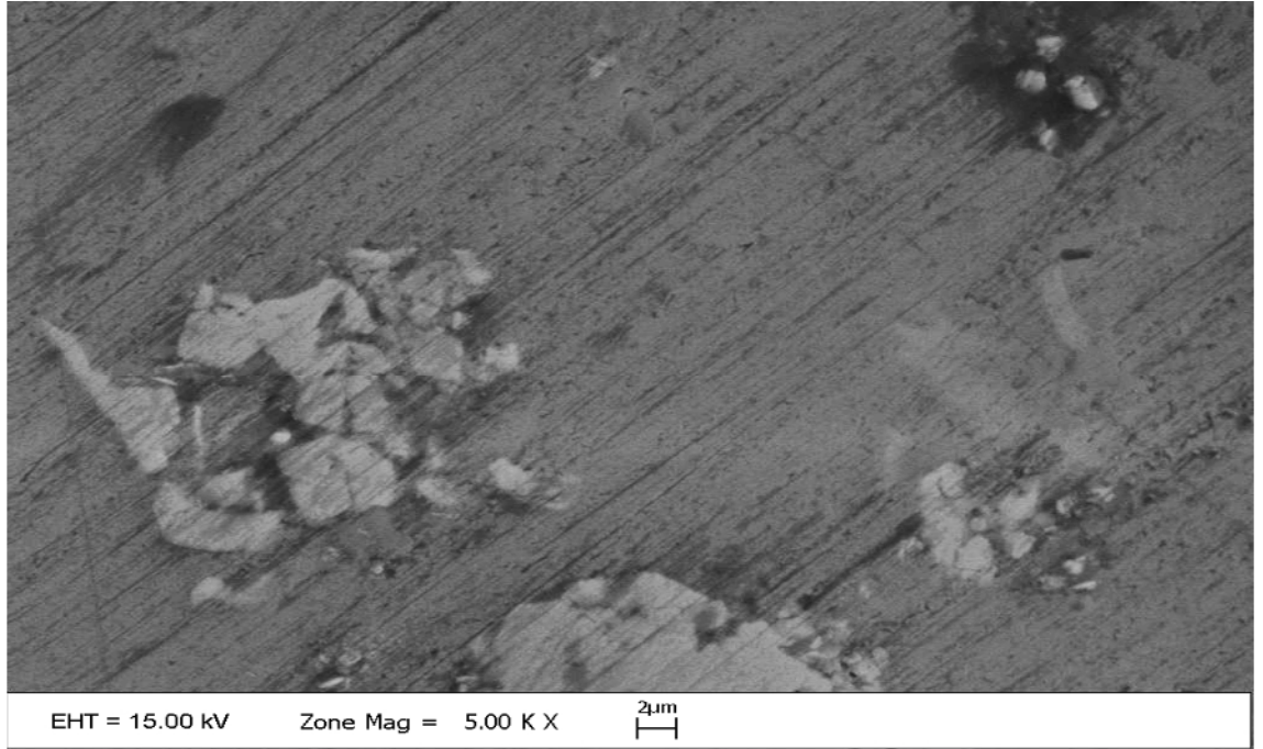
Şekil 7.79. 500 °C 4h tavllanmış % 5 Al-5Ti-1B katkılı ETİAL-177 numunesi SEM fotoğrafı
