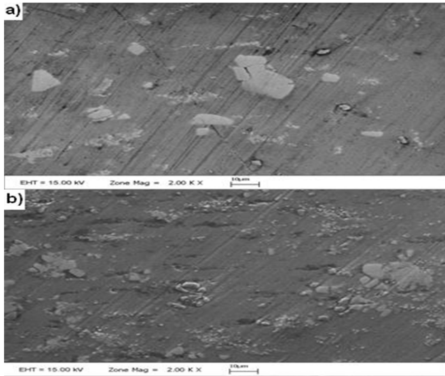
Şekil 4.17. Al-5Ti-1B SEM fotoğrafları a) 1 kere EKAP işlemli b) 2 kere EKAP işlemli
