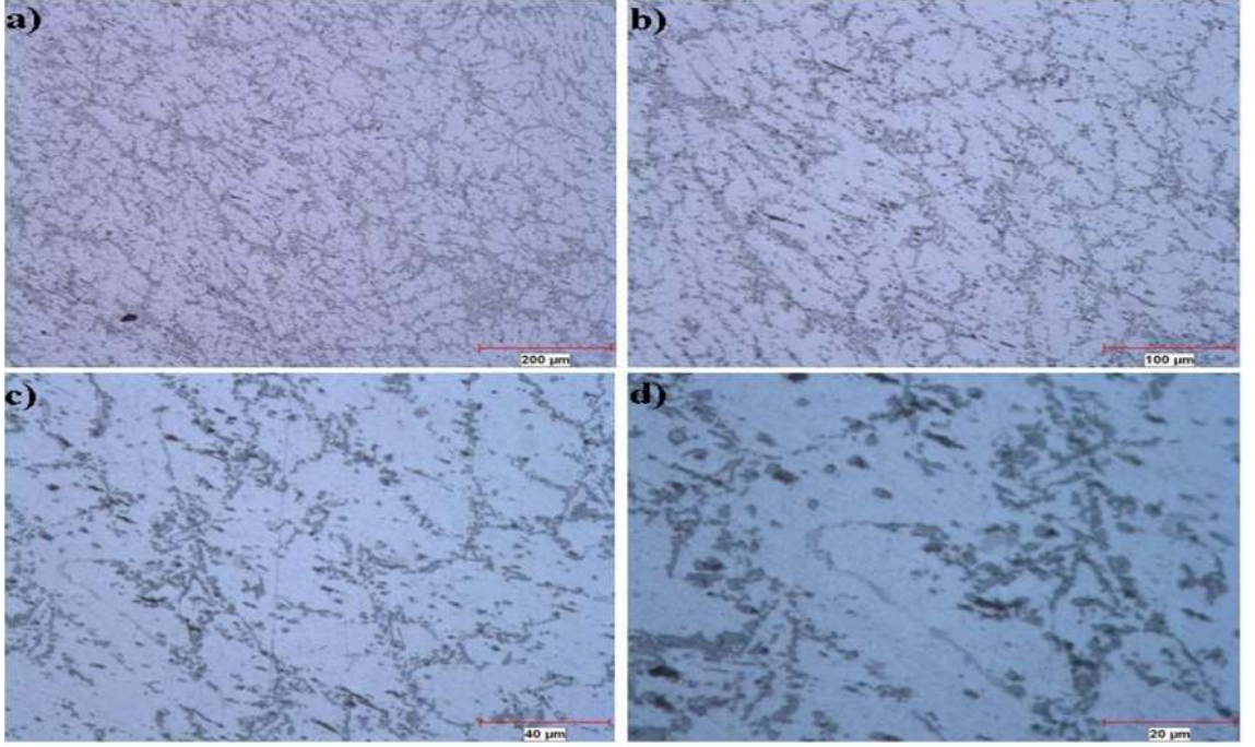
Şekil 7.25. % 5 Al-5Ti-1B 1 kere EKAP işlemli katkılı ETİAL-177 sıcak EKAP hali mikro yapı fotoğrafları a) 100x b) 200x c) 500x d) 1000x
