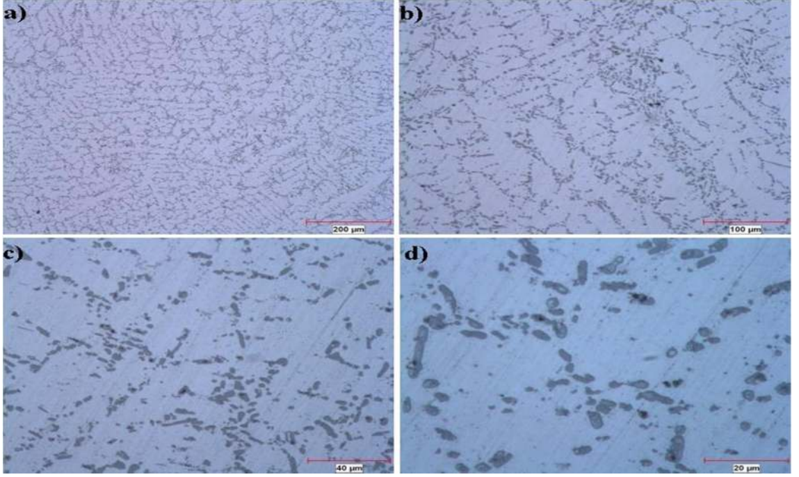
Şekil 7.17. % 0,2 Al-5Ti-1B EAPK işlemsiz katkılı ETİAL-177 2 kere sıcak EAPK hali mikro yapı fotoğrafları a) 100x b) 200x c) 500x d) 1000x
