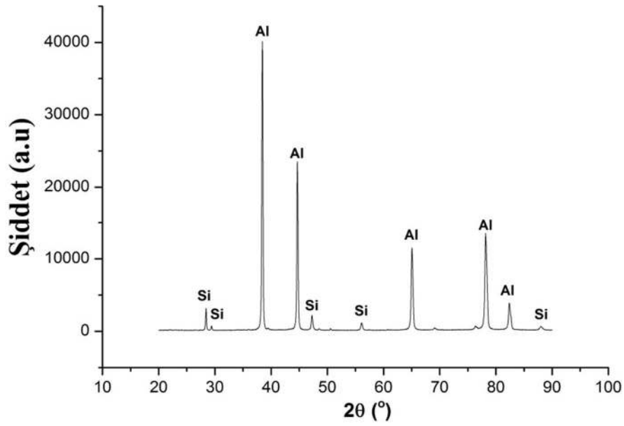
Şekil 7.68. Al-5Ti-1B sıcak EKAP sonrası 400 °C 4 saat tavlanmış katkılı ETİAL-177 numune XRD analiz grafiği
