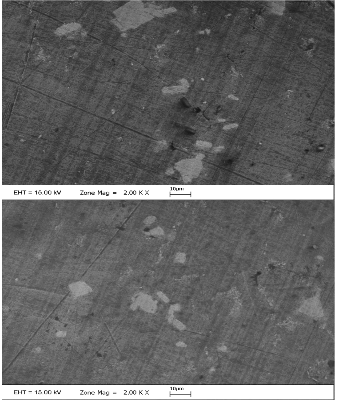
Şekil 7.76. 500 °C 4h tavlanmış Al-5Ti-1B numunesi SEM fotoğrafları
