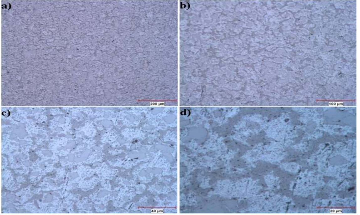
Şekil 7.50. Al-5Ti-1B döküm sonrası 600 °C 4 saat tavlanmış hali mikro yapı fotoğrafları a) 100x b) 200x c) 500x d) 1000x
