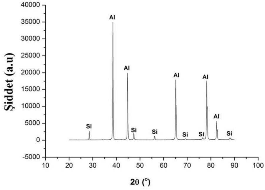
Şekil 7.63. Al-5Ti-1B 500 °C 4 saat tavllanmış numune katkılı ETİAL-177 XRD analiz grafiği
