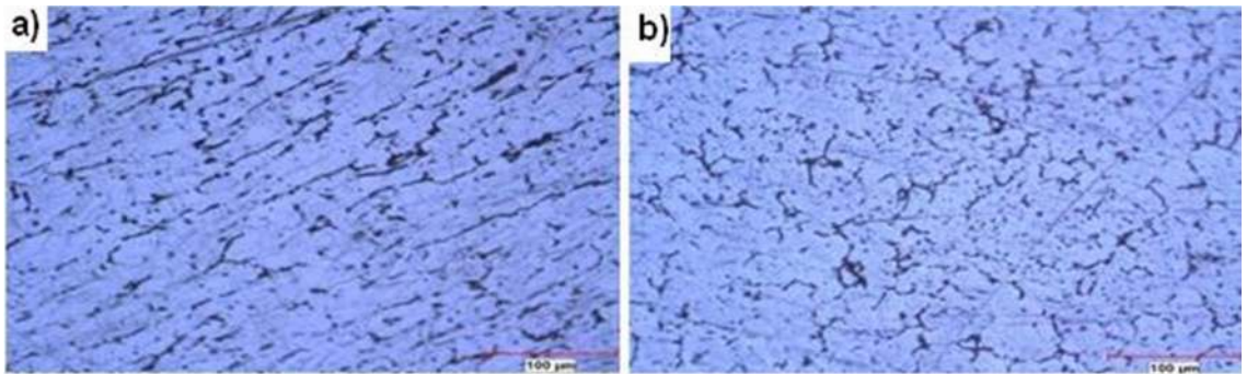
Şekil 4.15. % 5 EKAP işlemsiz Al-5Ti-1B katkılı ETİAL-220 mikro yapı fotoğrafları 200x a) 1 kere EKAP işlemi uygulanmış b) 2 kere EKAP işlemi uygulanmış
