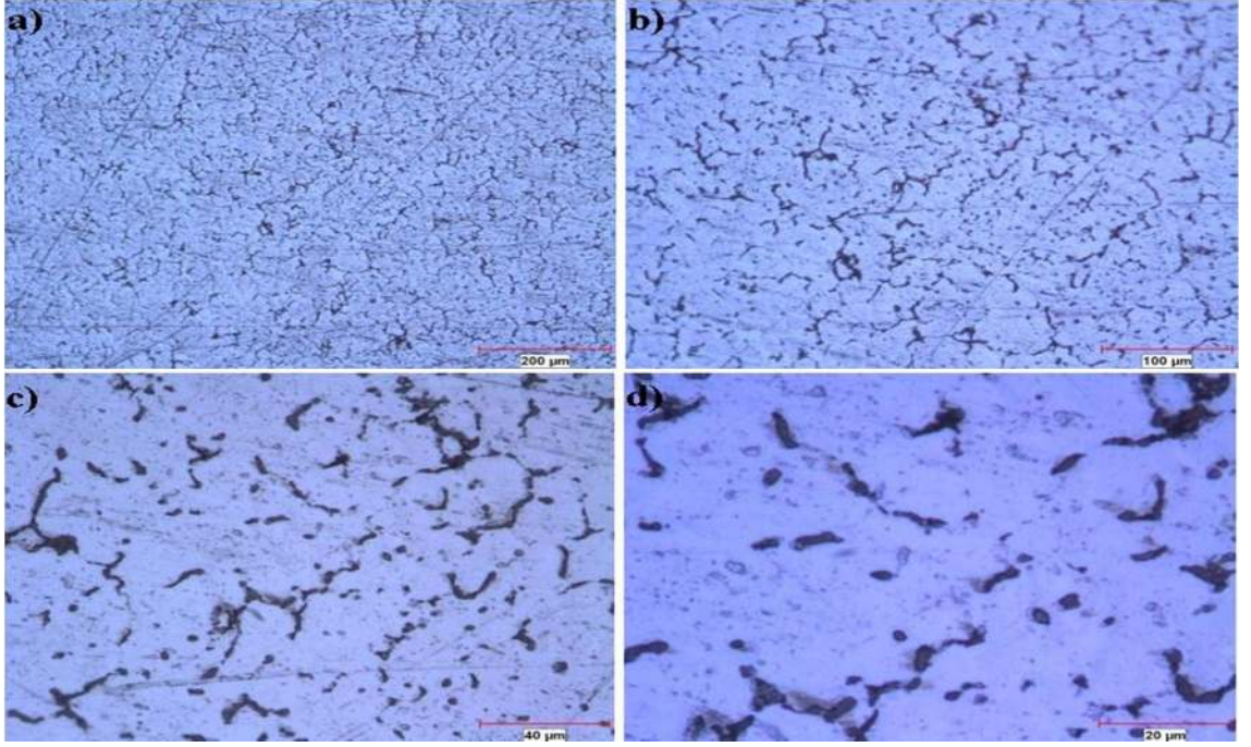
Şekil 7.38. % 5 Al-5Ti-1B EKAP işlemsiz katkılı ETİAL-220 2 kere EKAP hali mikro yapı fotoğrafları a) 100x b) 200x c) 500x d) 1000x
