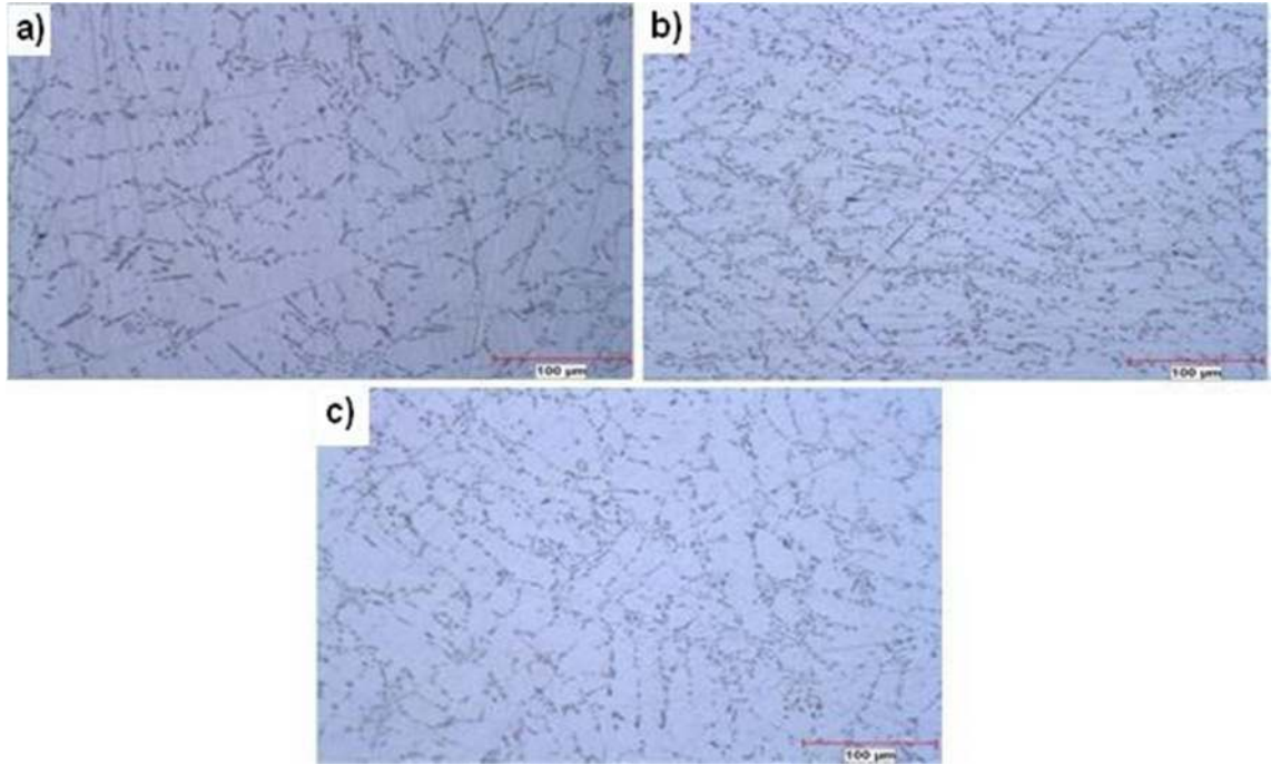
Şekil 4.11. % 0,2 Al-5Ti-1B katkılı ETİAL-177 mikro yapı fotoğrafları 200x a) homojenleştirme b) 1 kere EKAP işlemli c) 2 kere EKAP işlemli
