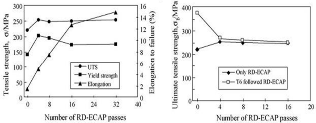
Şekil 2.2. EKAP paso sayısının çekme dayanımına etkisi (solda), EKAP öncesi T6 ısıt işleminin maksimum çekme dayanımına etkisi (sağda) (Ma vd 2005)
