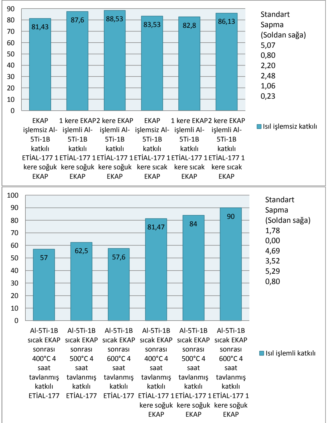
Şekil 4.4. % 5 Al-5Ti-1B katkı ETİAL-177 sertlik değerleri grafikleri
