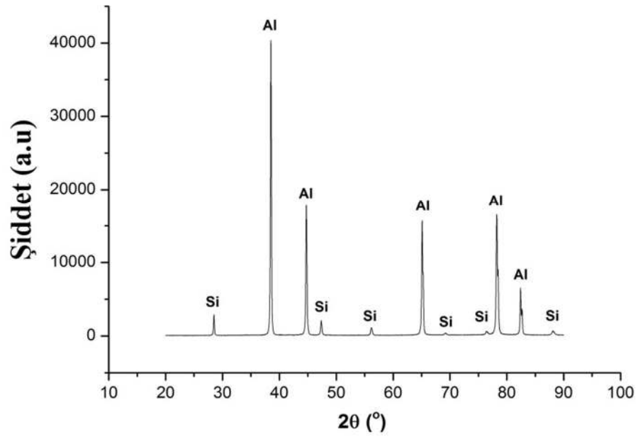
Şekil 7.62. Al-5Ti-1B 400 °C 4 saat tavllanmış numune katkılı ETİAL-177 XRD analiz grafiği
