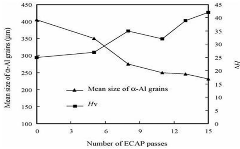
Şekil 2.17. EKAP yapılmış % 5 Ti katkılı Al alaşımı ortalama tane büyüklükleri ve mikrosertlikleri (Zhang vd 2006)
