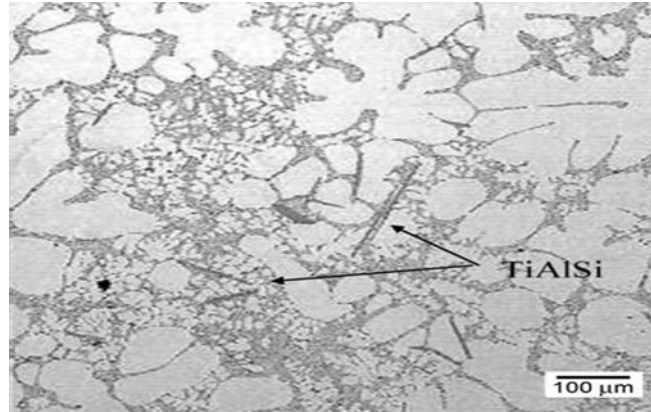
Şekil 2.16. Döküm dokusunda TiAlSi intermetalik fotoğrafı (Chen ve Fortier 2010)
