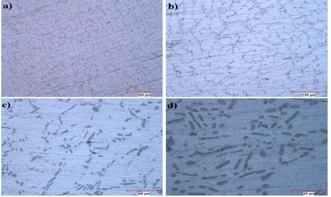
Şekil 7.11. Sr katkılı ETİAL-177 homojenleştirme sonrası 3 kere EKAP hali mikro yapı fotoğrafları a) 100x b) 200x c) 500x d)1000x
