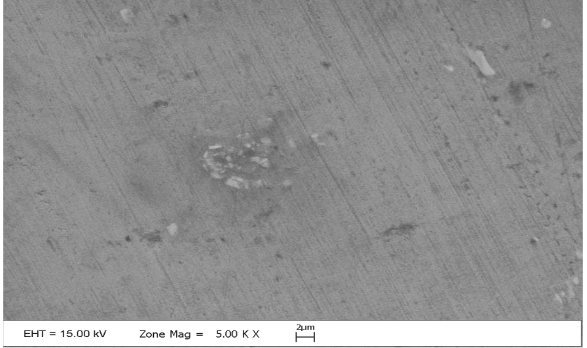
Şekil 7.78. 400 °C 4h tavllanmış % 5 Al-5Ti-1B katkılı ETİAL-177 numunesi SEM fotoğrafı
