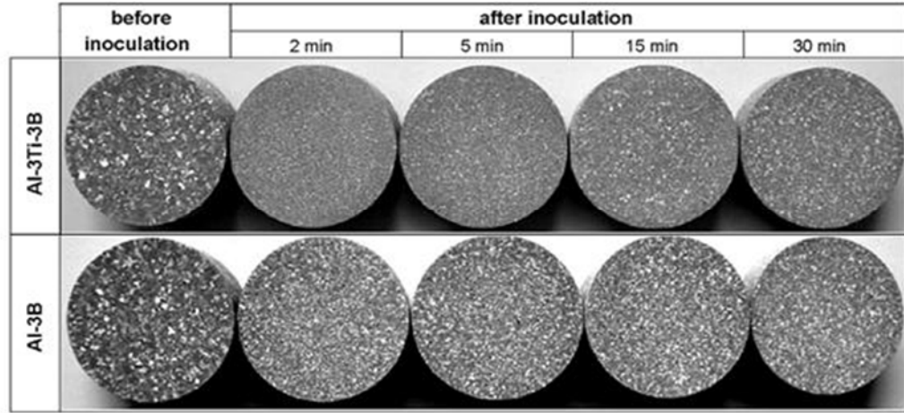
Şekil 2.15. Al-3B ve Al-3Ti-3B katkılarının tutma süresinin mikro yapıya etkisi (Bırol ve Novel 2009)
