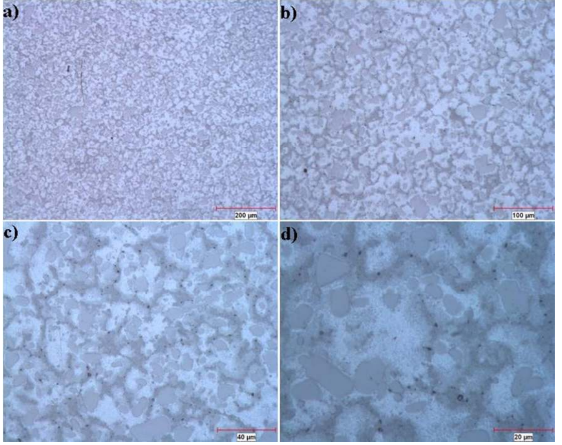
Şekil 7.56. Al-5Ti-1B sıcak EKAP sonrası 600 °C 4 saat tavlanmış hali mikro yapı fotoğrafları a) 100x b) 200x c) 500x d) 1000x
