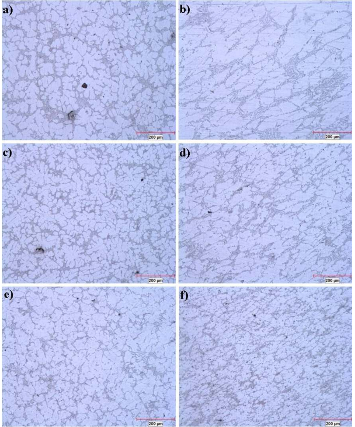
Şekil 7.27. % 5 Al-5Ti-1B 400-500-600 °C 4 saat tavlanmış katkılı ETİAL-177 EKAP hali mikro yapı fotoğrafları 100x a) 400 °C 4 saat tavlanmış katkılı döküm hali b) 400 °C 4 saat tavlanmış katkılı EKAP işlemleri c) 500 °C 4 saat tavlanmış katkılı döküm hali d) 500 °C 4 saat tavlanmış katkılı EKAP işlemleri e) 600 °C 4 saat tavlanmış katkılı döküm hali f) 600 °C 4 saat tavlanmış katkılı EKAP işlemleri
