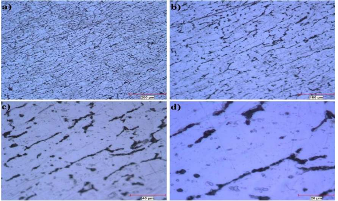
Şekil 7.37. % 5 Al-5Ti-1B EAP işlemsiz katkı ETİAL-220 1 kere EAP hali mikro yapı fotoğrafları a) 100x b) 200x c) 500x d) 1000x
