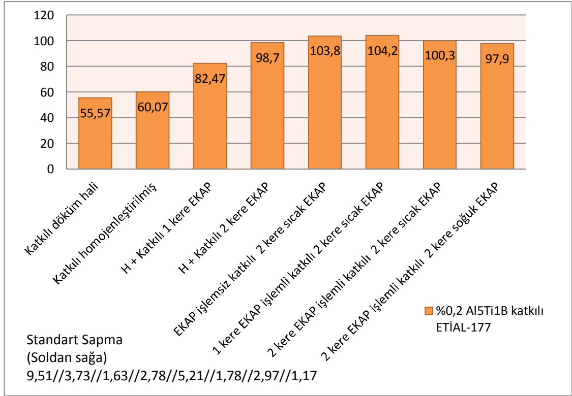
Şekil 4.3. % 0,2 Al-5Ti-1B katkılı ETİAL-177 sertlik değerleri grafiği
