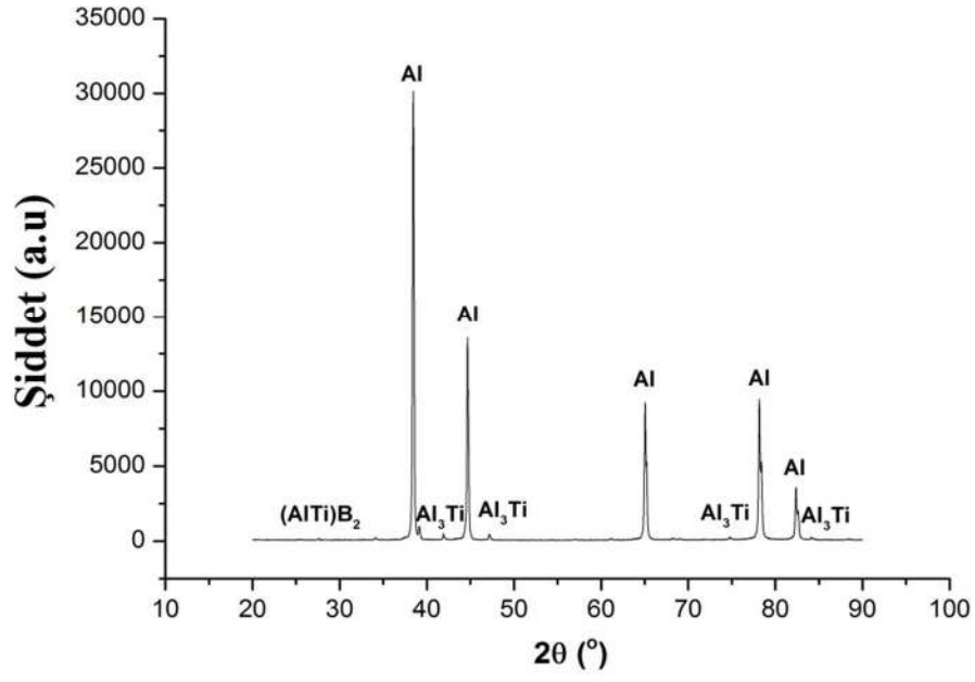
Şekil 7.61. Al-5Ti-1B 2 kere EKAP işlemlili numune XRD analiz grafiği
