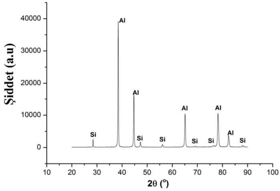
Şekil 7.70. Al-5Ti-1B sıcak EKAP sonrası 600 °C 4 saat tavllanmış katkılı ETİAL-177 XRD analiz grafiği
