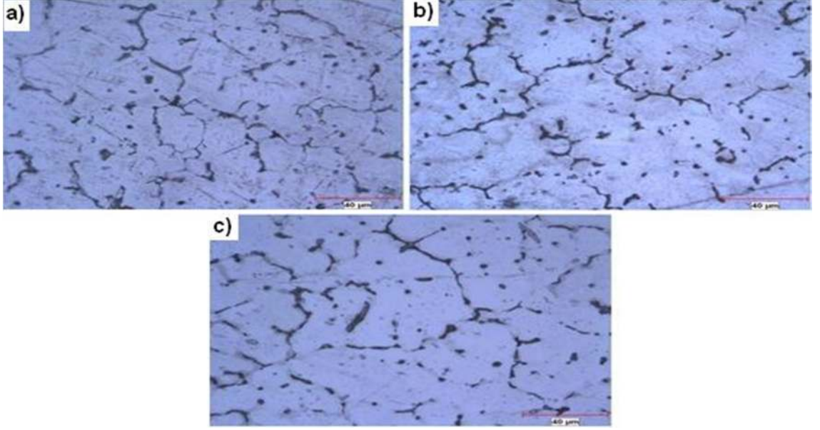
Şekil 4.14. % 5 Al-5Ti-1B katkılı ETİAL-220 mikro yapı fotoğrafları 500x a) EKAP işlemsiz katkı b) 1 kere EKAP işlemlili katkı c) 2 kere EKAP işlemlili katkı
