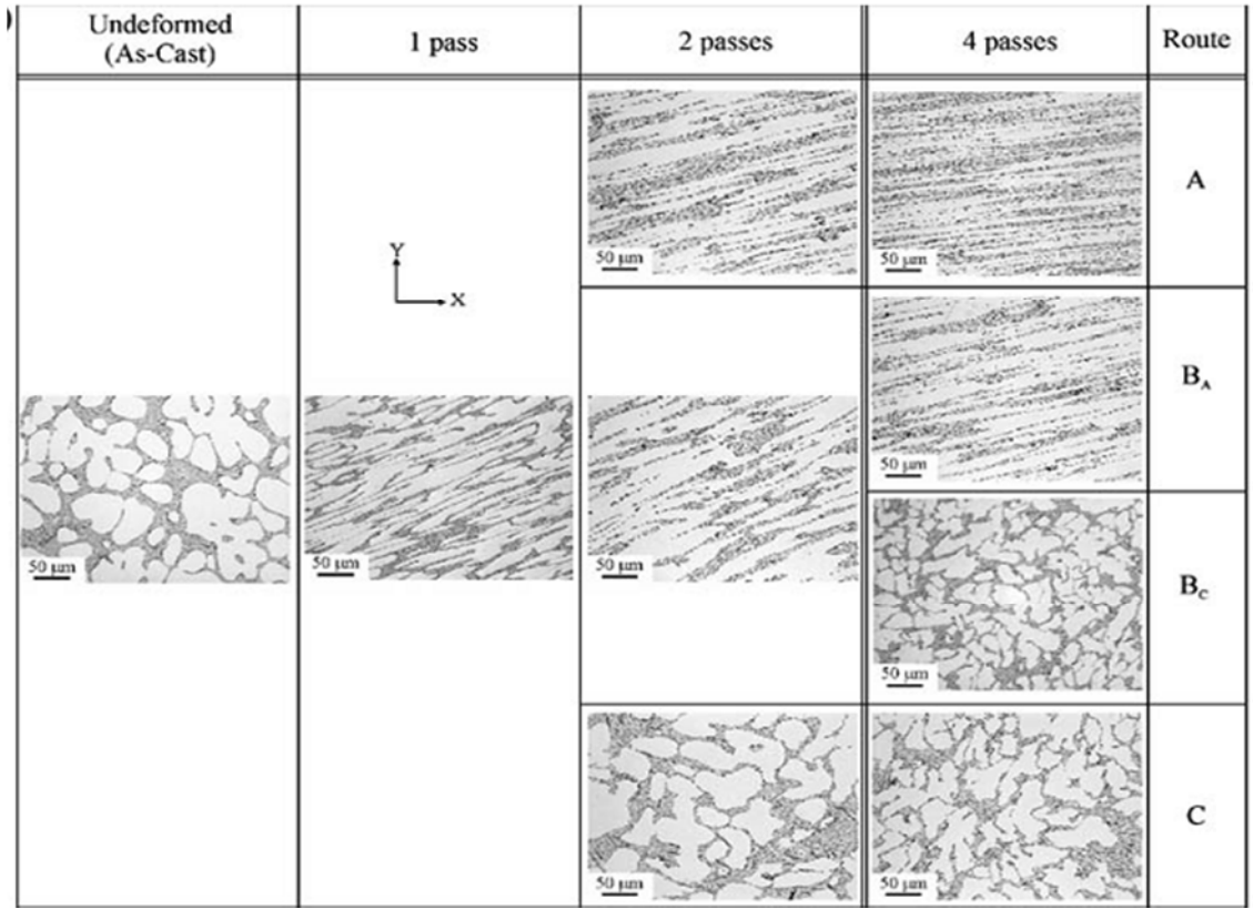
Şekil 2.9. EKAP yönleri ve EKAP paso sayısına göre değişen mikro yapı (Swaminathan vd 2008)
