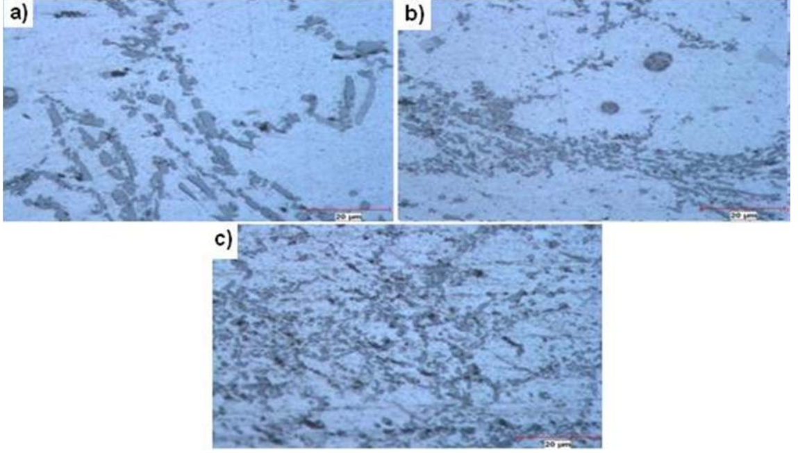
Şekil 4.12. % 5 Al-5Ti-1B katkılı ETİAL-177 mikro yapı fotoğrafları 1000x a) EKAP işlemsiz katkılı b) 1 kere EKAP işlemli katkılı c) 2 kere EKAP işlemli katkılı
