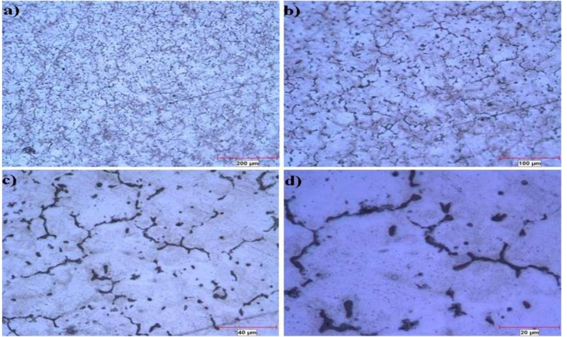
Şekil 7.39. % 5 Al-5Ti-1B 1 kere EKAP işlemlili katkılı ETİAL-220 hali mikro yapı fotoğrafları a) 100x b) 200x c) 500x d) 1000x
