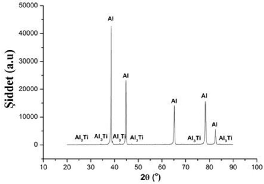
Şekil 7.60. Al-5Ti-1B 1 kere EKAP işlemleri numune XRD analiz grafiği
