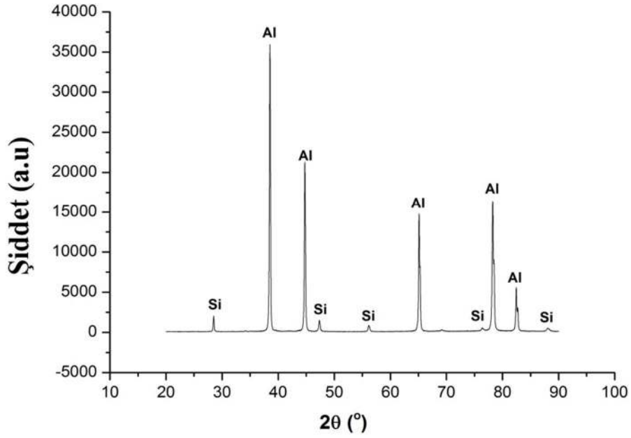
Şekil 7.64. Al-5Ti-1B 600 °C 4 saat tavllanmış numune katkılı ETİAL-177 XRD analiz grafiği
