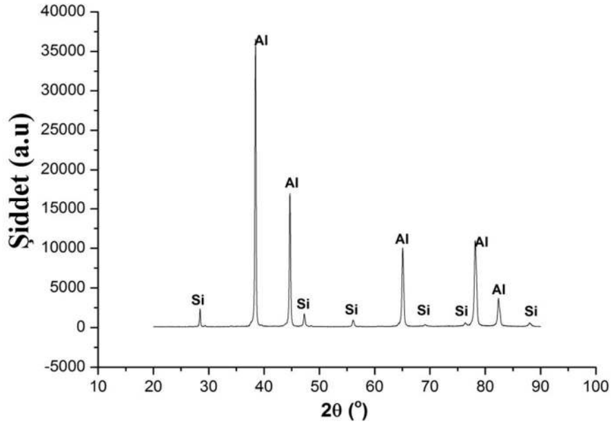
Şekil 7.69. Al-5Ti-1B sıcak EKAP sonrası 500 °C 4 saat tavllanmış katkılı ETİAL-177 XRD analiz grafiği
