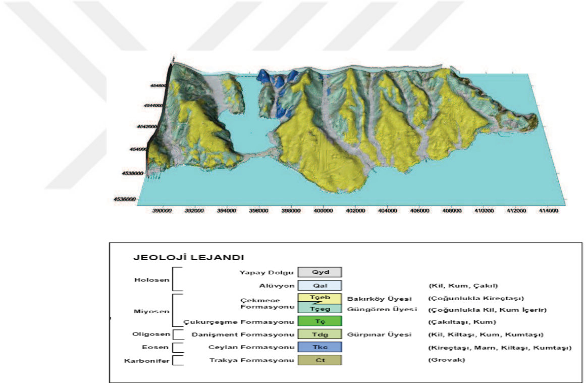
Harita 2: Araştırma Alanının Kuşbakışı Jeolojisi
