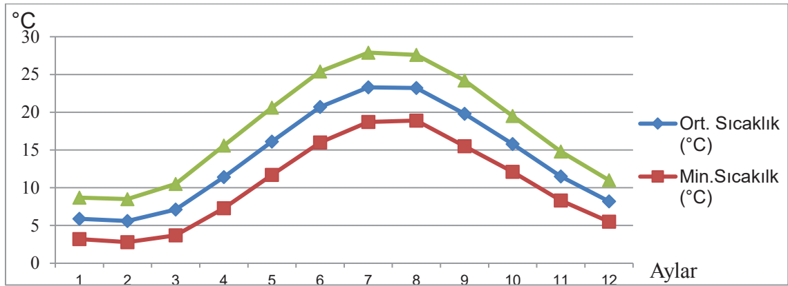
Şekil 3: Ortalama, Minimum ve Maksimum Sıcaklıkların Aylara Göre Dağılışı
