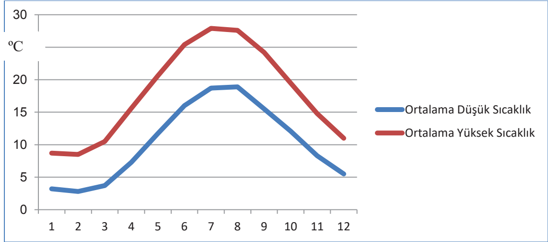
Şekil 2: Ortalama Yüksek ve Düşük Sıcaklıklar
