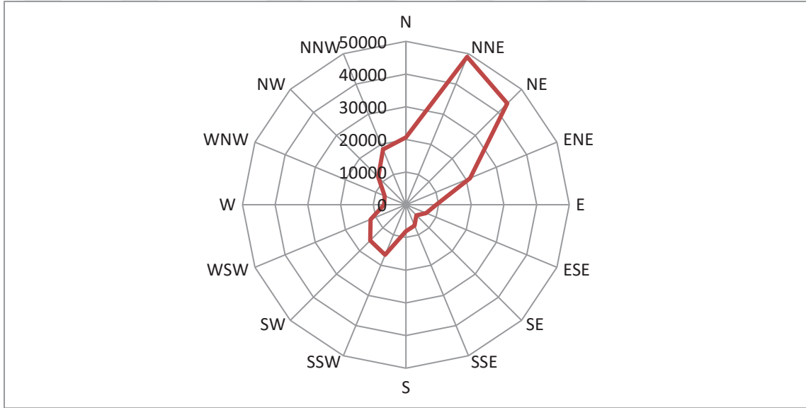
Şekil 6: Rüzgar Güllü Grafiği
