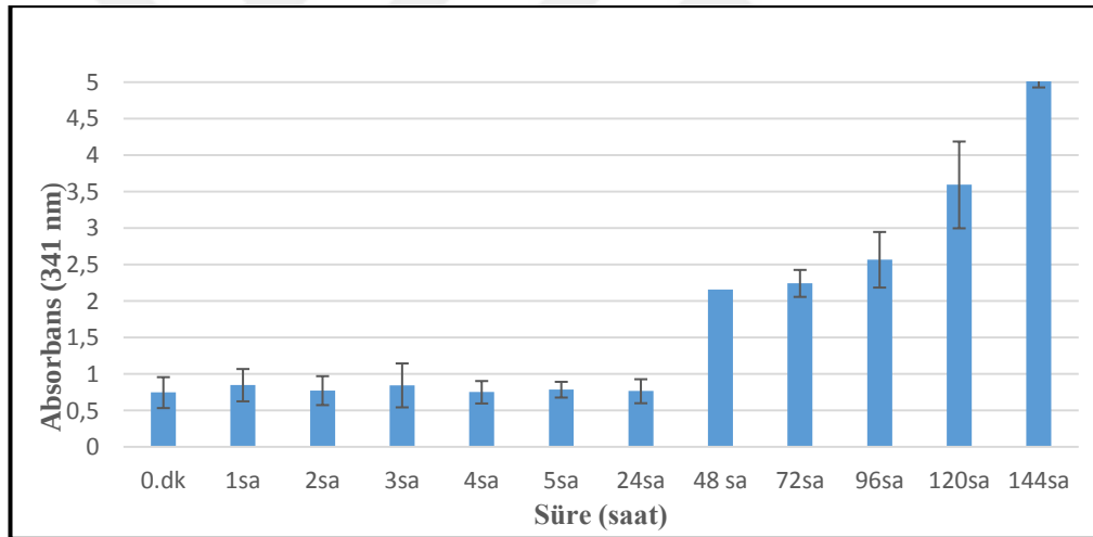
Şekil 4.16. 15 mM \text{TiO}_2 konsantrasyonunda, pH 8 ve 33^\circ\text{C} 'de inkübe edilen örneklerin zamana bağlı \text{TiO}_2\text{NP} üretiminin 341 nm'de ölçülen absorbans değerleri grafiği
