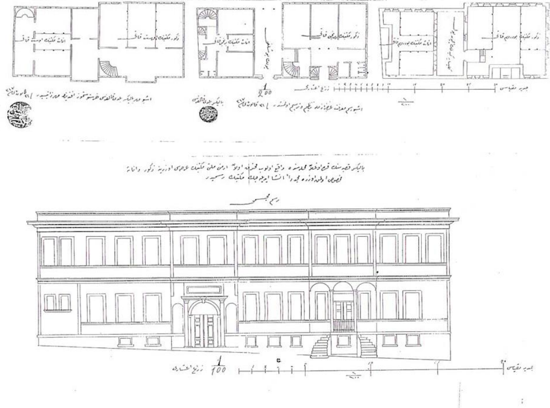
Şekil 2.10 Ermeni Mektebine ait Hristomos Efendi'nin tadilat raporlarında bulunan plan ve cephe çizimleri (Öntuğ, 2006)
