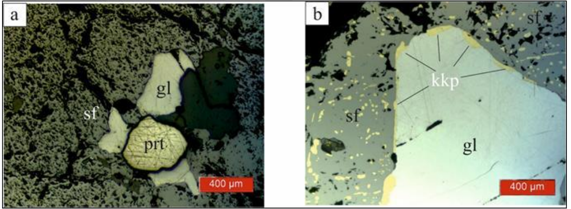
Şekil 7.15: (a) Piriti ornatın galen ile galeni ve piriti ornatın sfalerit, (b) galen çeperini sararak oluşın kalkopirit 2 (prt: pirit, sf: sfalerit, gl: galen, kkp: kalkopirit 1 ve kalkopirit 2) (Kuşcu, 2014).
