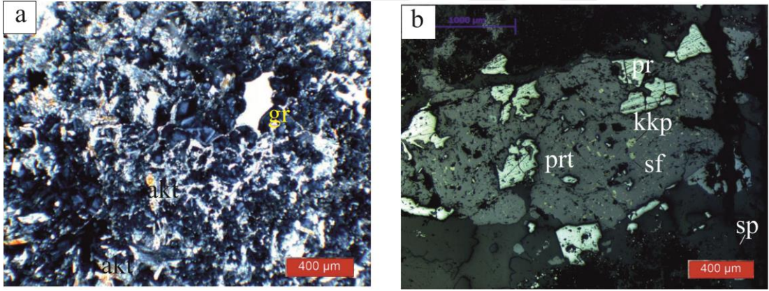
Şekil 7.19: (a) Kısmen karbonatlaşmış granat ve aktinolit, (b) sfalerit içinde yer alan kalkopirit eksolüsyonları ve ornatılmamış pirit adacıkları ve kenar kesimde spekülait (gr: granat, ak: aktinolit, kkp: kalkopirit, prt: pirit, sf: sfelait, sp: spekülait) (Kuşçu, 2014).
