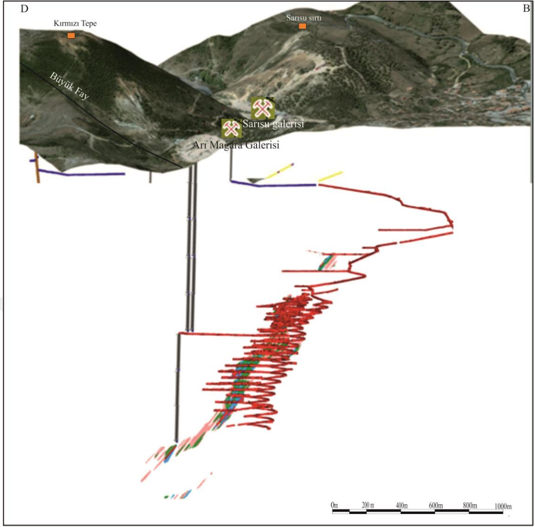
Şekil 7.3: Esan Balya Pb-Zn İşletmesi yeraltı üretim faaliyetlerinin 3 boyutlu bilgisayar programında hazırlanan görüntüsü.
