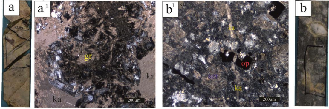
Şekil 7.18: (a-a¹) Prograd evreye ait granatları tamamen silen karbonatlaşma (kalsit 1), (b-b¹) cevher mineralini kesen kalsit 2 damarı (gr: granat, ka: kalsit, op: opak mineral, ser: serizit, a, b: karot numunesi, a¹, b¹: çift nikol) (Kuşçu, 2012).
