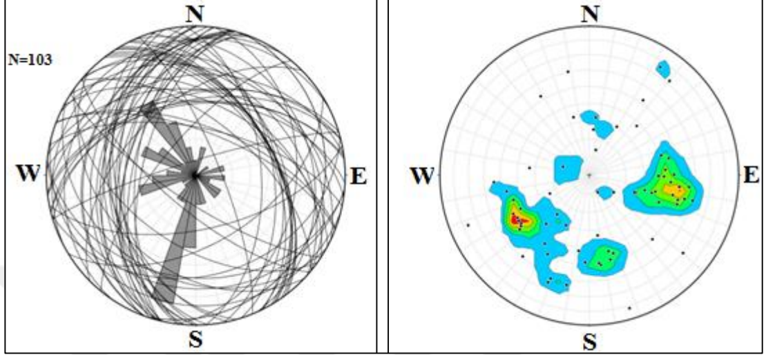
Şekil 5.25: Çatlaklar için hazırlanmış eklem doğrultularını gösteren gül diyagramı (N=103).
