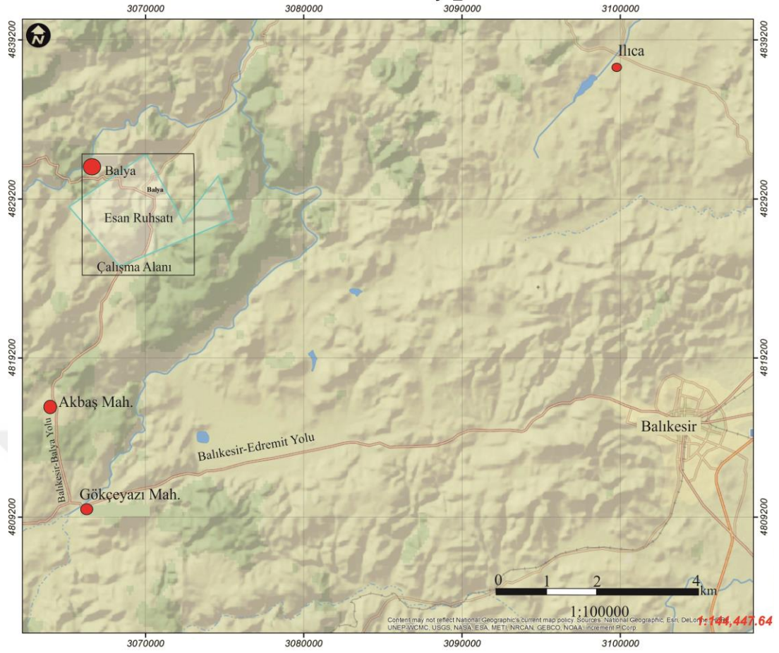
Şekil 1.1: İnceleme alanın yer bulduru haritası.
