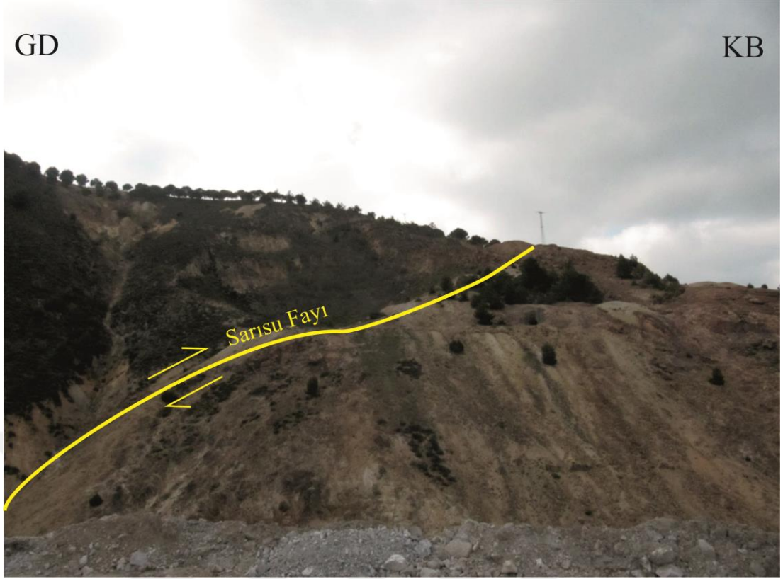
Şekil 5.27: Sarısu Sırtı'ndan geçen sol yanal doğrultu atımlı Sarısu Fayı.
