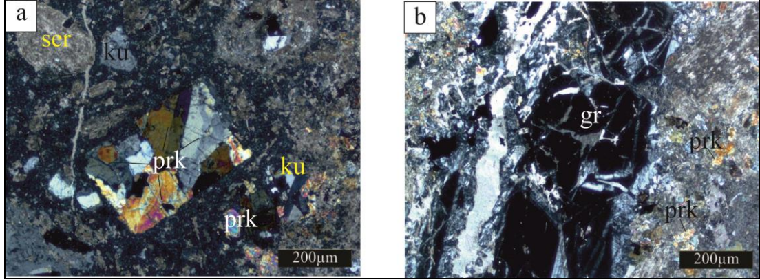
Şekil 7.11: (a) Plajiyoklaz psödomorfları içinde piroksen oluşumları, (b) granat damarı ve çeperler boyunca granatı üzerleyen piroksenler (gr: granat, prk: piroksen, ser: serizit, ku: kuvars) (Kuşcu, 2014).
