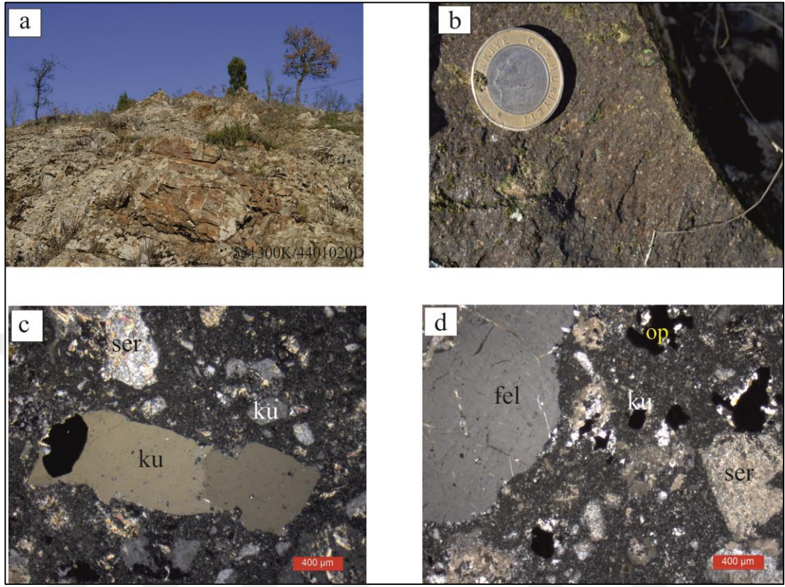
Şekil 5.14: (a), (b) Bahçelerarası Mahallesi’nde Doyuran volkanitlerine ait dasitler, (c) yer yer killeşmiş yarı özşekilli polisentetik ikizli plajiyoklaz ve magmatik kuvars, (d) iri taneli feldispat kenarları serizitleşmiş ve killeşmiş (fel: feldispat, ku: kuvars, op: opak mineral, plj: plajiyoklaz).
