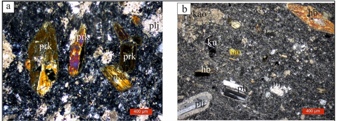
Şekil 5.20: (a) Plajiyoklazlarda killeşme, piroksenlerde opaklaşma, hamurda karbonatlaşma ve opaklaşma, (b) tamamen kaolenleşmiş plajiyoklaz ile kenar kesimleri boyunca hamurda killeşme ve kısmen karbonatlaşma (hb: hornblend, kao: kaolen, plj: plajiyoklaz, prk: piroksen) (Çift Nikol).
