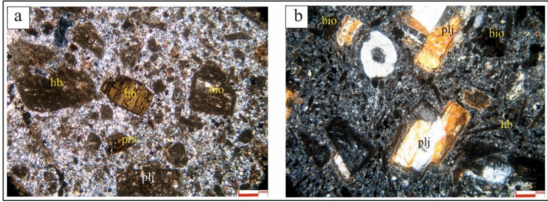
Şekil 5.18: (a) Hornblendelerde ve hamurda opaklaşma (b) plajiyoklaz fenokristalleri ile birlikte hamurda hornblend ve biyotitlerde opaklaşma (bi: biyotit, hb:hornblend, plj: plajiyoklaz).
