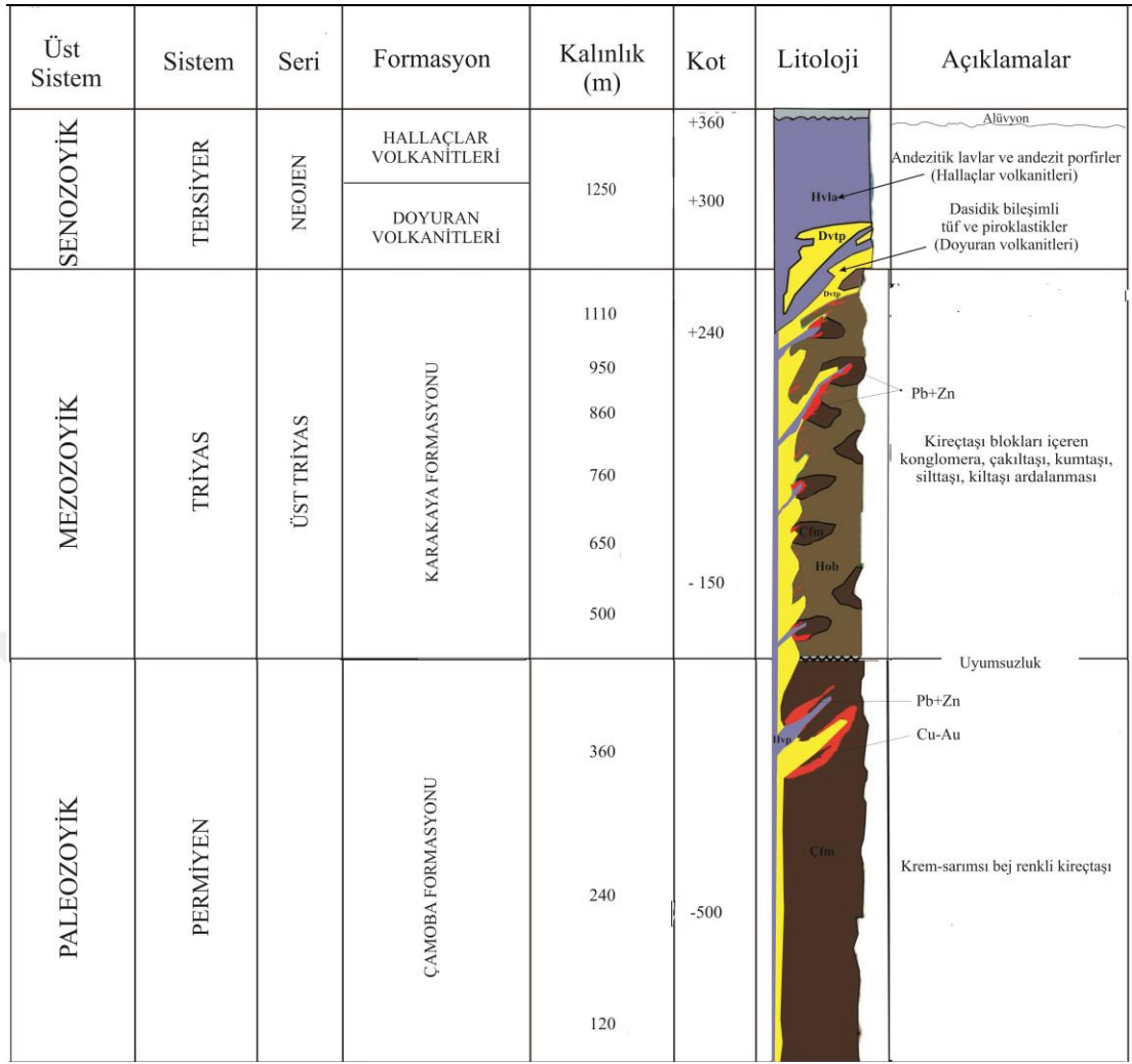
Şekil 5.2: İnceleme alanının genelleştirilmiş stratigrafik kolon kesiti (Akyol, 1977'den revize edilmiştir).
