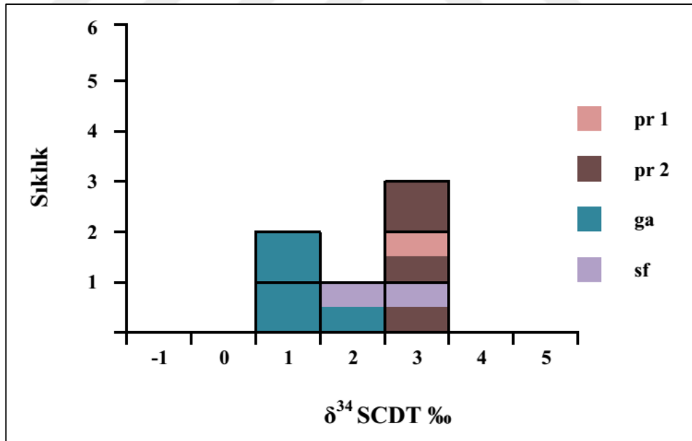
Şekil 9.1: Galen (ga), sfalerit (sf) ve pirit (pr) minerallerine ait \delta^{34}\text{S} CDT‰ frekans dağılımları.
