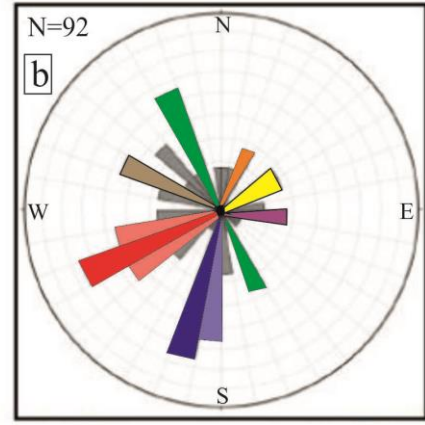
Şekil 7.21: (a) Sondaj kuyularında oryantasyon cihazı ile ölçülen sülfid mineral damarlarına ait gül diyagramı (her baskın yön farklı renk kodu ile gösterilmektedir), (b) sondaj kuyularında oryantasyon cihazı ile ölçülen geç evre karbonatları ile ilişkili pirit damarlarına ait gül diyagramı (her baskın yön farklı renk kodu ile gösterilmektedir).
