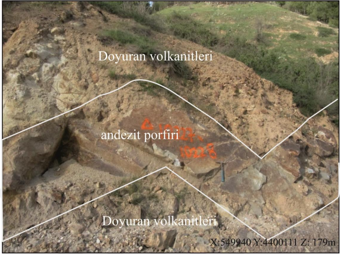
Şekil 5.19: Hallaçlar volkanitlerine ait andezit porfir daykısı.
