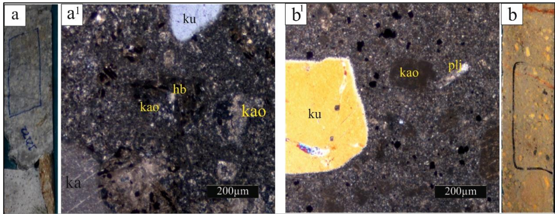
Şekil 7.16: (a-a¹) Dasit porfir dokusunu tamamen silen, killeşme, karbonatlaşma ve hepsini kesen kalsit 2 (b-b¹) Yaygın killeşmeye maruz kalmış dasit porfir (hb: hornblend, ka: kalsit, kao: kaolen, ku: kuvars, plj: plajiyoklaz, a, b: karot numunesi, a¹, b¹: çift nikol) (Kuşcu, 2012).
