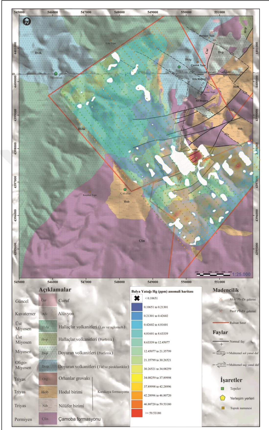
Şekil 8.7: Balya Pb-Zn Yatağı'ndaki toprak numunelerinin Hg element (ppm) dağılım haritası.
