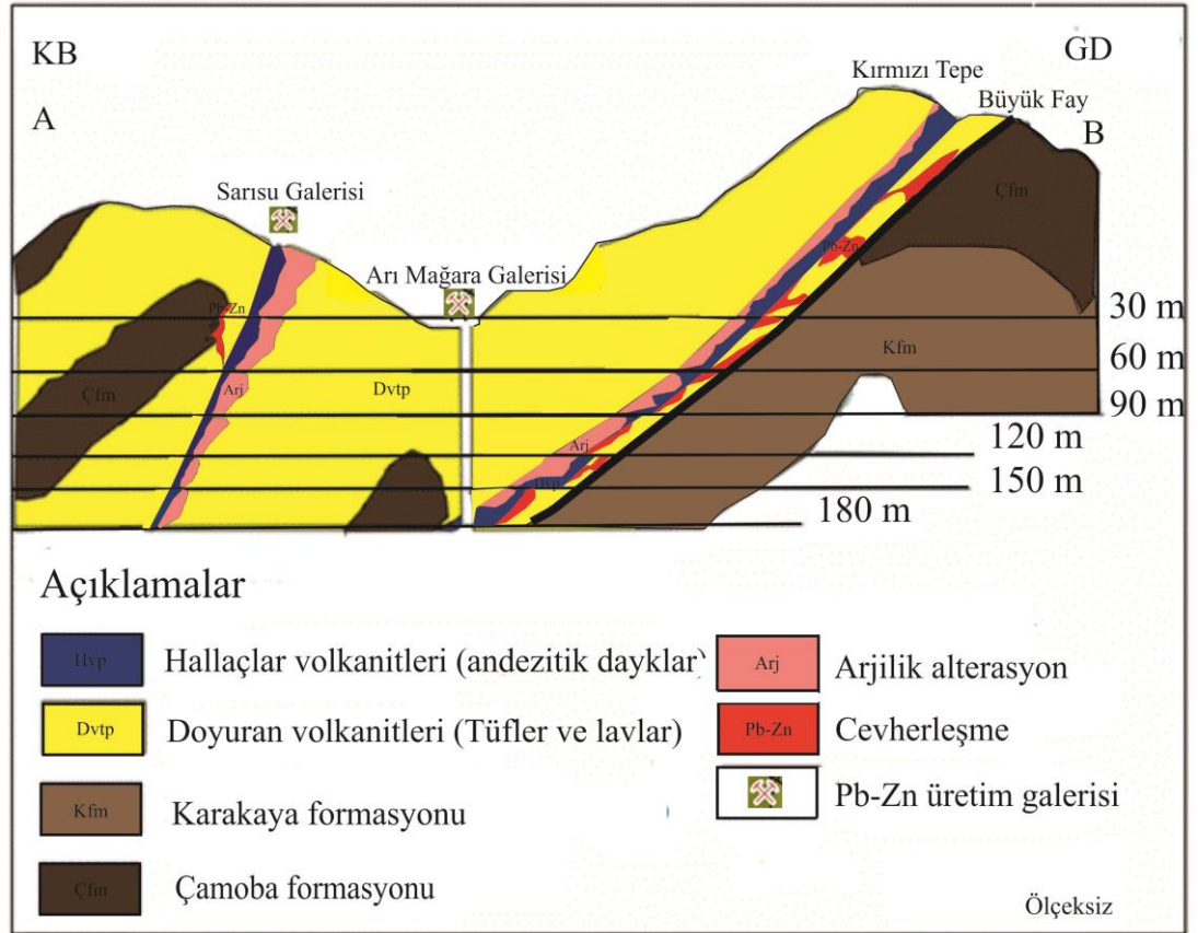
Şekil 7.7: Kırımızı Tepe ile Sarısu Galerisi arasının genelleştirilmiş enine kesiti üzerinde cevher-yankayaç ilişkileri (Kovenko 1940'dan revize edilmiştir).
