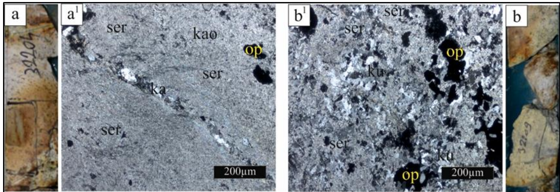
Şekil 7.9: (a-a') Killeşmiş kayacı ve serizitleşmiş plajiyoklazları kesen karbonat damarcığı, (b-b') killeşmiş dasit porfiri kesen kuvars pirit damarcığı (ku: kuvars, op: opak mineral, ser: serizit, a,b: karot numunesi, a'-b': çift nikol).
