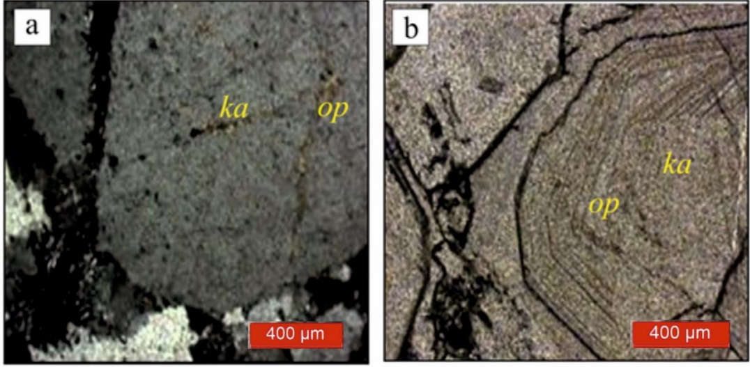
Şekil 5.5: (a), (b) Çamoba formasyonuna ait kireçtaşı polarizan mikrokobu görüntüsü (ka: kalsit, op: opak mineral) (Çift Nikol).
