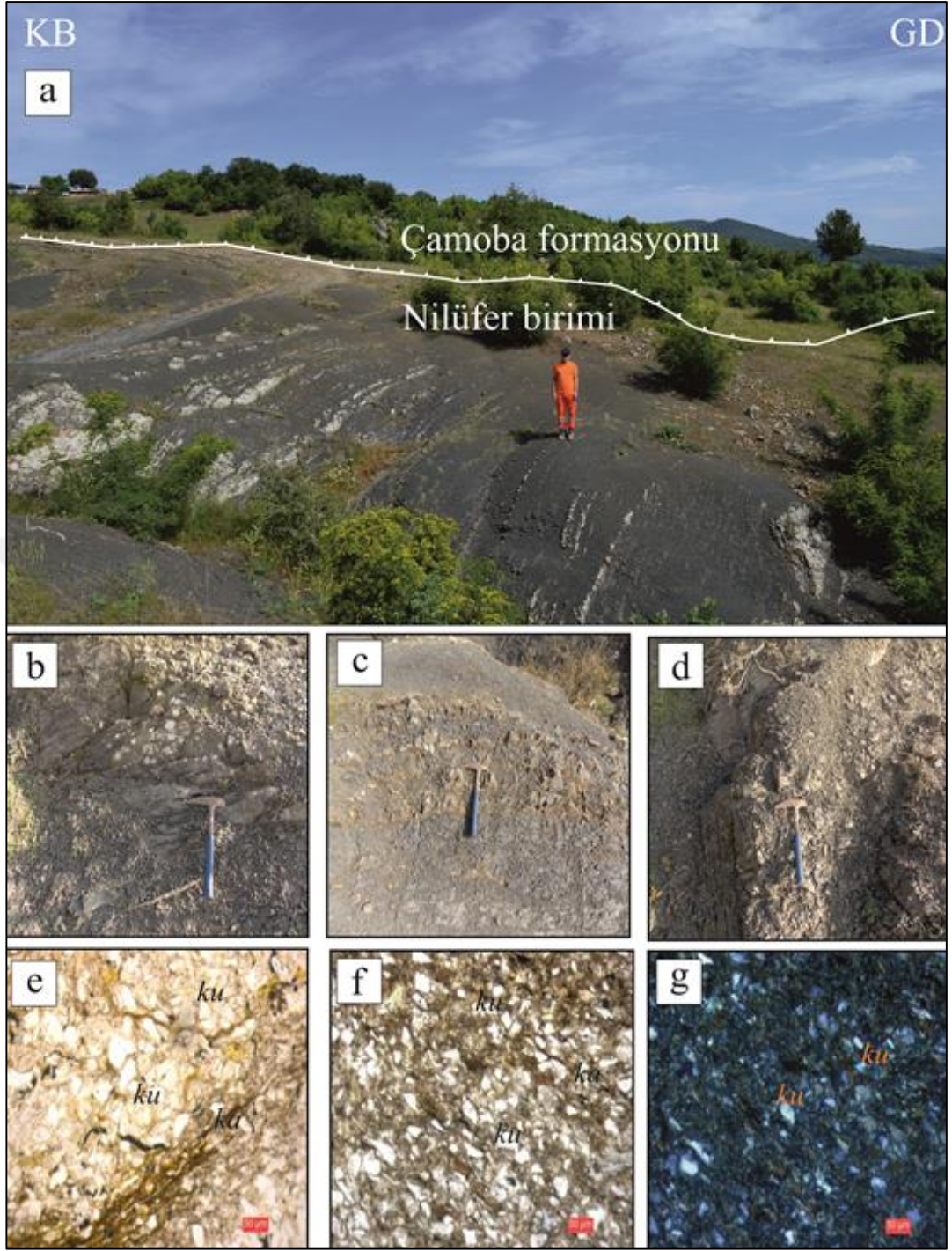
Şekil 5.6: (a) Nilüfer birimi ile Çamoba formasyonu arasındaki mekânsal ilişki, (b) metaçamurtaşı-fillat ardalanması, (c) fillat-çamurtaşı, (d) fillat-çamurtaşı, (e) ince taneli fillat (tek nikol), (f) ince taneli fillat ile yer yer killi siltli çamurtaşı (tek nikol), (g) fillat-çamurtaşı (çift nikol).
