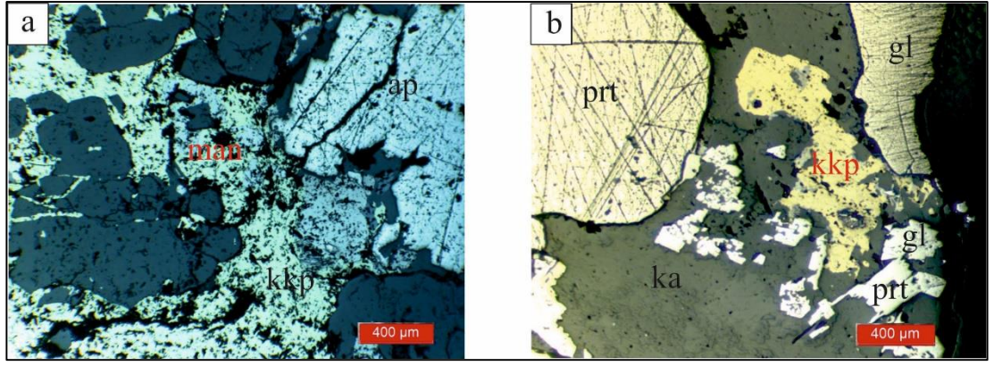
Şekil 7.14: (a) Kalkopirit 1 ve manyetitler tarafından ornatılan arsenopiritler, (b) kalkopiriti ornatın pirit 1 ve ikisini de ornatın galen (ap: arsenopirit, man: manyetit, kkp: kalkopirit, prt: pirit, gl: galen, ka: kalsit, a, b: karot numunesi, a 1 , b 1 : çift nikol) (Kuşcu, 2014).
