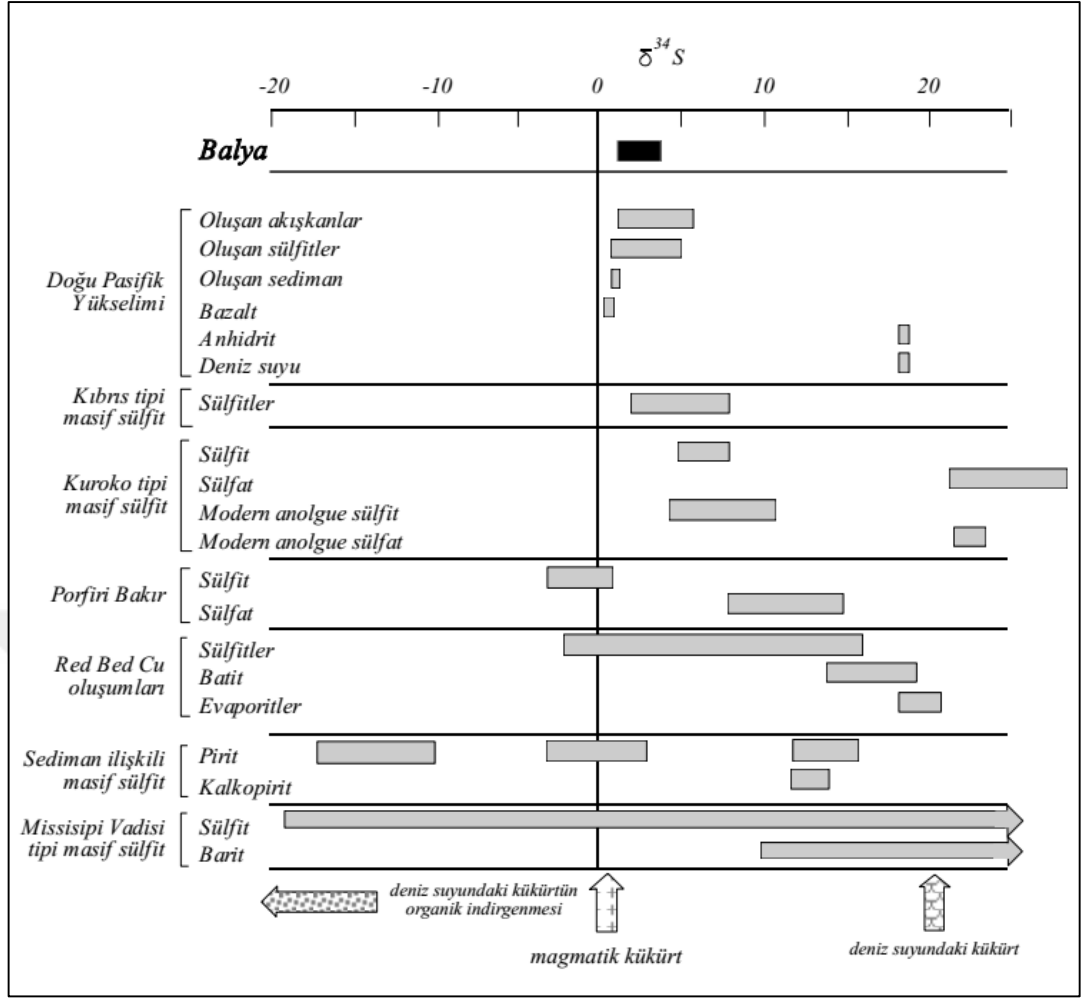
Şekil 9.2: Hidrotermal maden yataklarında kükürt içeren minerallerin \delta^{34}S değerleri ve Balya Yatağı'na ait \delta^{34}S değerlerinin dağılımı (Kerridge vd. (1983), Ohmoto ve Rye (1979), Halbach vd. (1989), Naylor vd. (1989) ve Eldridge vd. (1988) çalışmalarını derleyen Rollinson, 1993'den alınmıştır).
