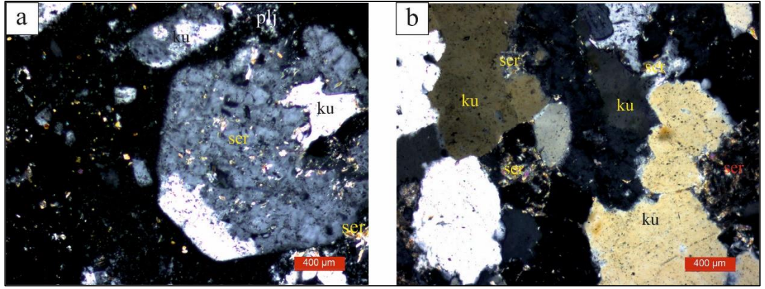
Şekil 5.15: (a), (b) Feldispatlarda yoğun serizitleşme ve killeşme (ku: kuvars, plj: plajiyoklaz, ser: serizit) (Çift Nikol).
