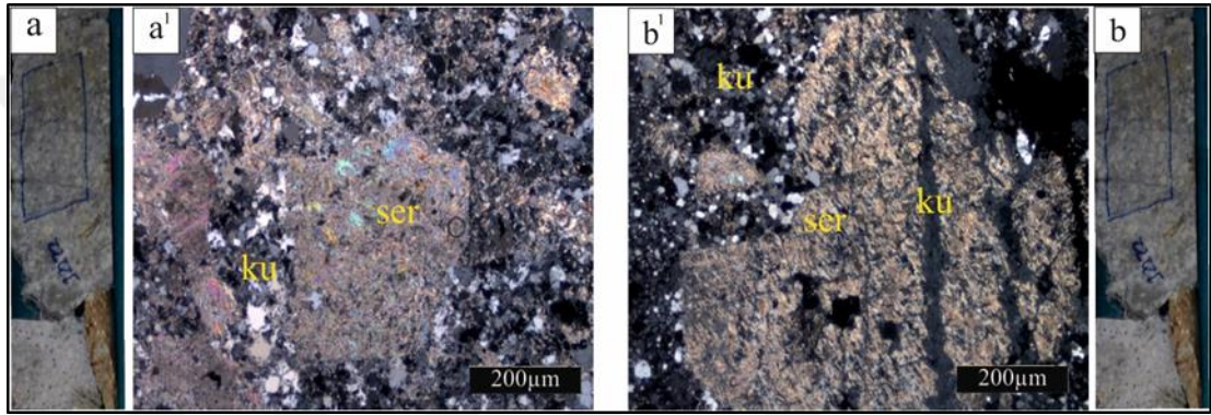
Şekil 7.8: (a-a') Serizitleşmiş killeleşmiş dasit porfir klastı, (b-b') serizitleşmeyi üzerleyen silisleşme ve kuvars damarcıkları (ku: kuvars, ser: serizit, a,b: karot numunesi) (a'-b': çift nikol).
