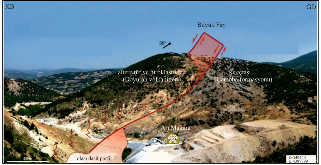
Şekil 5.26: Eğim atımlı normal fay karakterindeki Büyük Fay (Matias, 2012).
