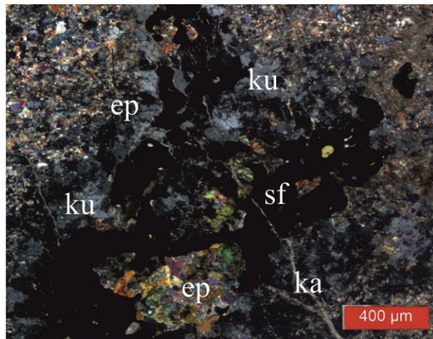
Şekil 7.17: Ortopiroksenleri ornatın epidotlar, onları da ornatın kuvarslar, aktinolitleşme ve sülfid mineral ornatmaları (ep: epidot, ka: kalsit, ku: kuvars, sf: sfalerit ) (Kuşcu, 2012).
