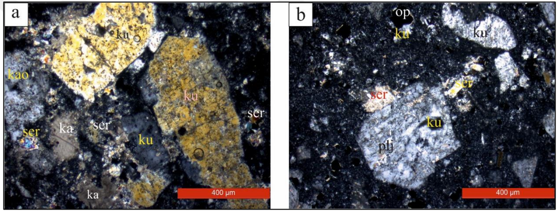
Şekil 5.13: (a) Feldspatları killeşmiş, hamuru silisleşmiş ve karbonatlaşmış dasidik tüf, (b) plajiyoklazları serizitleşmiş ve kısmen karbonatlaşmış hamuru silisleşmiş dasidik piroklastik (kao: kaolen, ka: kalsit, ku:kuvars, plj: plajiyoklaz, ser: serizit) (Çift Nikol).
