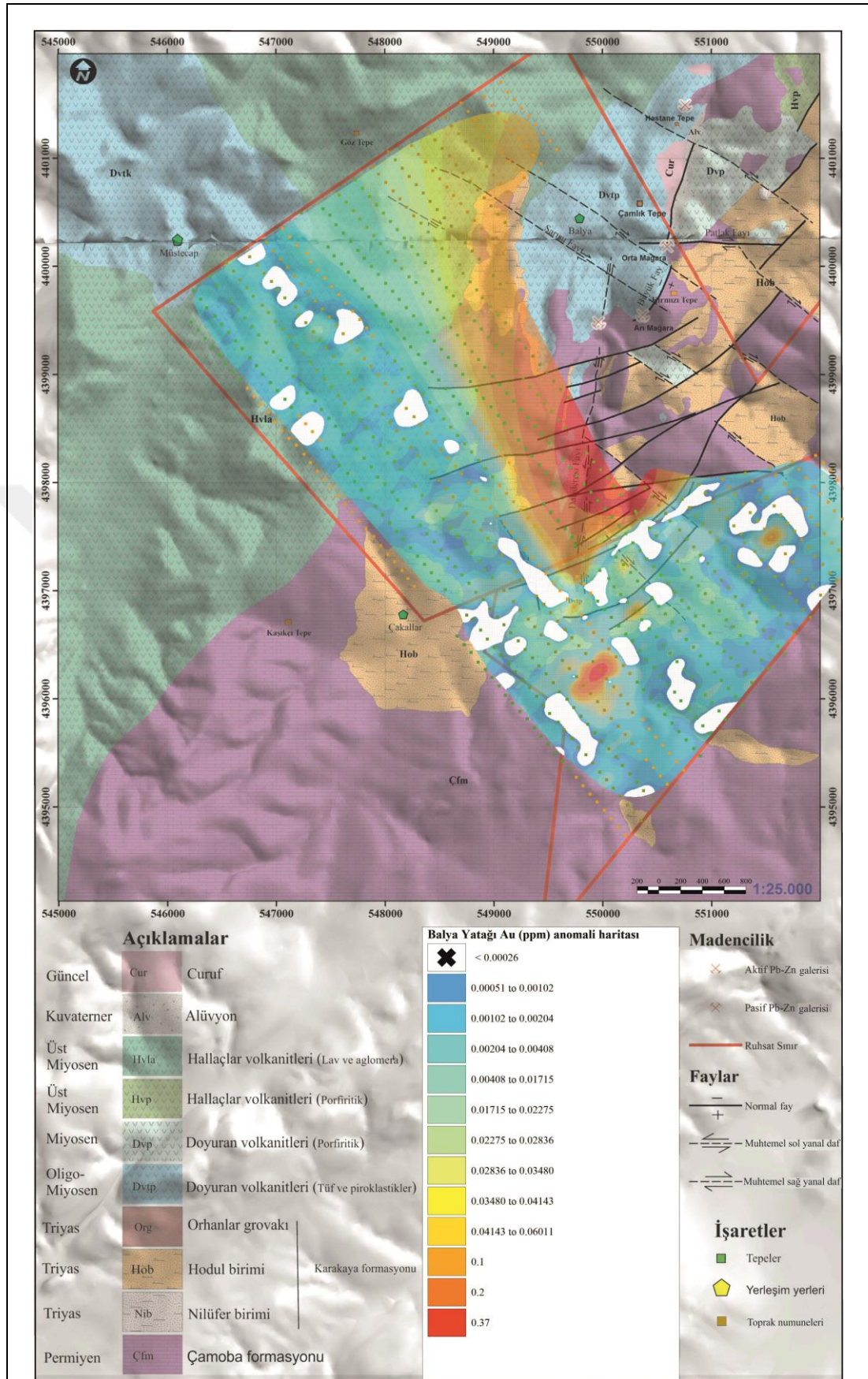
Şekil 8.8: Balya Pb-Zn Yatağı'ndaki toprak numunelerinin Au element(ppm)dağılım haritası.
