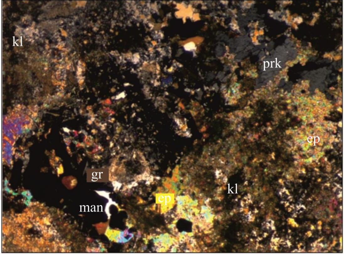
Şekil 7.12: Granatları ve piroksenleri üzerleyen epidotlaşma ve kloritleşmeler ile birlikte özşekilsiz manyetitler (ep: epidot, grt: granat, kl: klorit, prk: piroksen, man: manyetit) (Kuşcu, 2014).
