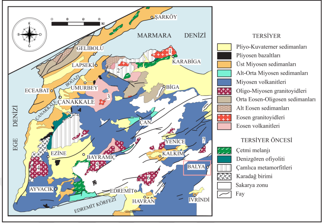
Şekil 4.1: Biga Yarımadası'nın genelleştirilmiş jeoloji haritası (1) Karabiga, (2) Şevketiye, (3) Kuşçayırı, (4) Ezine, (5) Bayramiç, (6) Eybek ve (7) Karacadağ granitoyidleri (Demirela vd., 2014).
