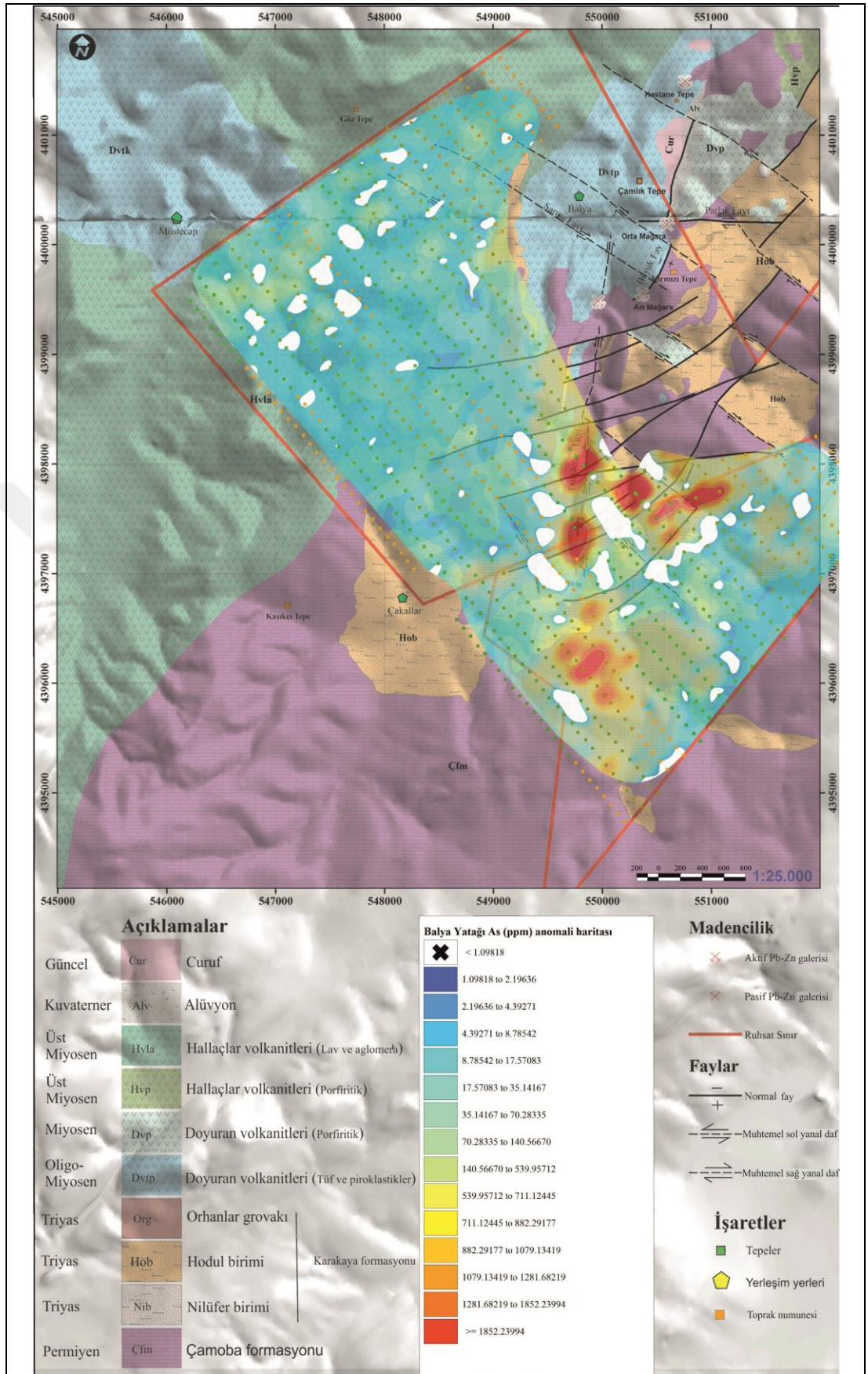
Şekil 8.5: Balya Pb-Zn Yatağı'ndaki toprak numunelerinin As element (ppm) dağılım haritası.
