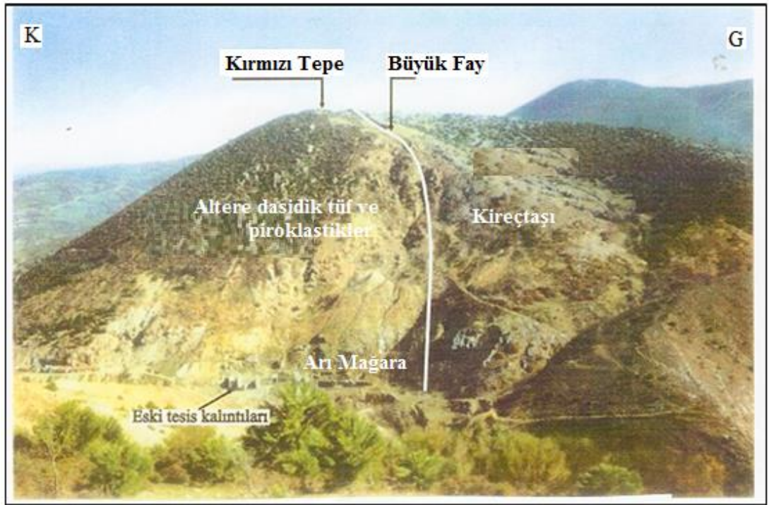
Şekil 7.5: Kırmızı Tepe üzerinden geçen Büyük Fay (Doyuran volkanikleri ile Çamoba formasyonu arasındaki tektonik dokanak) (Yıl: 2002).
