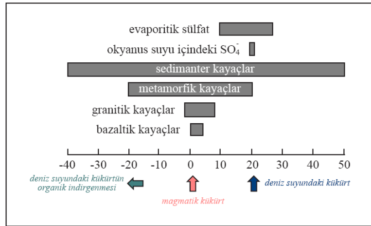
Şekil 9.3: Çeşitli kayaç gruplarının \delta^{34}S değerleri ile evaporitik ve okyanus suyu içindeki sülfatların \delta^{34}S değerleri (Hoefs, 1987'den alınmıştır)
