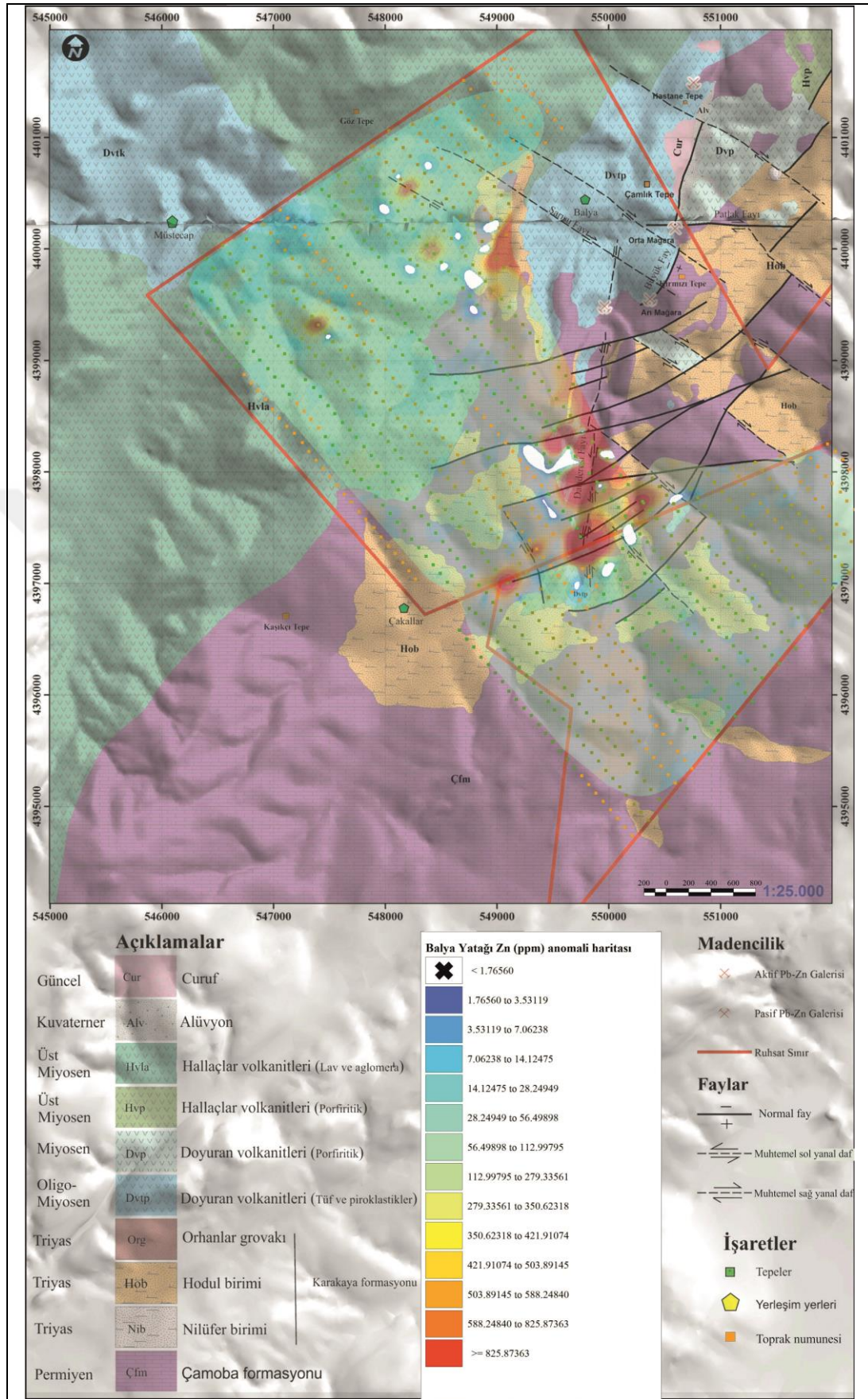
Şekil 8.2: Balya Pb-Zn Yatağı'ndaki toprak numunelerinin Zn element (ppm) dağılım haritası.
