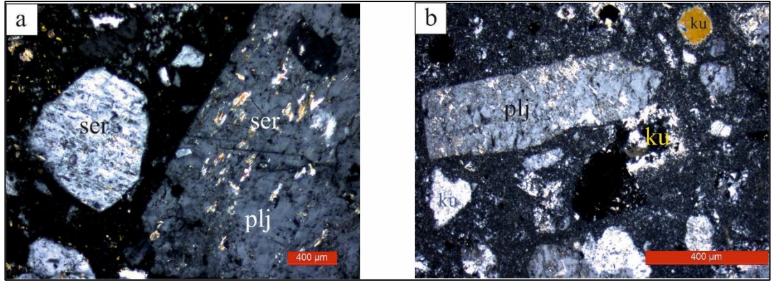
Şekil 5.12: (a) Polisentetik ikizlenme gösteren plajiyoklazlarda serizitleşme, (b) plajiyoklazlarda serizitleşme, hamurda serizitleşme ve magmatik kuvarslar (plj: plajiyoklaz, ku:kuvars, hb:hornblend, ser: serizit) (Çift Nikol).
