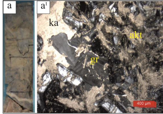
Şekil 7.13: (a-a¹) Granatlarda aktinolitleşmeler ile birlikte aktinolitlerde karbonatlaşma (gr: granat, ka: kalsit, akt, a: karot numunesi, a¹: çift nikol) (Kuşcu, 2012).
