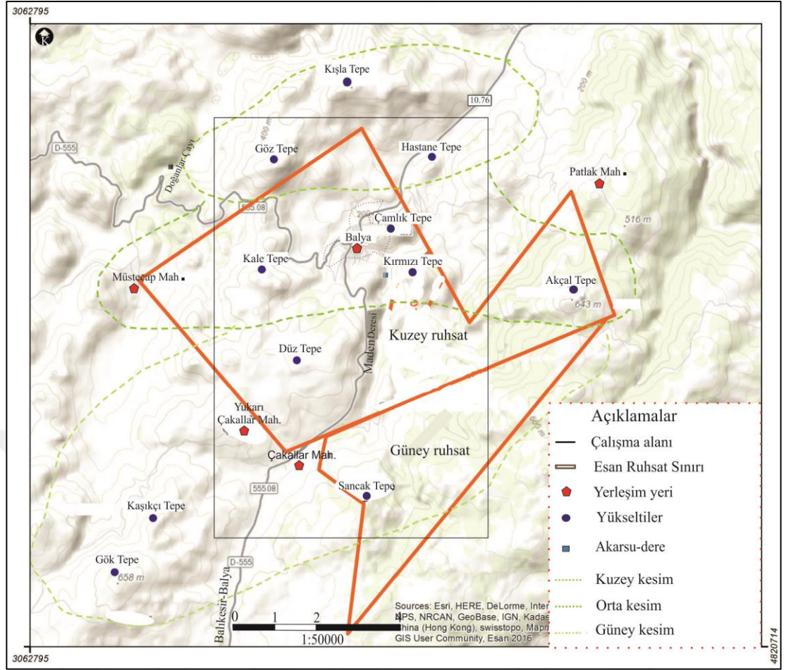
Şekil 1.2: İnceleme alanının 1/25000 ölçekli Google Earth ve DEM haritalarından üretilmiş topografik haritası.
