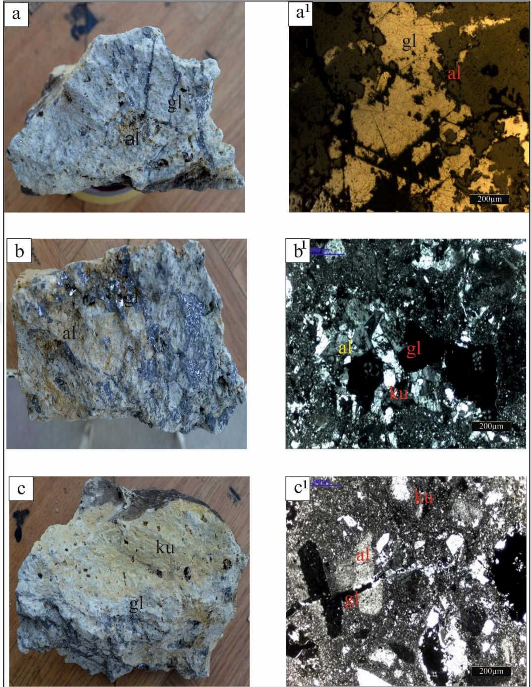
Şekil 7.10: (a-a¹) Boşluk dolgusu şeklindeki galen oluşumları, (b-b¹) kovuklu yapılu kuvars ve boşluk dolgusu şeklinde ortaya çıkmış galen ile Na-alunit veya plajiyoklazlar (c-c¹) kovuklu yapıyı dolduran Na-alunit ve kısmen silisleşmiş mikro fay oluşumları, boşukları dolduran galen (ku: kovuklu kuvars, gl: galen, al: alunit, a, b: karot numunesi, a¹, b¹: çift nikol) (Kuşcu 2015).
