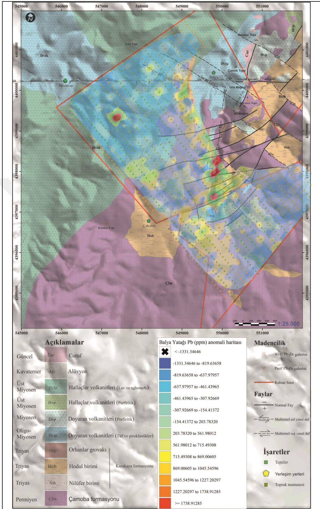
Şekil 8.1: Balya Pb-Zn Yatağı'ndaki toprak numunelerinin Pb element (ppm) dağılım haritası.
