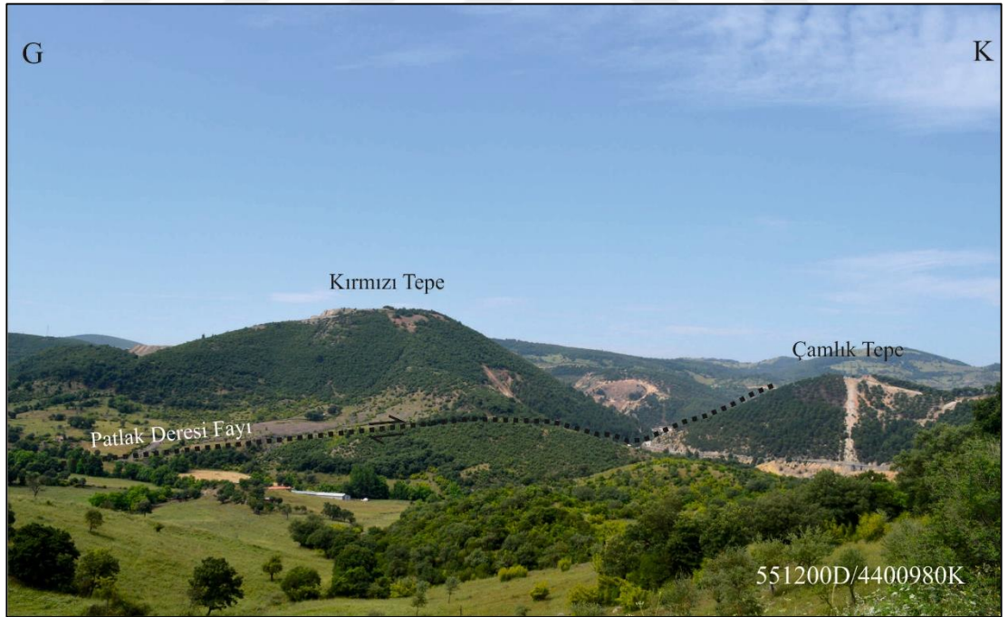
Şekil 5.28: Patlak Mahallesi'nin batısından geçen yaklaşık D-B yönlü sağ yanal doğrultu atımlı Patlak Deresi Fayı'na ait görünüm.
