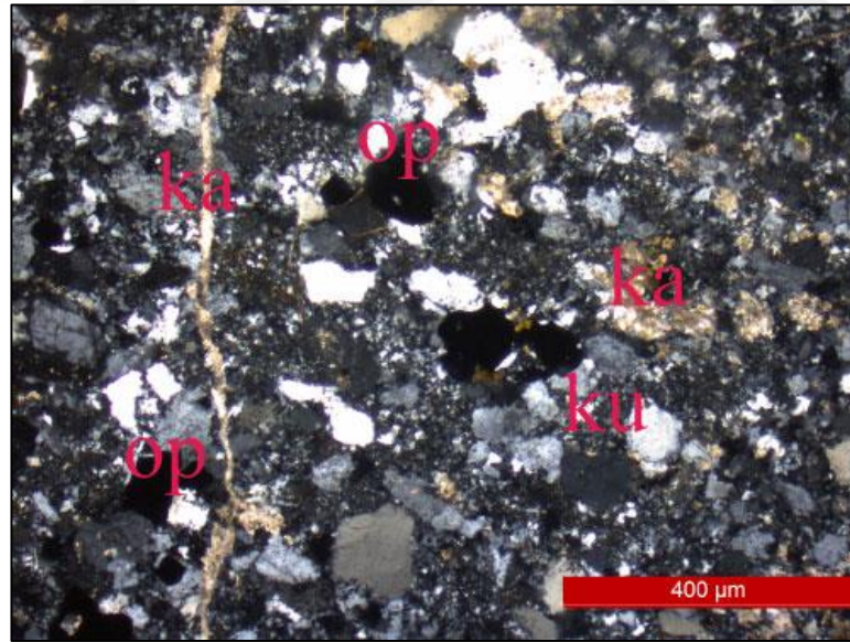
Şekil 5.16: Dasit içinde karbonatlaşma, ikincil kalsit damarı, kısmen silisleşme ve opak mineral saçınımları (Çift Nikol).
