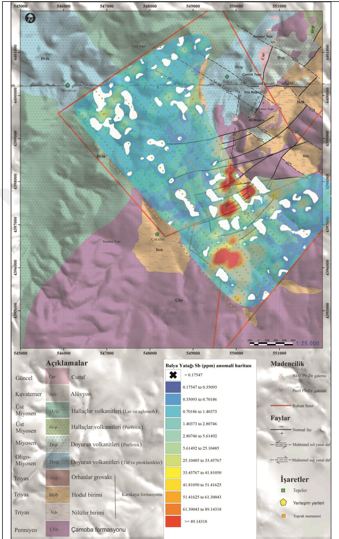
Şekil 8.6: Balya Pb-Zn Yatağı'ndaki toprak numunelerinin Sb element (ppm) dağılım haritası.
