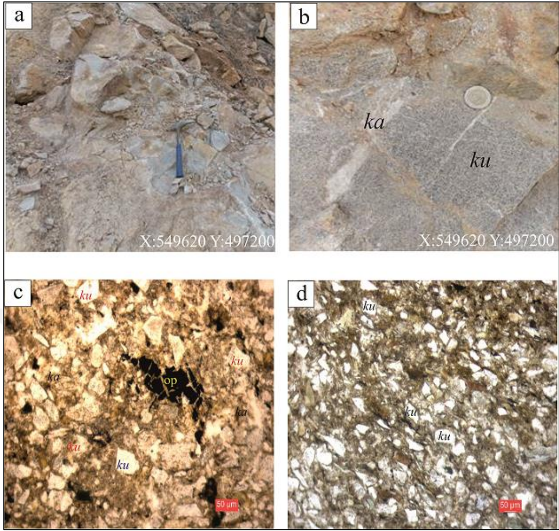
Şekil 5.8: (a) Orhanlar grovakına ait çakıltaşlarının genel görünümü, (b) Orhanlar grovakını kesen kalsit damarı, (c) çakıltaşları içerisinde yer yer silttaşı - kumtaşı klastları (çift nikol), (d) kumtaşlarında kataklastik deformasyon izleri. (ku: kuvars, ka: kalsit, op: opak).
