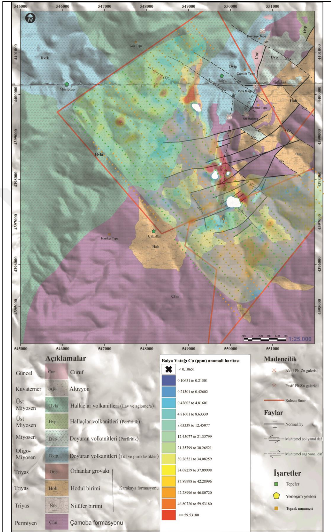
Şekil 8.4: Balya Pb-Zn Yatağı'ndaki toprak numunelerinin Cu element (ppm) dağılım haritası.
