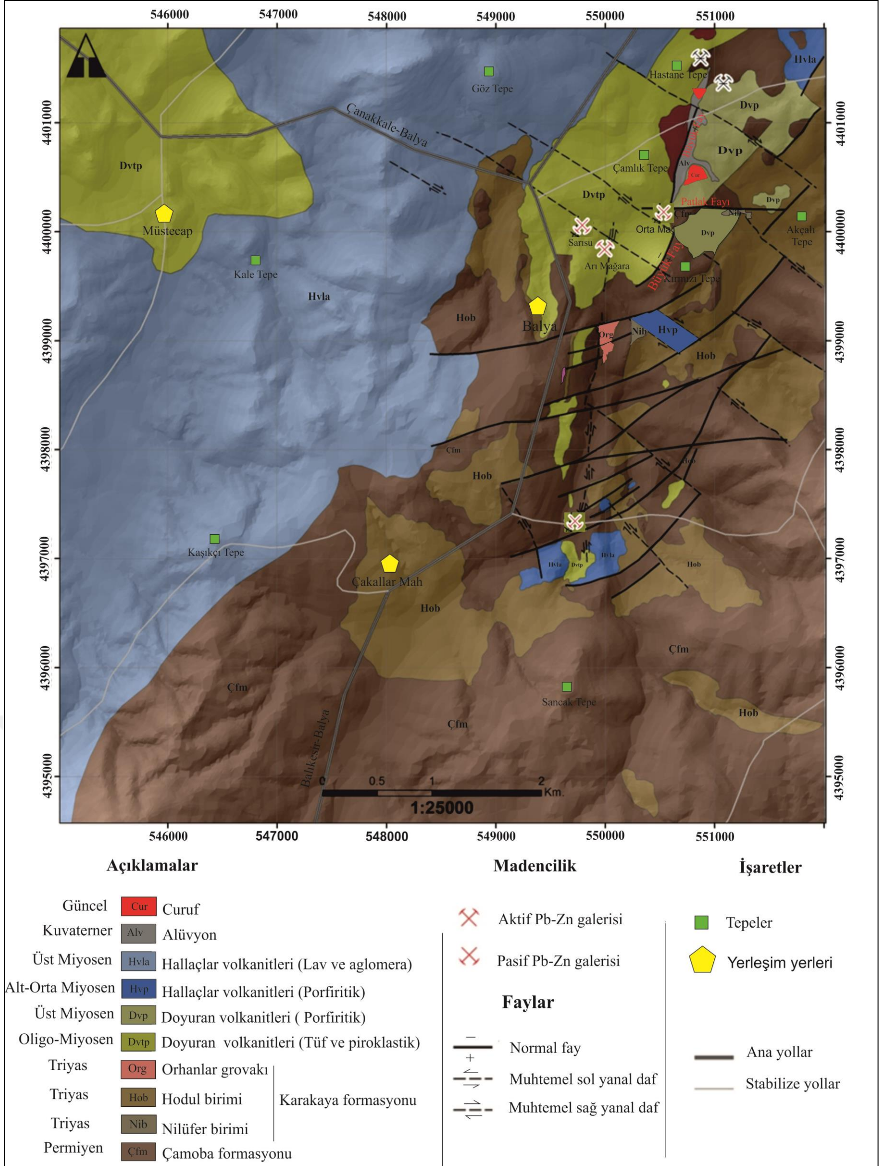
Ek-A: İnceleme alanının 1/25000 ölçekli genel jeoloji haritası.
