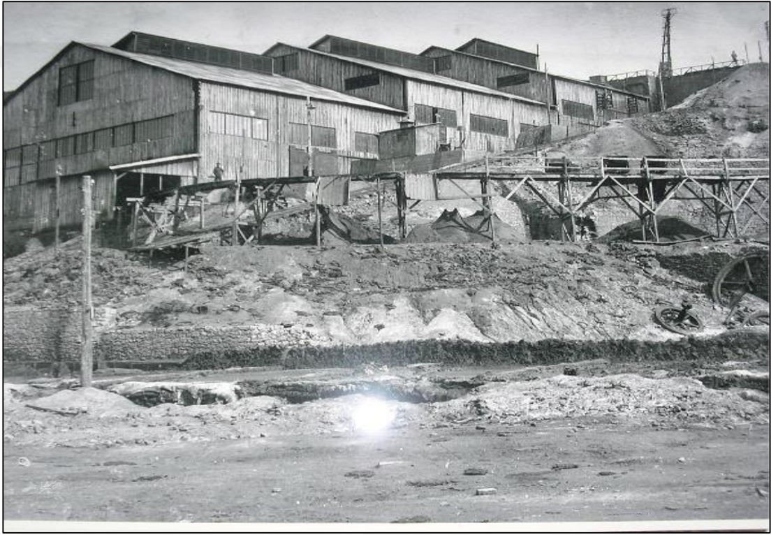
Şekil 7.2: Balya Madeni içinde Fransız Dönemi ne ait izabe tesisi (Yıl:1904).
