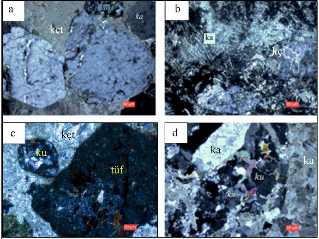
Şekil 5.23: (a), (b) Traverten içerisinde karbonatlı kırıntılı kayaç parçaları, (c) traverten içerisinde dasitik tüf klastları, (d) traverten içerisinde kuvars kapanımları (ka: kalsit, ku: kuvars, kçt: kireçtaşı klastı) (Çift nikol).
