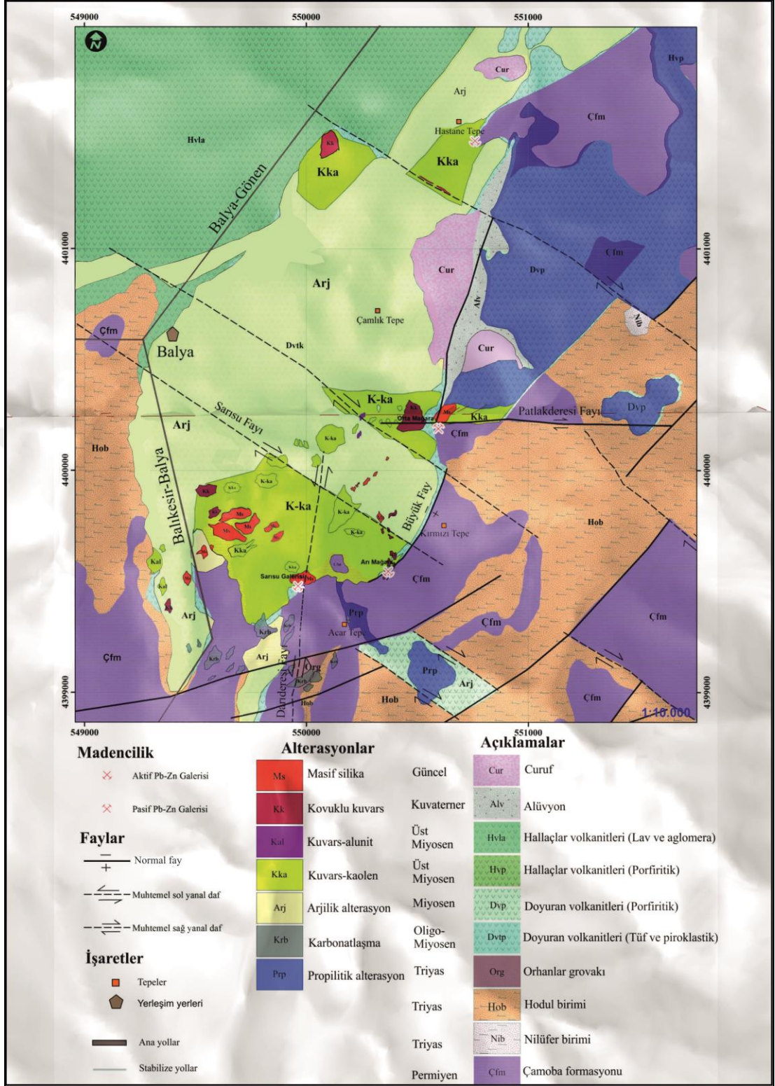
Şekil 7.4: İnceleme alanının maden jeolojisi haritası (ayrıntılar için Ek-B'ye bakınız).
