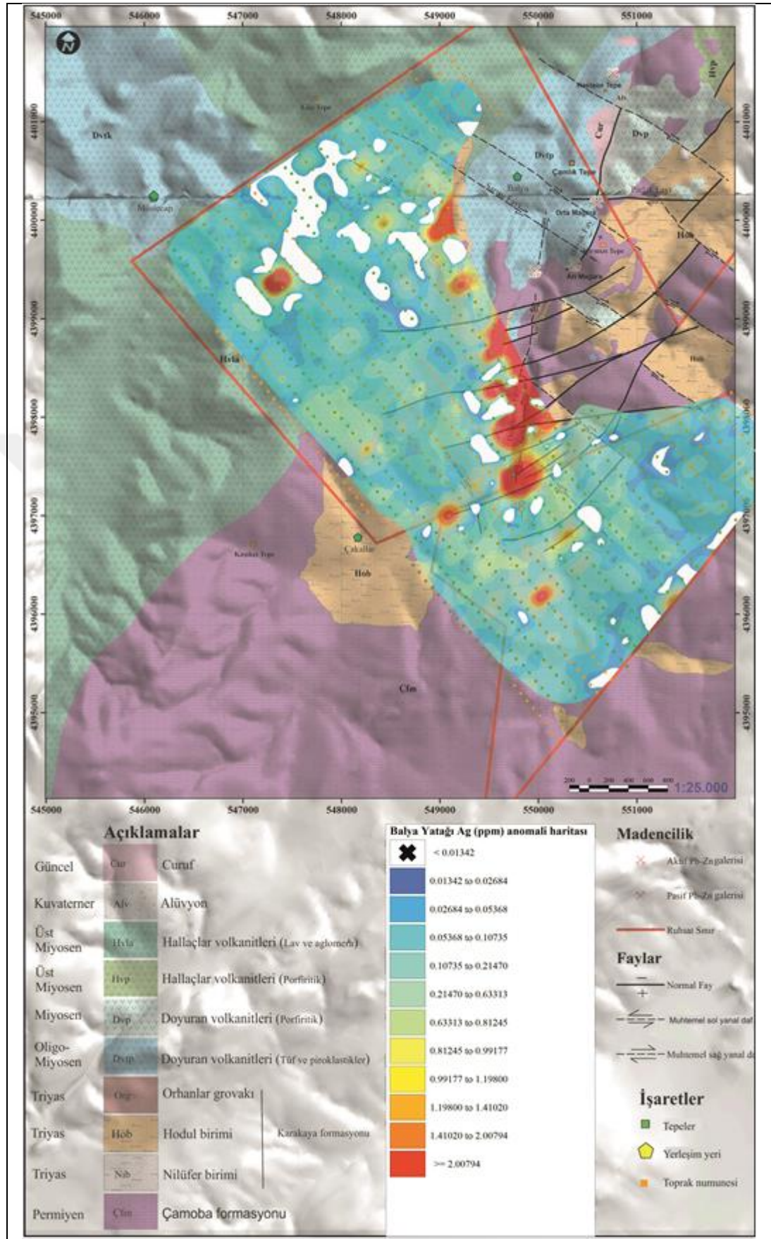
Şekil 8.3: Balya Pb-Zn Yatağı'ndaki toprak numunelerinin Ag element (ppm) dağılım haritası.
