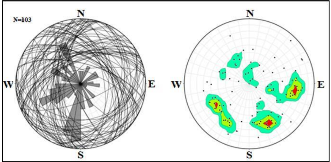
Şekil 7.20: Sülfid minerali içeren damarlar için hazırlanmış damar yönlerini (doğrultularını) gösteren gül diyagramı (N=103).
