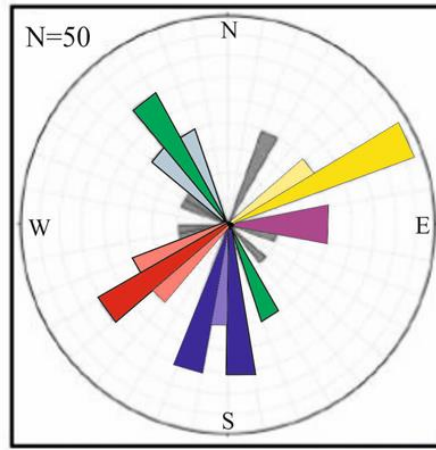
Şekil 7.22: Sondaj kuyularında oryantasyon cihazı ile ölçülen geç evre karbonat (kalsit 1 ve kalsit 2) damarlarına ait gül diyagramı (her baskın yön farklı renk kodu ile gösterilmektedir).
