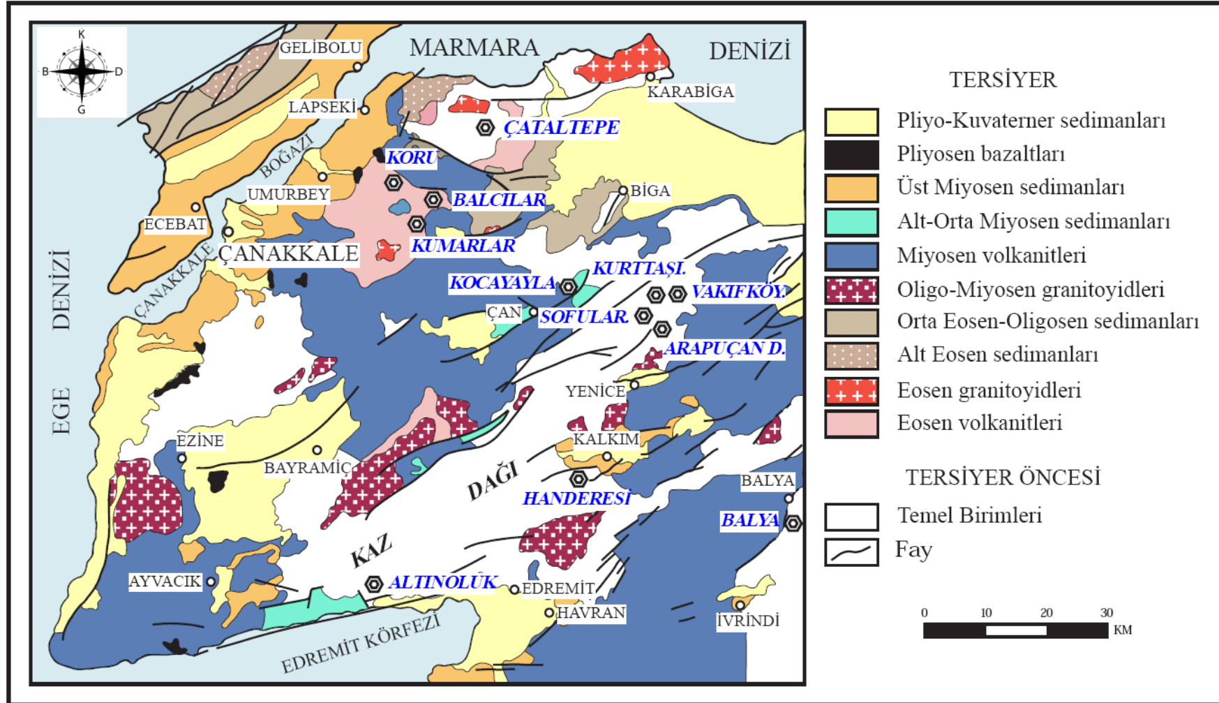
Şekil 6.1: Biga Yarımadası'nda yer alan Pb-Zn cevherleşmeleri (Demirela 2011).
