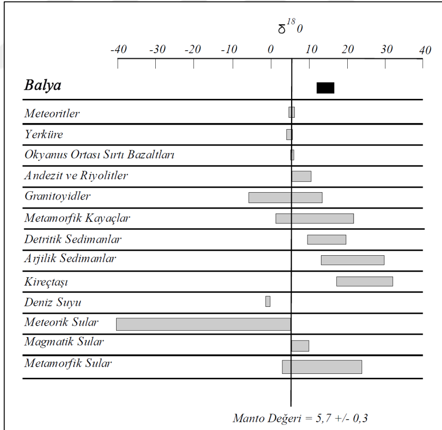
Şekil 9.4: Çeşitli kayaç gruplarının ve suların \delta^{18}\text{O} değerleri ve Balya Yatağı'na ait \delta^{18}\text{O} değerlerinin dağılımı (Rollinson, 1993'den aynen alınmıştır).
