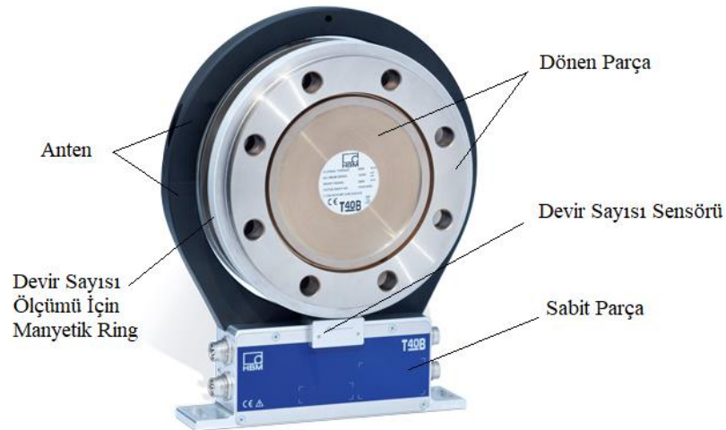
Şekil 4.9. Torkmetre parçaları
