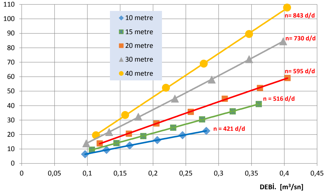
Şekil 5.1. Debiye Bağlı Güç Değişimi (10m, 15m, 20m, 30m, 40m Düşülerde)
