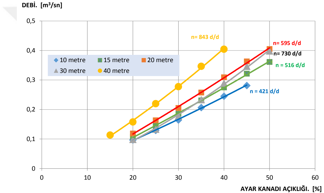
Şekil 5.5. Ayar kanadı açıklığına bağlı debi değişimi (10m, 15m, 20m, 30m, 40m düşülerde)
