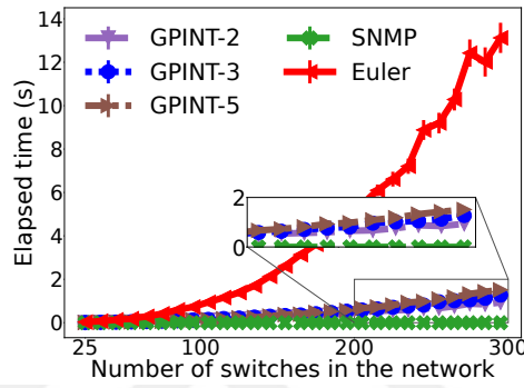
(d) Time to generate a solution
