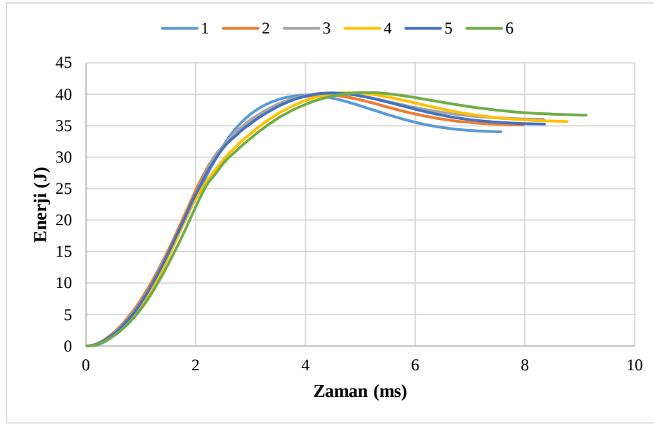
Şekil 4.4. 40 J için enerji-zaman grafiği
