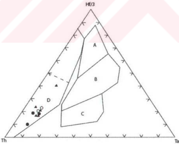
Şekil 4.10. İnceleme alanındaki mafik magmatik kayaların Hf-Th-Ta diyagramında (Wood, 1980) dağılımı. Alanlar Şekil 4.9'daki, Simgeler Şekil 4.1'deki gibidir.
