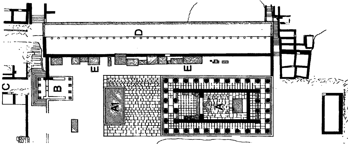
Şekil 4.11 Priene Kenti Athena Polias Tapınağı ( A- Tapınak , A1-Sunak , B Propylon , C-Athena Caddesi , D- Dorik Stoa )
