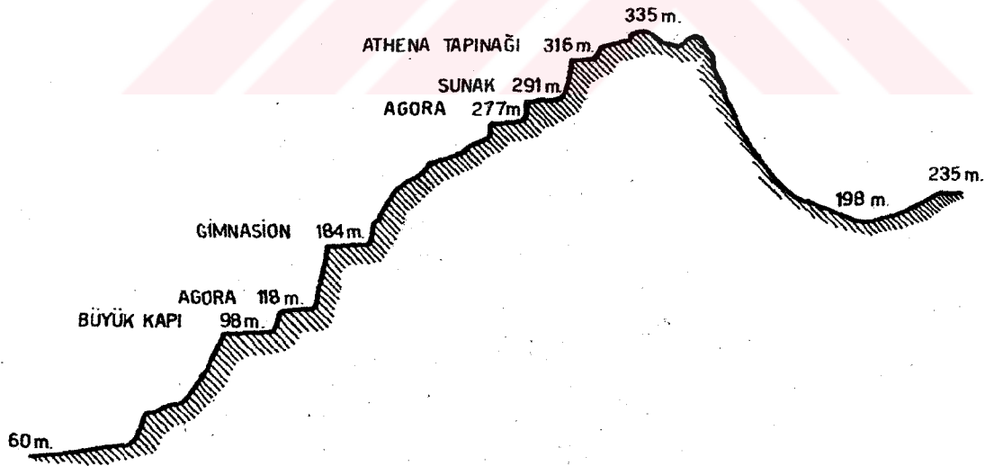
Şekil 5.29 Pergamon Kenti Arazisi
