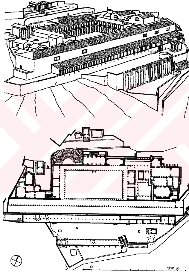
Şekil 5.42 Pergamon Kenti Aşağı Gymnasium Plan ve Aksonometri (W.RADT, 1989, Tafel : 29)
