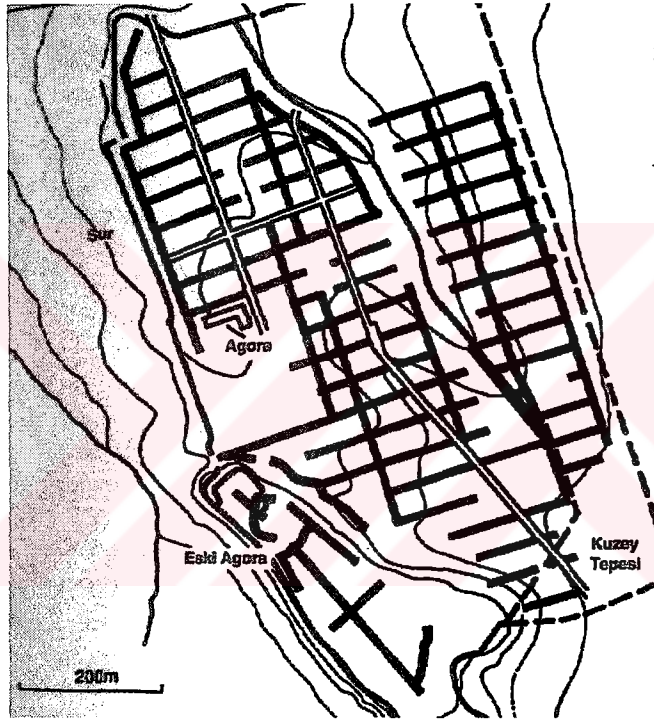
Şekil 3.15 Olinthos Kenti Sokak Dokusu
