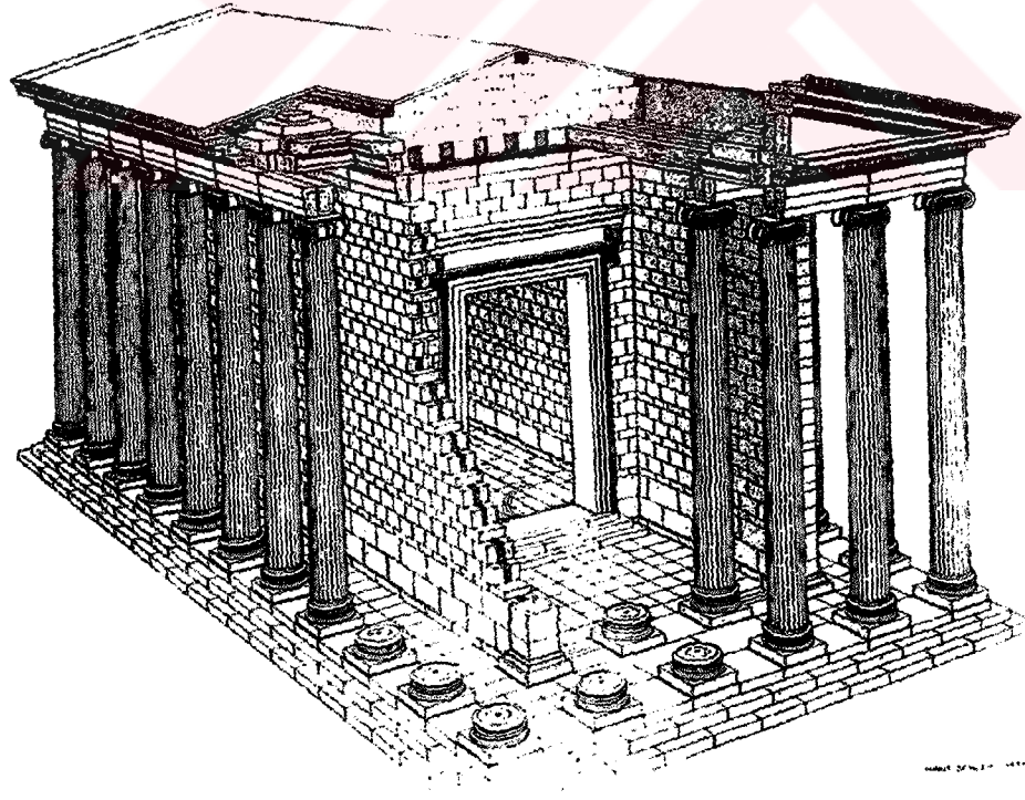
Şekil 5.9 Priene Athena Tapınağı Aksonometrisi
