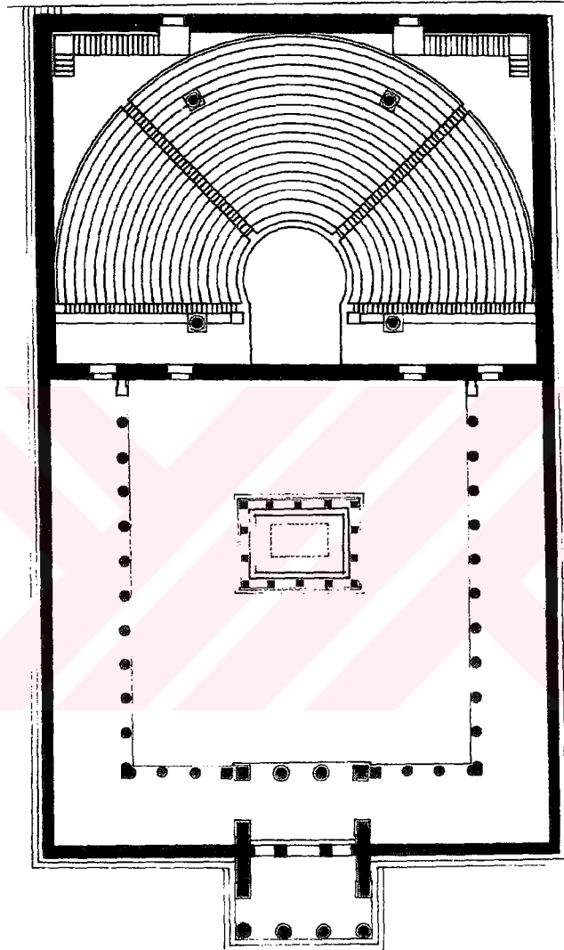
Şekil 4.13: Milet Kenti Bouleuterionu
