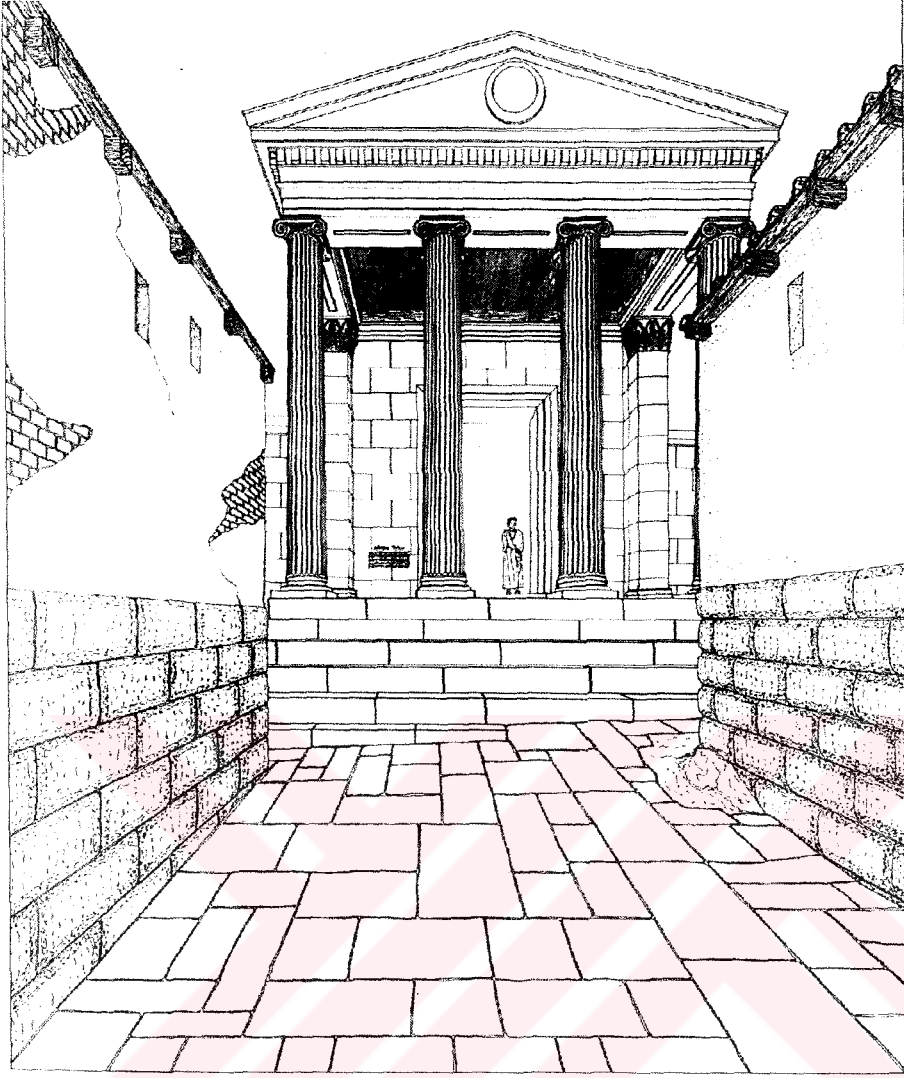
Şekil 5.22 Priene Athena Tapınağı propylonu (W.KOENİNGS,1999, Fig: 94 s:113)
