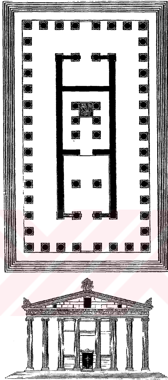
Şekil 4.16 Magnesia Kenti Zeus Tapınağı Planı (O.BİNGÖL s:25 şekil 28)
