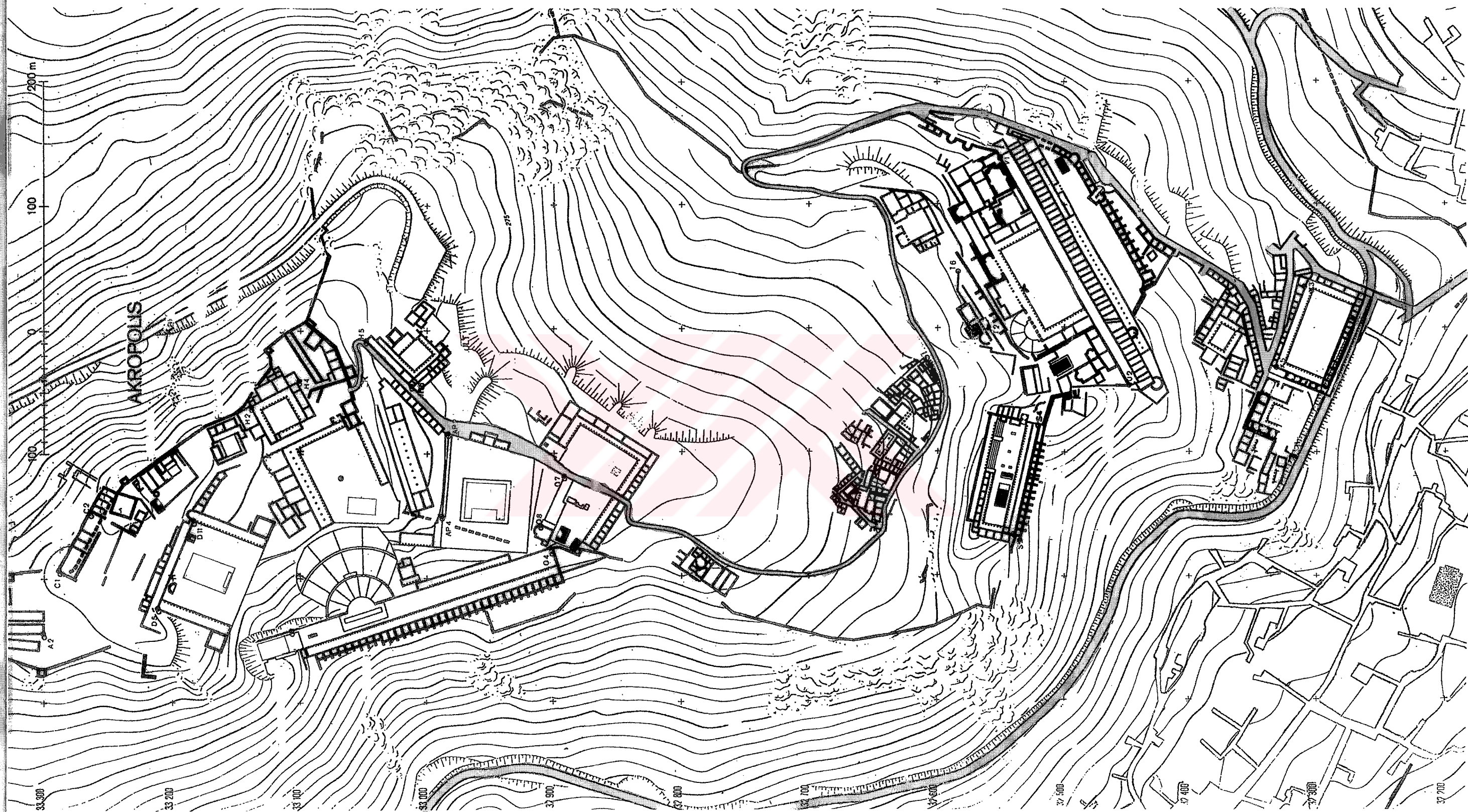
Harita 5.8 Pergamon Kenti Sokak Dokusu
