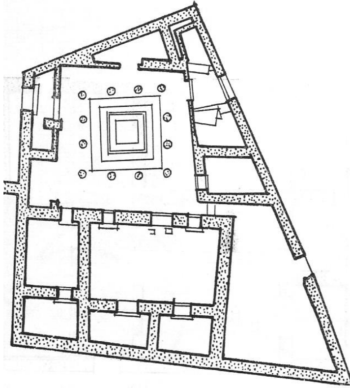
Şekil 55a: Delos Düzensiz Peristyl Konut Tipi
