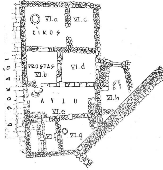
Şekil 91: Kolophon D caddesinin doğusunda yer alan 6 nolu Konut
