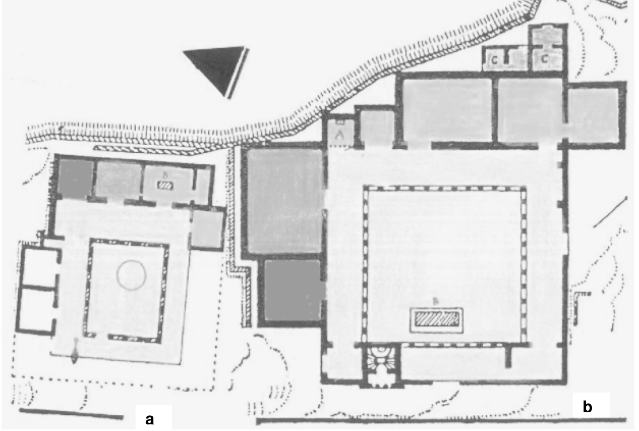
Şekil 115 a; Pergamon I.Attalos'un Sarayı; b: II.Eumenes'in Sarayı
