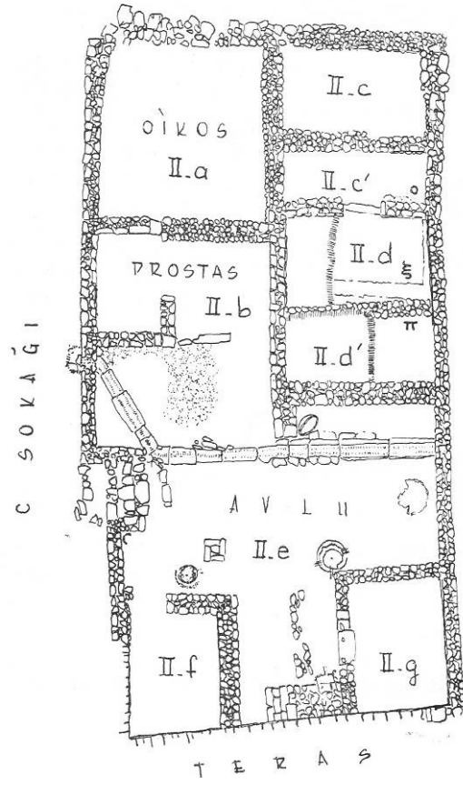
Şekil 89: Kolophon 2 Nolu Konut
