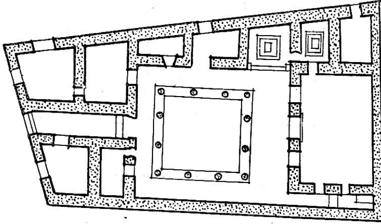
Şekil 31: Olynthus Konut Tipi
