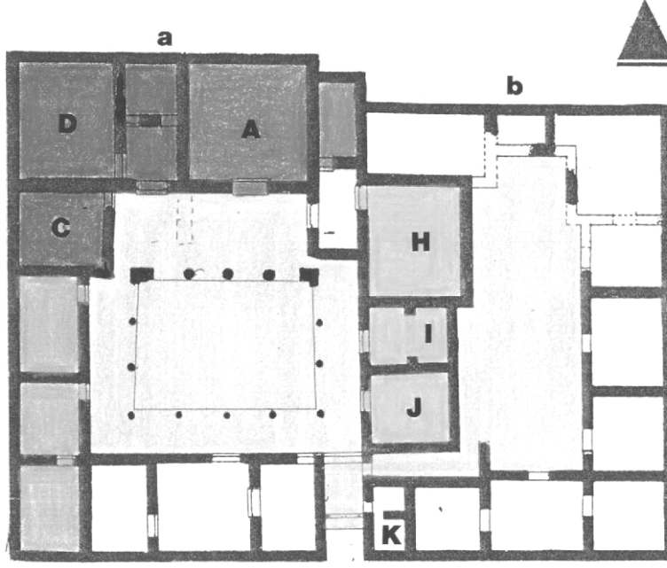
Şekil 109 d: Priene XXXIII nolu Evin Peristyl Hali
