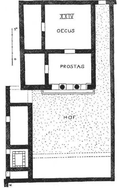
Şekil 48b: Prostas Tarzı Plan Tipi
