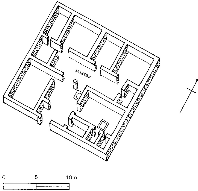
Şekil 32: Pastas Plan Tipinde Olynthus Evi
