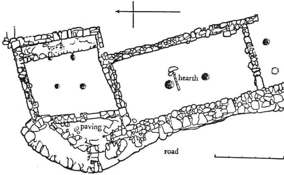
Şekil 18: Emporio Ev Planı
