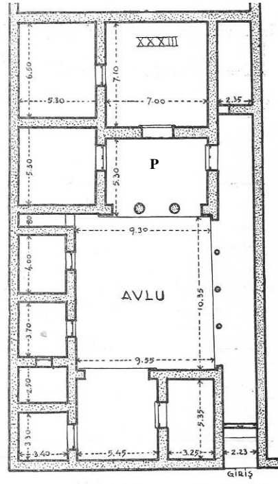
Şekil 109a: Priene XXXIII nolu Ev İlk hali
