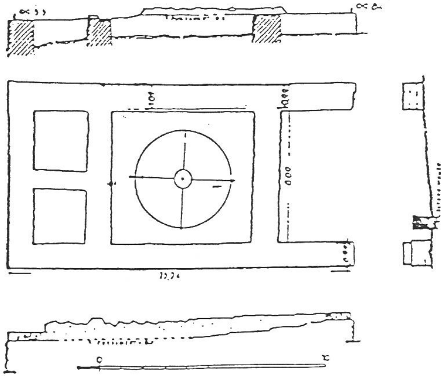
Şekil 79b: Larisada ki Megaronun Planı
