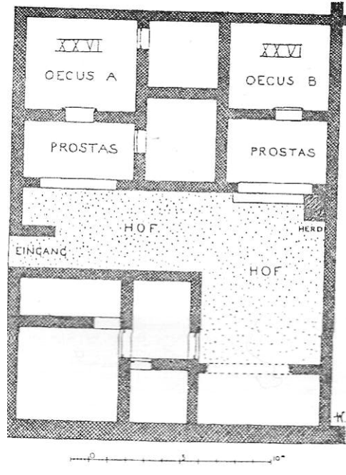
Şekli 48c: Priene M.Ö 4.Yüzyıl Evi
