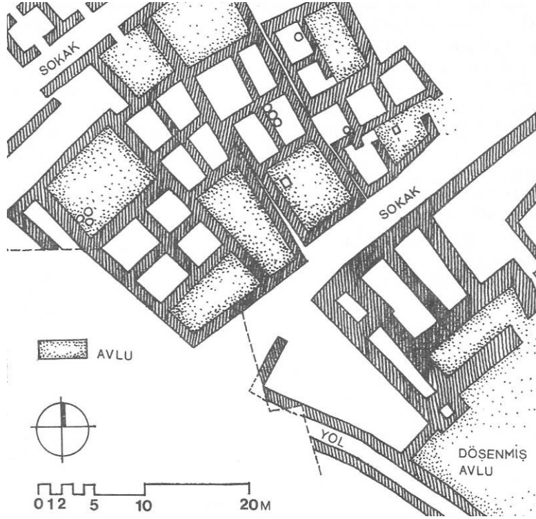
Şekil 15: Hattuşa'da Aşağı Kentte Yer alan Tapınak l'in Kuzeyinde yer Alan Konut Dokusu
