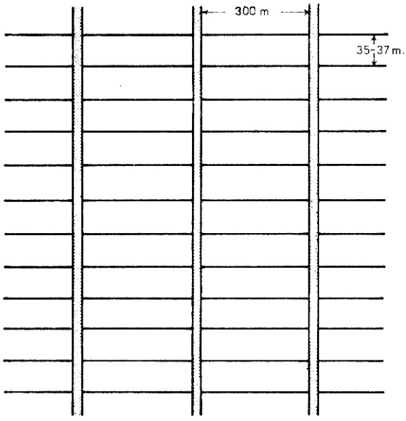
Şekil 41: İtalya'da Izgara Planı
