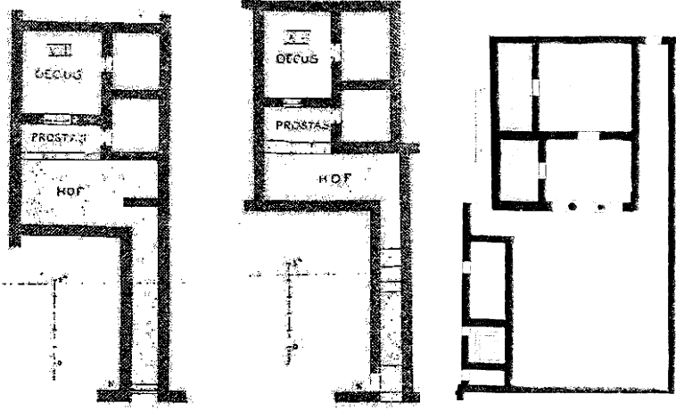
Şekil 101a-b-c: Priene VIII, XV, XIV nolu Evler
