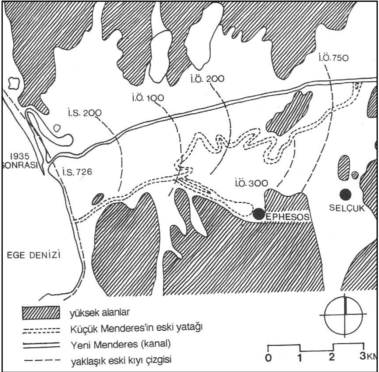
Harita 3: Küçük Menderes Nehrinin Jeomorfolojik Değişimi
