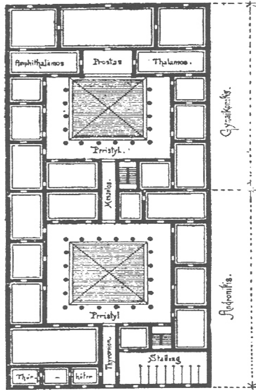
Şekil 63: Thalamos ve Ampithalamos
