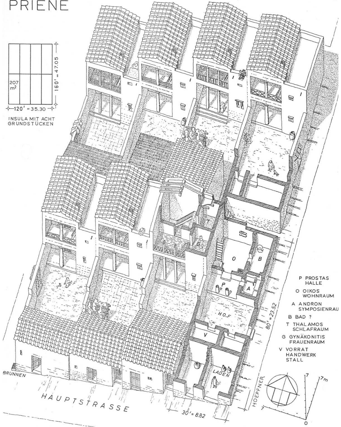
Şekil 109 c: Priene XXXIII nolu Evin Rekonstrüksiyonu ve Genel Olarak Batı Anadolu'da Geçerli Olan Prostas Planın Şeması
