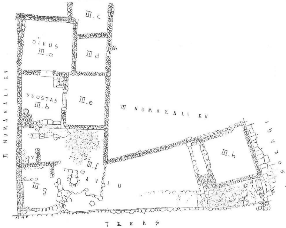
Şekil 88: C ve D caddeleri arasındaki üç konut bloğunun ortasında bulunan 3 nolu konut
