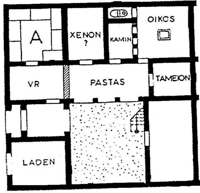
Şekil 47a: Pastas Plan Tipi
