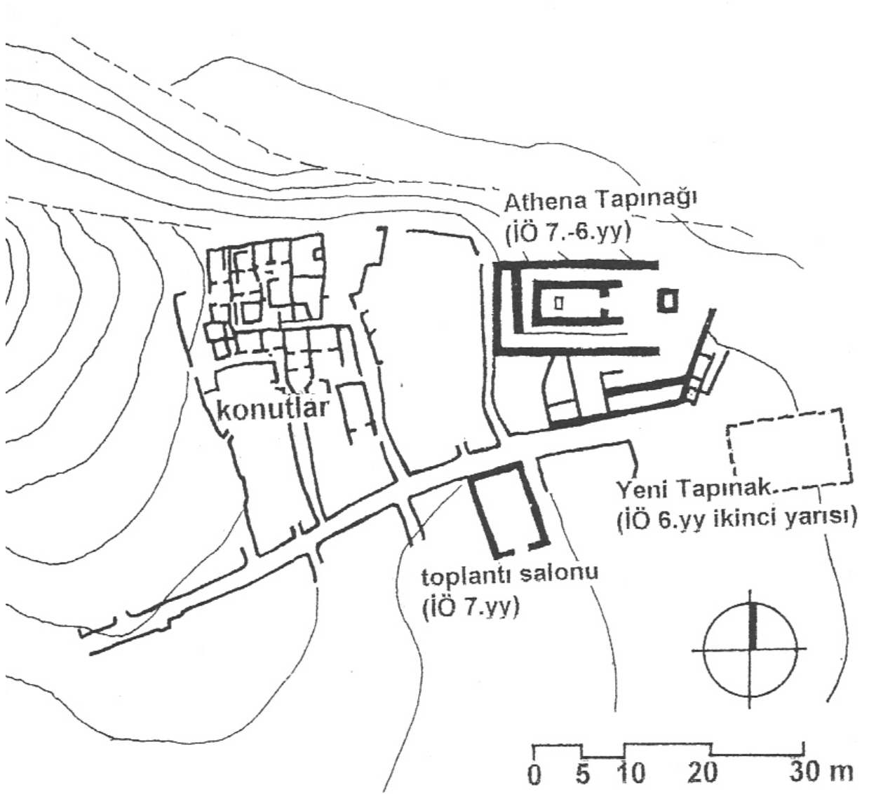
Şekil 71: Smyrna M.Ö 7.ve 6. Yüzyıl Yerleşim Alanı
