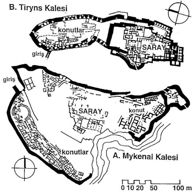
Şekil 27: Mykenai ve Tiryns Yerleşimleri
