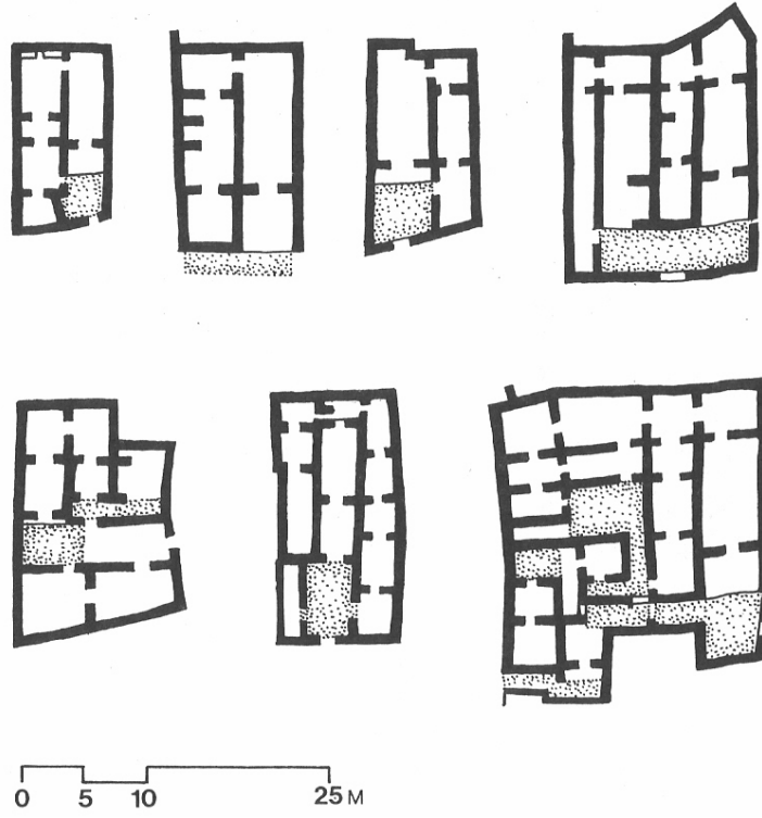
Şekil 11b: Troia II Yapı Katında ki Farklı Büyüklükteki Konutlar
