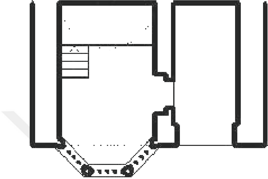
Çizim No. 22: Beşir Ağa Sebil Planı.
