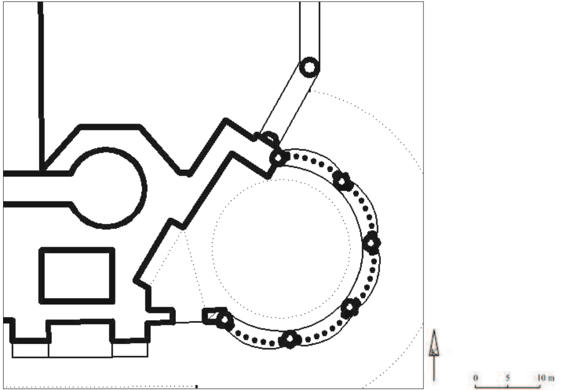
Damat İbrahim Paşa Sebil Planı
