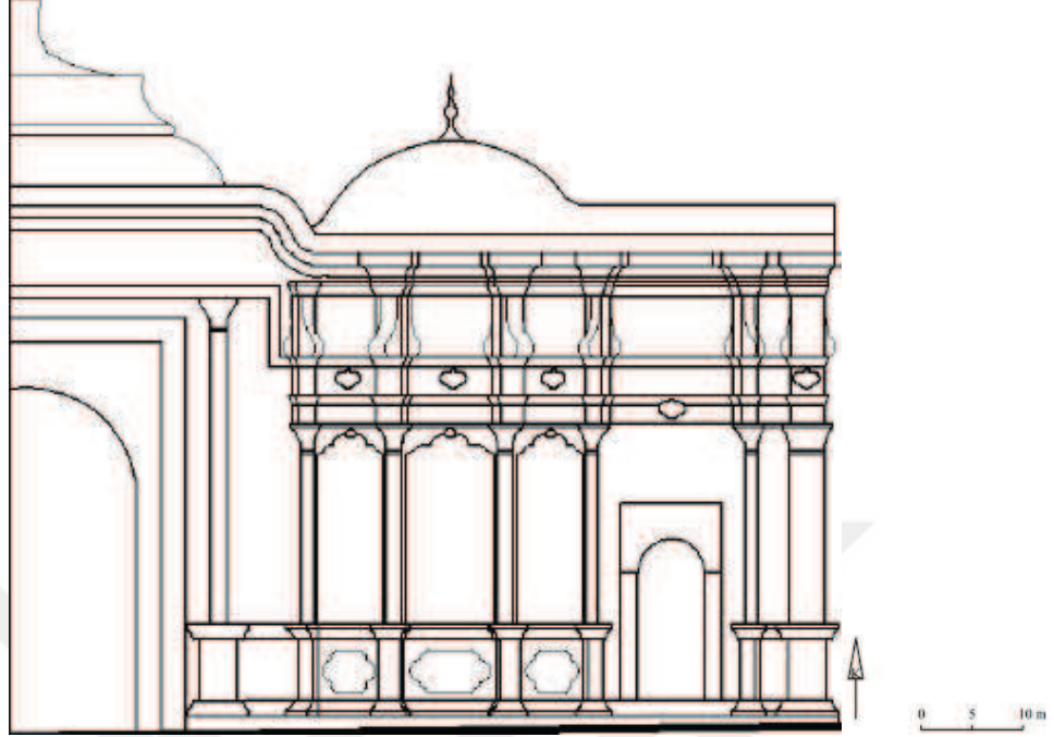
Çizim No. 35: Nuruosmaniye Sebili Cephe Çizimi.
