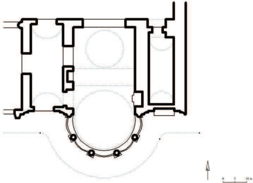
Mehmet Emin Ağa Sebil Planı.
