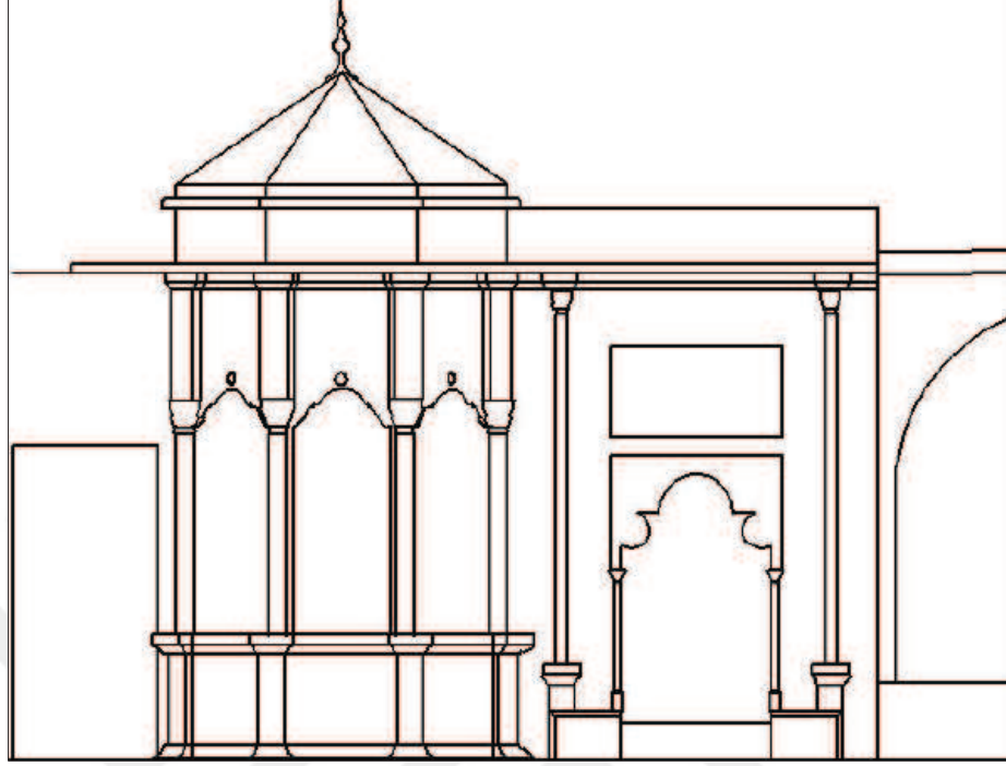
Çizim No. 27: Sadettin Efendi Sebil Cephe Çizimi.
