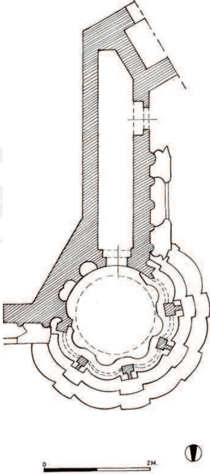
Çizim No. 40: Hamidiye Sebil Planı.
