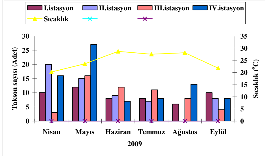
Şekil 3.3.3.1. Yüzey su sıcaklığı ile epipsammikte kaydedilen takson sayılarının istasyonlardaki aylık değişimi
