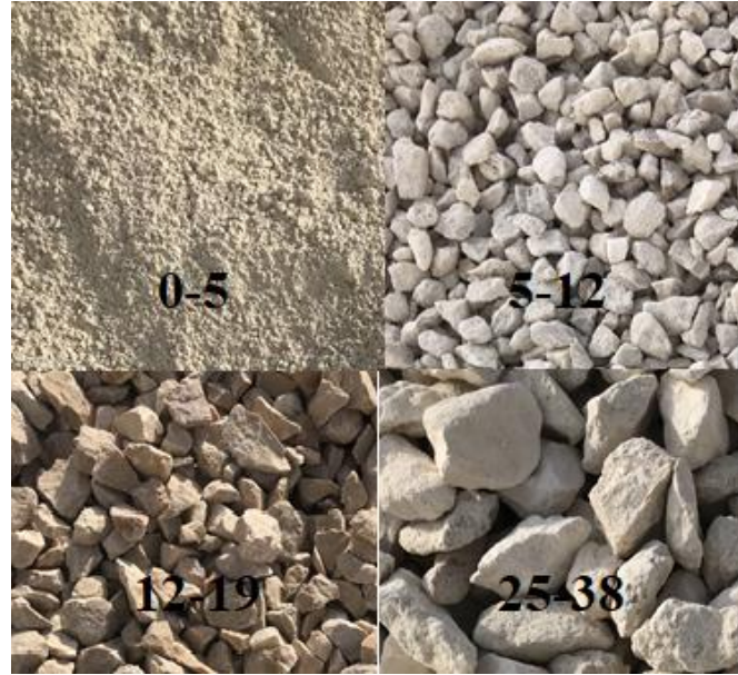
Şekil 5.3. Agregat boyutlarını gösteren bir örnek
