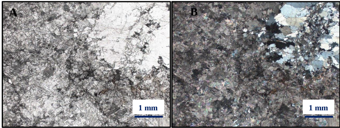
Şekil 7.13. DKÇ-1 kodlu Rekristalize Kireçtaşı numunesine ait ince kesit görüntüleri (A-Tek nikol, B-çift nikol)
