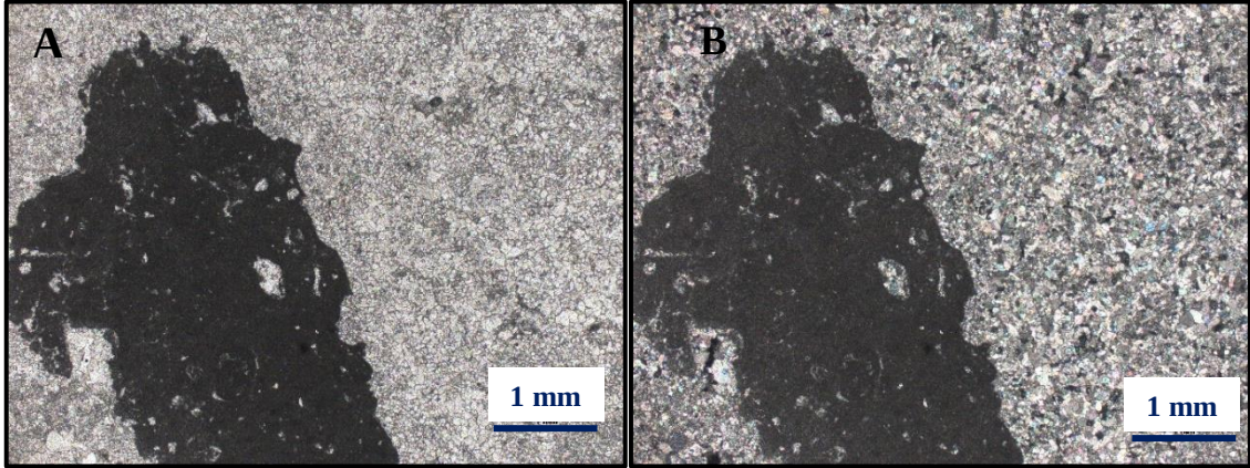
Şekil 7.10. DHK-6 kodlu Kalkitik Dolomit numunesine ait ince kesit görüntüleri (A-Tek nikol, B-çift nikol)
