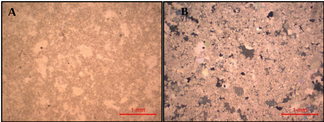
Şekil 7.18. DHK-4 kodlu numuneye ait ince kesit görüntüleri (A-Tek nikol, B-çift nikol)
