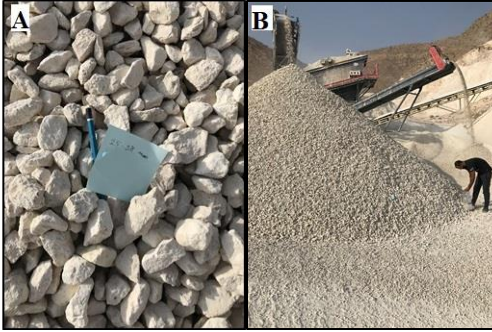
Şekil 6.42. Yeni Hasankeyf konkasörü (DHK-4)' ne ait 25-38 mm boyutundaki agregası (A-yakın stok, B-uzak bant altı)
