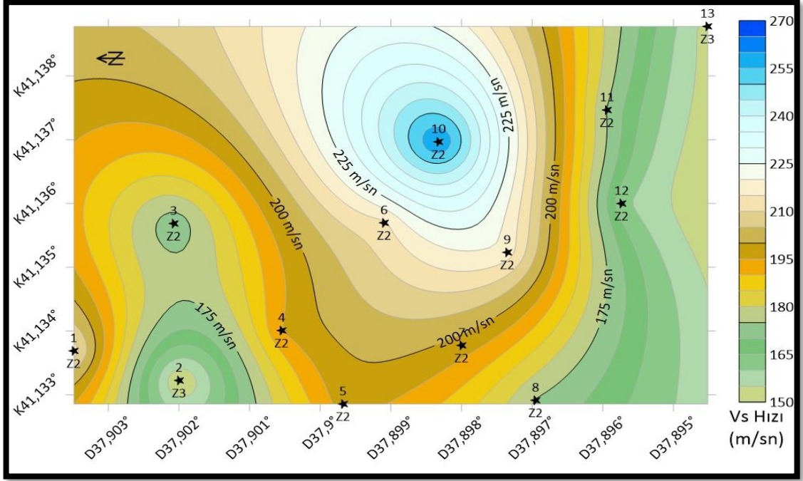
Şekil 4.46. Gap ve Bahçelievler Mahallelerinde yapılan mikrotremor ölçümlerinden elde edilen F_0 baskın frekans değerleri üzerinden Kanai, (1983)'nin ana kaya üzerindeki yumuşak zemin tabakası için ileri sürdüğü T = \Sigma 4H_i/V_{si} formülünü kullanarak 15m derinlik için V_s hızlarının hesaplanarak oluşturulan hız haritası modeli ve bu değerlere karşılık gelen zemin sınıfları
