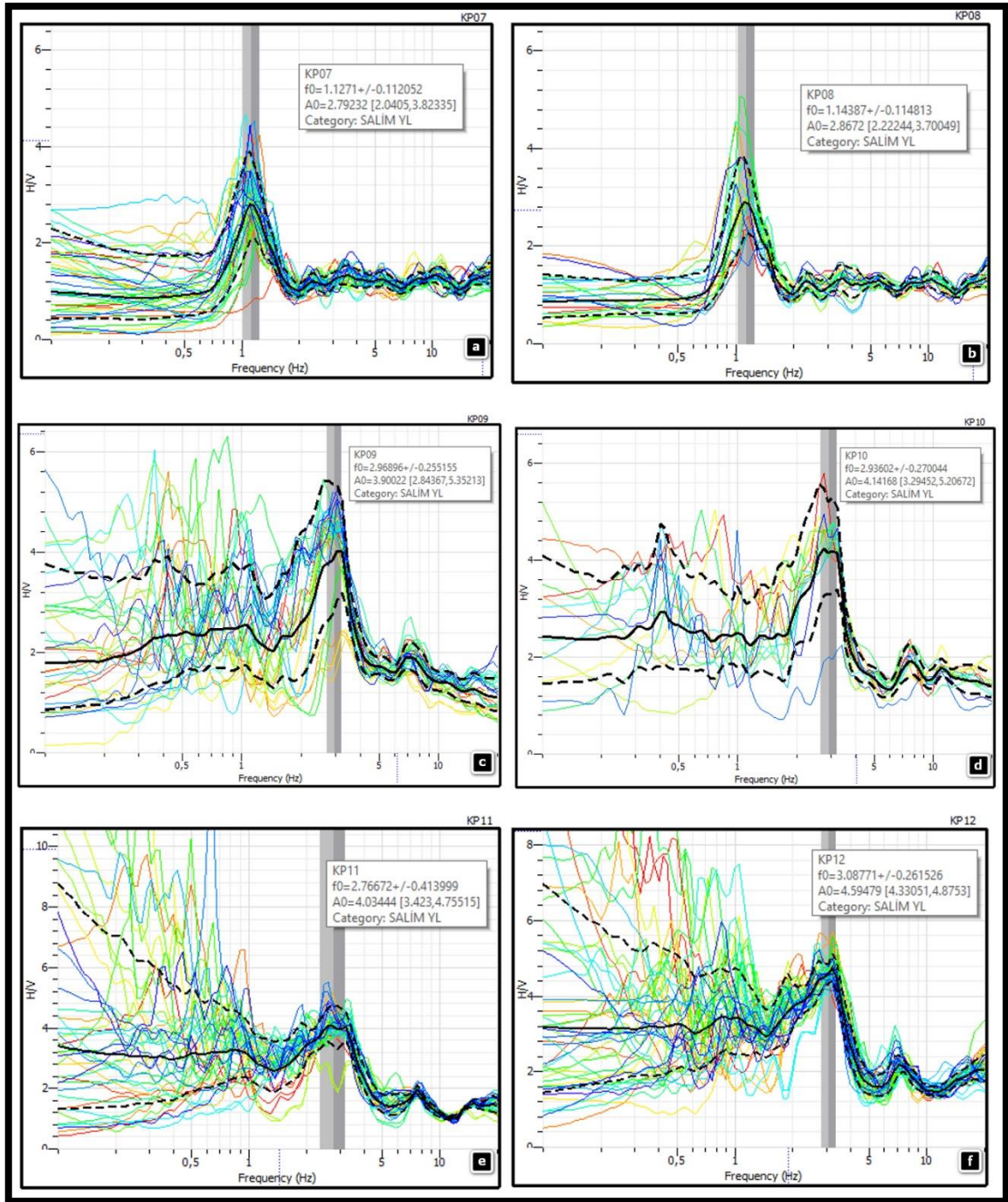
Şekil 4.32. Kültür ve Pazaryeri Mahallelerinde yapılan mikrotremor ölçümlerinden son 6 noktanın ölçüm noktasına ait H/V oran spektrumları
