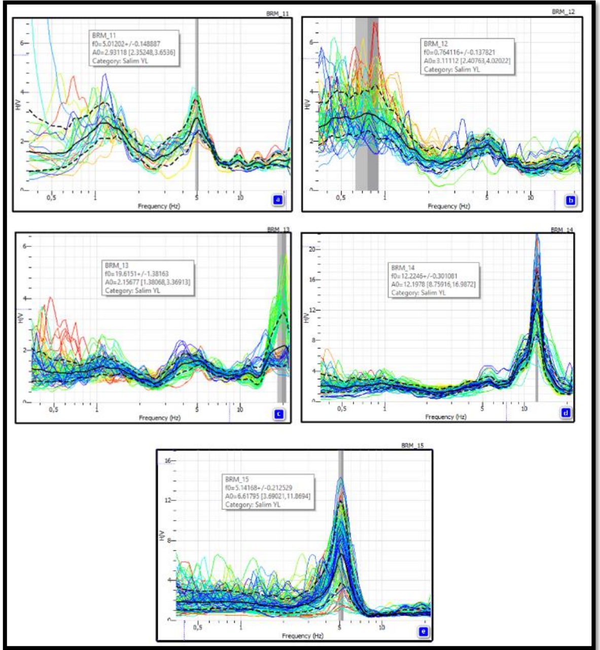
Şekil 4.18.Batı Raman kampüs alanında yapılan mikrotremor ölçümlerinden üçüncü 5 noktanın ölçüm noktasına ait H/V oran spektrumları
