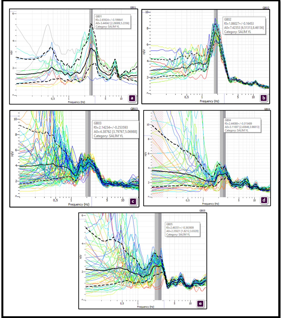
Şekil 4.42. Gap Mahallesinde yapılan mikrotremor ölçümlerinden ilk 5 noktanın ölçüm noktasına ait H/V oran spektrumları
