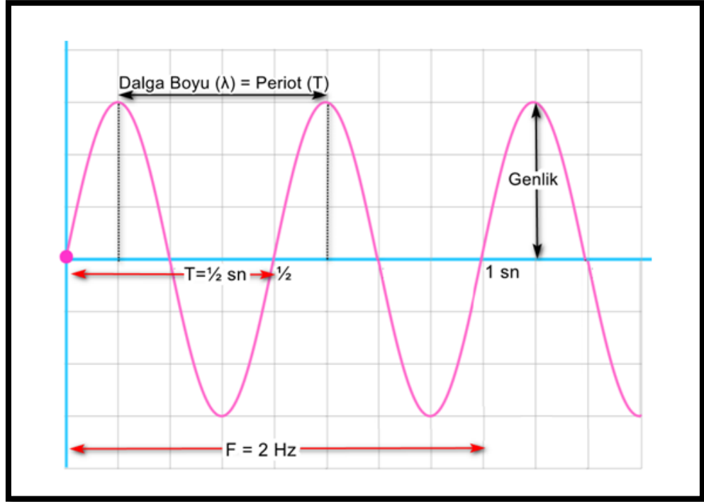
Şekil 3.1. Sismik dalga bileşenleri
