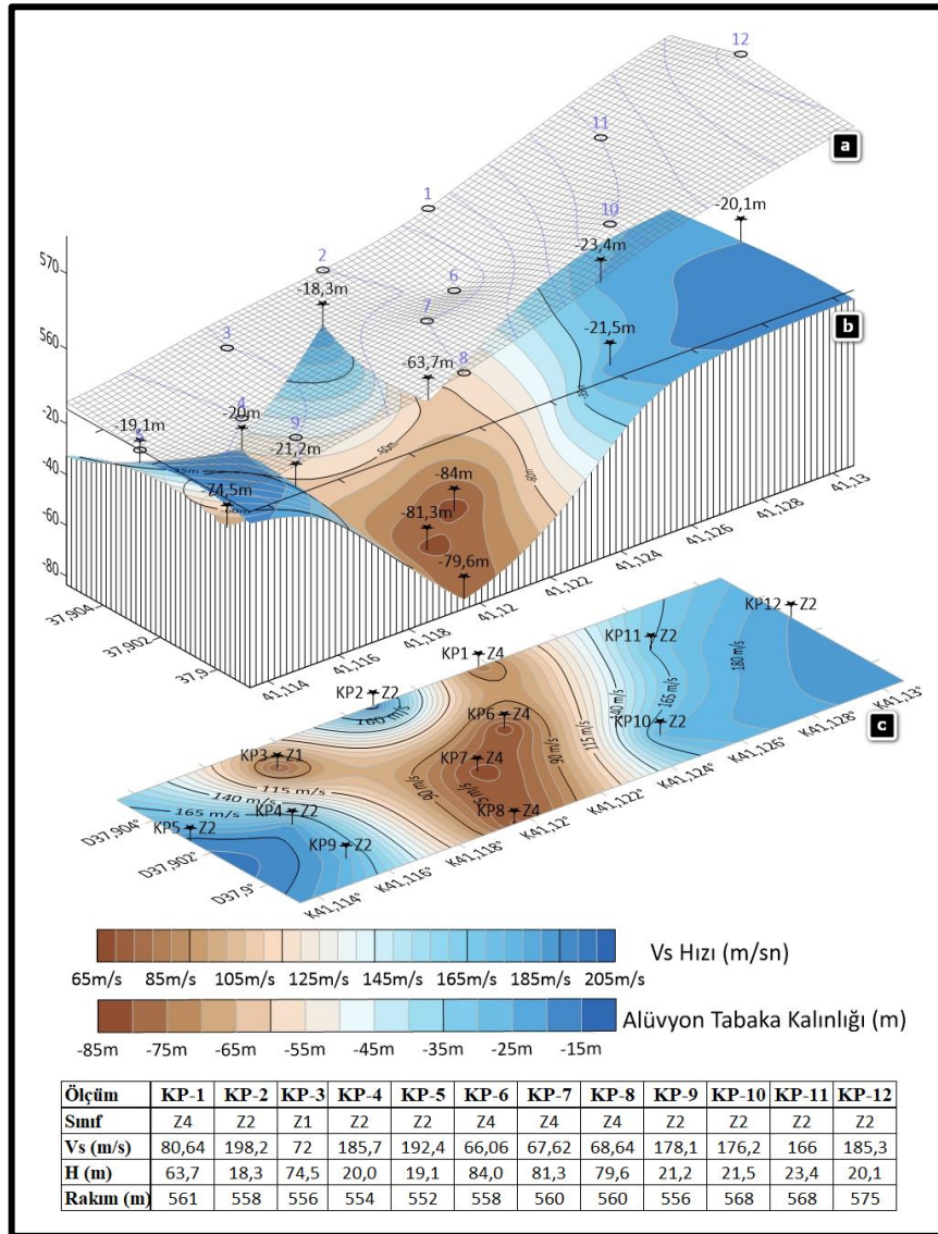
řekil 4.38. K lt r Pazaryeri Mahalleleri a)  l  m alanının eř y kseklik haritası. b) Seht ve Wohlenberg (1999)'in yumuřak sediman kalınlıęı H = 96f^{-1.388} baęıntısı ile hesaplanan (H) derinlik deęeri. c)
