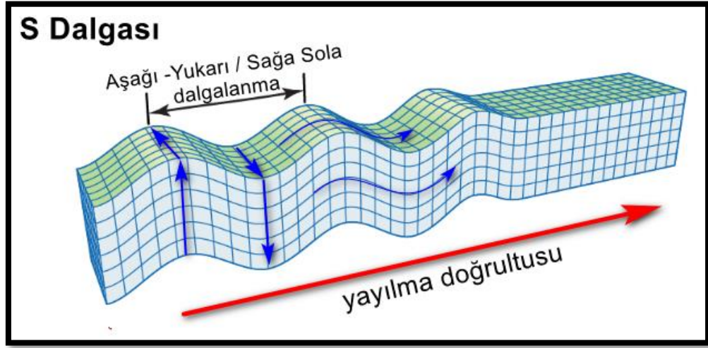
Şekil 3.3.S-dalgası tanecik hareketinin şematik gösterimi
