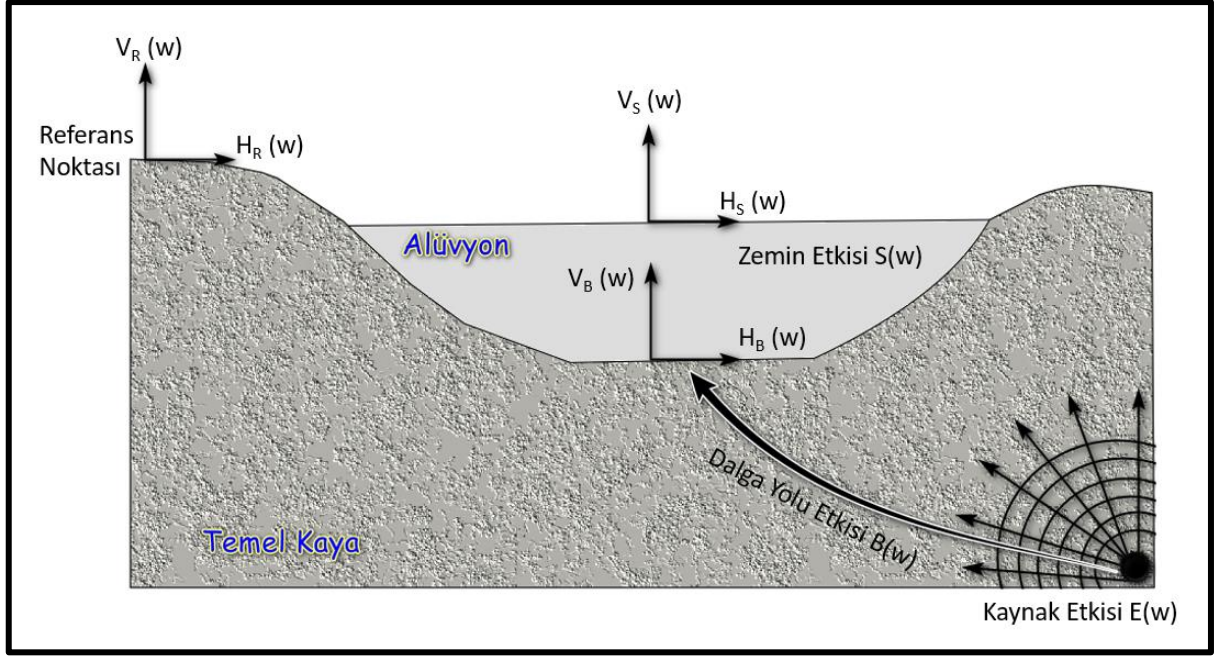
Şekil 3.7.Referans noktası yöntemi ölçüm alım modeli (Dikmen, 2006)
