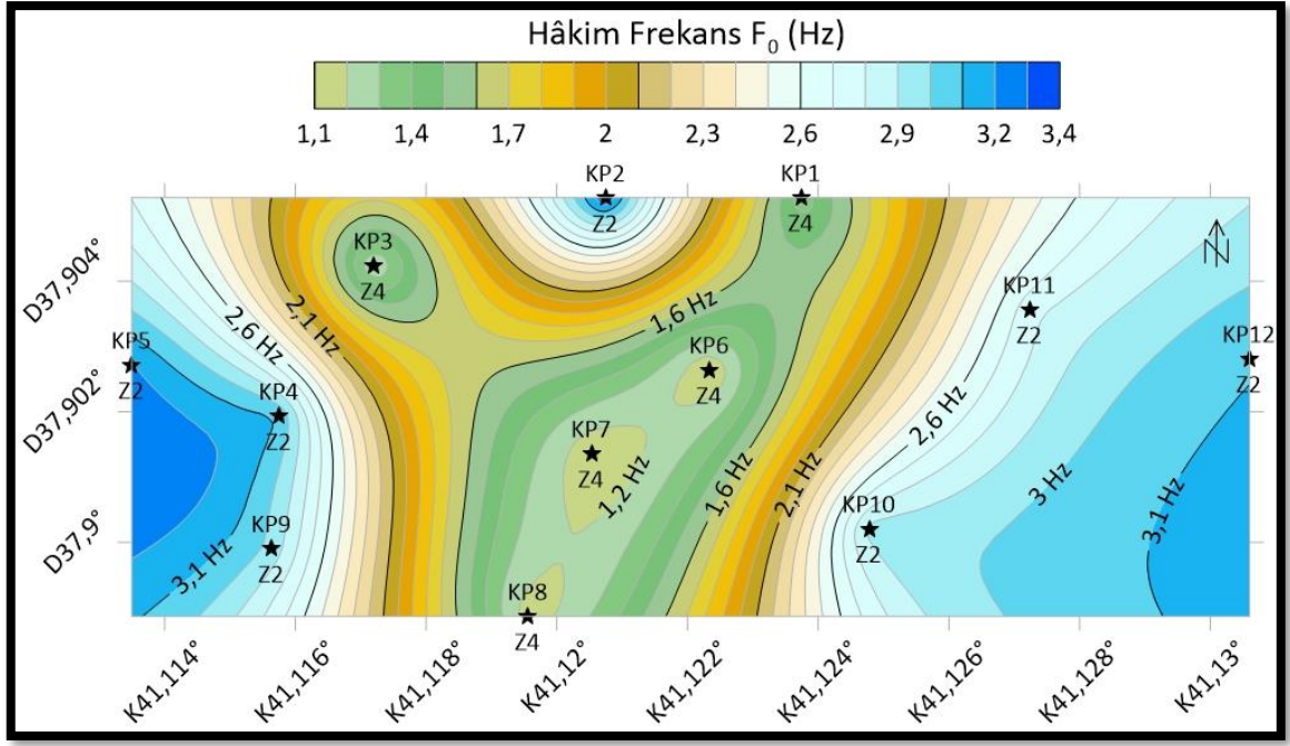
Şekil 4.33. Kùltür ve Pazaryeri Mahallelerinde yapılan mikrotremor ölçümlerinden elde edilen F_0 Baskın Frekans değeri ve bu değere karşılık gelen zemin sınıfları. Frekans değeri ve zemin sağlamlığı ile doğru orantılı olduğu, frekans büyüdükçe zeminin sağlamlığı görülmektedir
