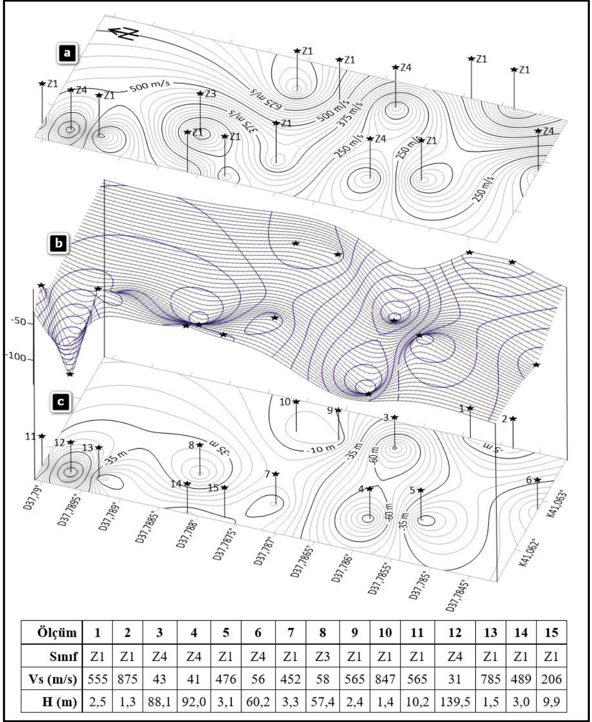
Şekil 4.23. Batı Raman kampüs alanında yapılan mikrotremör ölçümlerinden elde edilen F_0 Baskın Frekans değerleri üzerinden a) V_s hızlarının hesaplanmasıyla oluşturulan hız haritası ve bu değerlere karşılık gelen zemin sınıfları. b) ve c) Yumuşak sediman kalınlığı H = 96f^{-1.388} bağıntısı ile hesaplanan (H) derinlik değeri.
