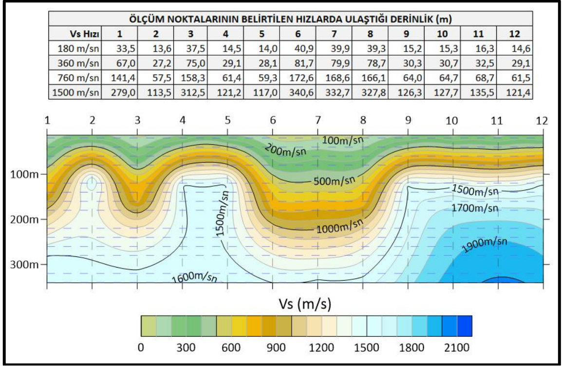
Şekil 4.12. Kültür Pazaryeri mahalleleri mikrotremor kayıtları kullanılarak Kanai (1983)'nin bağıntısı üzerinden bilinen zemin sınıflama hızlarına karşılık gelen derinlik değerleri ile ölçümlerin eşit aralıklarla düz bir profil üzerinden alınmış olduğu varsayılsaydı ortaya çıkacak olan hızla bağlı derinlik modeli.
