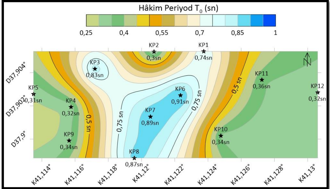
Şekil 4.34. Kùltür ve Pazaryeri Mahallelerinde yapılan mikrotremor ölçümlerinden elde edilen T Baskın Periyot değeri ve bu değere karşılık gelen zemin sınıfları. Periyot değeri ve zemin sağlamlığı ile ters orantılı olduğu, periyot küçüldükçe zeminin sağlamlığı bilinmektedir.
