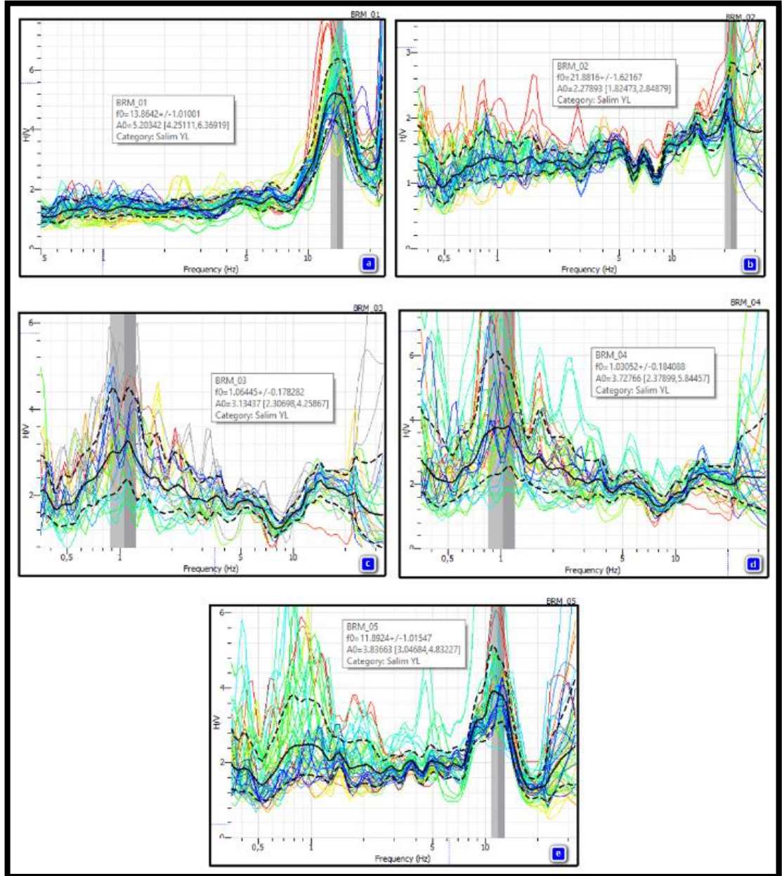
Şekil 4.16. Batı Raman kampus alanında yapılan mikrotremor ölçümlerinden ilk 5 noktanın ölçüm noktasına ait H/V oran spektrumları
