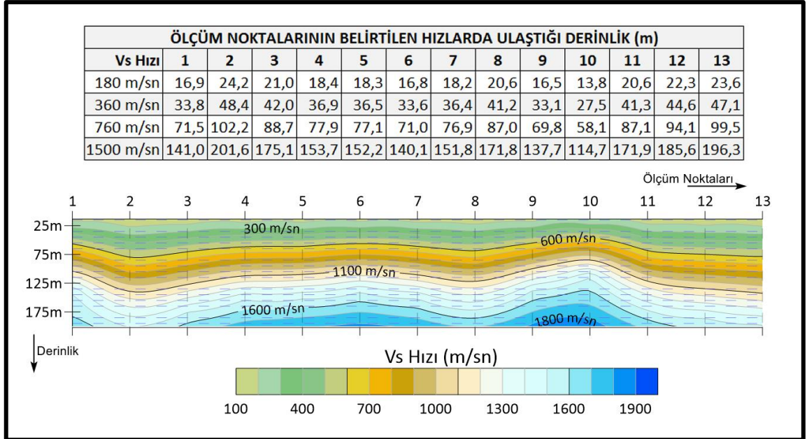
Şekil 4.47. Gap ve Bahçelievler mahallelerinde mikrotremor kayıtları kullanılarak Kanai (1983)'nin bağıntısı üzerinden bilinen zemin sınıflama hızlarına karşılık gelen derinlik değerleri ile ölçümlerin eşit aralıklarla düz bir profil üzerinden alınmış olduğu varsayılsaydı ortaya çıkacak olan hıza bağlı derinlik modeli
