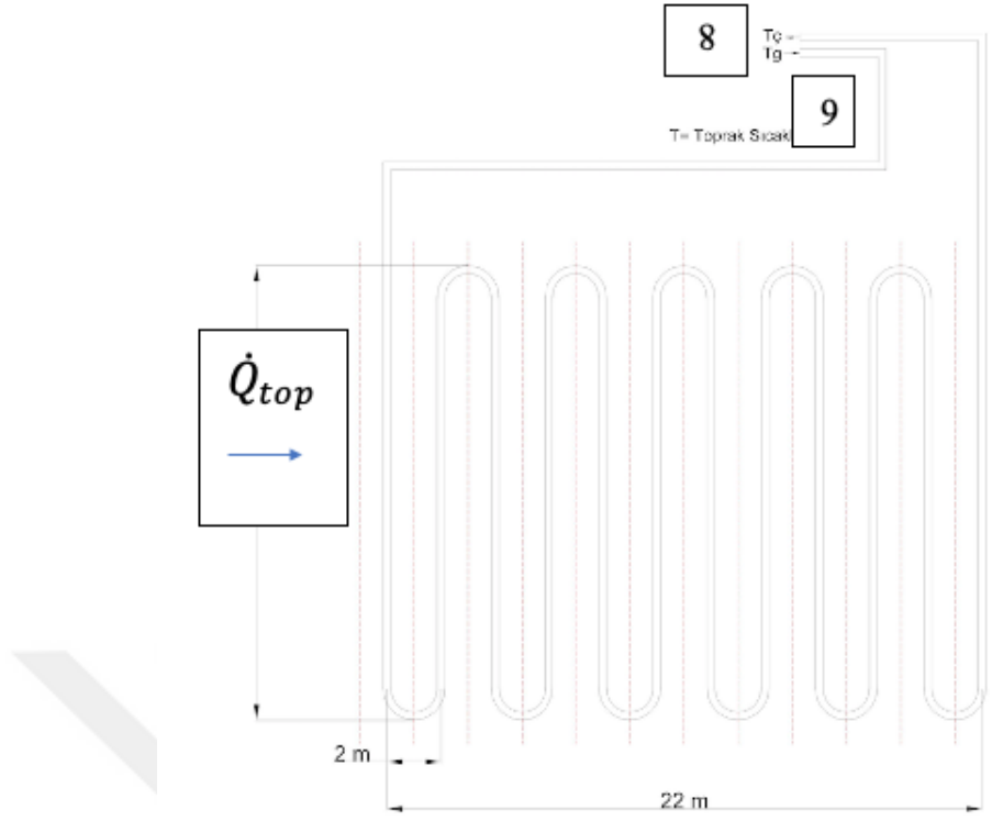
Şekil 5.50. TID çizim şeması
