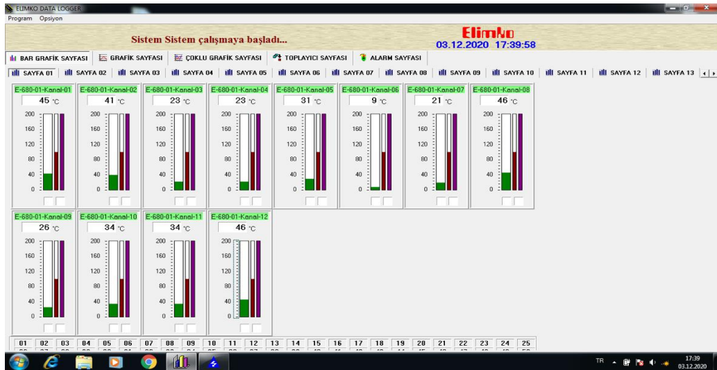
Şekil 3.16. Datalogger ekran görüntüsü
