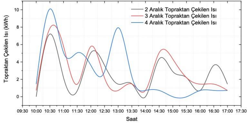
Şekil 5.14. Toprakdan çekilen ısı miktarı (kW) zamanla değişimi
