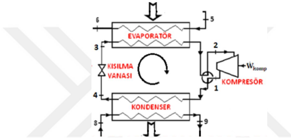
Şekil 5.30. Isı pompası devresi
