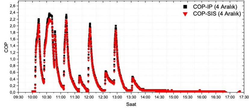
Şekil 5.25. 4 Aralık tarihlerinde elde edilen COP_{SIS} ve COP_{IP} değerleri
