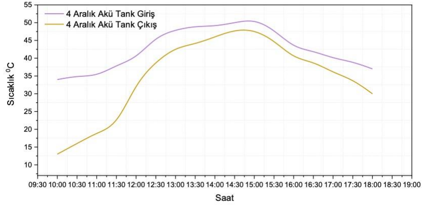
Şekil 5.22. 4 Aralık akümülayon tankı giriş-çıkış sıcaklık değerleri
