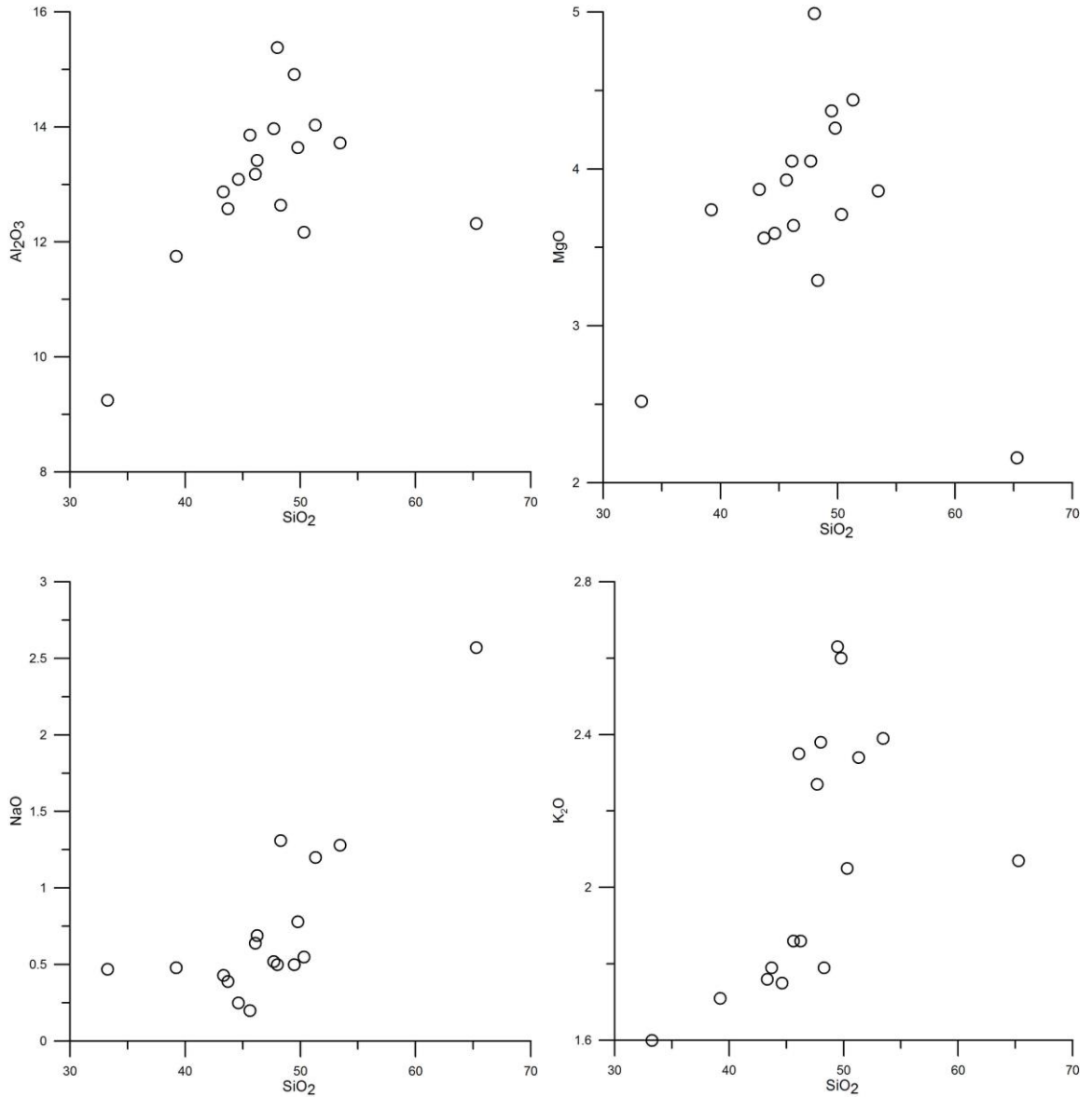
Şekil 4.3 İnceleme alanından alınan örneklere ait Harker Diyagramları ( \text{SiO}_2 - \text{Al}_2\text{O}_3 , \text{SiO}_2 - \text{MgO} , \text{SiO}_2 - \text{NaO} , \text{SiO}_2 - \text{K}_2\text{O} )
