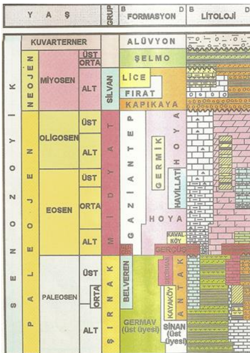
Şekil 2.2 Güneydoğu Anadolu Bölgesinin Genelleştirilmiş Stratigrafik Kesit
