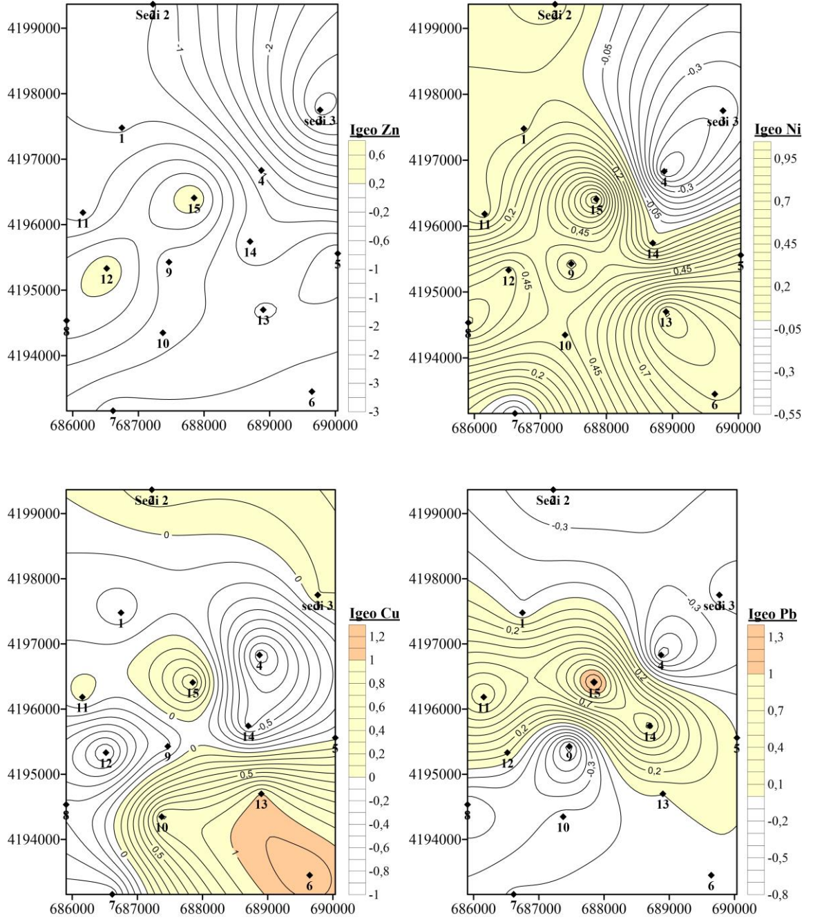
Şekil 4.10 Zn, Ni, Cu ve Pb elementleri için hesaplanan Jeobirikim indeksi değerlerinin inceleme alanındaki dağılımları
