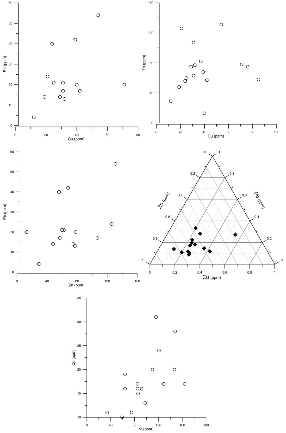
Şekil 4.7 İnceleme alanına ait örneklerin iz element korelasyonları
