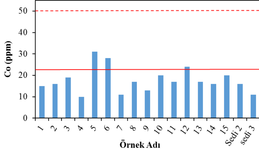
Şekil 4.27 İnceleme alanına ait örneklerin Co içeriklerinin sağlık açısından değerlendirilmesi
