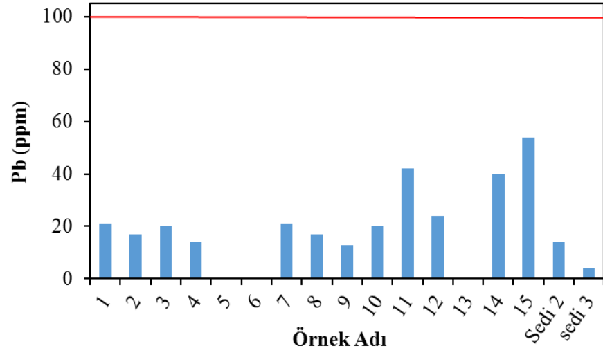
Şekil 4.24 İnceleme alanına ait örneklerin Pb içeriklerinin sağlık açısından değerlendirilmesi
