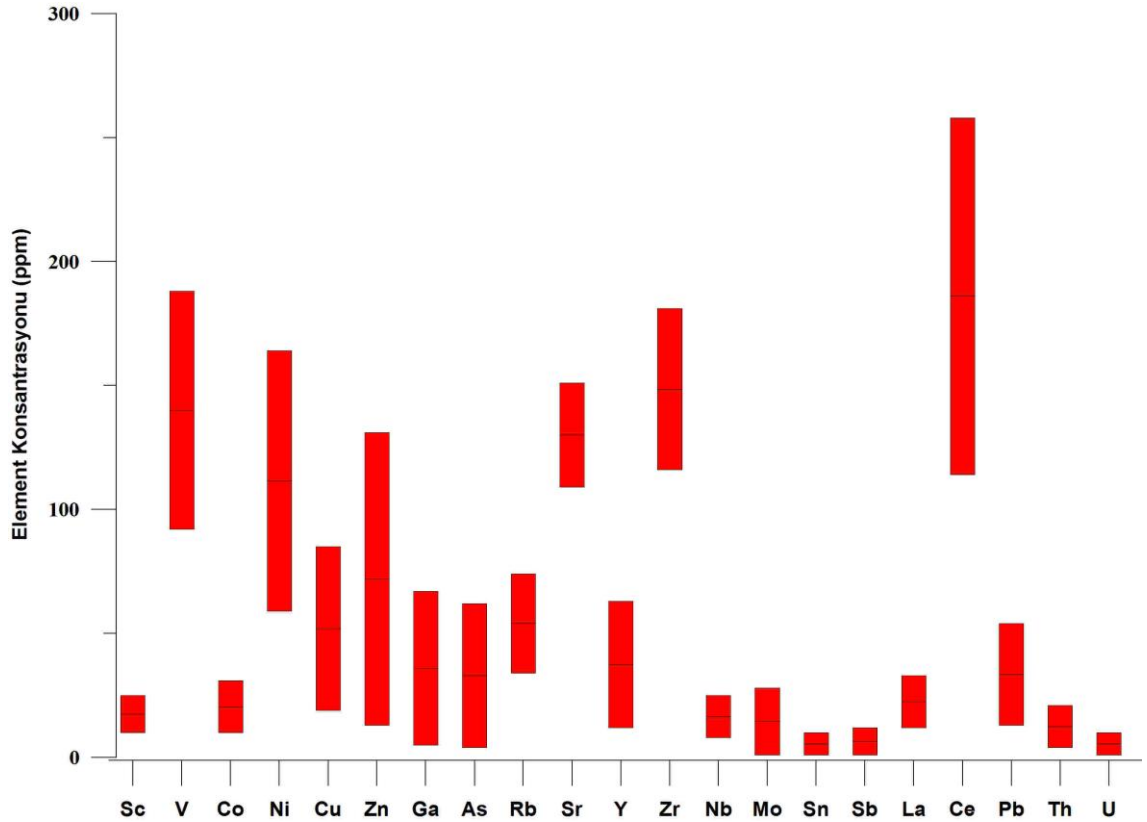
Şekil 4.8 İnceleme alanına ait örneklerdeki elementlerin dağılımını gösteren kutu diyagramı
