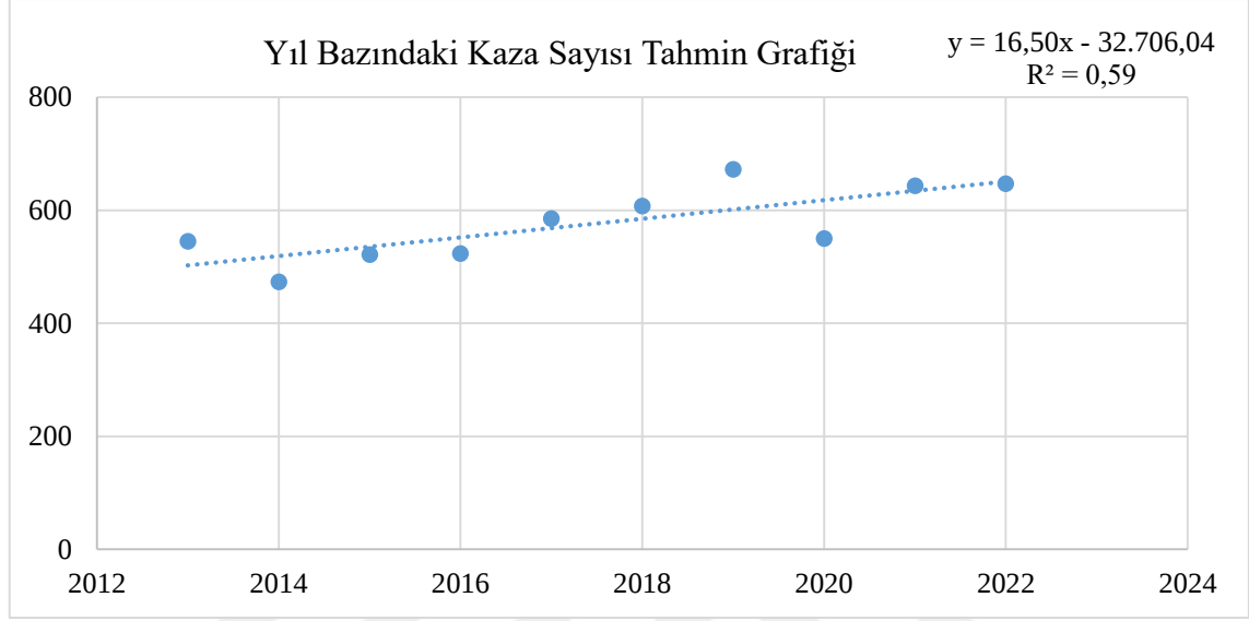
Şekil 33.31. Yıl bazındaki kaza sayısı tahmin grafiği
