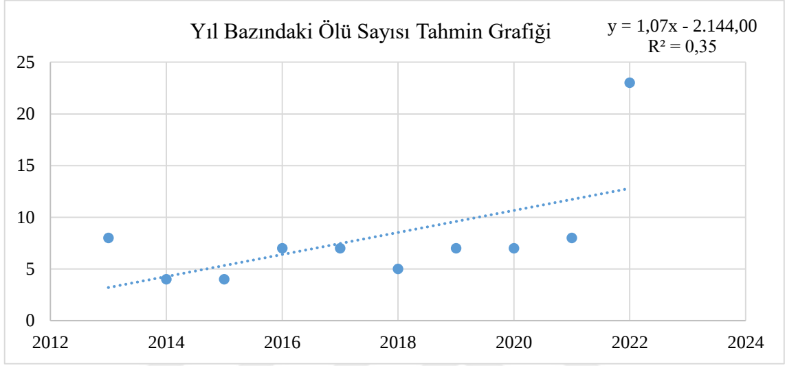
Şekil 31.29. Yıl bazındaki ölü sayısı tahmin grafiği
