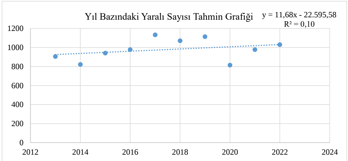
Şekil 32.30. Yıl bazındaki yaralı sayısı tahmin grafiği
