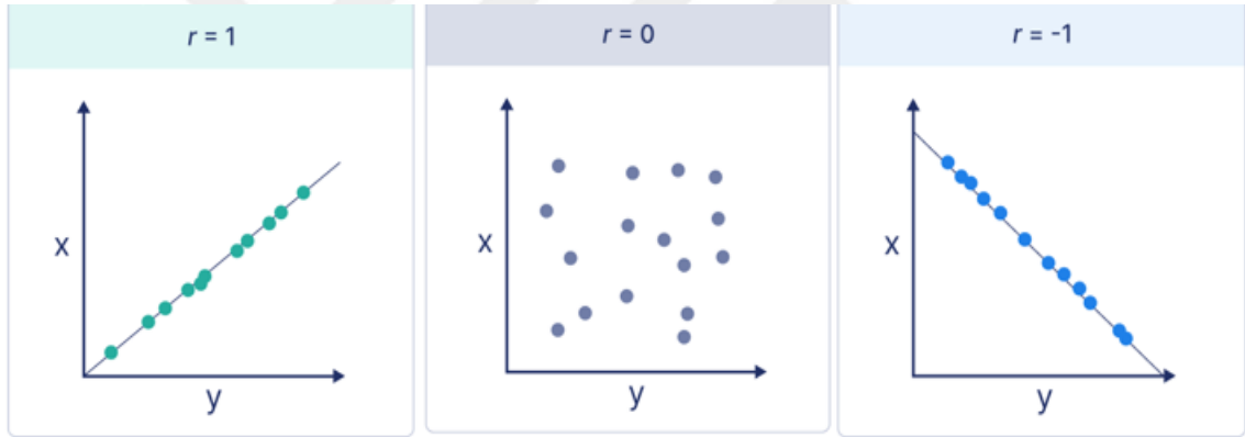
Şekil 2.2. Pearson korelasyon grafikleri
