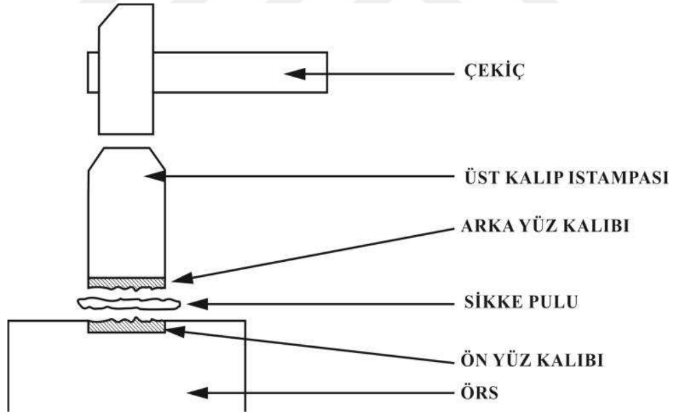
Şekil 3.3. Çekiç İle Darp Tekniği(Tekin,2008, s.22).
