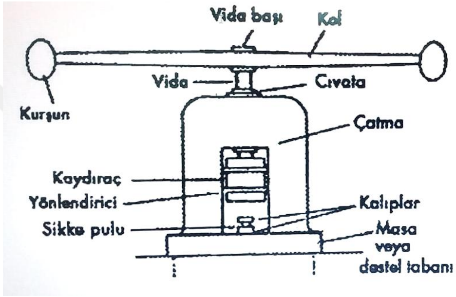
řekil 3.5. Mekanik Darp Teknięi (kaldıralı pres). (Kemaloęlu, 2023, s. 51).
