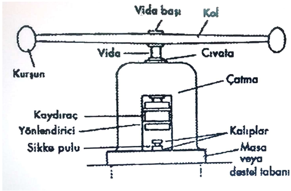
Şekil 3.5. Mekanik Darp Tekniği (kaldıraçlı pres). (Kemaloğlu, 2023, s. 51).
