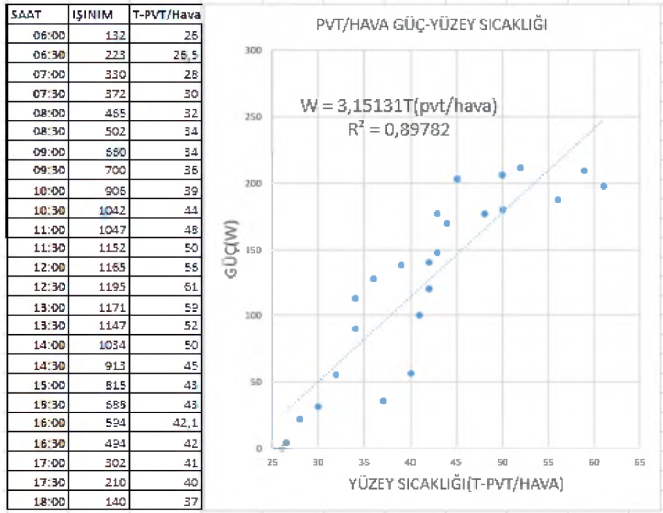
Şekil 5.42. PV/T-Hava için güç-yüzey sıcaklığı
