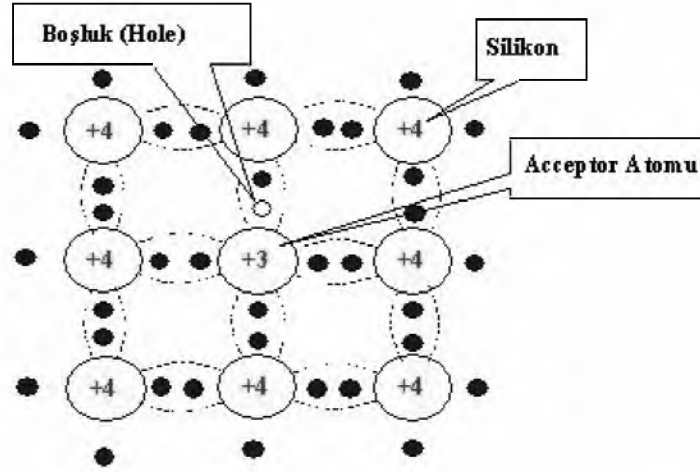
Şekil 3.6. P Tipi Yarı İletken (Karamanav,2007)
