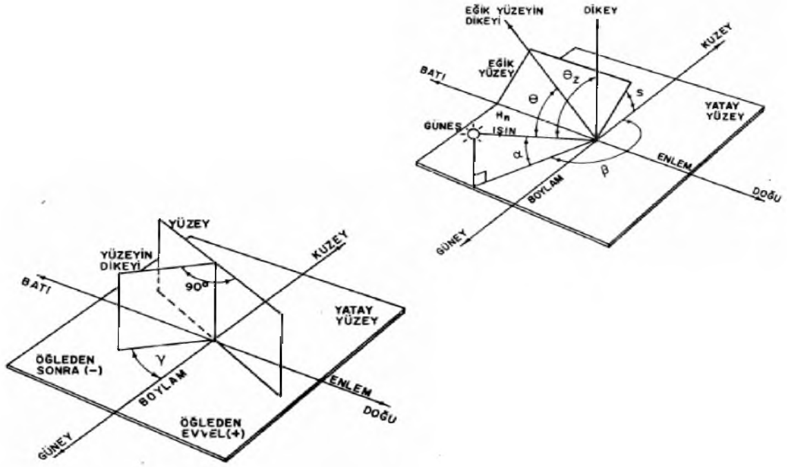
Şekil 4.20. Açı konumları (Anonim,2018e)
