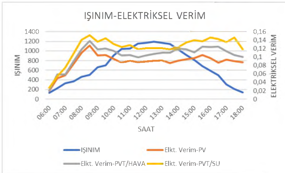
Şekil 5.14. 0.016 l/s, 3mm kalınlıkta Işınım-Elektriksel Verim grafiği
