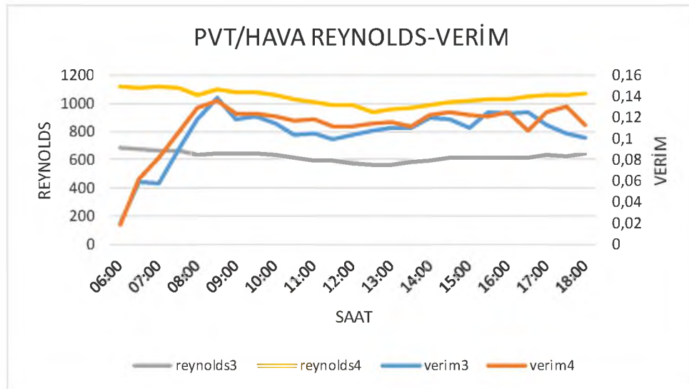
Şekil 5.48. Hava soğutmalı sistemde Reynolds sayısı verim karşılaştırması
