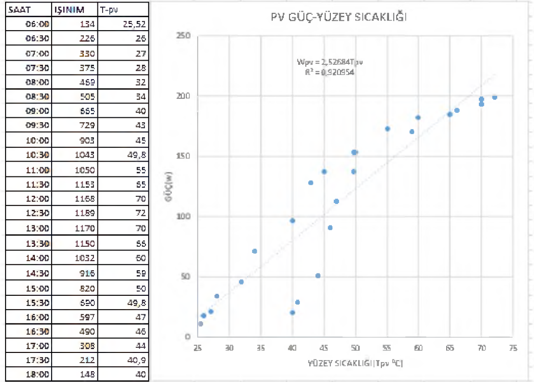
Şekil 5.35. PV için güç-yüzey sıcaklığı
