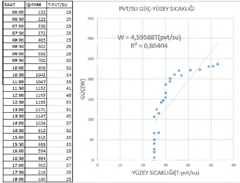
Şekil 5.43. PV/T-Su için güç-yüzey sıcaklığı
