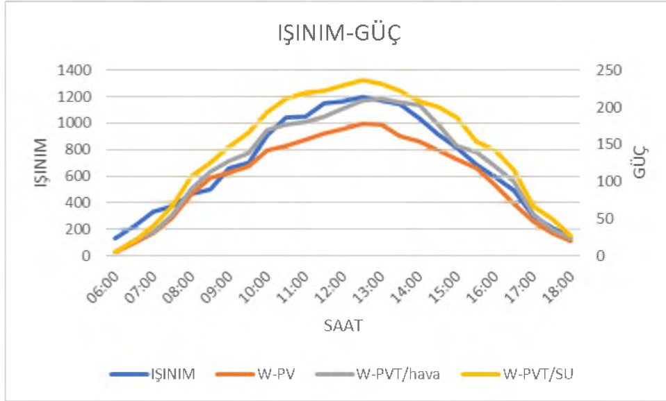
Şekil 5.13. 0.016l/s, 3mm kalınlıkta Işınım-Güç grafiği
