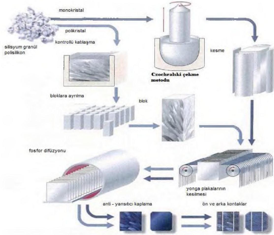
Şekil 3.1. Czochralski Monokristal ve Polikristal Silisyum Üretimi (Boz, 2011)
