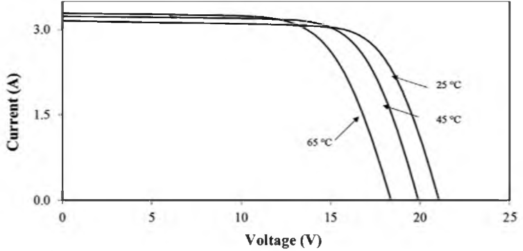
Şekil 3.10. Volt Amper ilişkisi (Andreev,2003)
