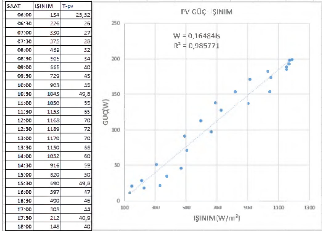
Şekil 5.32. PV için güç-ışınım.
