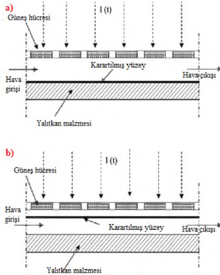
Şekil 1.6. (a) hava toplayıcı kesit görünümü, hava karartılmış yüzey üzerinde akar. (b) hava toplayıcı kesit görünümü, karartılmış yüzeyin altında hava akımları (Alfegi, 2009)
