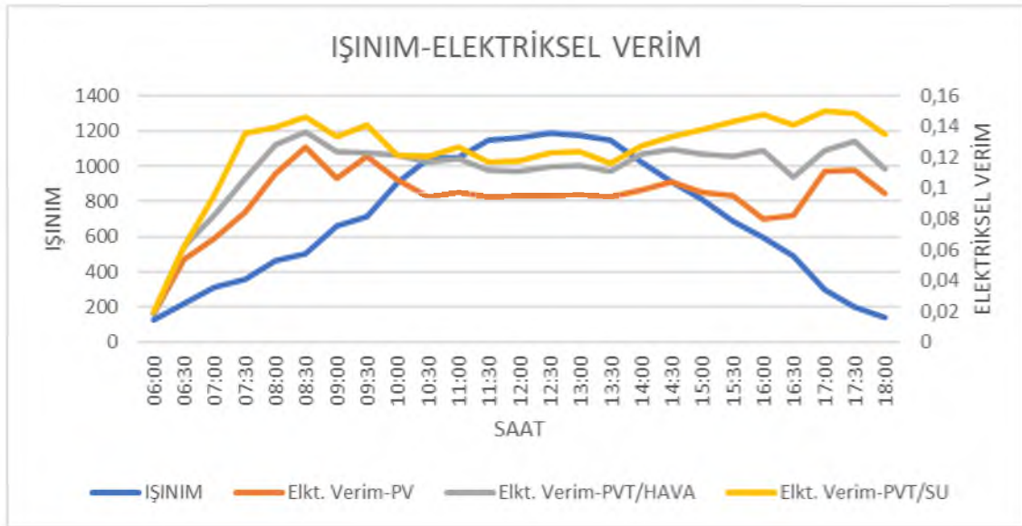
Şekil 5.17. 0.032 l/s, 3mm kalınlıkta ısıtım-elektriksel verim grafiği
