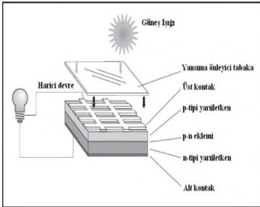
Şekil 3.2. PV sistemin parçaları (Anonim,2008b)
