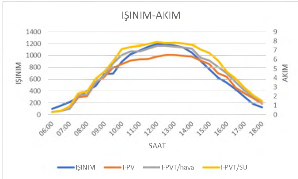
Şekil 5.25. Işınım-Akım grafiği
