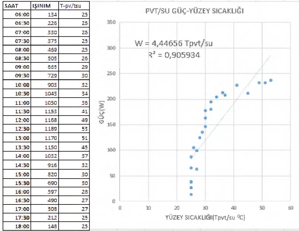
Şekil 5.37. PV/T-Su için güç-yüzey sıcaklığı
