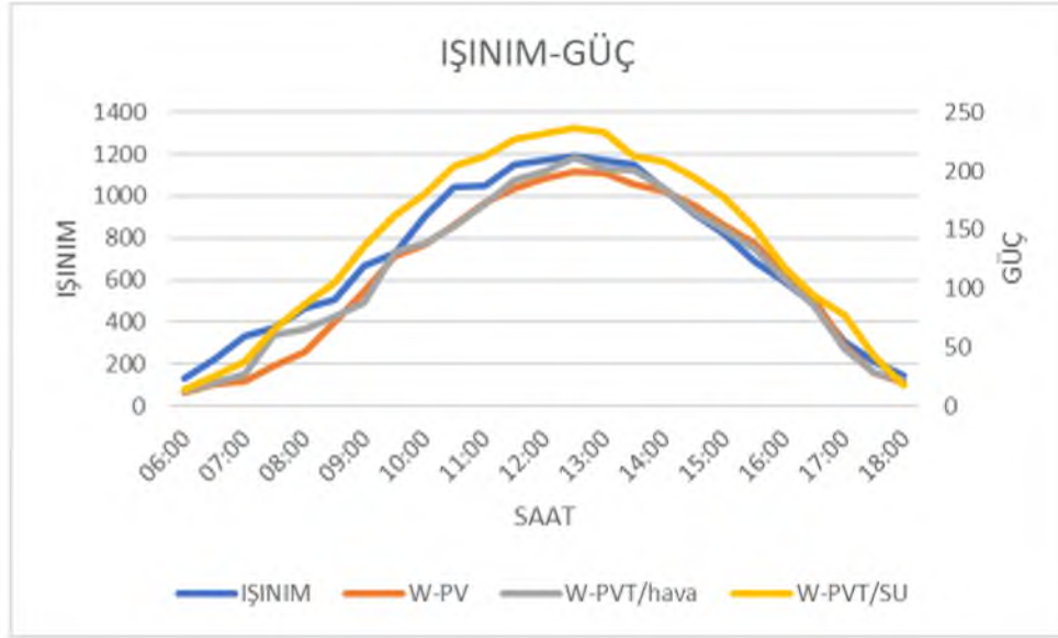
Şekil 5.7. Debi 0.032 l/s., kanal yüksekliği 5mm'de Işınım-Güç grafiği
