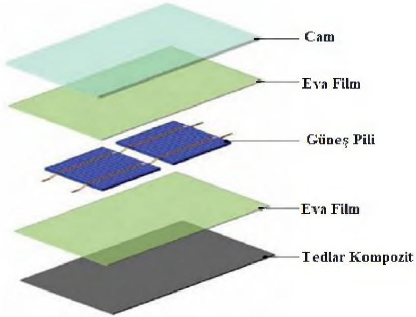
Şekil 3.3. Panel katmanları
