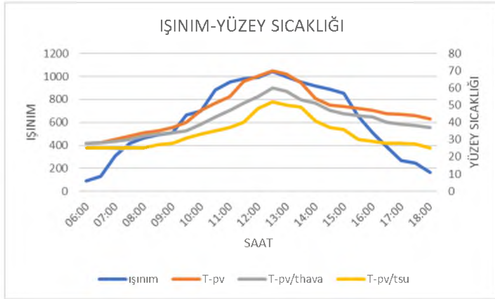
Şekil 5.19. 0.032 l/s, 3mm kalınlıkta ısıtım-yüzey sıcaklığı grafiği
