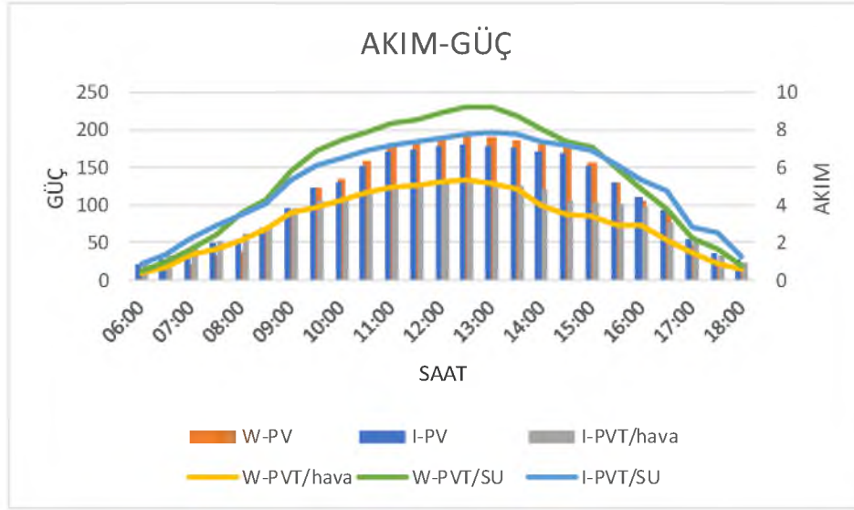
Şekil 5.3. Debi 0.016 l/s, kanal yüksekliği 5mm’de Güç-Akım grafiği
