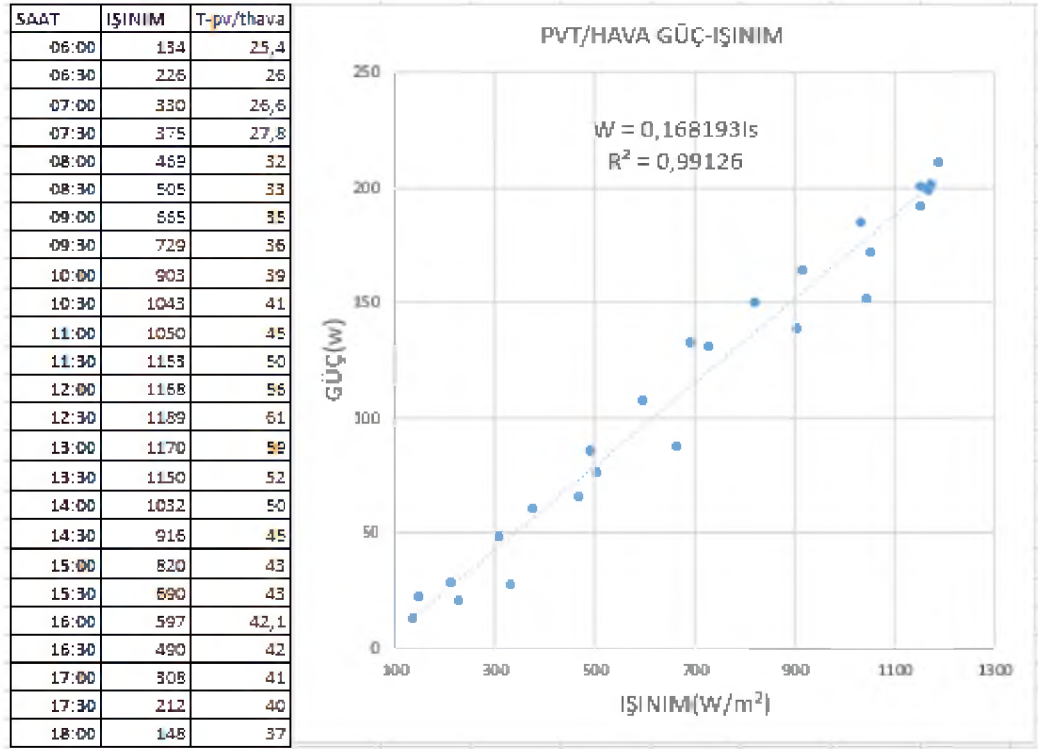
Şekil 5.33. PV/T-Hava için güç-ışınım
