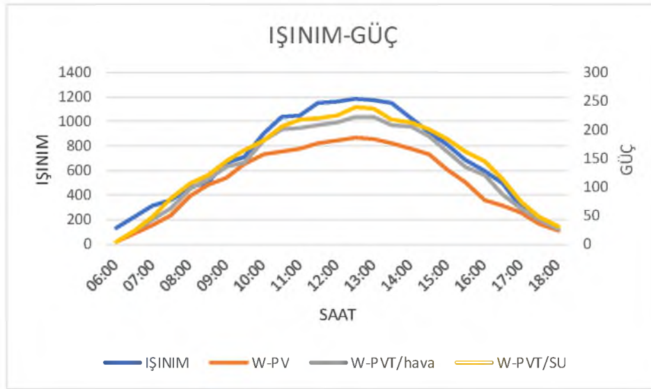
Şekil 5.16. 0.032 l/s, 3mm kalınlıkta ısıtım-güç grafiği
