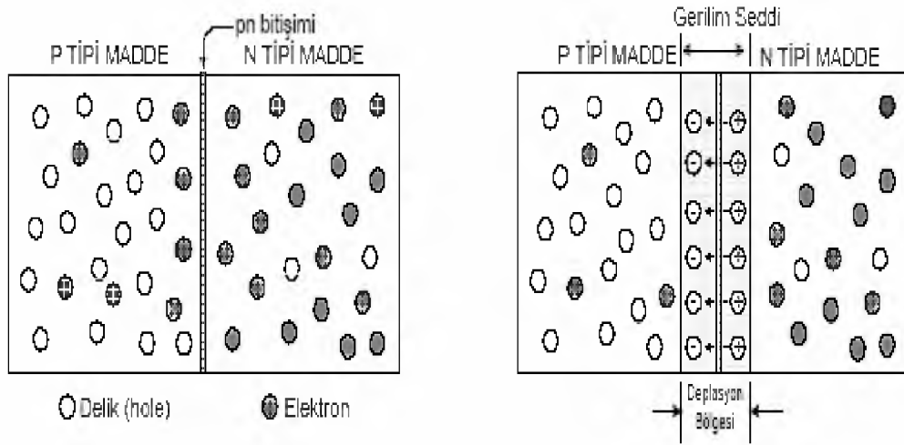
Şekil 3.7. P – N Kavşağının Oluşumu (Karamanav,2007)
