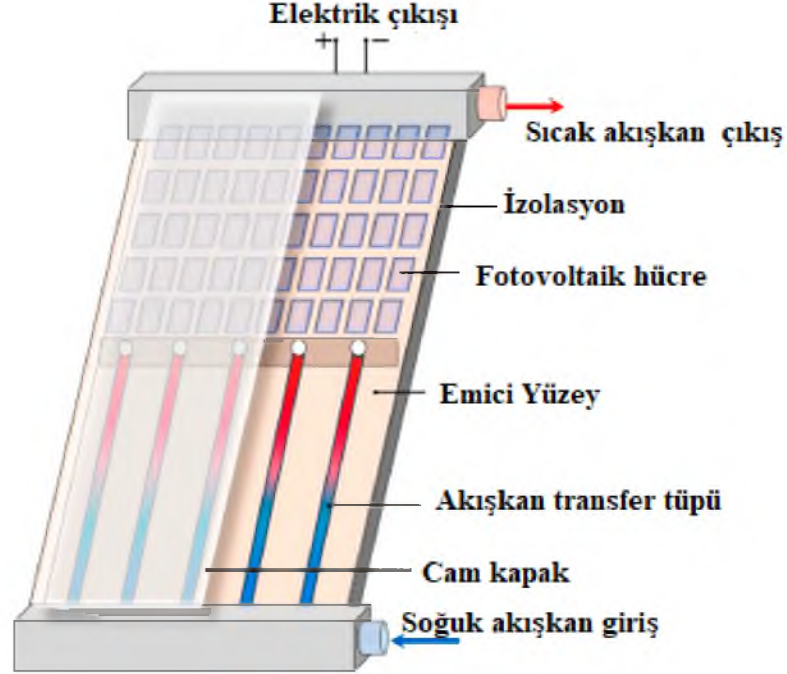
Şekil 3.14. Hibrid fotovoltaik-termal kollektör (Chow, 2010)
