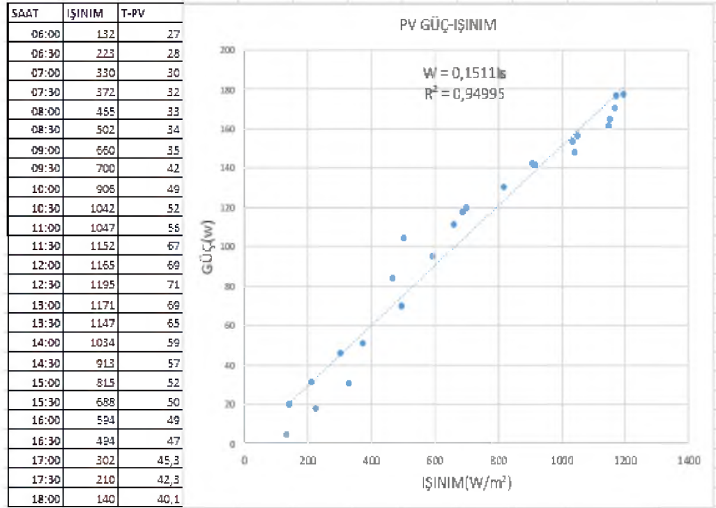
Şekil 5.38. PV için güç-ışınım
