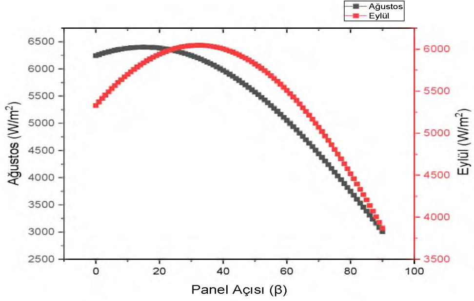
Şekil 4.31. Ağustos ve eylül Ayları optimum açışınım ilişkisi
