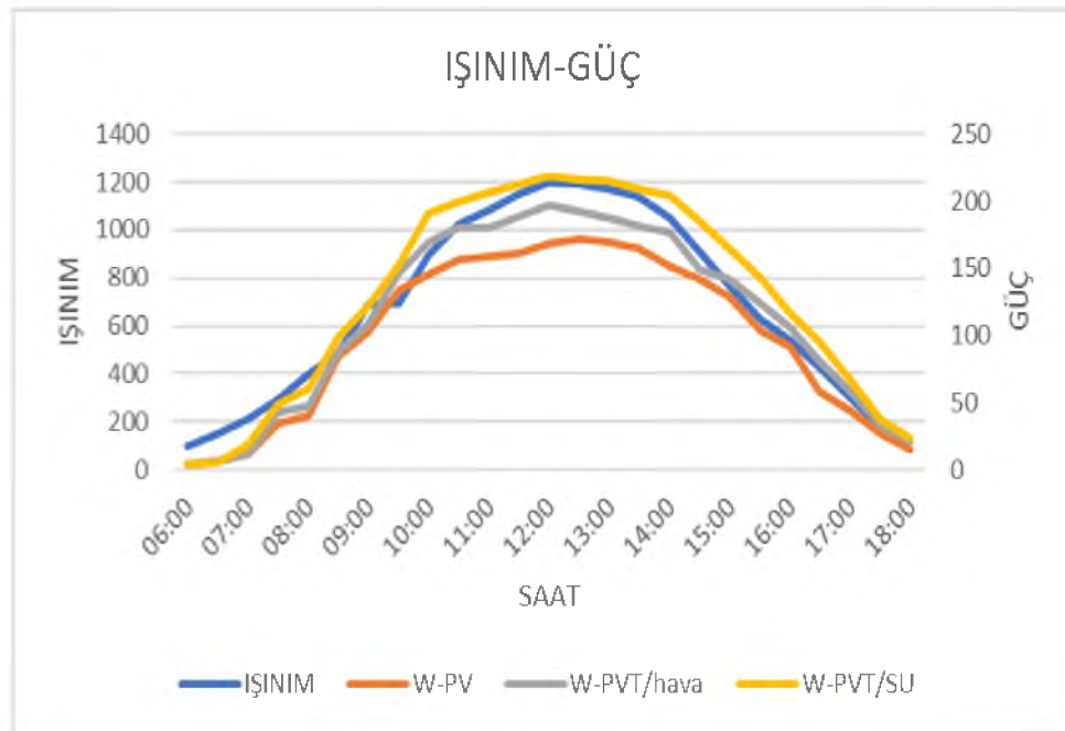
Şekil 5.23. Işınım-güç grafiği
