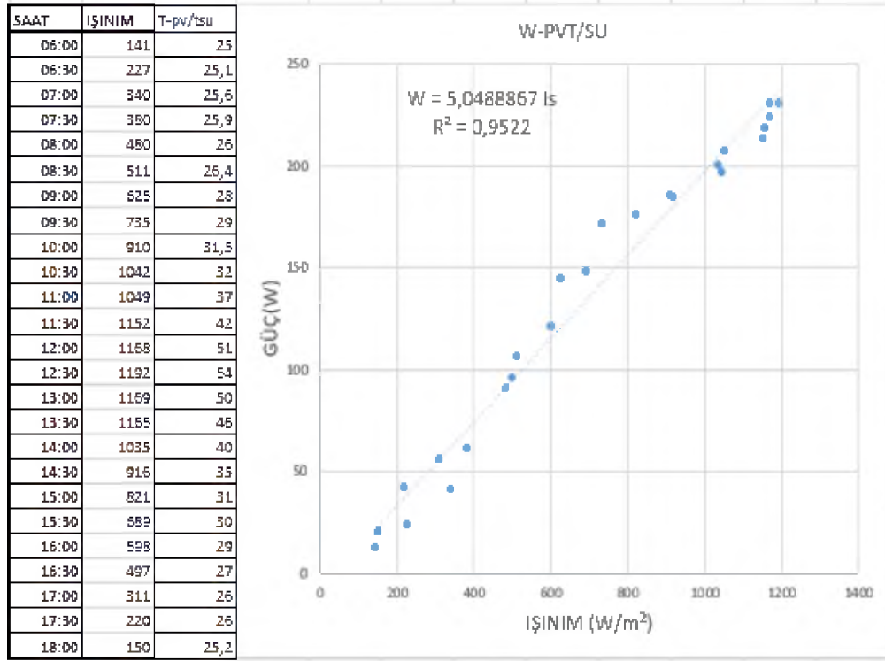
Şekil 5.28. PV/T-Su için güç-ışınım ilişkisi
