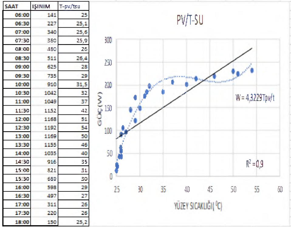
Şekil 5.31. PV/T-Su için güç-yüzey sıcaklığı
