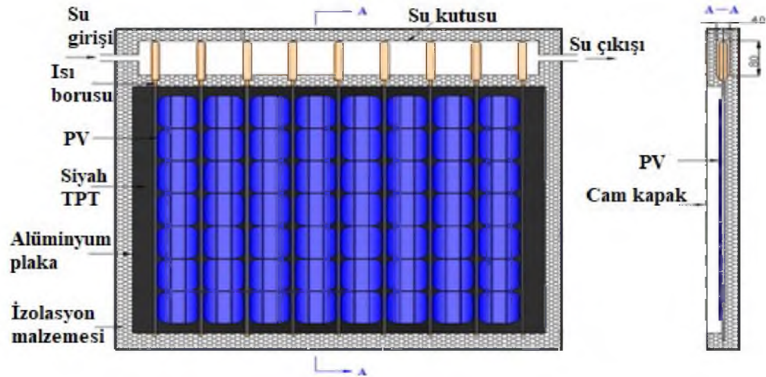
Şekil 3.15. Bir HP-PV/t güneş kollektör şematik diyagramı (Pei, 2012)
