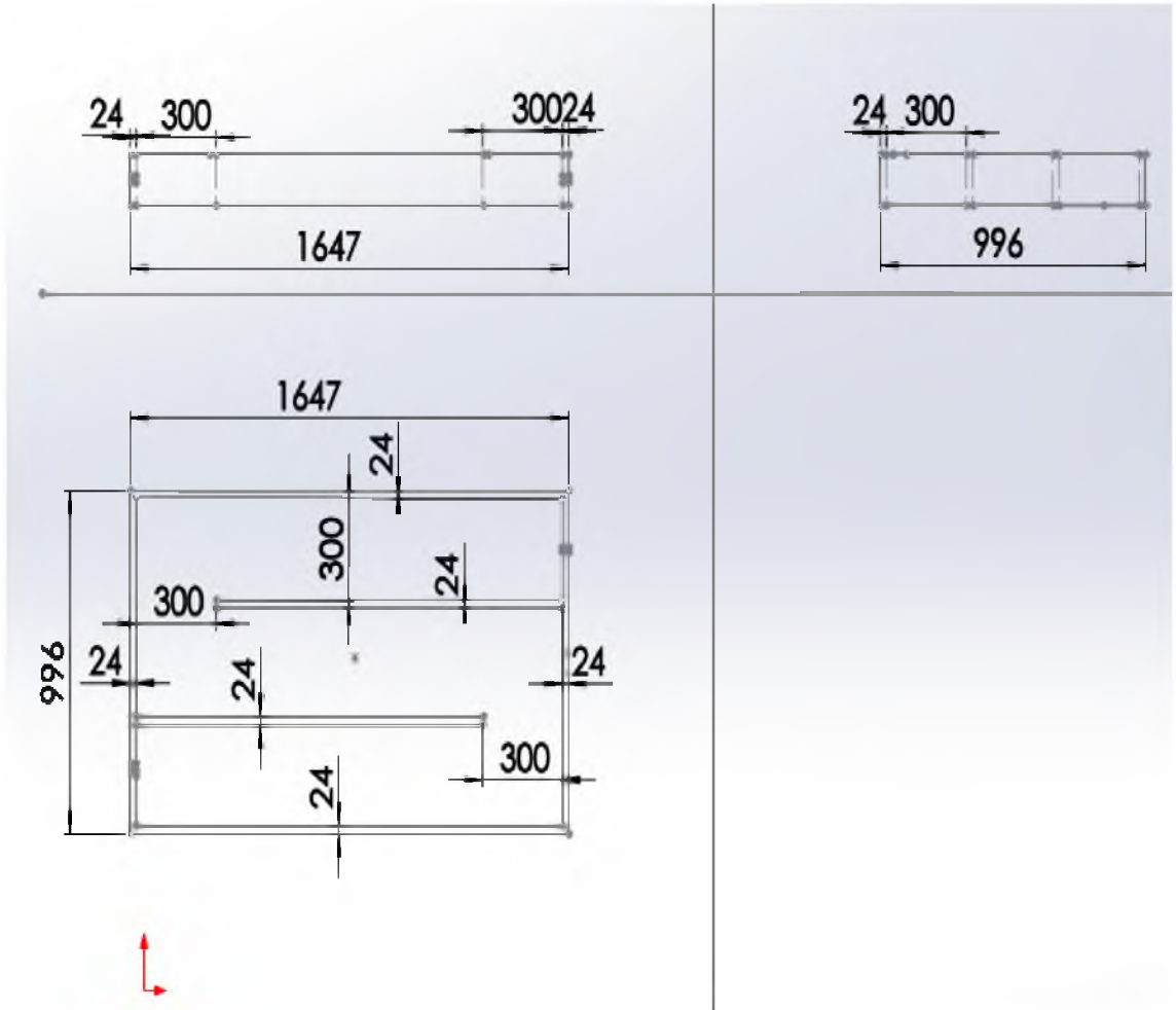
Şekil 4.37. Deney düzeneğinin teknik resmi
