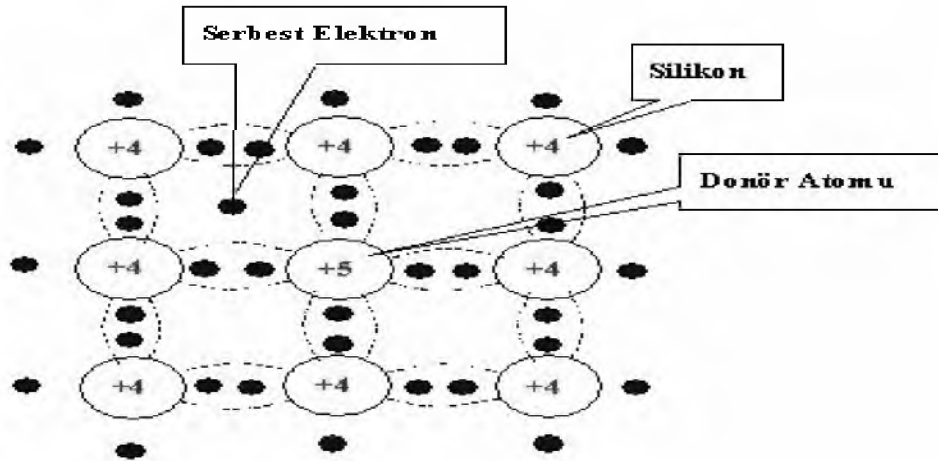
Şekil 3.5. Bir n tipi yarıiletken (Karamanav, 2007)
