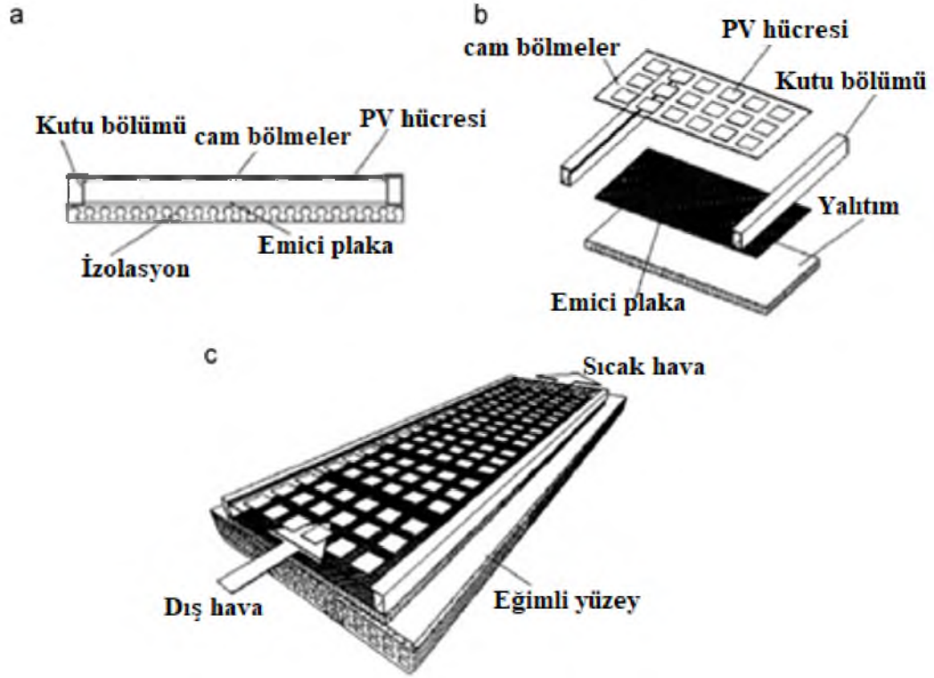
Şekil 3.12. PV/t hava toplayıcı (a) kesit görünümü. (B) montaj görünümü. (C) dizi görünümü
