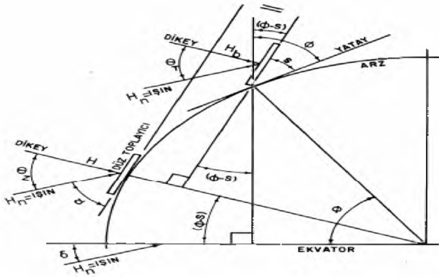
Şekil 4.22. Enlem açısı ve eğim açısı arasındaki ilişki (Anonim,2018e)
