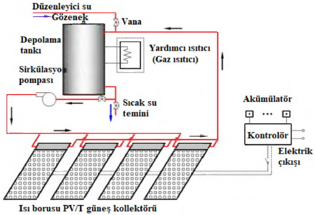
Şekil 3.16. HP-PV/T sisteminin şematik diyagramı (Pei, 2012)
