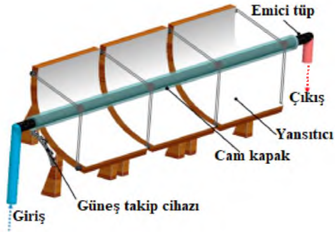
Şekil 2.4. Parabolik oluklu güneş enerji kollektörleri (Price, 2002)
