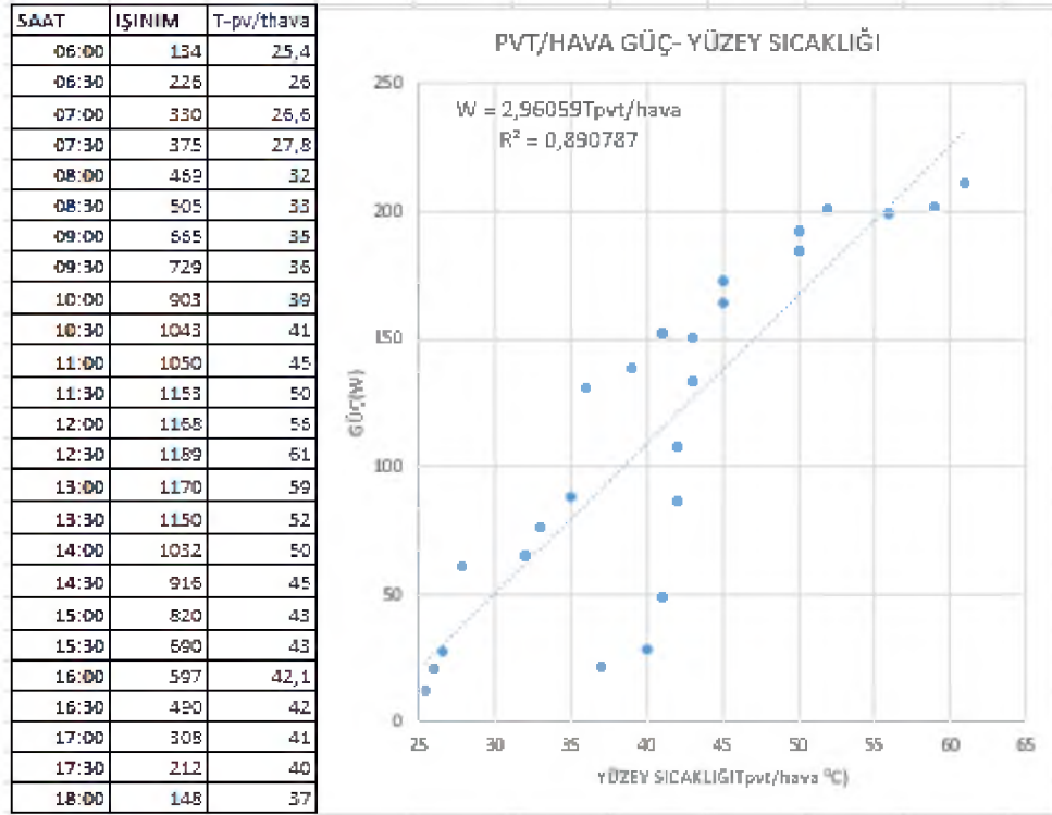
Şekil 5.36. PV/T-Hava için güç-yüzey sıcaklığı
