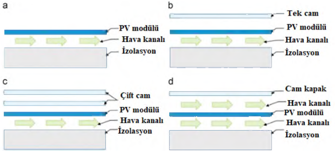
Şekil 3.11. (a) hava PV/t kollektör. (b) tek camlı hava PV/t kollektör. (c) çift camlı hava PV/t kollektör. (d) çift geçişli camlı hava PV/t kollektör (Kalogirou,2006)
