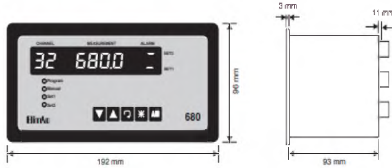
Şekil 4.4. Datalogger Teknik çizimi
