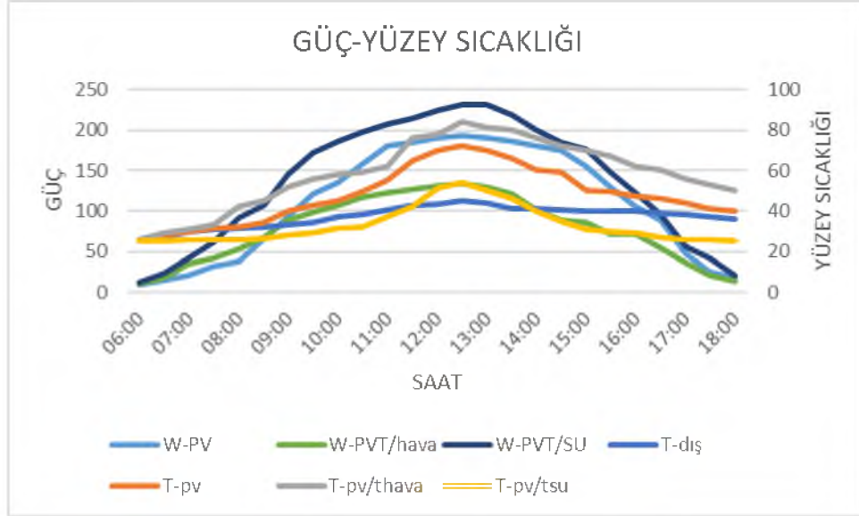
Şekil 5.5. Debi 0.016 l/s, kanal yüksekliği 5mm'de Güç-Yüzey Sıcaklığı
