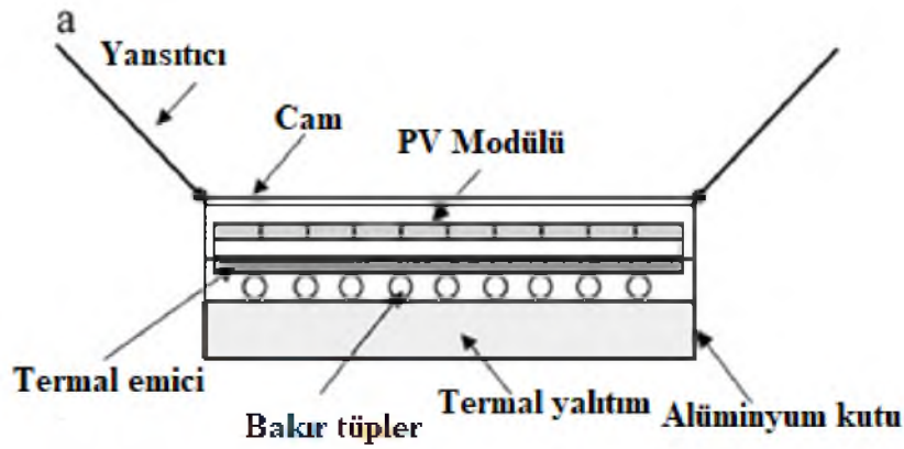
Şekil 3.19. Yoğunlaştırıcı PV/T kolektörü (Tyagi,2012)
