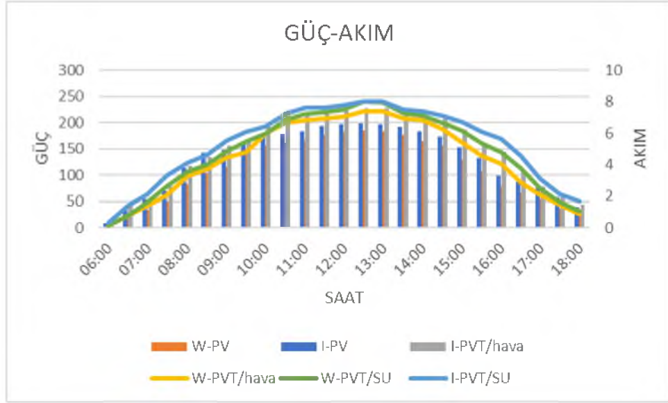
Şekil 5.18. 0.032 l/s, 3mm kalınlıkta güç-akım grafiği
