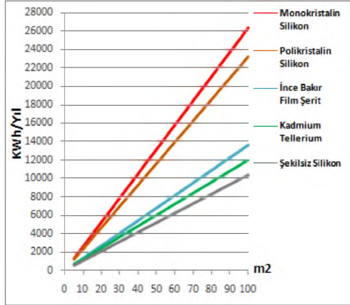
Şekil 4.19. Merkez PV Tipi-Alan-Üretililecek Enerji (KWh-Yıl) (Anonim,2018d)
