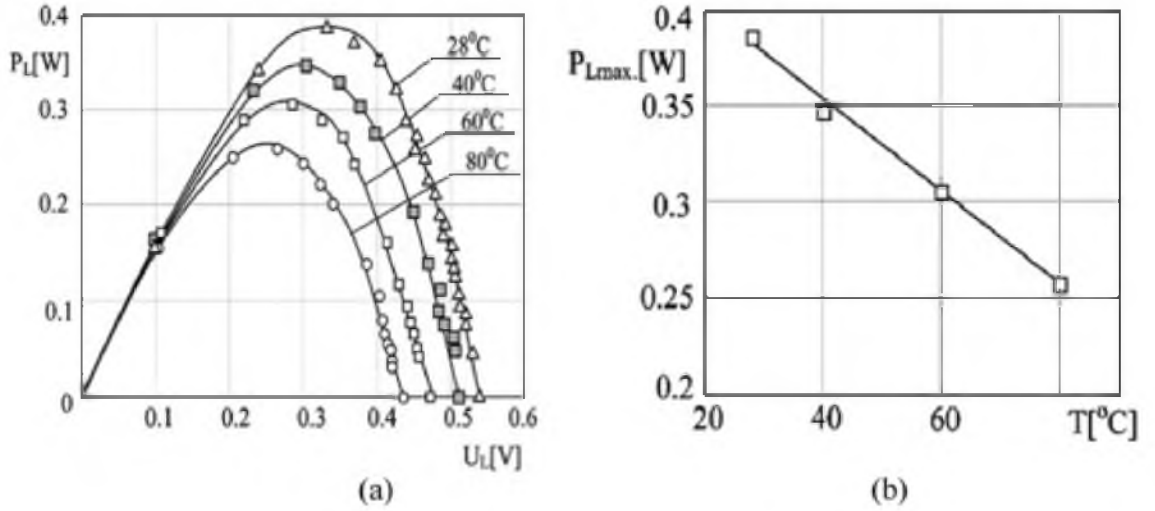
Şekil 3.9. (a) Farklı çalışma sıcaklıklarında tek kristalli silikon PV hücrelerinin çıkış gücü(b) maksimum çıkış gücünün sıcaklıkla olan ilişkisi (E. Radziemska,2003)
