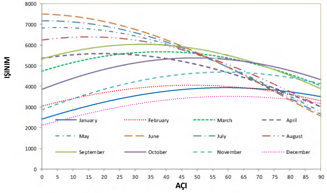
Şekil 4.29. Batman İli için eğim açısı yıllık grafiği
