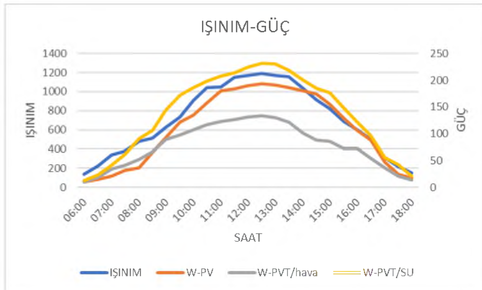
Şekil 5.1. Debi 0.016 l/s, kanal yüksekliği 5mm'de Işınım-Güç grafiği
