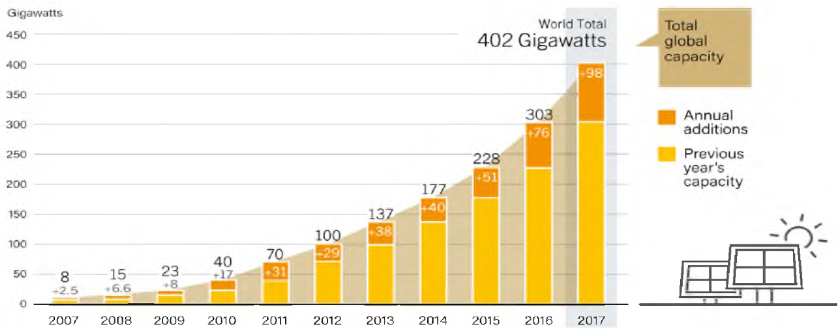
Şekil 3.23. Dünya geneli PV sistemler ile elde edilen elektrik enerjisi artışı (Anonim, 2018 c)
