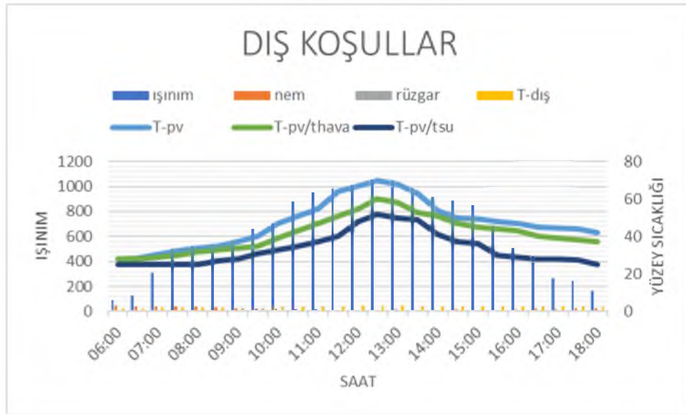
Şekil 5.21. 0.032 l/s, 3mm kalınlıkta ışıınım, sıcaklık, nem, rüzgâr etkisi
