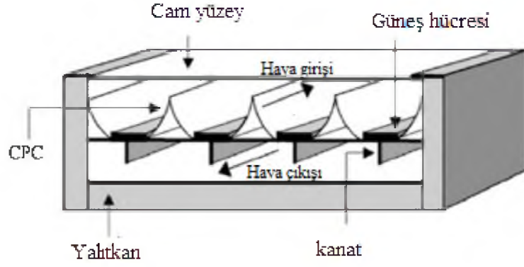
Şekil 1.7. Çift geçişli CPC ve kanallı termal güneş kolektörü (Othman, 2005).
