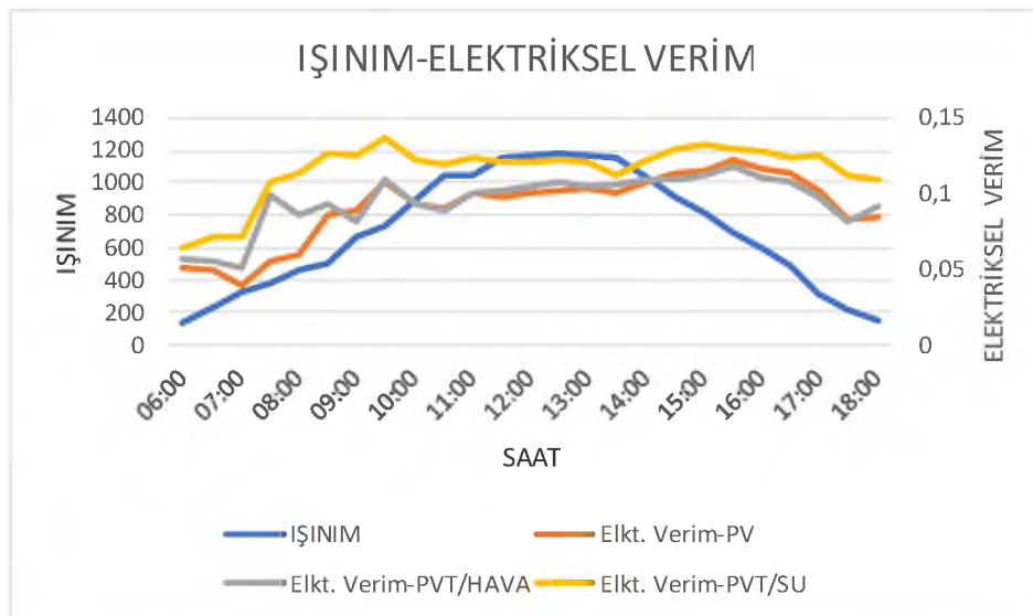
Şekil 5.8. Debi 0.032 l/s, kanal yüksekliği 5mm'de elektriksel verim grafiği
