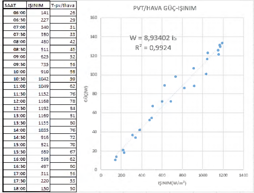
Şekil 5.27. PV/T-Hava için güç-ışınım ilişkisi
