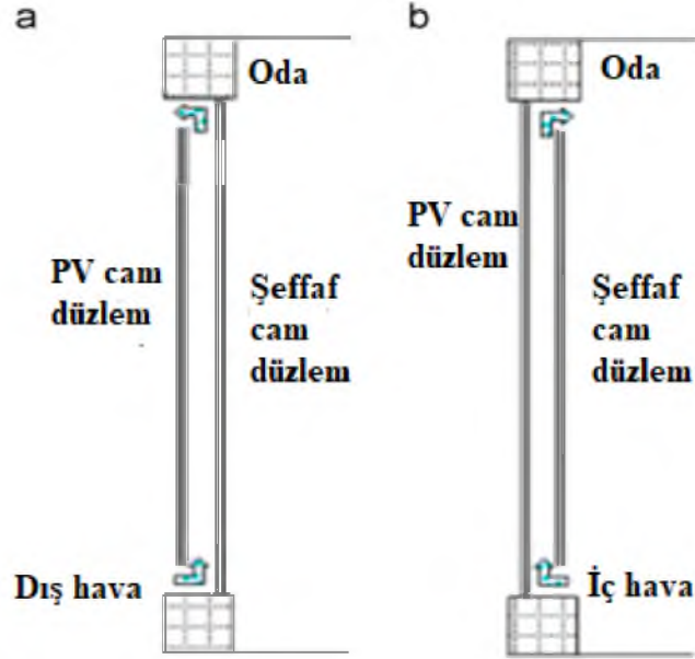
Şekil 3.17. Entegre PV/T sistemleri oluşturmak için havalandırılmalı PV sırlama işlemi (a) soğutma modu. (B) ısıtma modu (H Wei,2014)
