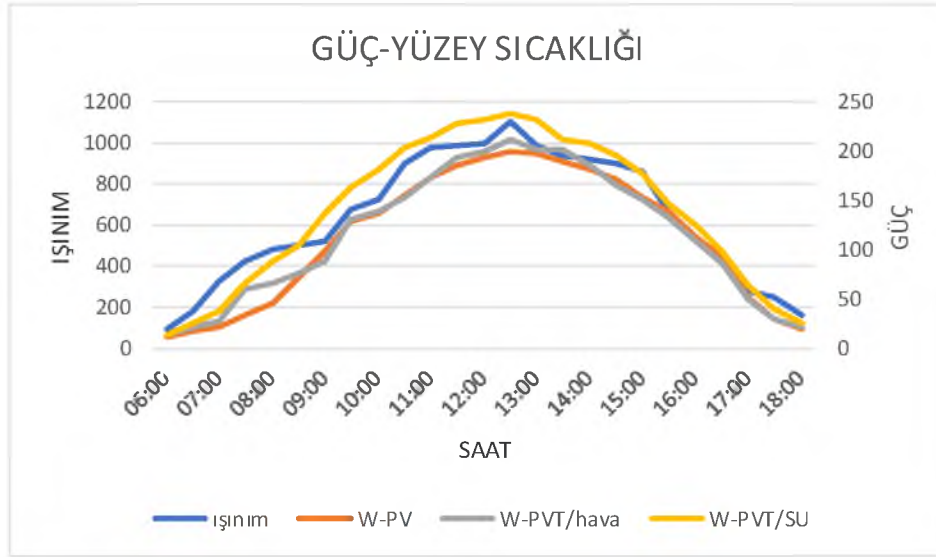
Şekil 5.11. Debi 0.032 l/s, kanal yüksekliğı 5mm’de Güç- ışıınım grafiğı
