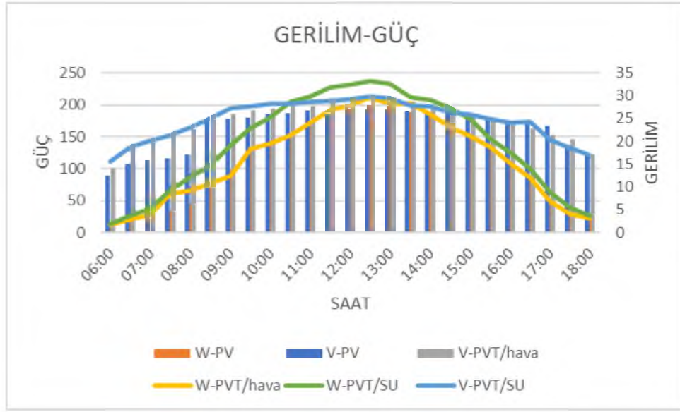
Şekil 5.9. Debi 0.032 l/s, kanal yüksekliği 5mm'de Gerilim-Güç grafiği
