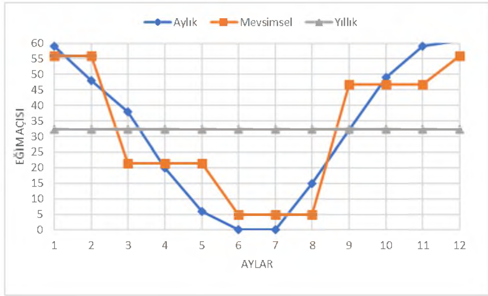
Şekil 4.28. Batman şartlarında aylara göre \beta (Eğim Açısı)
