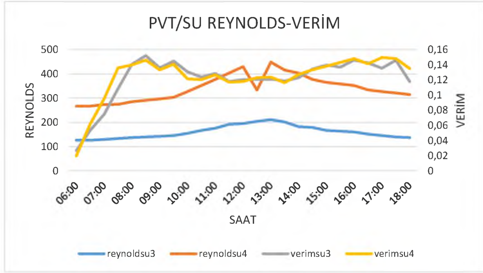
Şekil 5.50. 3mm kalınlıktaki su soğutmalı sistemin Reynolds sayısı ve verim karşılaştırması
