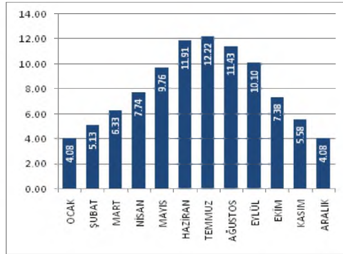
Şekil 4.18. Merkez Güneşlenme Süreleri (Saat) (Anonim,2018d)
