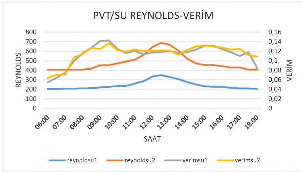
Şekil 5.49. 5mm kalınlıktaki su soğutmalı sistemin Reynolds sayısı ve verim karşılaştırması
