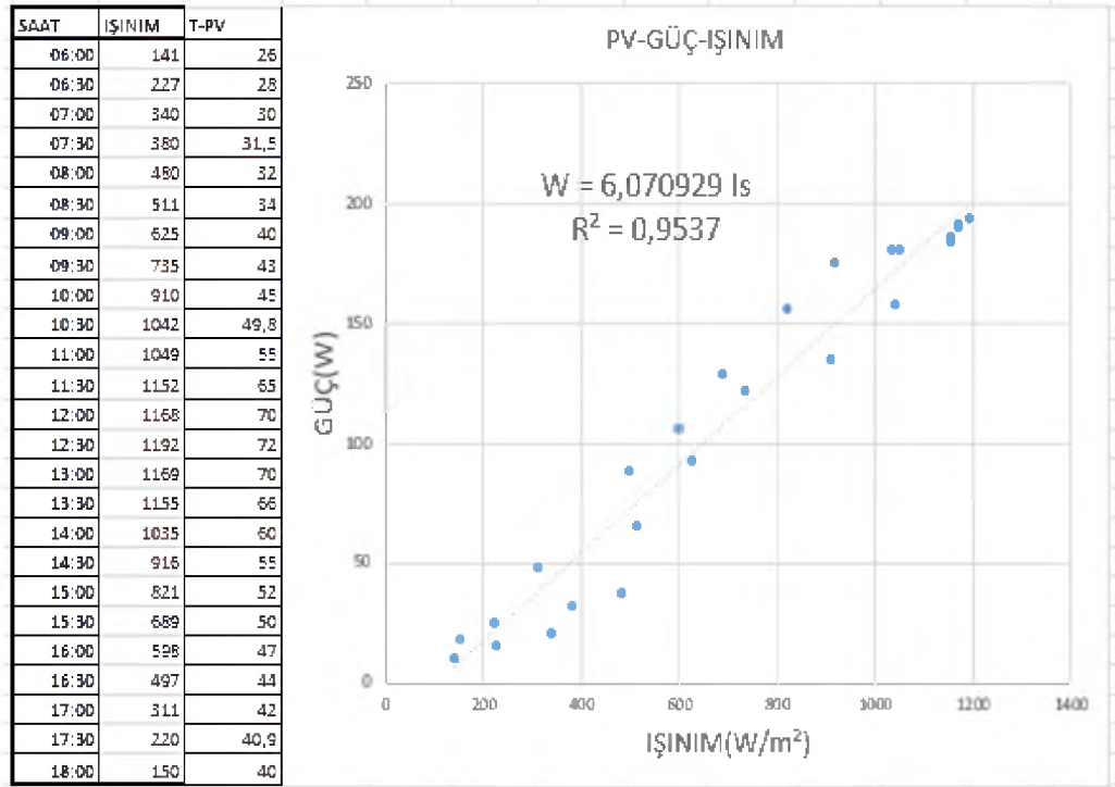
Şekil 5.26. PV için güç-ışınım ilişkisi
