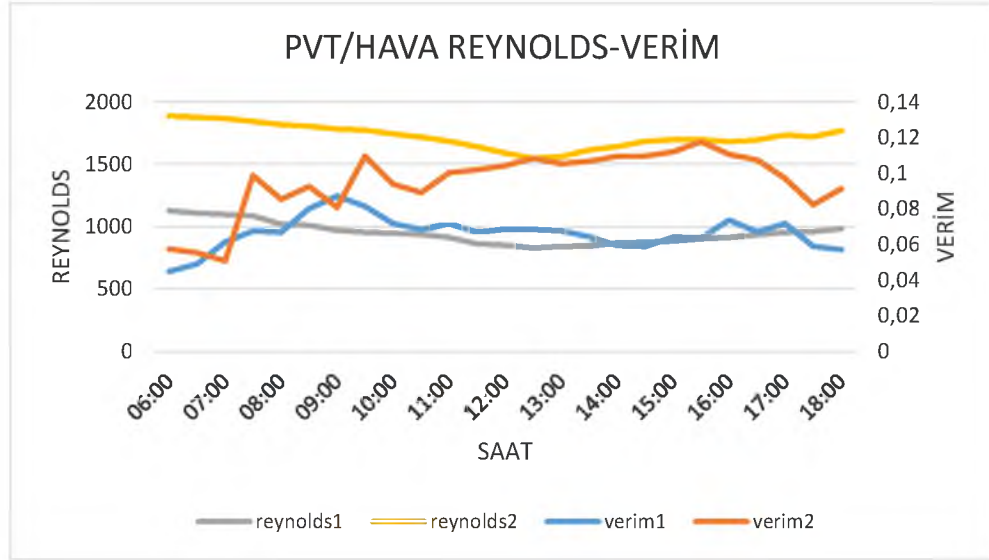
Şekil 5.47. Hava soğutmalı sistemde Reynolds sayısı verim karşılaştırması
