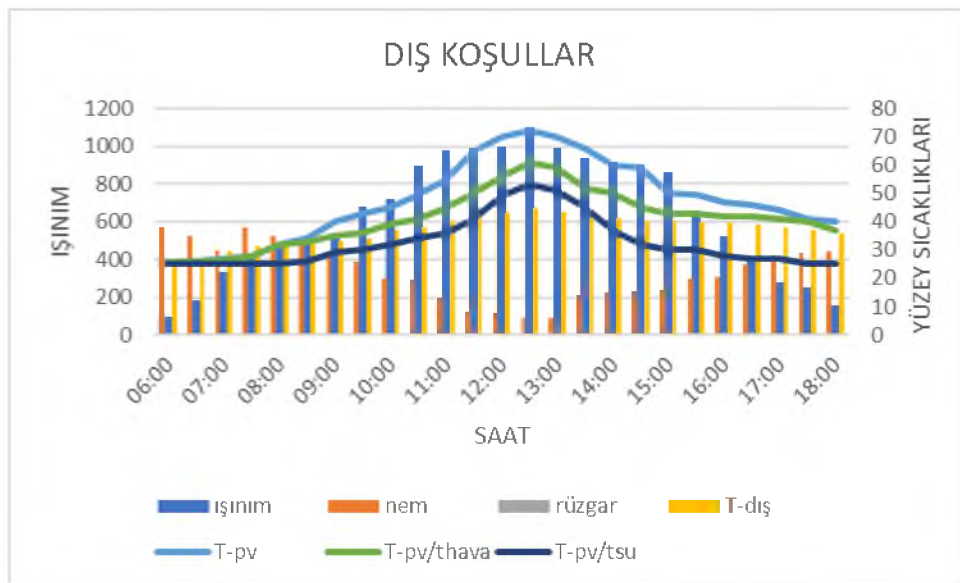
Şekil 5.12. Debi 0.032 l/s, kanal yüksekliğı 5mm’de nem, sıcaklık, rüzgâr, etkisi
