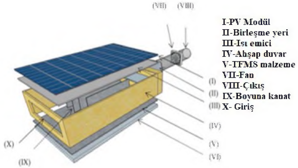
Şekil 1.5. PV/T örneği (Ahmed, 2018)
