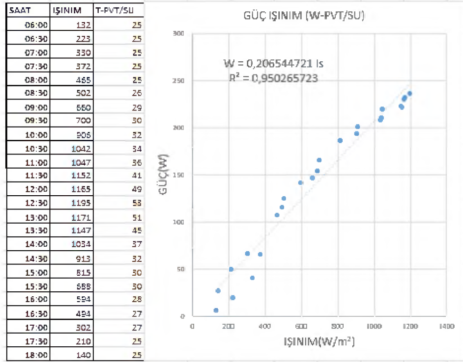
Şekil 5.40. PV/T-Su için güç-ışınım
