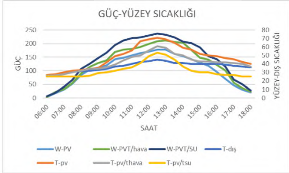
Şekil 5.15. 0.016 l/s, 3mm kalınlıkta güç-yüzey sıcaklığı grafiği
