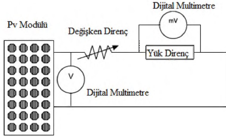
Şekil 4.36. Deney düzeneğinin şematik görünümü
