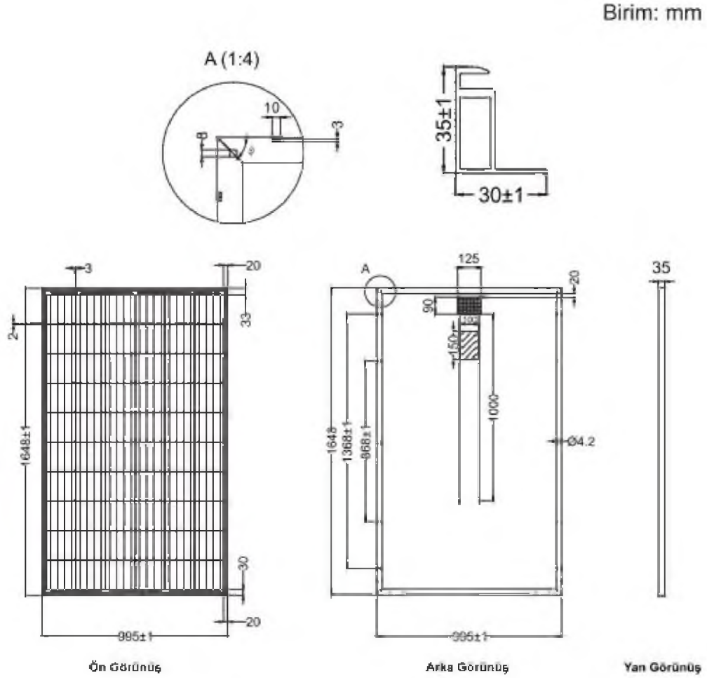
Şekil 4.1. Deneyde kullanılan panelin teknik resim çizimi
