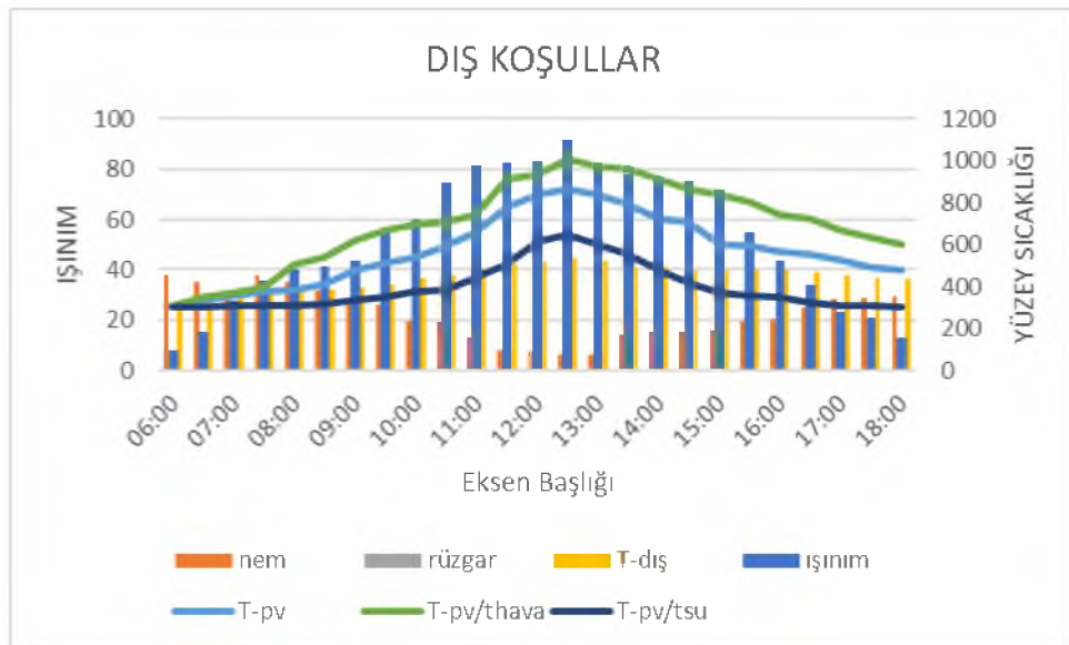
Şekil 5.6. Debi 0.016 l/s, kanal yüksekliği 5mm'de nem, rüzgâr, sıcaklık etkisi
