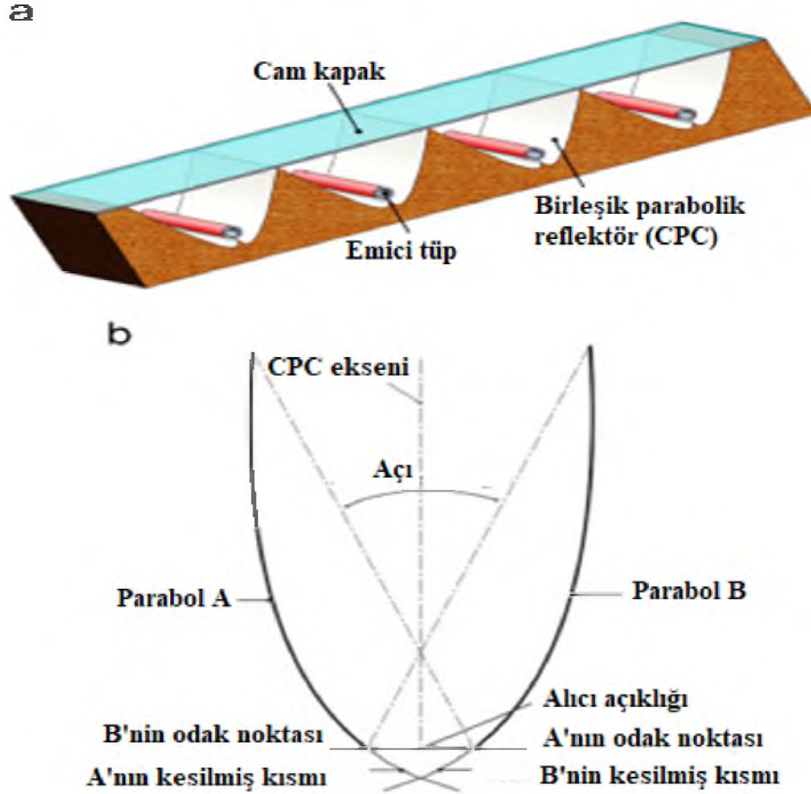
Şekil 2.3. Bileşik parabolik kolektör: (a) 3D görünümü ve (b) 2D şematik (Price, 2002)
