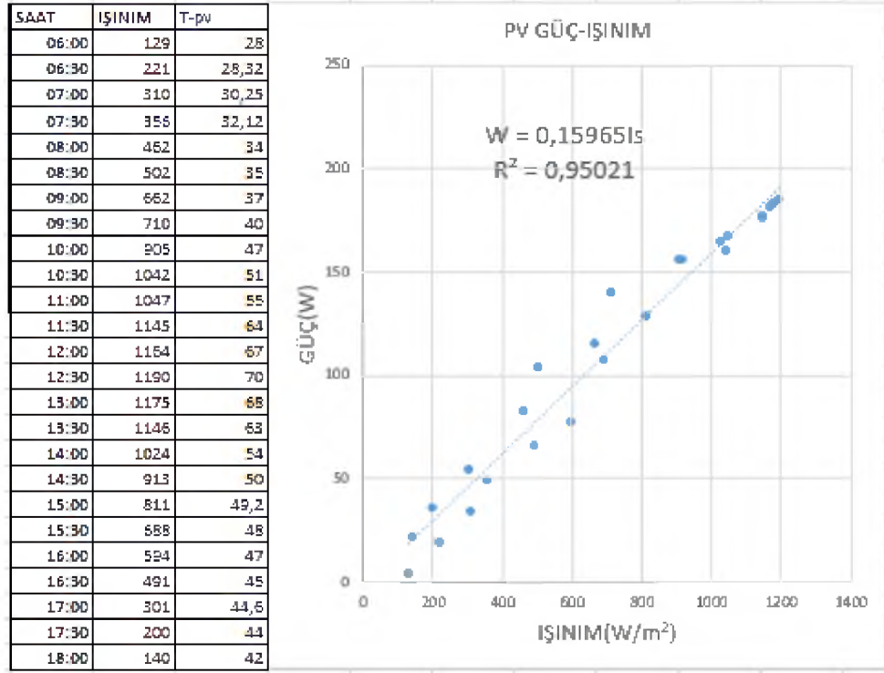
Şekil 5.44. PV için güç-ışınım
