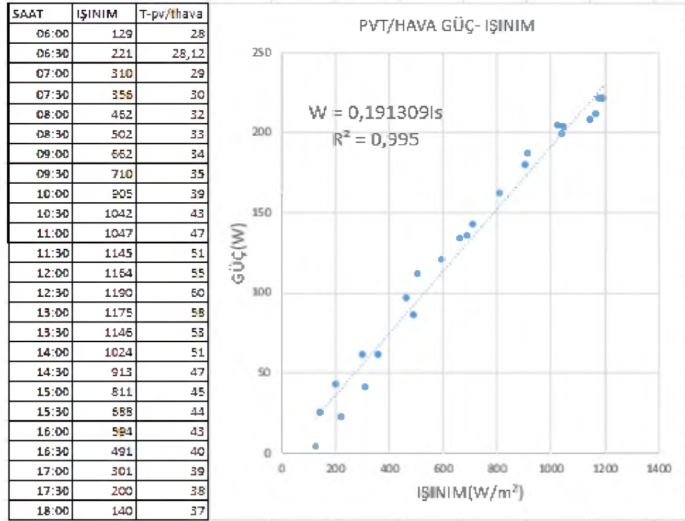
Şekil 5.45. PV/T-Hava için güç-ışınım
