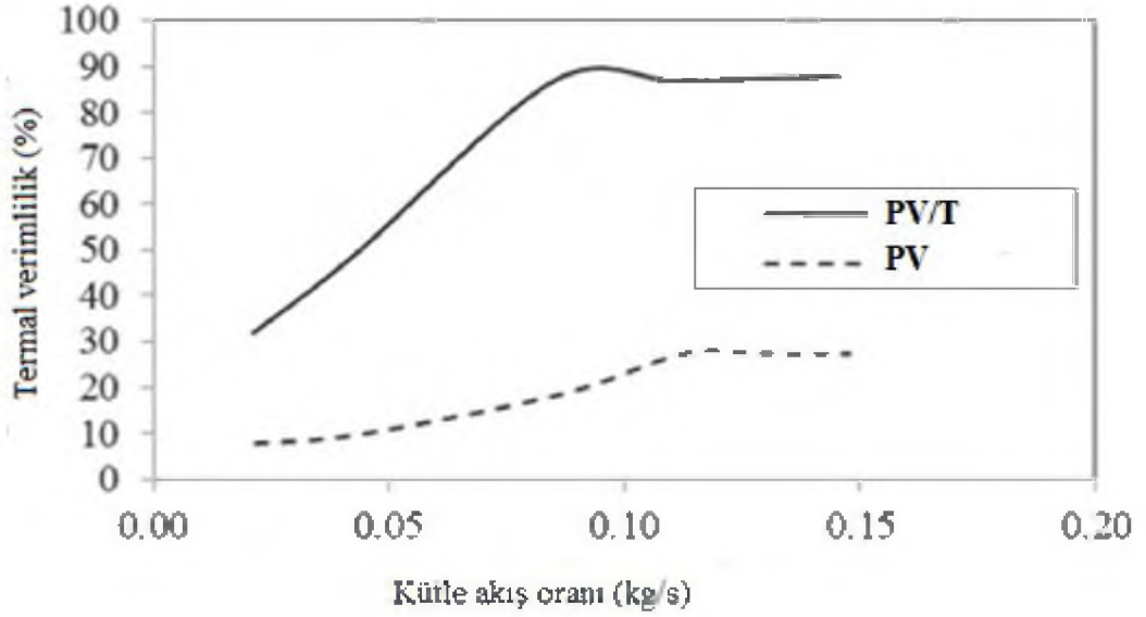
Şekil 3.22. Her iki toplayıcının da termal verimliliği (F. Hussain,2013)
