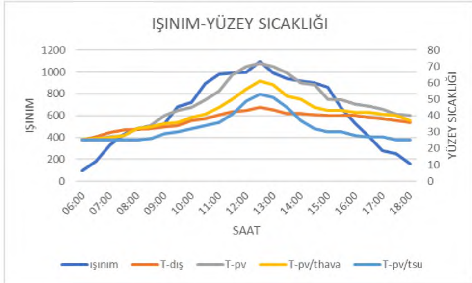
Şekil 5.10. Debi 0.032 l/s, kanal yüksekliği 5mm'de Işınım-Yüzey sıcaklığı grafiği
