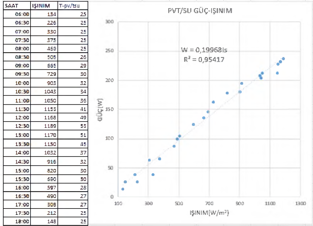
Şekil 5.34. PV/T-Su için güç-ışınım
