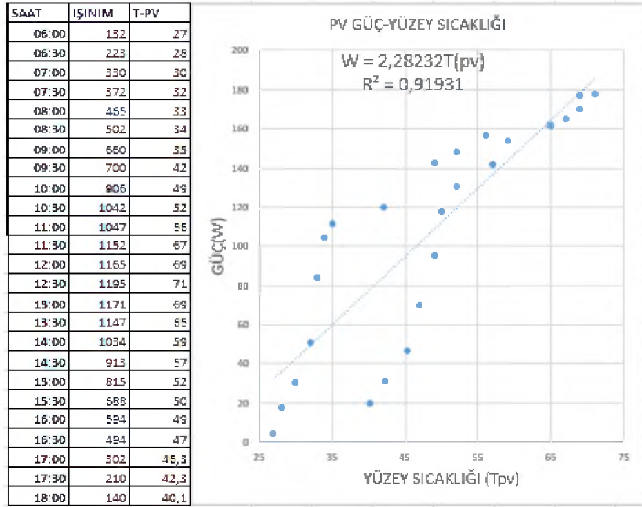
Şekil 5.41. PV için güç-yüzey sıcaklığı
