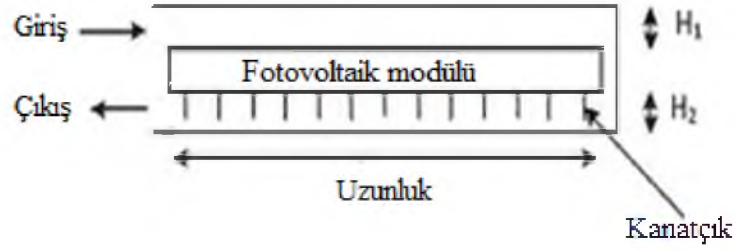
Şekil 1.4. Yüzgeç kullanımı (Kumar,2015)
