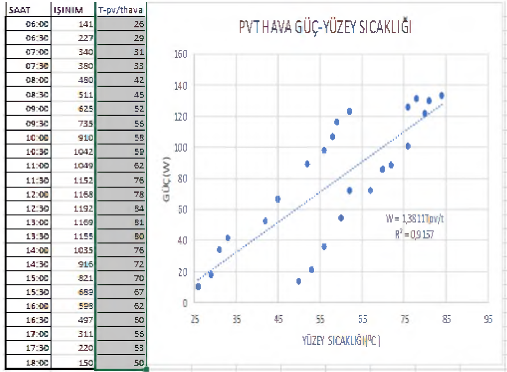
Şekil 5.30. PV/T-Hava için güç-yüzey sıcaklığı
