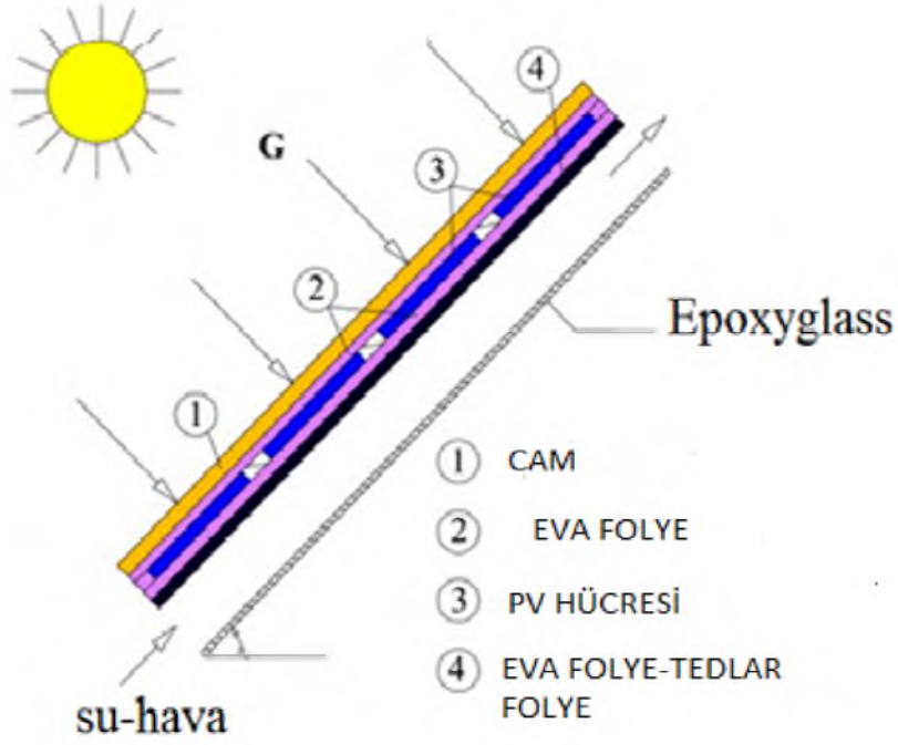
Şekil 4.35. Sistemin yandan görünümü
