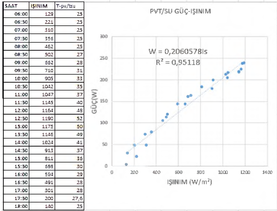
Şekil 5.46. PV/T-Su için güç-ışınım
