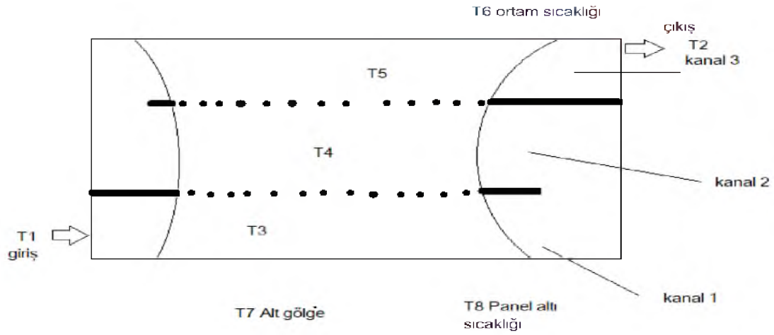
Şekil 4.34. Sistemin sıcaklık noktaları
