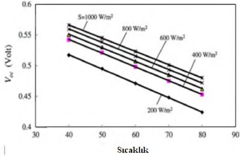
Şekil 3.8. PV hücre kavşak sıcaklığı ile açık devre voltajı değişimi(B.J. Huang,2011)
