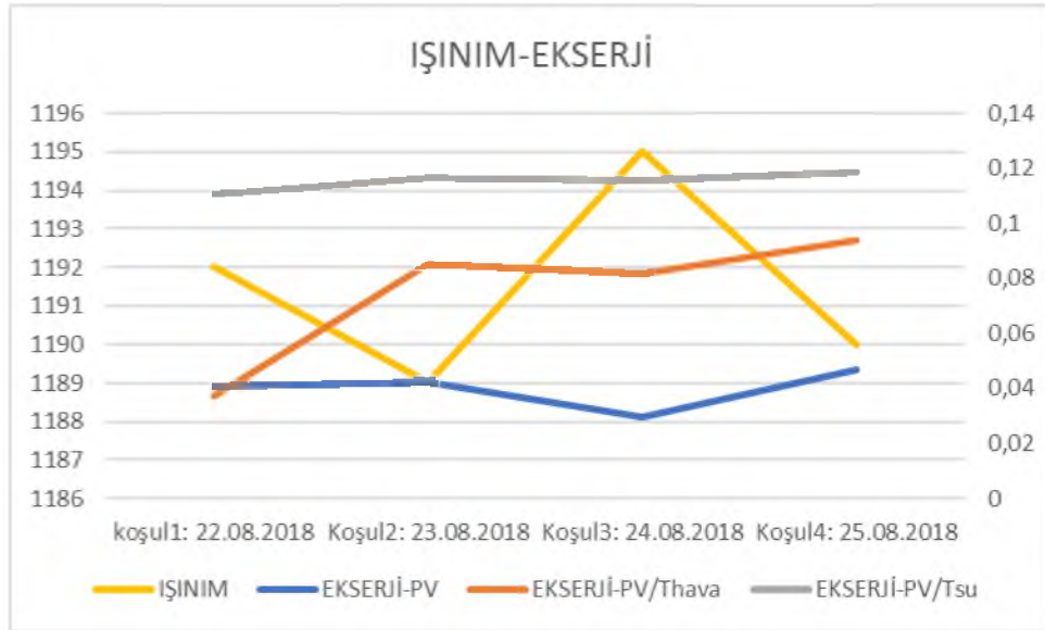
Şekil 5.22. Farklı İşinım altında ekserji analizi
