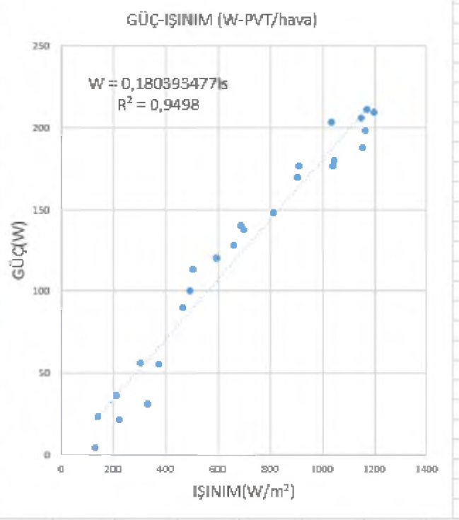
Şekil 5.39. PV/T-Hava için güç-ışınım
