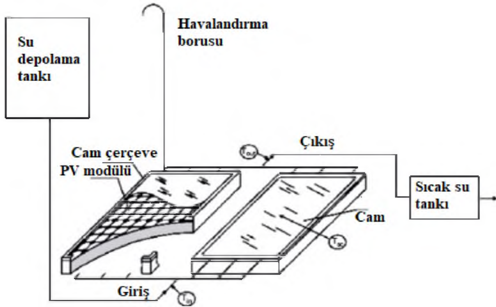
Şekil 3.13. PV/t su toplayıcı şematik diyagramı (V.V.Tyagi,2012)
