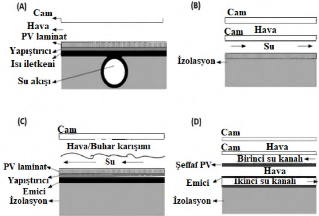
Şekil 3.20. Çeşitli toplayıcı kavramları: (A), tabaka-ve-borulu PV / T, (B), bir kanal PV / T, (C) serbest akış PV / T, (D), iki emici PV / T (yalıtımlı tip)(Zondag, 2003)
