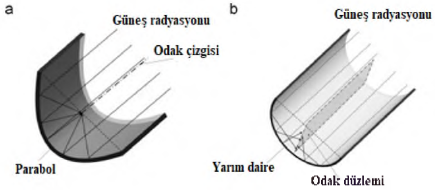
Şekil 2.5. Silindirik Oluklu Kollektörler (Price, 2002)
