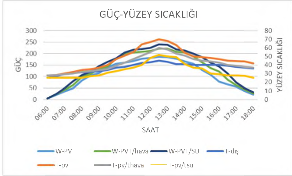
Şekil 5.20. 0.032 l/s, 3mm kalınlıkta güç-yüzey sıcaklığı grafiği
