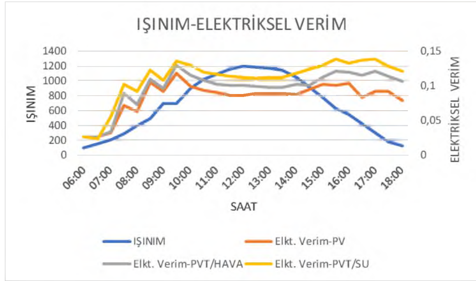
Şekil 5.24. Işınım-Elektriksel verim grafiği
