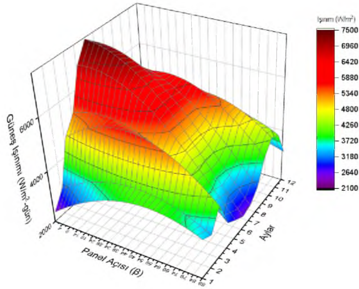
Şekil 4.30. Batman İli Yıllık panel açısı ışınlm değişim grafiği
