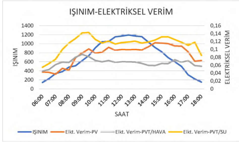
Şekil 5.2. Debi 0.016 l/s, kanal yüksekliği 5mm’de elektriksel verim grafiği
