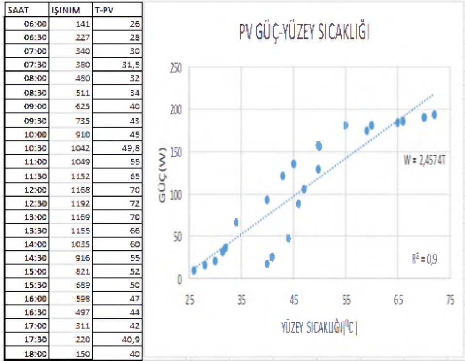
Şekil 5.29. PV için güç-yüzey sıcaklığı
