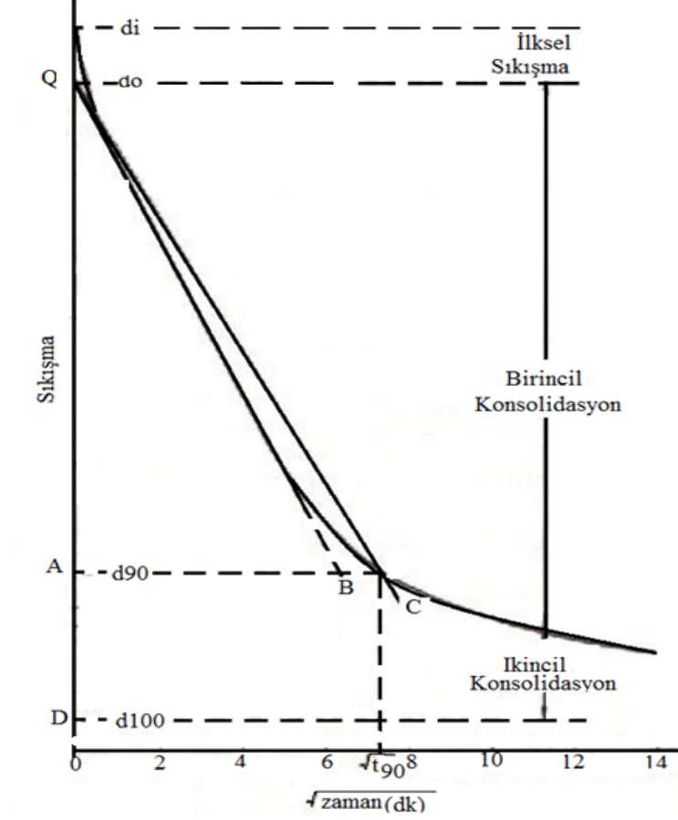
Şekil 2.7. Karekök yöntemi ile konsolidasyon katsayısının belirlenmesi [13, Uyarlanmıştır]
