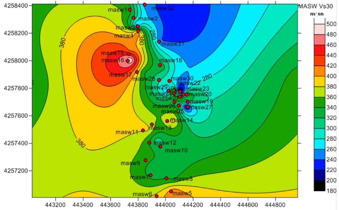
Şekil 3.11 Masw çalışması V_{s30} alansal dağılım haritası
