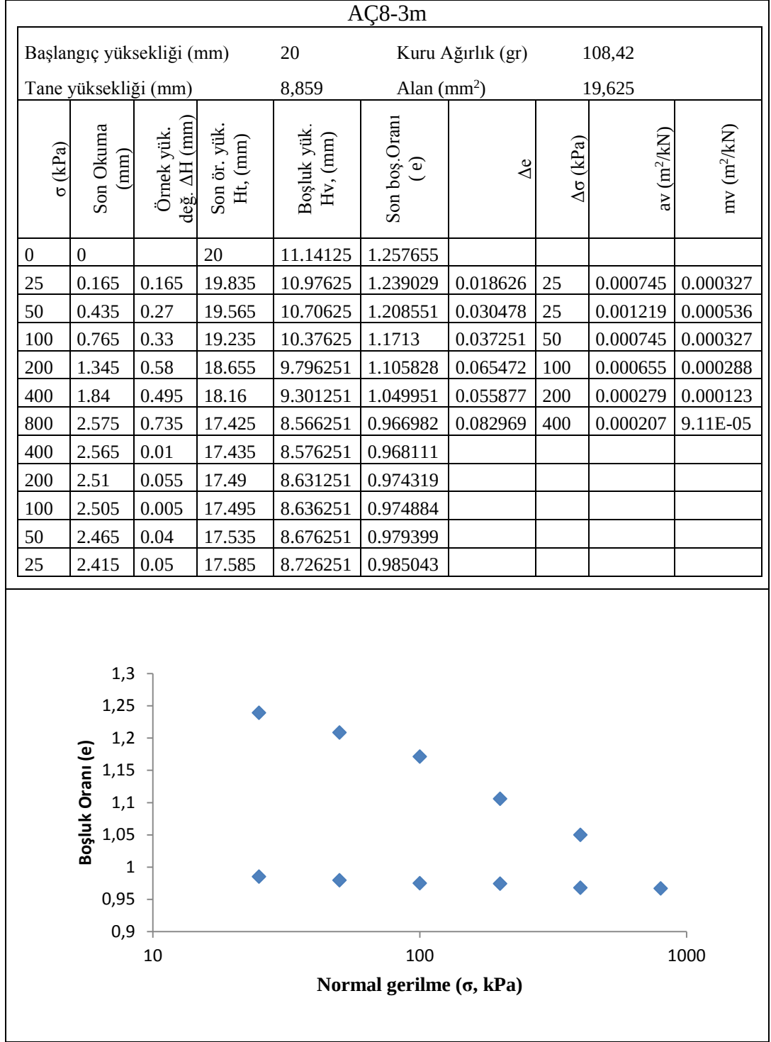
Şekil 4.35 8-3m e- \sigma Grafiği
