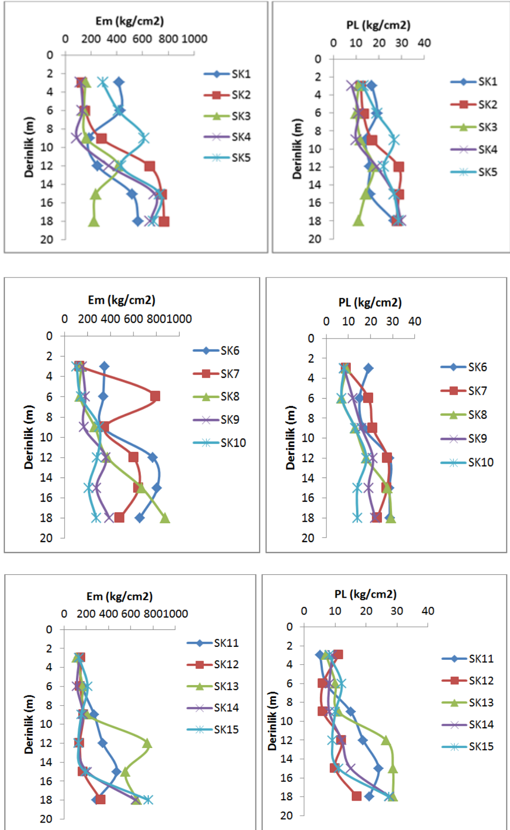
Şekil 4.21 Çalışma alanı Em ve PL değerleri
