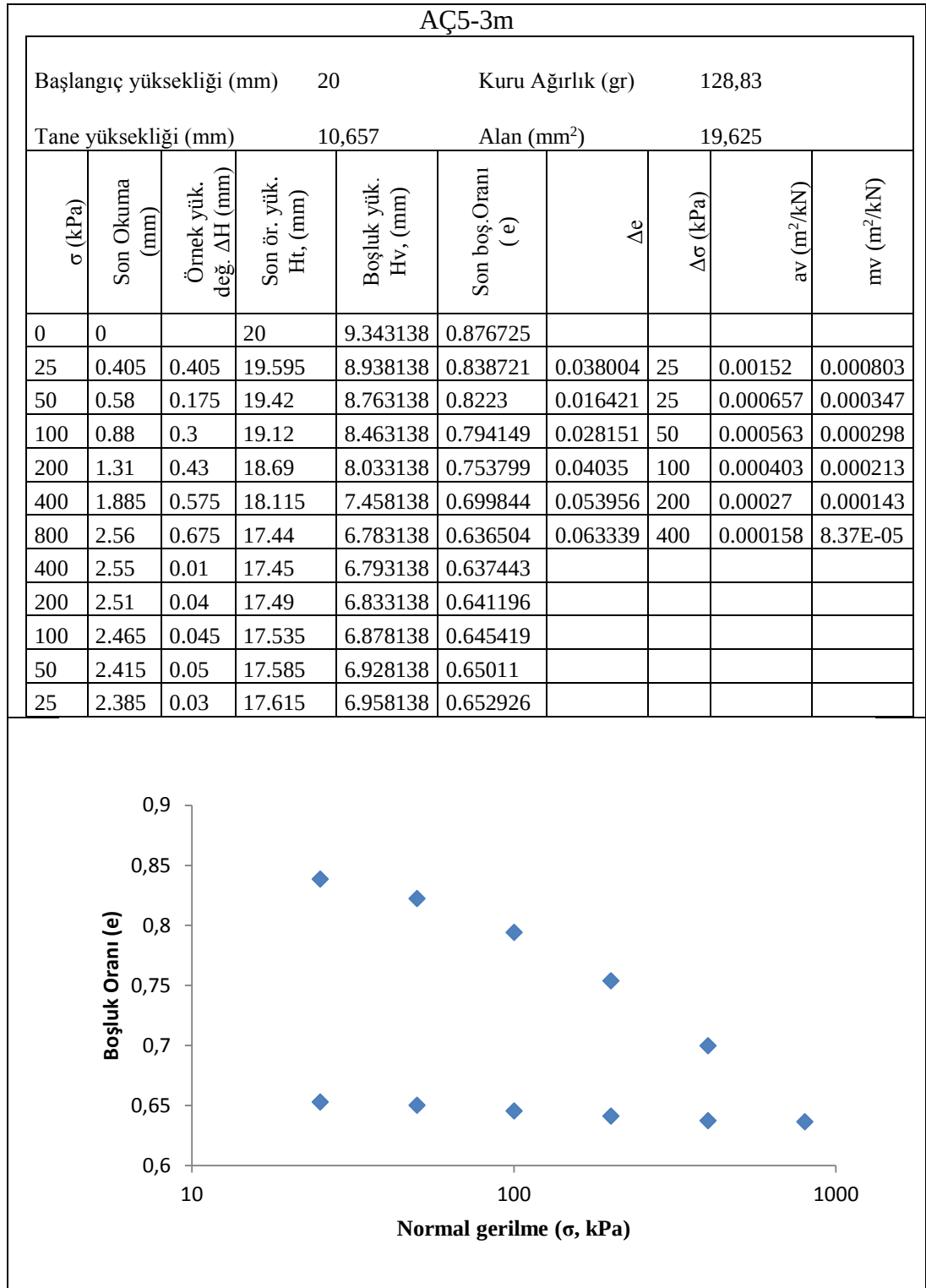
Şekil 4.32 AÇ5-3m e- \sigma Grafiği
