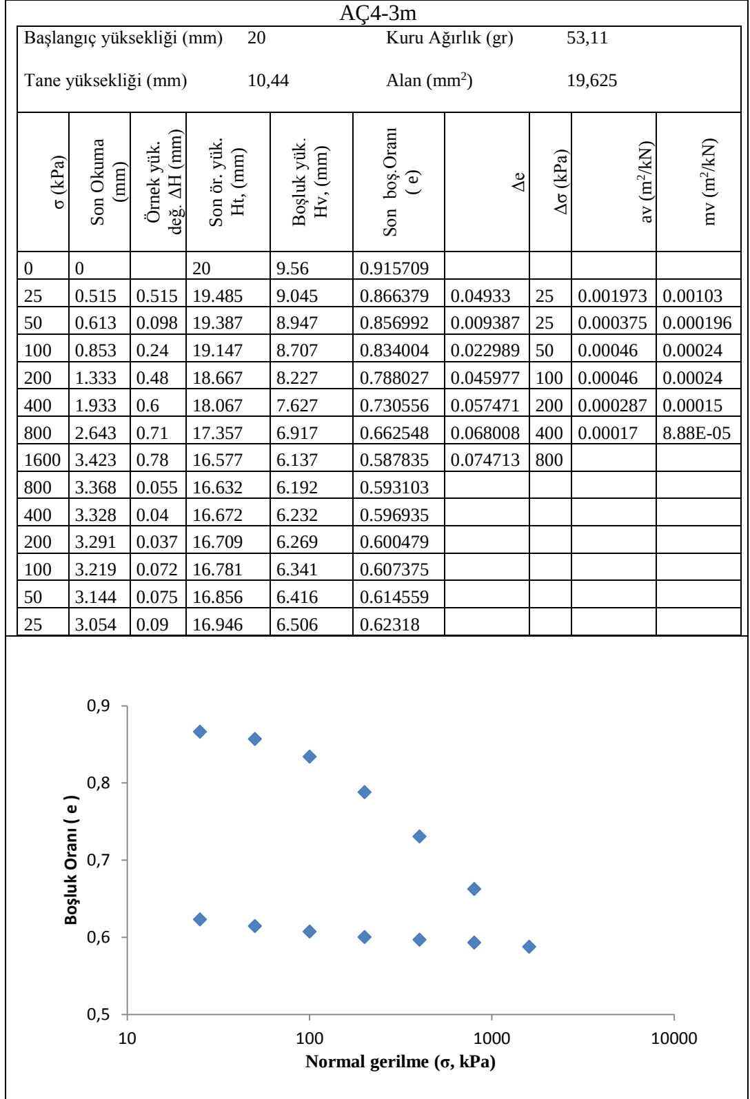
Şekil 4.31 Konsolidasyon deneyi AÇ4-3m e-σ Grafiği
