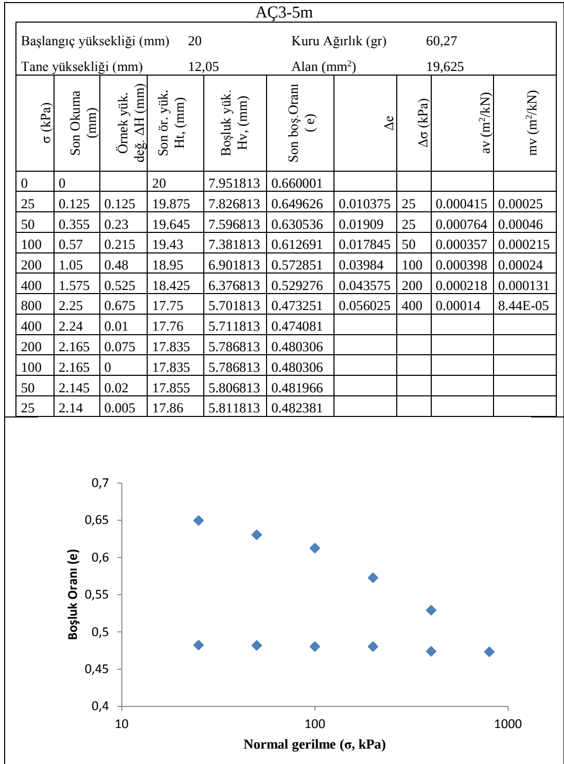
Şekil 4.30 Konsolidasyon deneyi AÇ3-5m e- \sigma Grafiği
