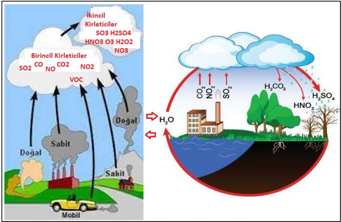
Şekil 2: Doğal ve Antropojenik Kaynaklardan Atılan Bazı Hava Kirlenitileri (URL-2)
