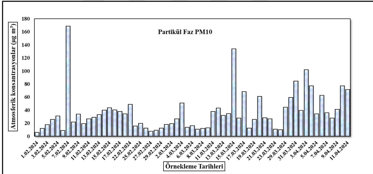
Şekil 18: PM 10 Konsantrasyonları (Kış Mevsimi Örneklem Tarihleri)
