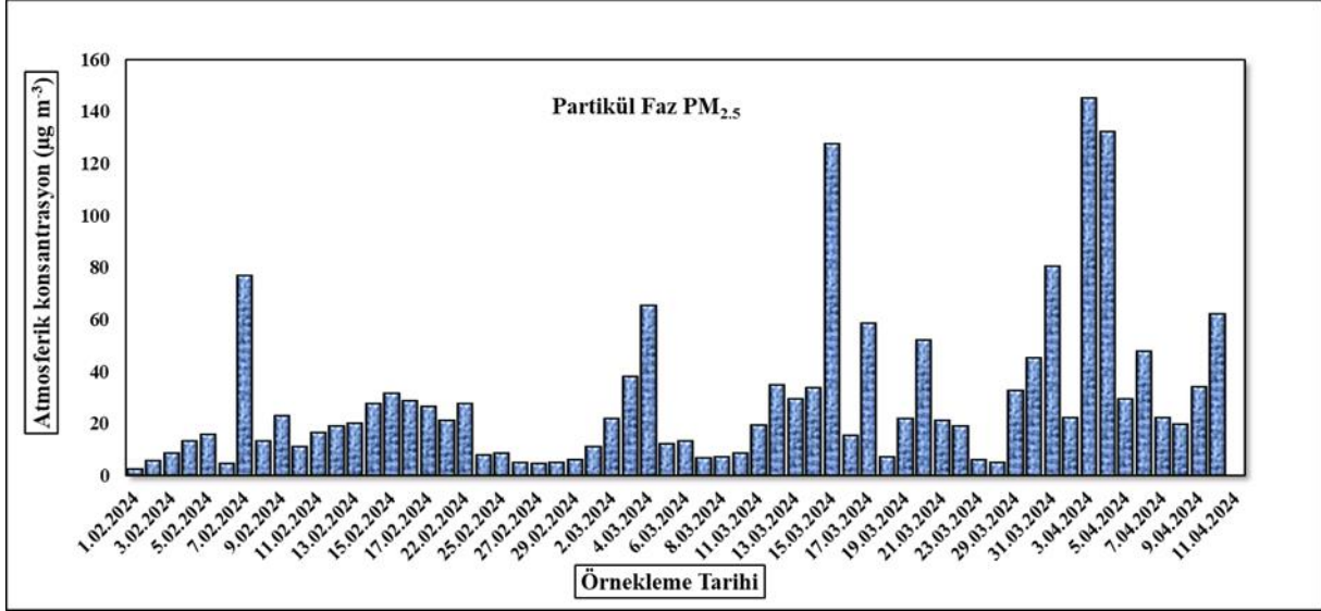
Şekil 17: PM 2,5 Konsantrasyonları (Kış Mevsimi Örneklem Tarihleri)
