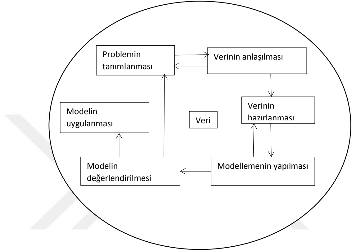
Şekil 2.2. CRISP-DM Uygulama Sürecinin Aşamaları
