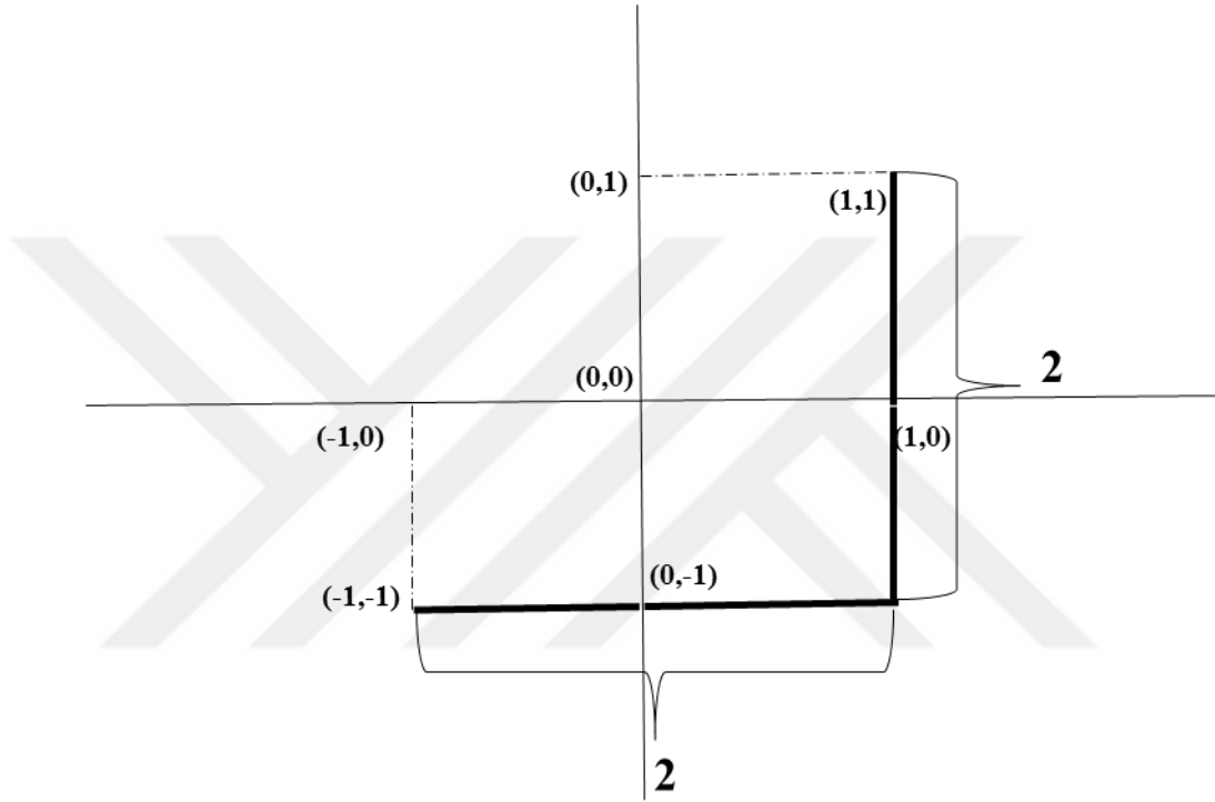
Şekil 2.4. Manhattan City-Block uzaklığına göre hesaplanmış olan (1,1) ve (-1,-1) noktaları arasındaki uzaklıkların koordinat sistemi üzerinde gösterimi
