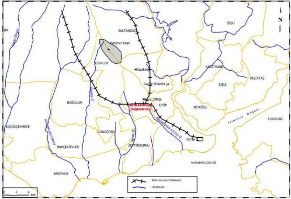
Resim 5.4: İstanbul Suyolları Gösterir Haritası - 1970(C.BAKAR, 2017, s.257)
