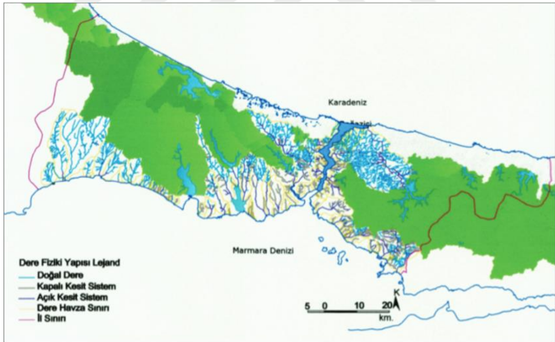
Şekil 2.3: İstanbul Sınırlarındaki Derelerin Fiziki Yapısını Gösterir Harita;
