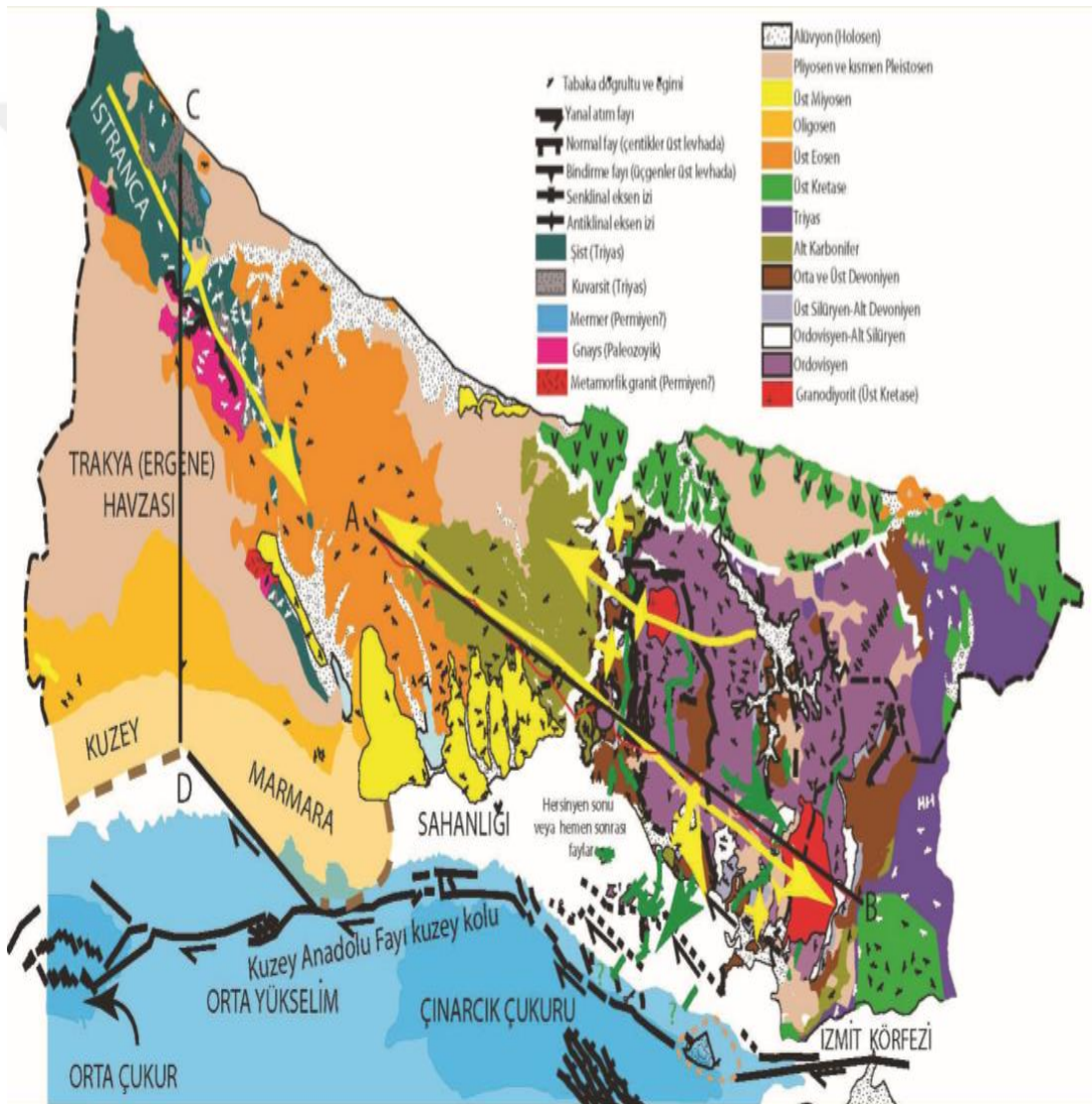
Şekil 2.1: İstanbul ve çevresinin paleotektonik evrimi
