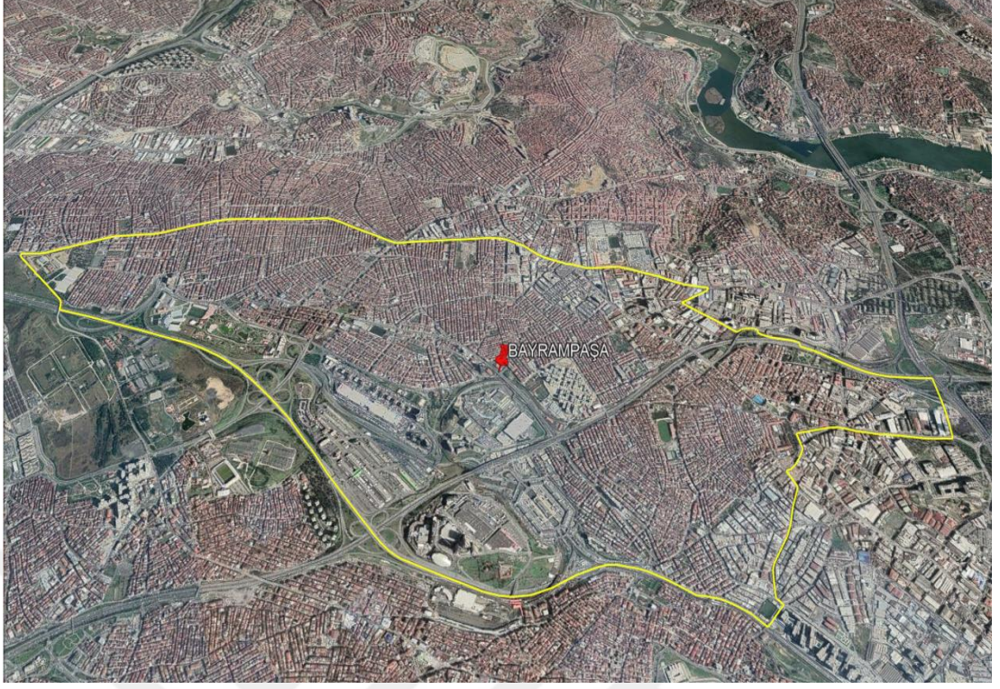
Resim 2.6: Bayrampaşa Uydu Görüntüsü
