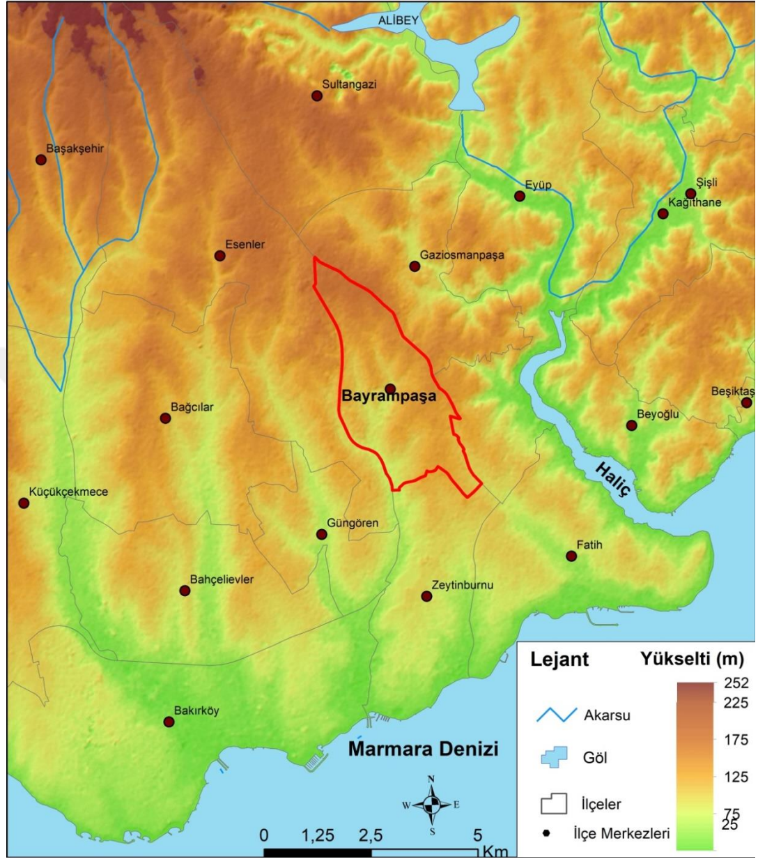
Şekil 2.2: Bayrampaşa ve çevresi jeomorfoloji haritası
