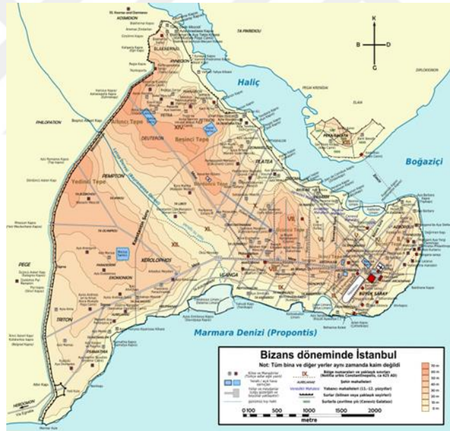
Şekil 3.2: Bayrampaşa (Lykos) Deresi Havzası ve Ağzındaki Yenikapı (Theodosius) Limanı Kıyı Alanındaki (Marmara Denizi) Değişim Süreçleri; Levent Erel, Kadir Eriş, Sena Akçer, Demet
