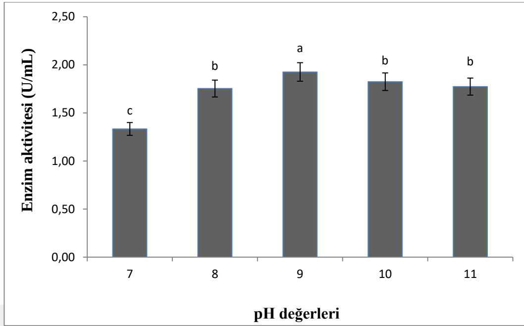
Şekil 4.3. Bacillus sp. VGA7 izolatının poligalakturonaz üretimine pH'ın etkisi.
