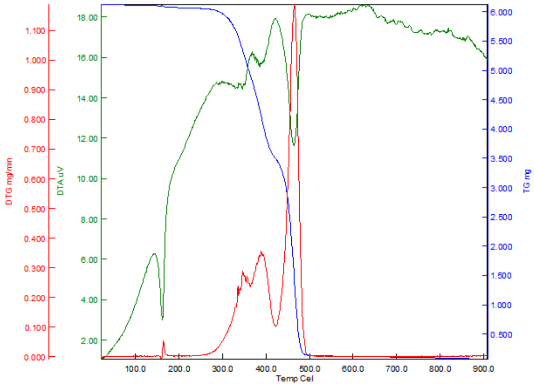
EK 3 - Şekil 8.6. % 50 PP + % 50 TPU + % 2 h- BN Kompozitinin TGA Grafiği (MKC-6)
