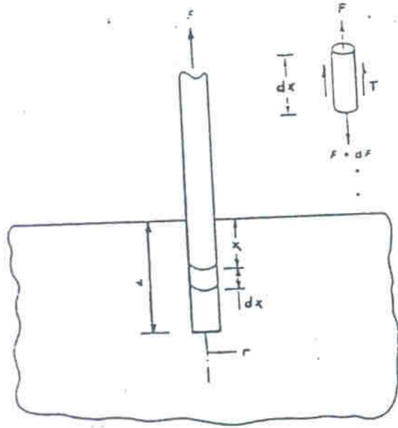
Şekil 3.2. Arabirim bağ mukavemetinin ölçülmesi
