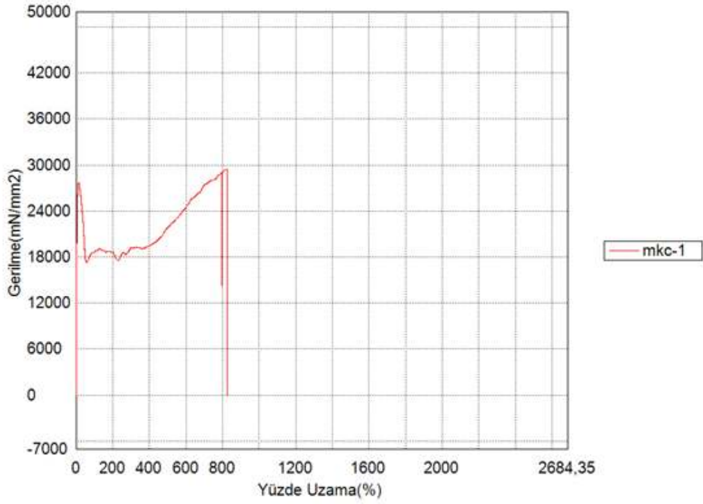
EK 5 - Şekil 8.1. % 100 PP Kompozitinin Çekme Grafiği (MKC-1)
