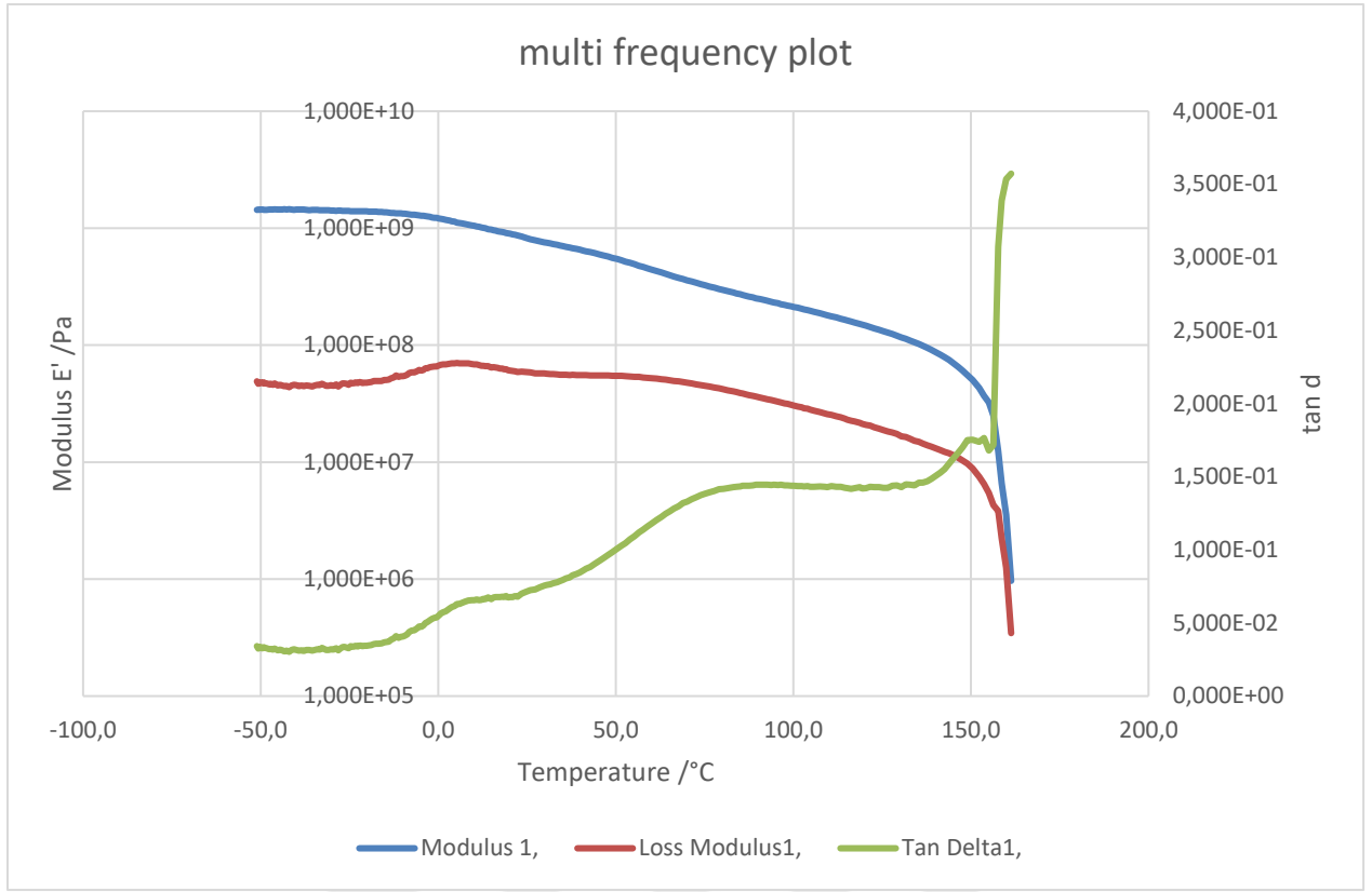
EK 4 - Şekil 8.4. % 100 PP + % 4 h- BN Kompozitiinin DMA Analizi (MKC-3)
