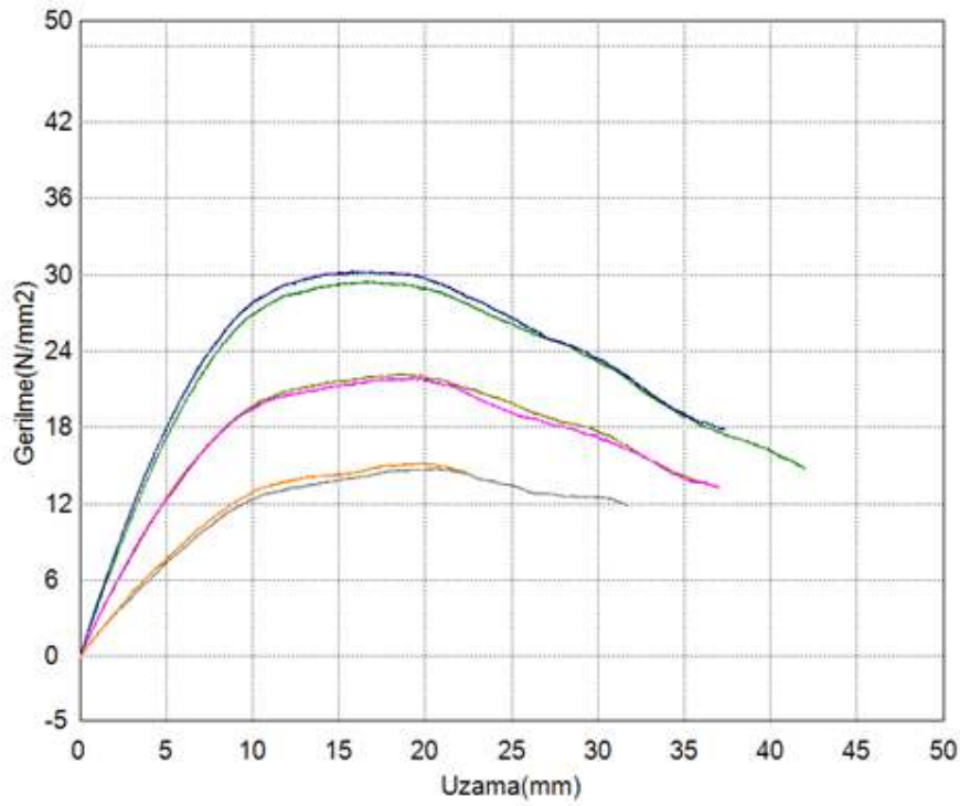
EK 6 - Şekil 8.18. Şekil 21,22,23 Birleşim Üç Nokta Eğme Grafiği
