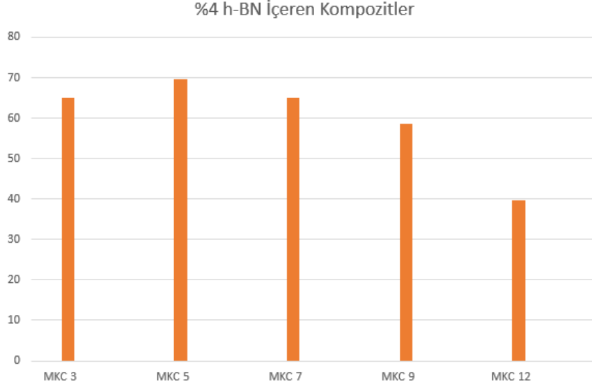
Şekil 8.21. %4 h-BN İeren Numunelerin Sertlik lm Grafiđi
