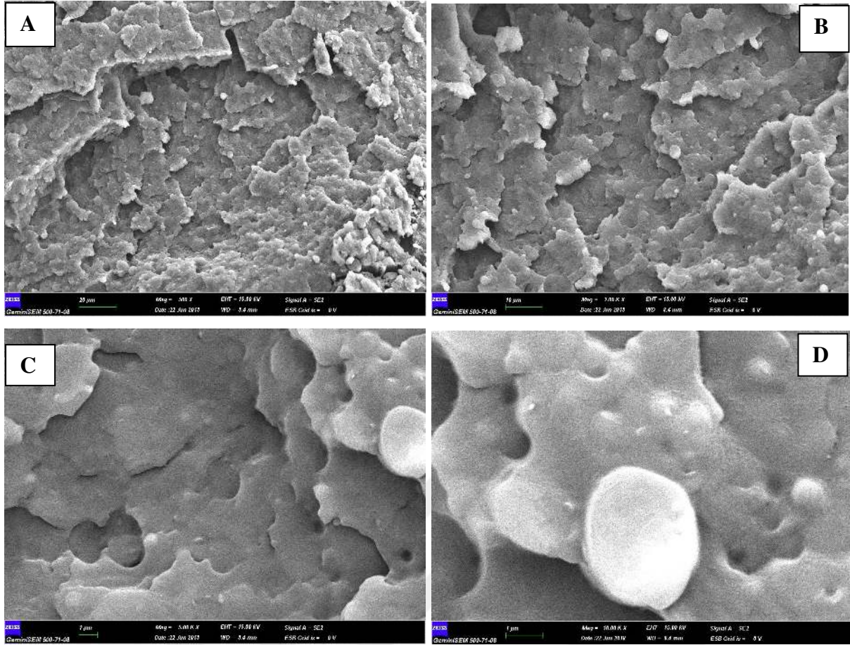
EK 7 - Şekil 8.8. % 50 PP + % 50 TPU + % 4 h- BN (MKC 7) Kompozitinin Kesitinin SEM Görüntüleri A) Büyütme 500 X B) Büyütme 1.00 KX C) Büyütme 5.00 KX D) Büyütme 10.00 KX
