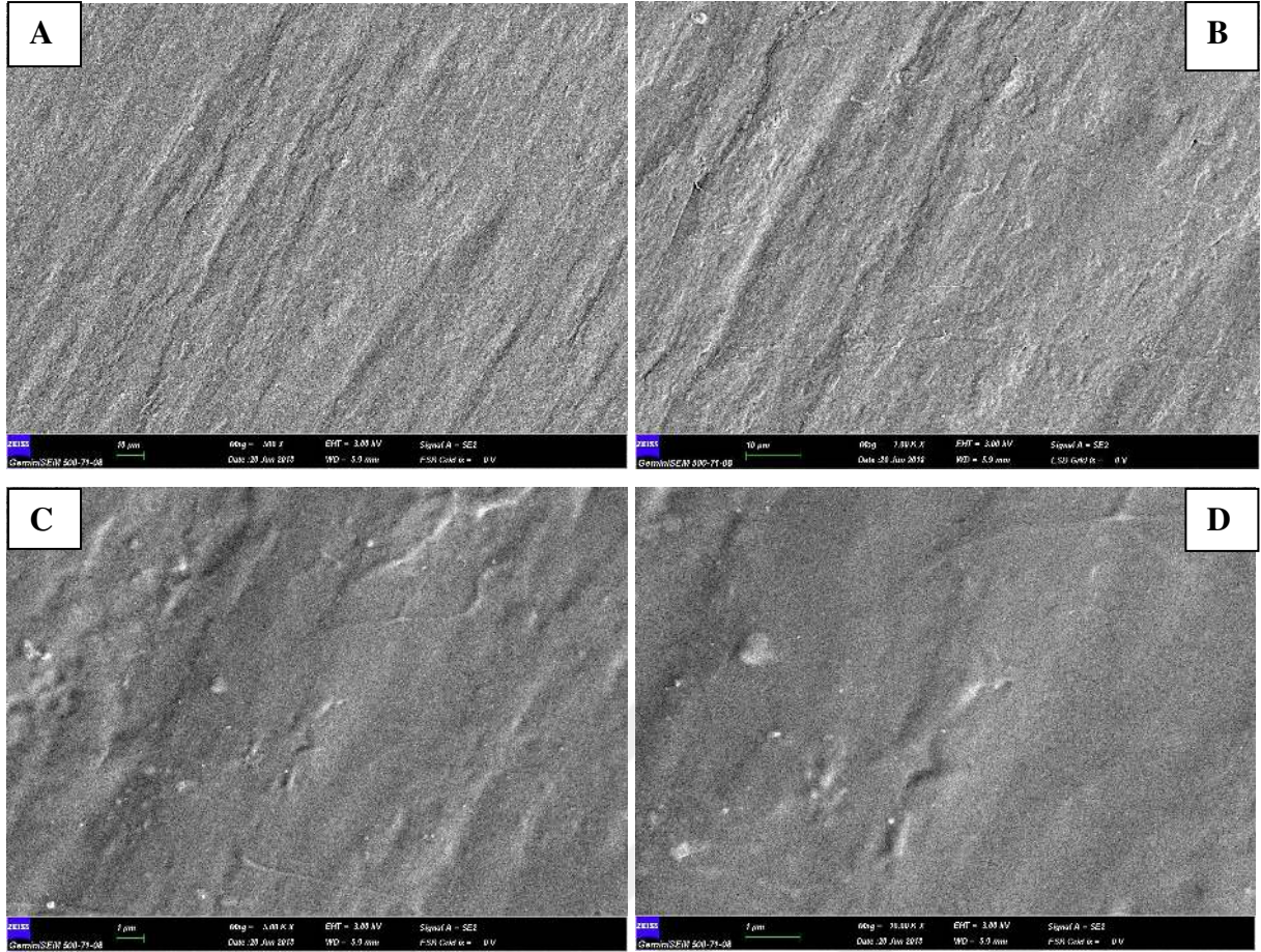
EK 7 - Şekil 8.5. % 75 PP + % 25 TPU + % 4 h- BN (MKC 5) Kompozitinin Yüzey SEM Görüntüleri A) Büyütme 500 X B) Büyütme 1.00 KX C) Büyütme 5.00 KX D) Büyütme 10.00 KX
