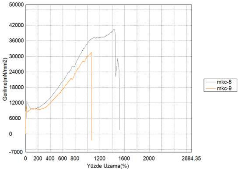
EK 5 - Şekil 8.18. MKC-8 / MKC-9 Kompozitlerinin Çekme Grafiği
