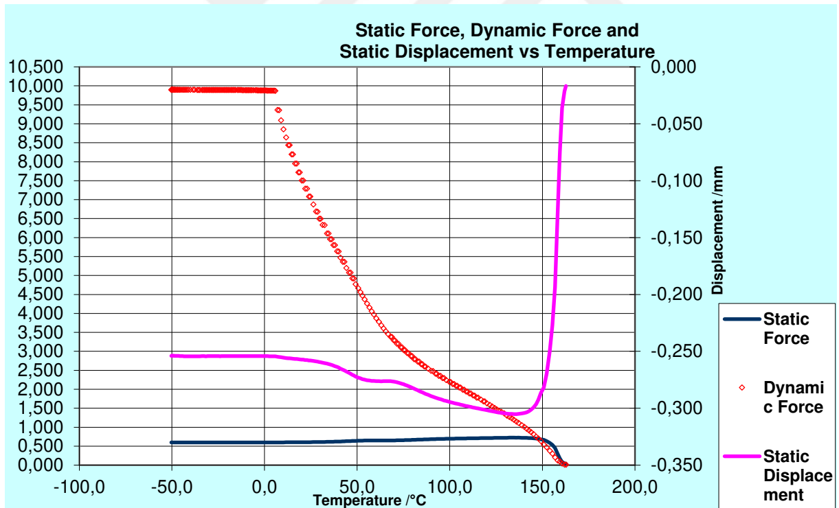
EK 4 - Şekil 8.1. % 100 PP Kompozitinin DMA Analizi (MKC-1)
