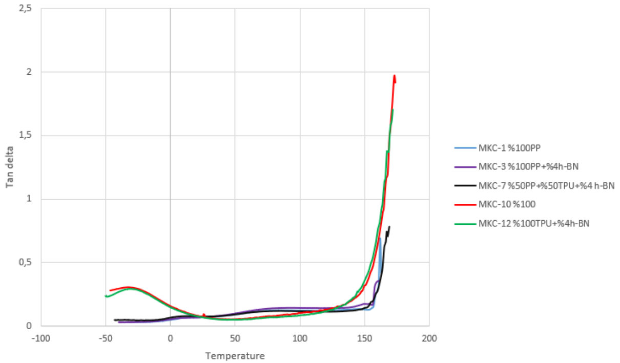
Şekil 8.12. Kompozitlerin Tan \delta – Sıcaklık DMA Grafiği
