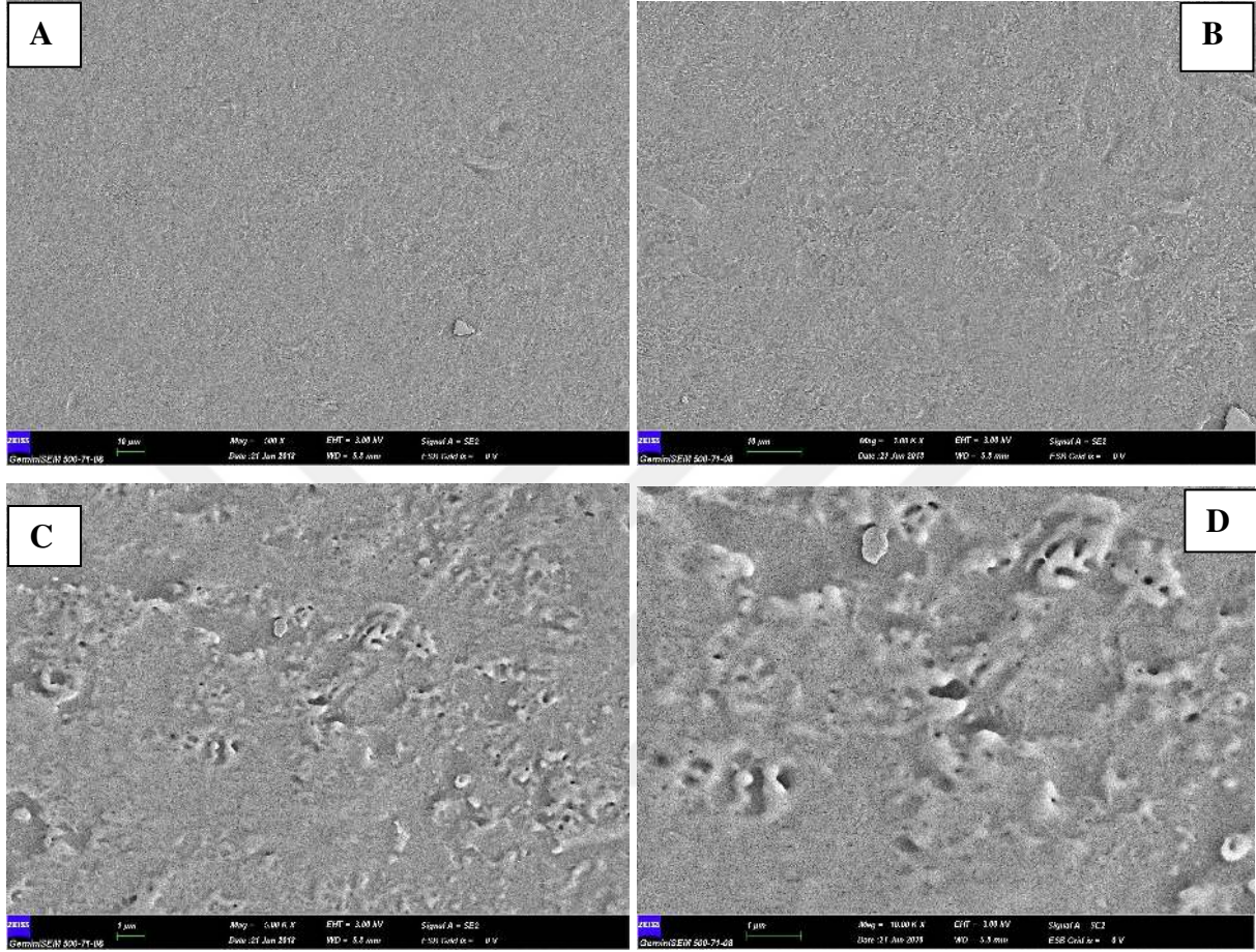
EK 7 - Şekil 8.13. % 100 TPU + % 4 h-BN (MKC 12) Kompozitinin Yüzey SEM Görüntüleri A) Büyütme 500 X B) Büyütme 1.00 KX C) Büyütme 5.00 KX D) Büyütme 10.00 KX
