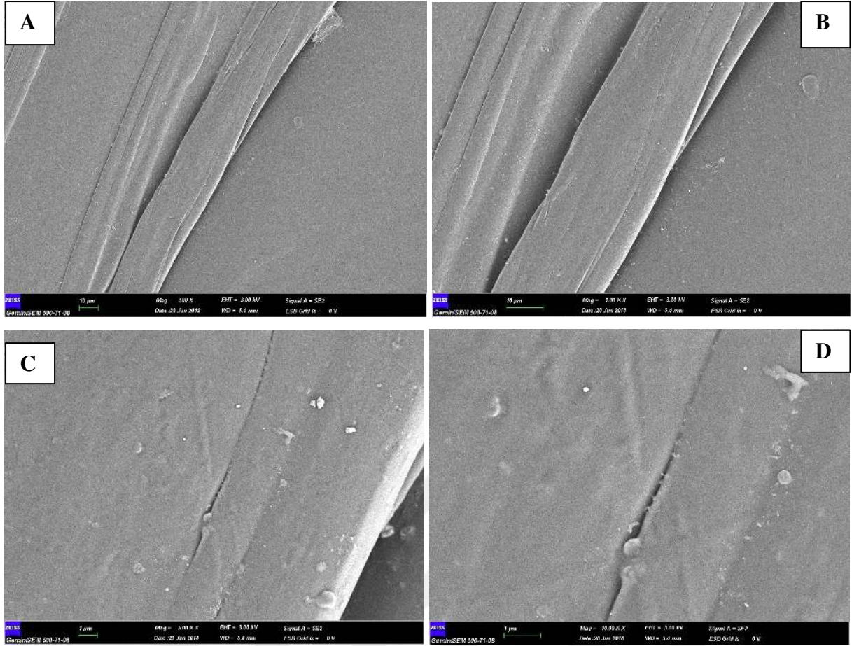
EK 7 - Şekil 8.3. % 100 PP + % 4 h- BN (MKC 3) Kompozitinin Yüzey SEM Görüntüleri A) Büyütme 500 X B) Büyütme 1.00 KX C) Büyütme 5.00 KX D) Büyütme 10.00 KX
