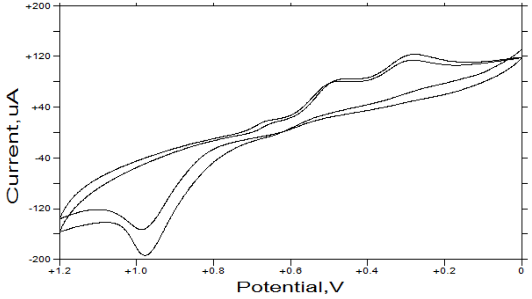
Şekil 4.53. 0,5 M \text{H}_2\text{SO}_4 içerisinde 2 mM \text{HAuCl}_4 çözeltisinin PASA/GCE yüzeyinde çevrimli voltamogramı
