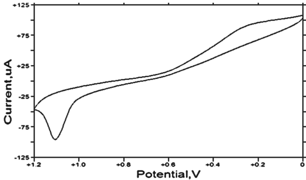
Şekil 4.7. PA/GCE yüzeyinde 0,5 M \text{H}_2\text{SO}_4 içerisinde 2 mM \text{HAuCl}_4 çözeltisinin 2 çevrimlik voltamogramı
