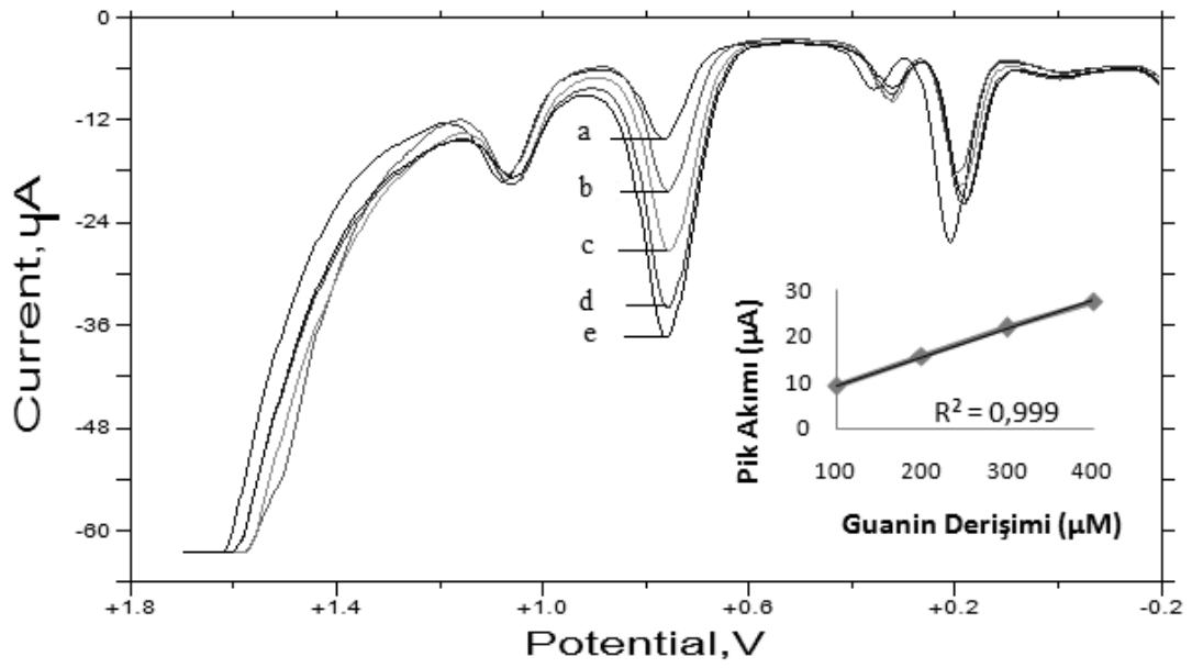
Şekil 4.45. Optimum şartlarda hazırlanan elektrodun PBS pH 5’de 100 μM’lık guanine, adenin, ürik asit ve dopamin içeren karışımda a) 100, b) 200, c) 300, d) 400, e) 500μM guanine yanıtları
