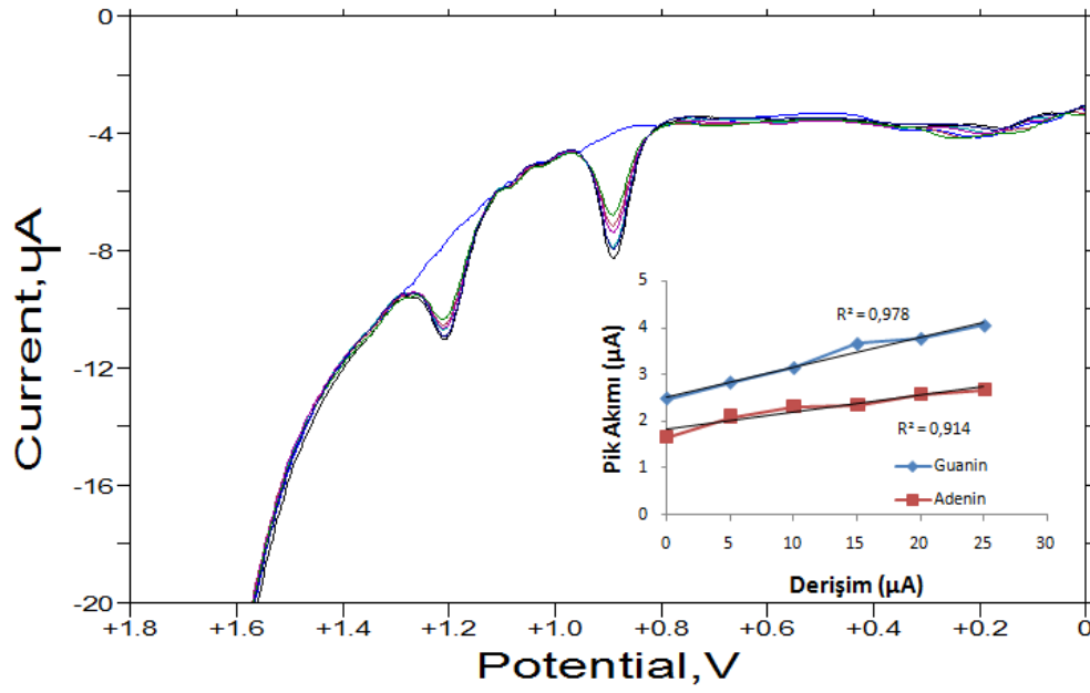
Şekil 4.71. Optimum şartlarda hazırlanan elektrodun PBS pH 4'te a) zemin, b) 50μL ssDNA, c) 5 μM, d) 10 μM, e) 15 μM, f) 20 μM g) 25 μM Guanin ve Adenin DPV yanıtları
