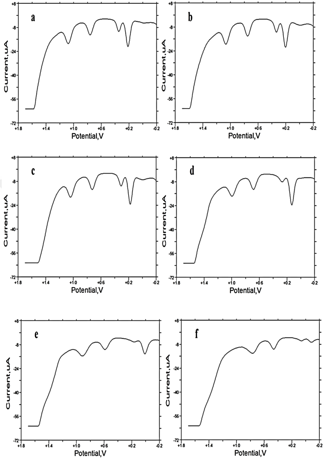
Şekil 4.43. Optimize şartlarda hazırlanan nanokompozit elektrodun a) pH 4, b) pH 5, c) pH 6, d) pH 7, e) pH 8, f) pH 9’da 100 \mu\text{M} ’lık guanin, adenin, ürik asit ve dopamin içeren karışıma ait DPV yanıtları
