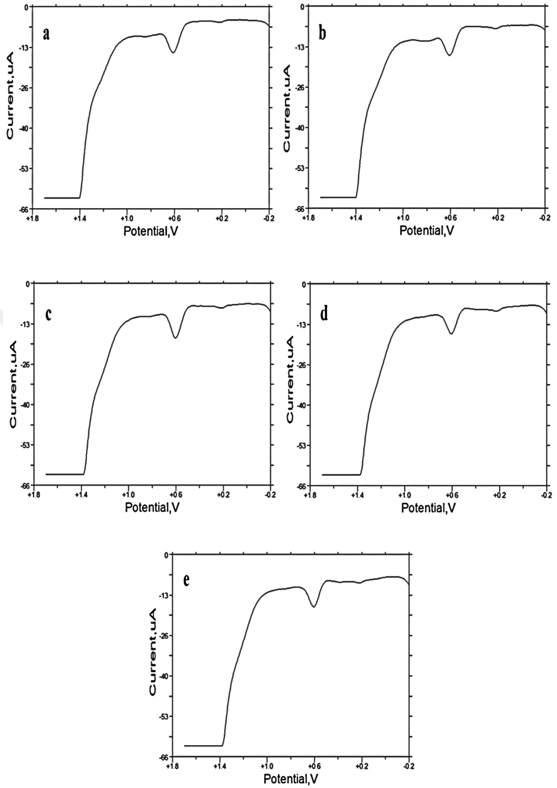
Şekil 4.16. a) 0,025 M, b) 0,05 M, c) 0,1 M, d) 0,2 M, e) 0,4 M KCl içerisinde 25 mM anilin çözeltisinden hazırlanan nano-Au/PA/GC elektrodun 100 μM guanine yanıtları
