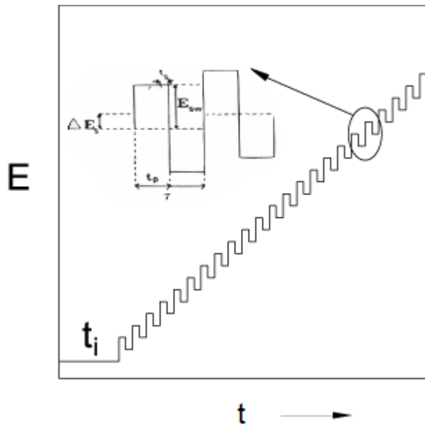
Şekil 2.2. Kare Dalga Voltametrisi için potansiyel- zaman dalga şekli ve akım ölçümü
