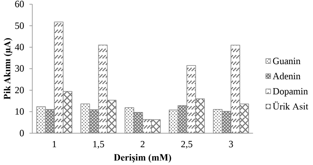
Şekil 4.40. \text{HAuCl}_4 derişiminin guanin, adenin, dopamin ve ürik asit yanıtları üzerine etkisi
