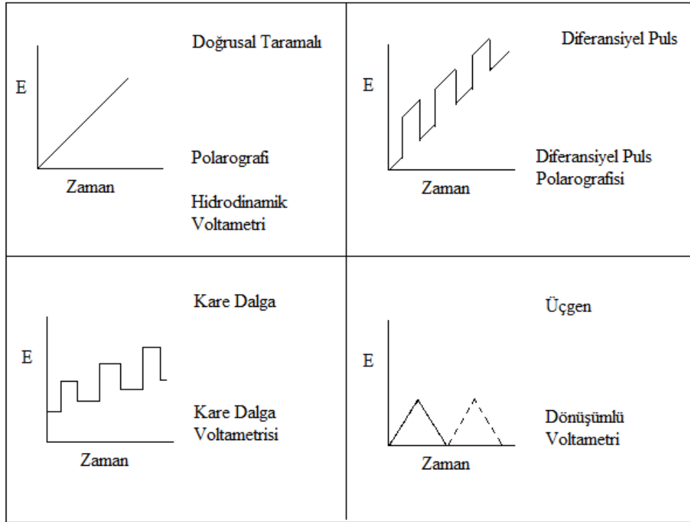
Şekil 2.1. Voltametrizde kullanılan uyarma sinyalleri
