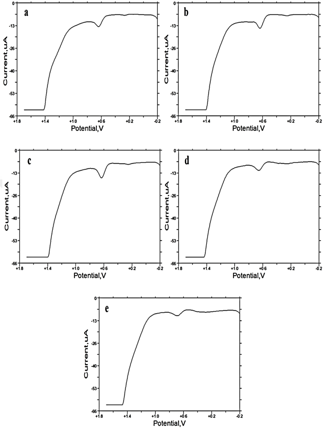
Şekil 4.20. PA üzerine 2 mM H Au Cl 4 çözeltisinden a) 2, b) 4, c) 6, d) 8, e) 10 çevrim nano-Au kaplanan elektrodun 100 \mu M guanin yanıtları
