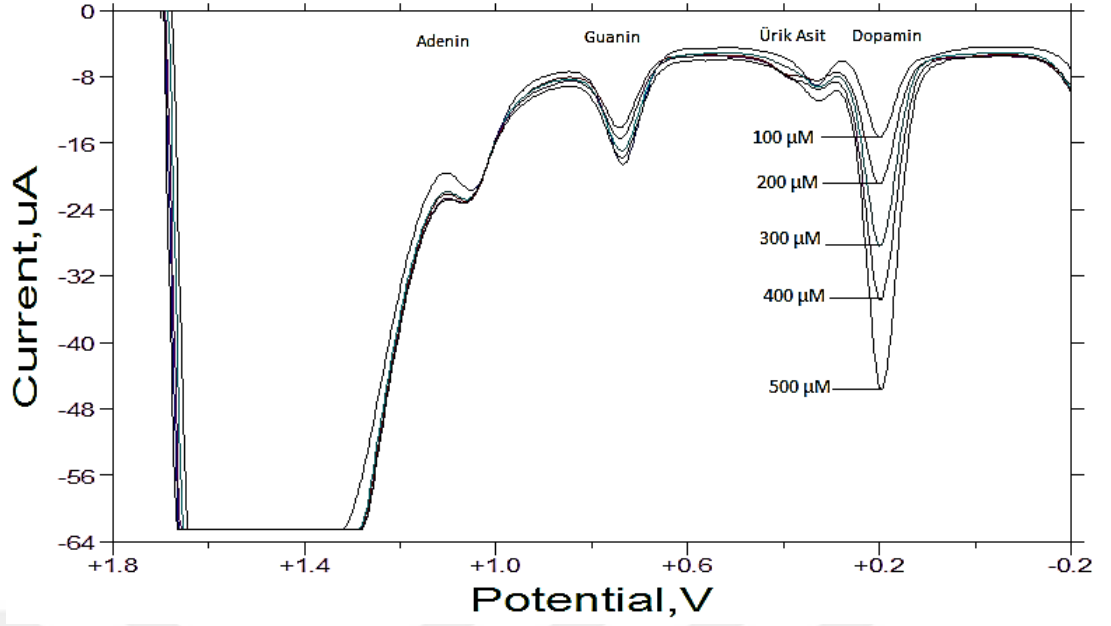
Şekil 4.27. Optimum şartlarda hazırlanan elektrodun PBS pH 5’de 100 \mu\text{M} ’lık guanin, adenin, ürik asit ve dopamin içeren karışımda artan dopamin derişimi yanıtları
