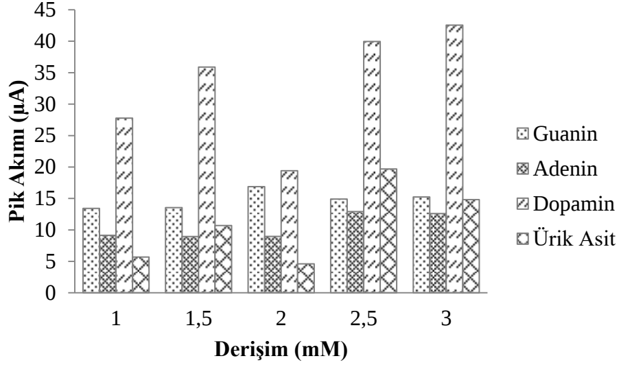
Şekil 4.64. Guanin, adenin, dopamin ve ürik asit yanıtları üzerine \text{HAuCl}_4 derişiminin etkisi
