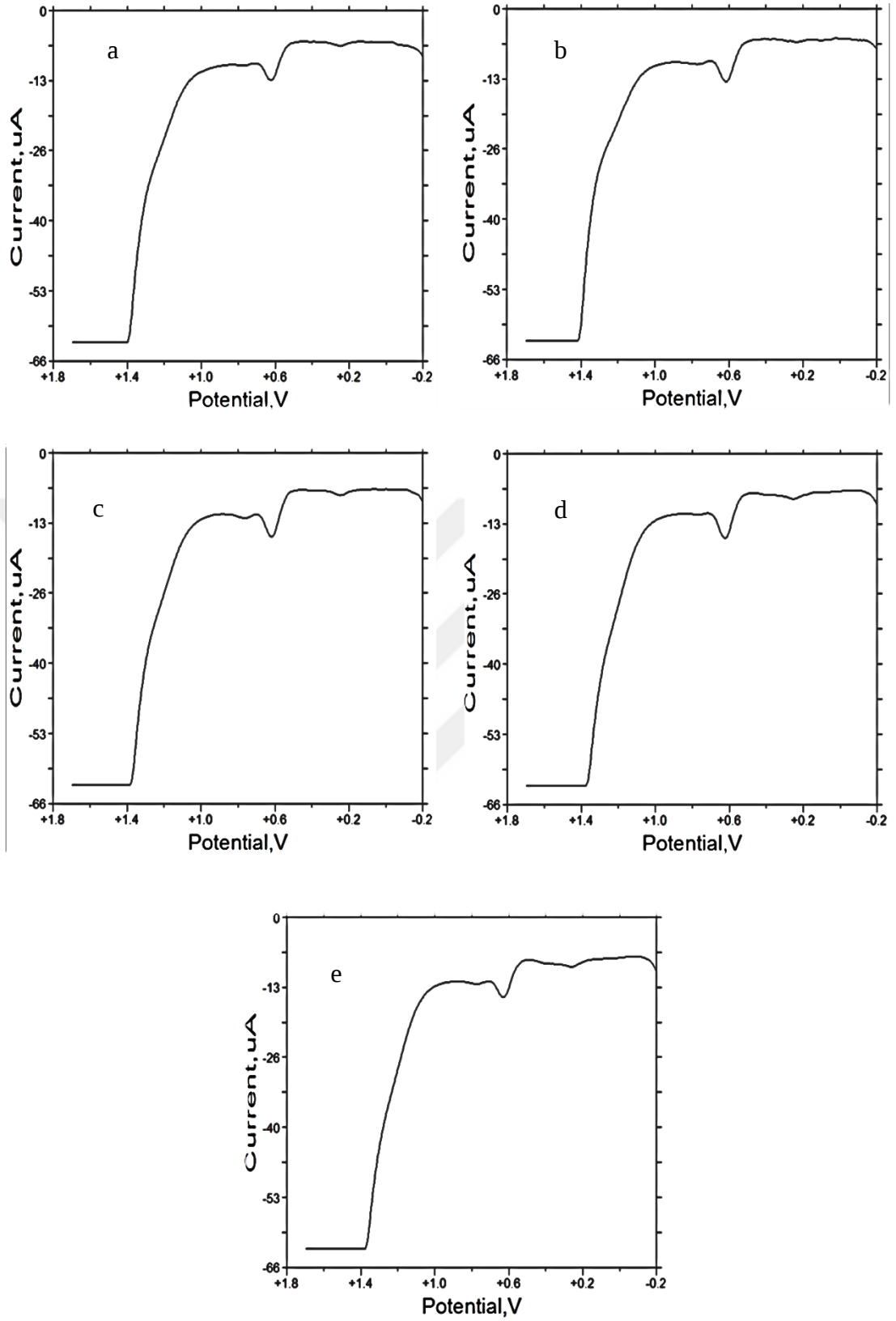
Şekil 4.12.0,1 M KCl içerisinde a) 10 mM, b) 15 mM, c) 20 mM, d) 25 mM, e) 30 mM anilin çözeltisinden hazırlanan nano-Au/PA/GC elektrodun 100 μM guanine yanıtları
