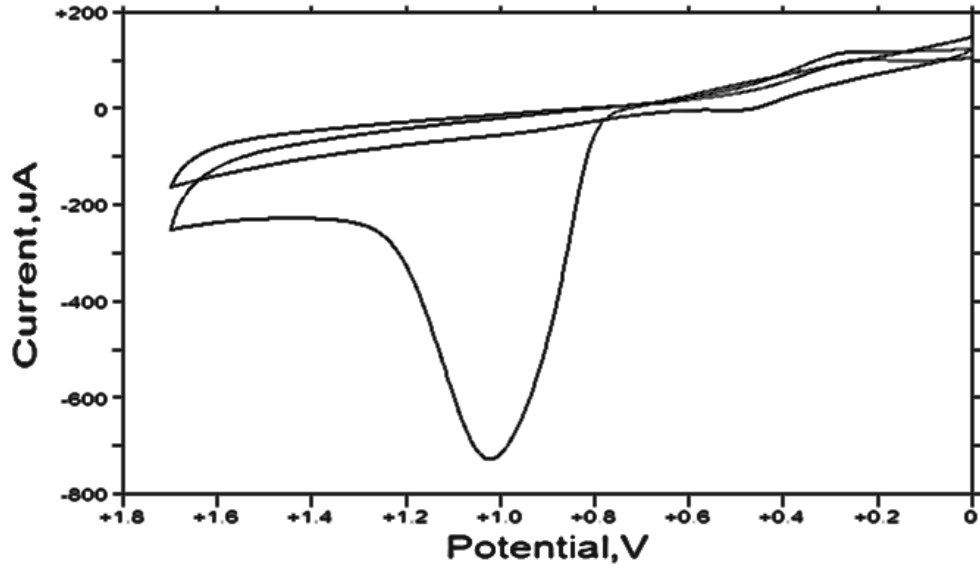
Şekil 4.6.0,5 M \text{H}_2\text{SO}_4 içerisinde (destek elektroliti 0,1 M KCl) 20 mM anilin çözeltisinin GCE yüzeyinde 4 çevrimlik voltamogramı
