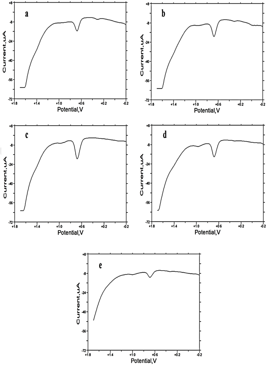
Şekil 4.41. a) 0,1, b) 0,15, c) 0,2, d) 0,25 ve e) 0,3 M KCl içerisinde 30 mM, N -Metil pirol 1,5 mM \text{HAuCl}_4 çözeltisinden 8 çevrimlik hazırlanan filmlerin 100 \mu\text{M} guanin yanıtları
