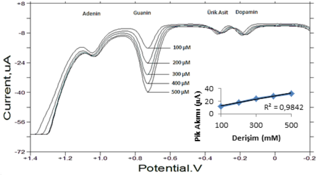
Şekil 4.25. Optimum şartlarda hazırlanan elektrodun PBS pH 5’de 100 \mu M’lık guanin, adenin, ürik asit ve dopamin içeren karışımda artan guanin derişim yanıtları
