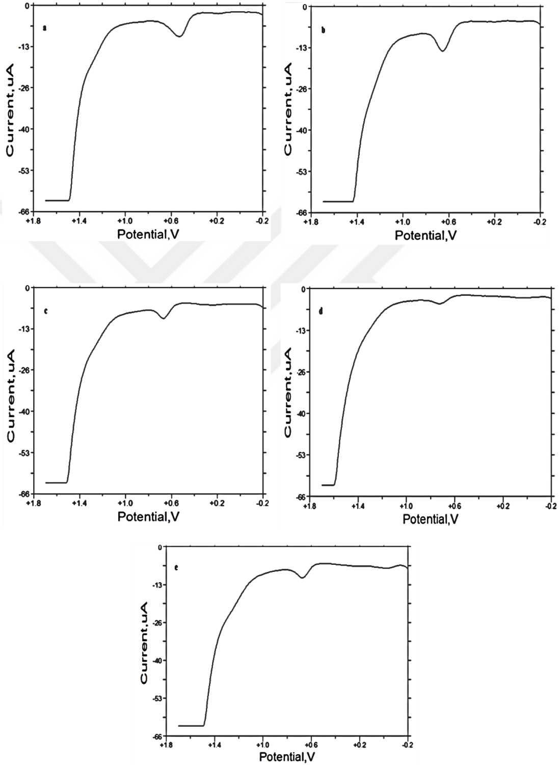
Şekil 4.8. 20 mM anilin çözeltisinden (destek elektroliti 0,1 M KCl) a) 2, b) 4, c) 6, d) 8, e) 10 çevrim olarak hazırlanıp üzerine 2 mM H Au Cl 4 çözeltisinden 2 çevrim nano-Au kaplanan elektrodun 100 μM guanin yanıtları
