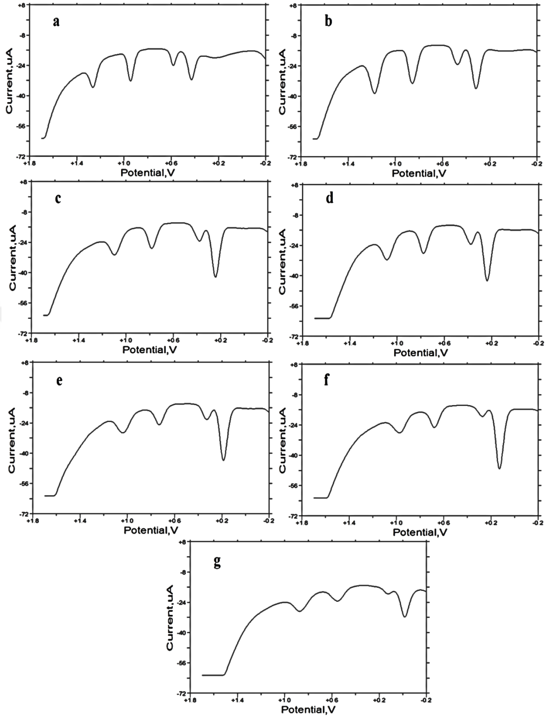
Şekil 4.65. Optimize elektrodun a) pH 3, b) pH 4, c) pH 5, d) pH 6, e) pH 7, f) pH 8, g) pH 9’da 100 \mu\text{M} ’lık guanin, adenin, ürik asit ve dopamin içeren karışıma ait DPV yanıtları
