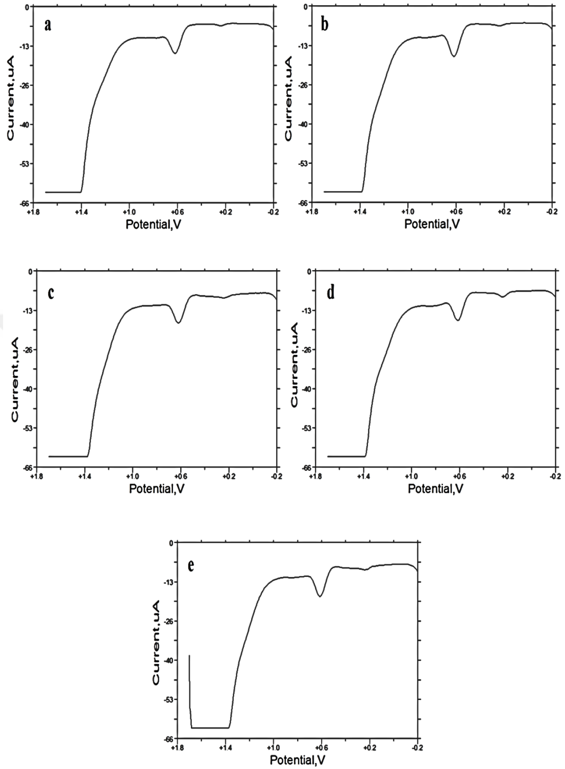
Şekil 4.22. PA film üzerine a) 1, b) 1,5, c) 2, d) 2,5, e) 3 mM H Au Cl 4 çözeltisinden 6 çevrim nano-Au kaplanan elektrodun 100 μM guanin yanıtları
