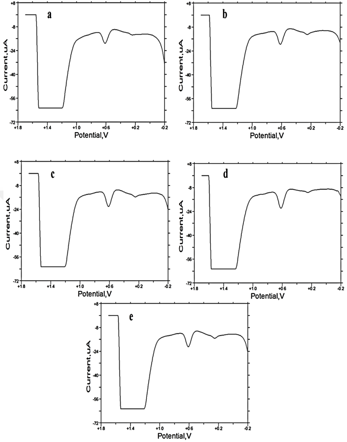
Şekil 4.35. 0,2 M KCl içerisinde 30 mM N -Metil pirol ve 2 mM HAuCl 4 çözeltisinden a) 2, b) 4, c) 6, d) 8, e) 10 çevrim olarak hazırlanan elektrodun 100 \mu M guanin yanıtları
