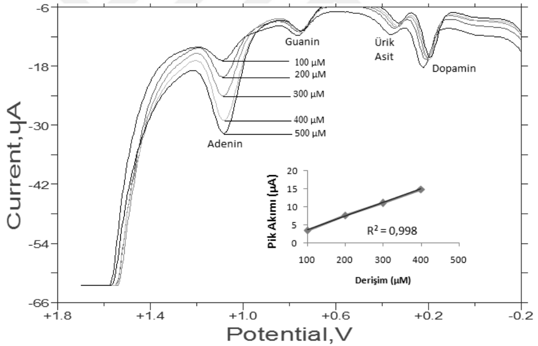
Şekil 4.46. Optimum şartlarda hazırlanan elektrodun PBS pH 5’de 100 μM’lık guanine, adenin, ürik asit ve dopamin içeren karışımda artan adenin derişim yanıtları
