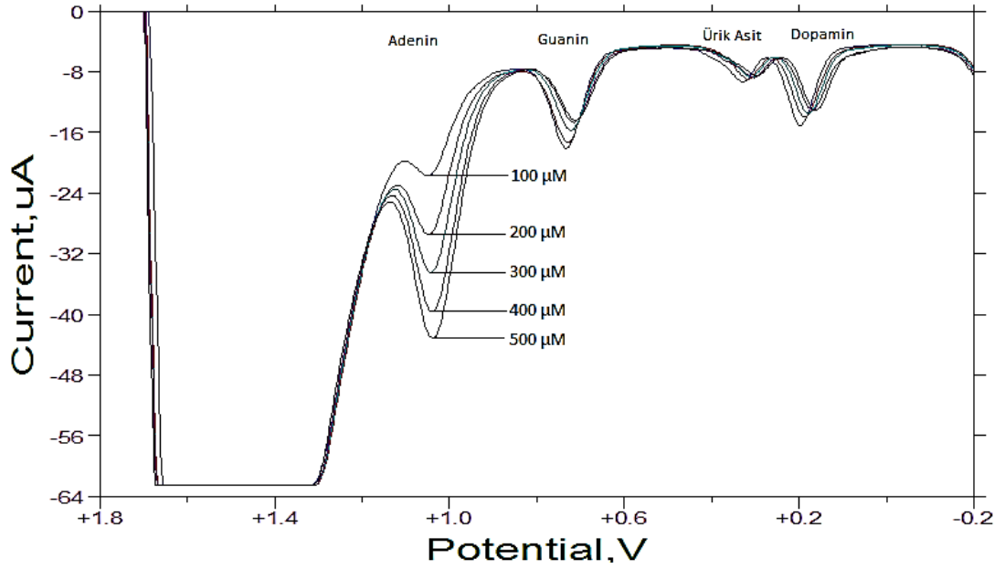
Şekil 4.26. Optimum şartlarda hazırlanan elektrodun PBS pH 5’de 100 \mu M’lık guanin, adenin, ürik asit ve dopamin içeren karışımda artan adenin derişim yanıtları
