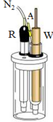
Şekil 3.2. Mikro hücre ve montajı; A: yardımcı elektrot, W: çalışma elektrodu, R: referans elektrot [32]
