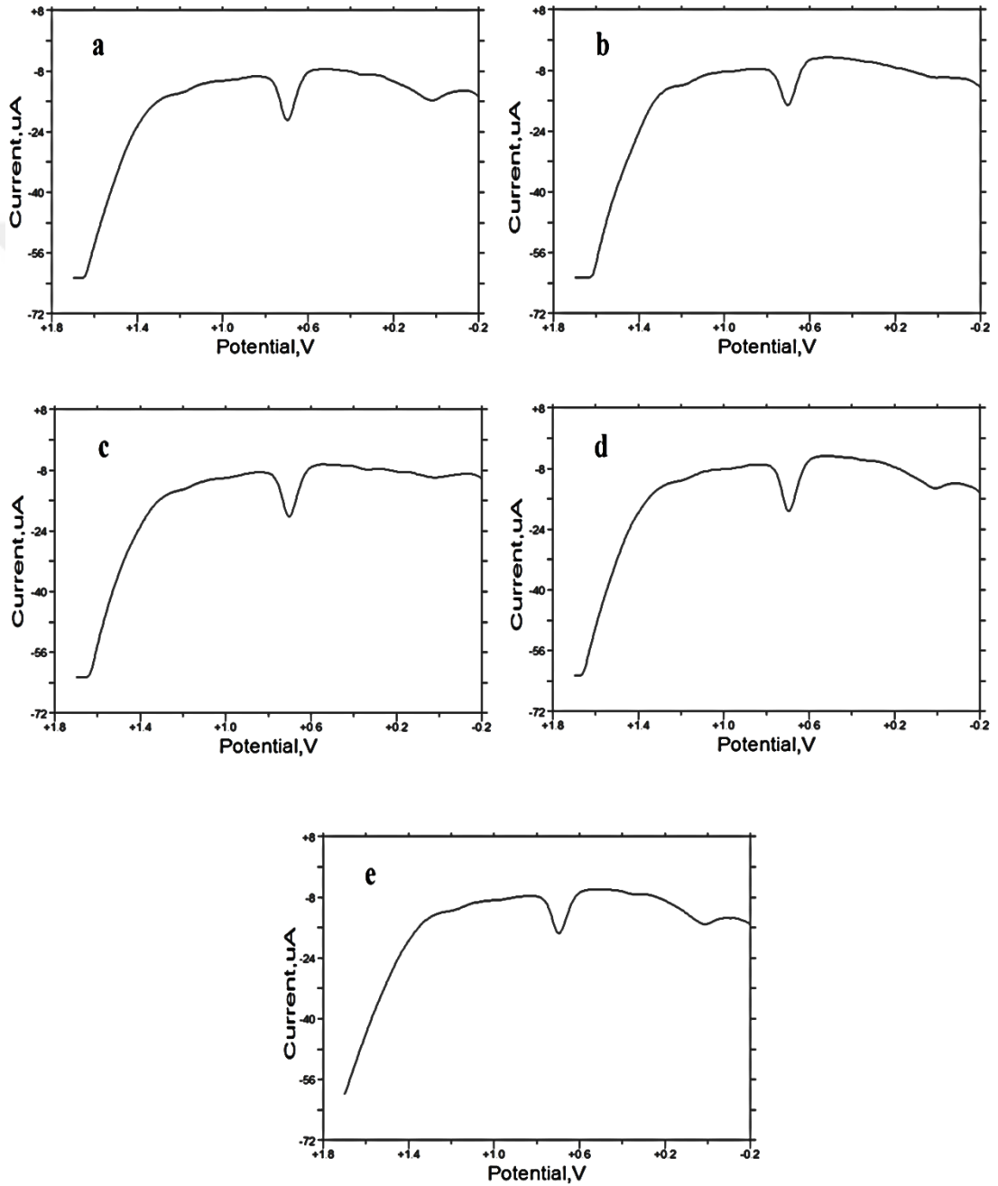
Şekil 4.55. 0,2 M KCl içerisinde 30 mM anilin-2-sülfonik asit çözeltisinden a) 2, b) 4, c) 6, d) 8 ve e) 10 çevrim olarak hazırlanıp üzerine nano-Au kaplanan elektrodun 100 \mu M guanin yanıtları
