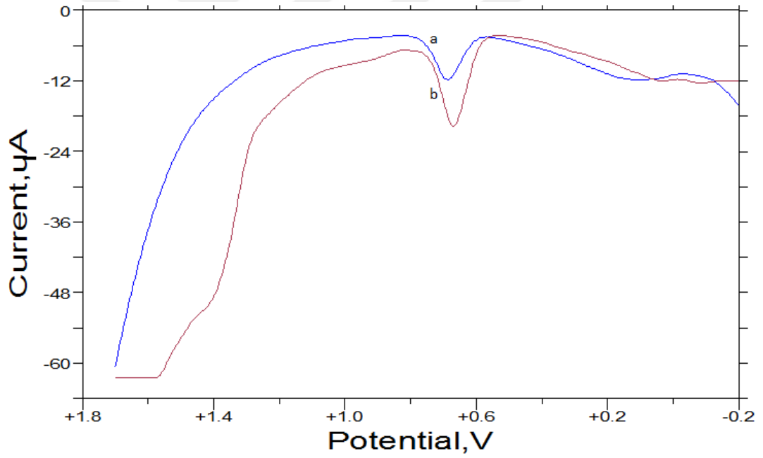
Şekil 4.53. 0,5 M \text{H}_2\text{SO}_4 içerisinde 2 mM \text{HAuCl}_4 çözeltisinin PASA/GCE yüzeyinde çevrimli voltamogramı
