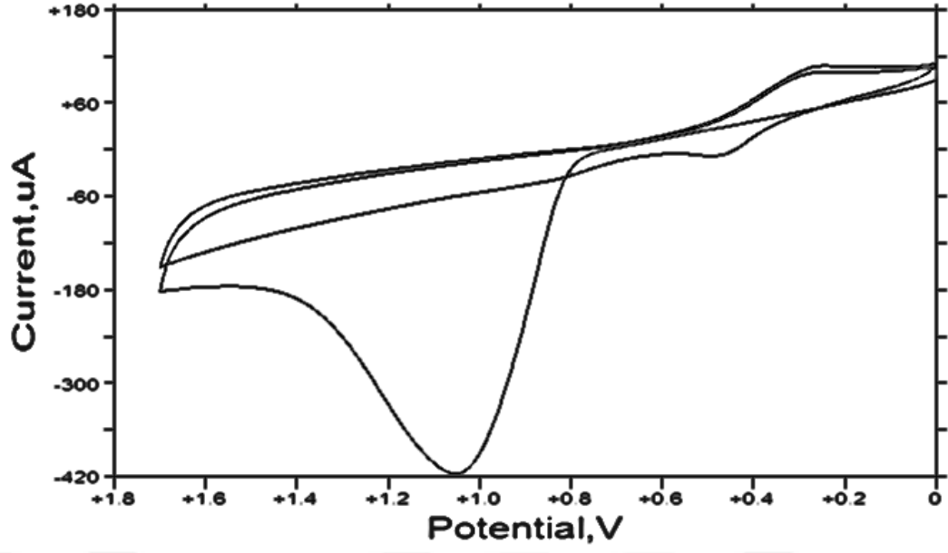
Şekil 4.18. 0,5 M \text{H}_2\text{SO}_4 içerisinde (destek elektroliti 0,1 M KCl) 20 mM anilin çözeltisinin GCE yüzeyinde 4 çevrimlik voltamogramı
