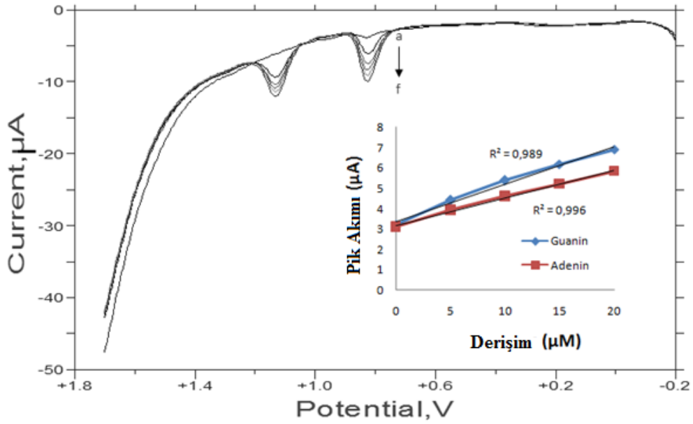
Şekil 4.30. Optimum şartlarda hazırlanan elektrodun PBS pH 5’de a) zemin, b) 50μL ssDNA, c) 5 μM Guanin ve Adenin, d) 10 μM Guanin ve Adenin, e) 15 μM Guanin ve Adenin, f) 20 μM Guanin ve Adenin DPV yanıtları
