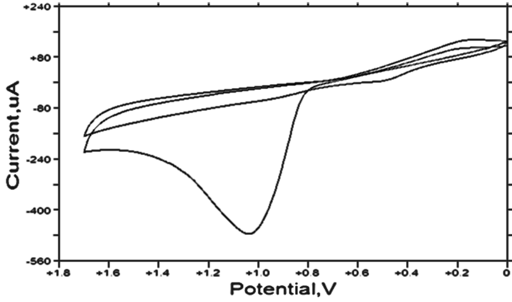
Şekil 4.10. 0,5 M \text{H}_2\text{SO}_4 içerisinde (destek elektroliti 0,1 M KCl) 20 mM anilin çözeltisinin GCE yüzeyinde 4 çevrimlik voltamogramı
