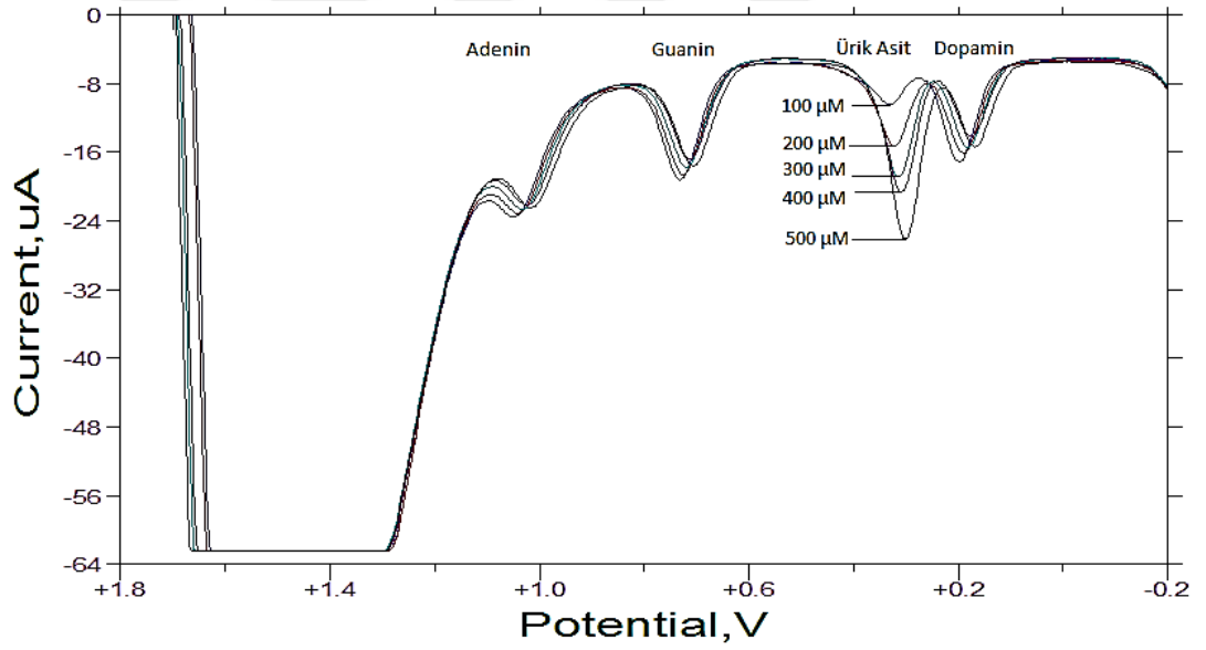
Şekil 4.28. Optimum şartlarda hazırlanan elektrodun PBS pH 5’de 100 \mu\text{M} ’lık guanin, adenin, ürik asit ve dopamin içeren karışımda artan ürik asit derişim yanıtları
