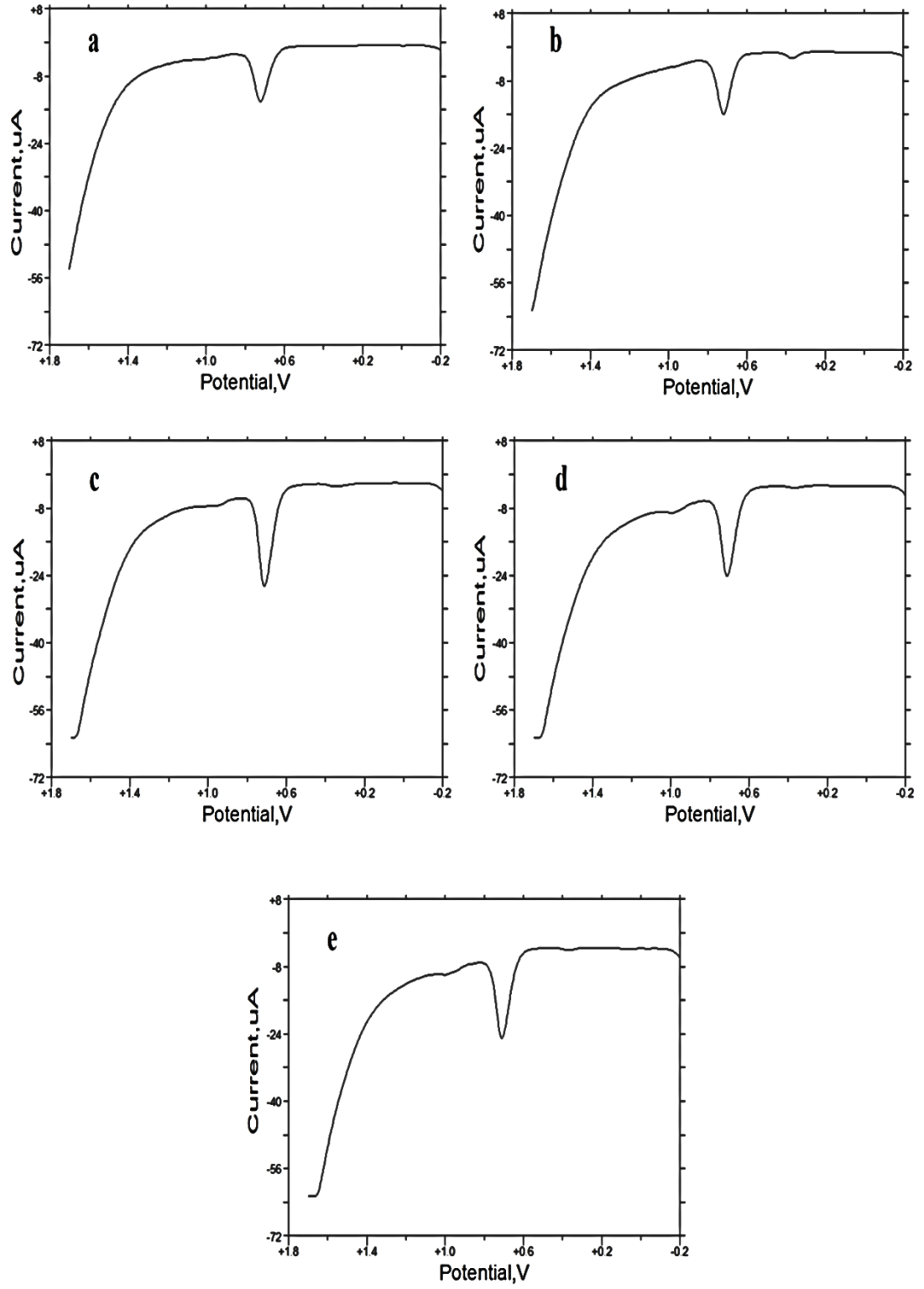
Şekil 4.61. PASA film üzerine 2 mM \text{HAuCl}_4 çözeltisinden a) 2, b) 4, c) 6, d) 8, e) 10 çevrim nano-Au kaplanan elektrodun 100 \mu\text{M} guanin yanıtları
