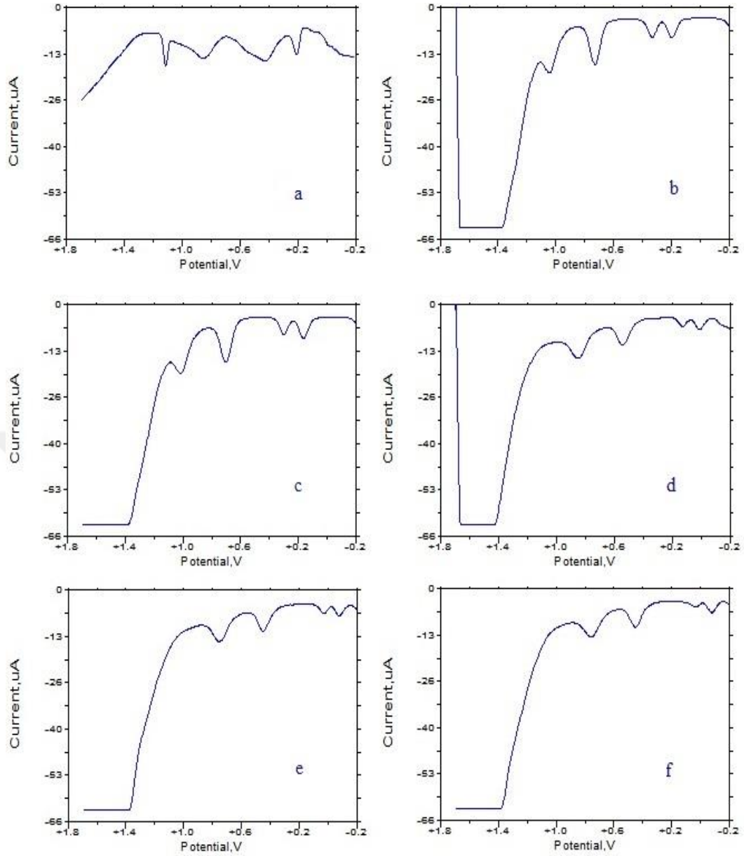
Şekil 4.24. Optimum şartlarda hazırlanan elektrodun a) pH 4, b) pH 5, c) pH 6, d) pH 7, e) pH 8, f) pH 9’da 100 \mu M’lık guanin, adenin, ürik asit ve dopamin içeren karışıma ait yanıtları
