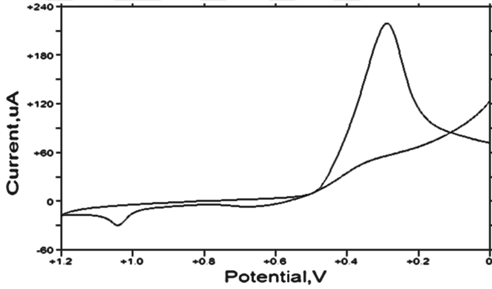
Şekil 4.11. PA/GCE yüzeyinde 0,5 M \text{H}_2\text{SO}_4 içerisinde 2 mM \text{HAuCl}_4 çözeltisinin 2 çevrimlik voltamogramı
