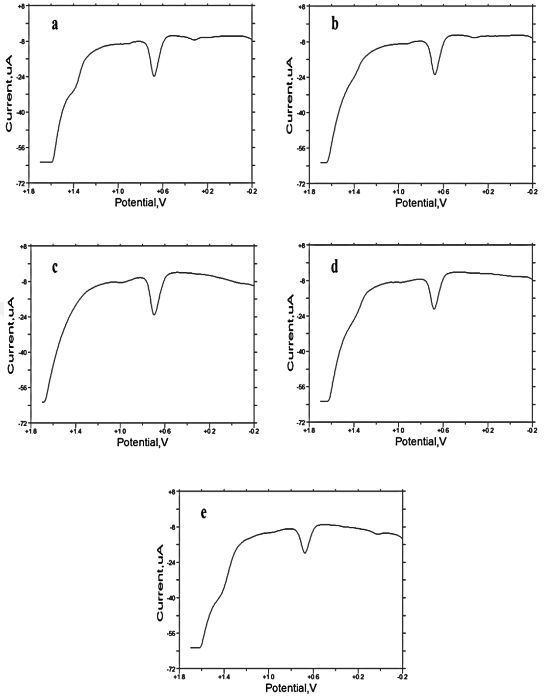
Şekil 4.37. 0,2 M KCl içerisinde a) 10, b) 20, c) 30, d) 40, e) 50 mM N -Metil pirol ve 2 mM \text{HAuCl}_4 çözeltisinden 8 çevrimlik hazırlanan filmlerin 100 \mu\text{M} guanin yanıtları
