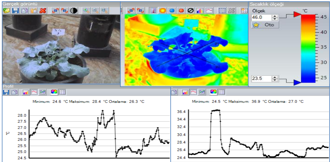
Şekil 3.9. IRTSoft yazılımı ile termal görüntülerin işlenmesi
