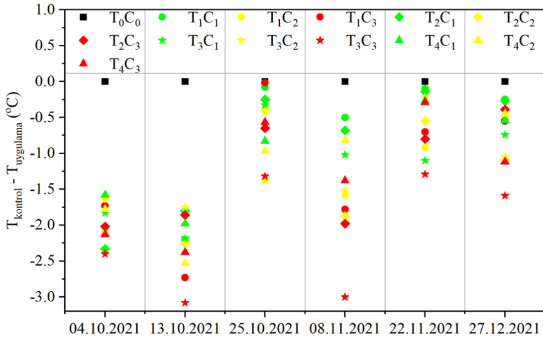
Şekil 4.2. Brokoli bitkisinde 13:00-14:00 saatleri arası tuz uygulamalarının kontrol konusuna göre sıcaklık farklılıkları
