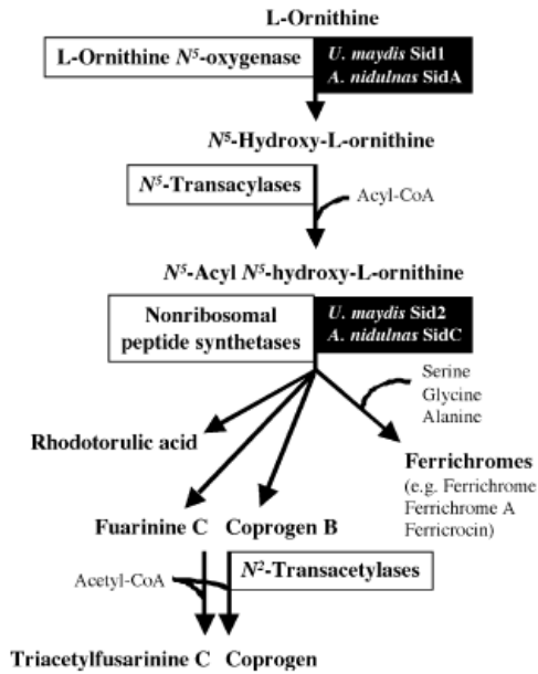
Şekil 2.1: Fungal hidroksamat tip sideroforların Plattner ve Diekman'a göre genel biyosentez yolu. (1994)
