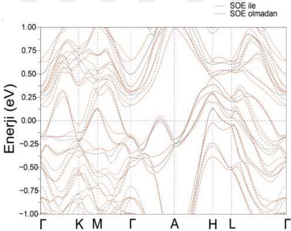
Şekil 4.3. Hekzagonal örgünün birinci Brillouin bölgesinde yüksek simetri yönleri boyunca spin-orbit etkileşim (SOE) olan ve olmayan Re 7 B 3 'ün hesaplanan elektronik bant yapısı. Enerji ölçeği, Fermi düzeyi E_F = 0 'a göre tanımlanır.
