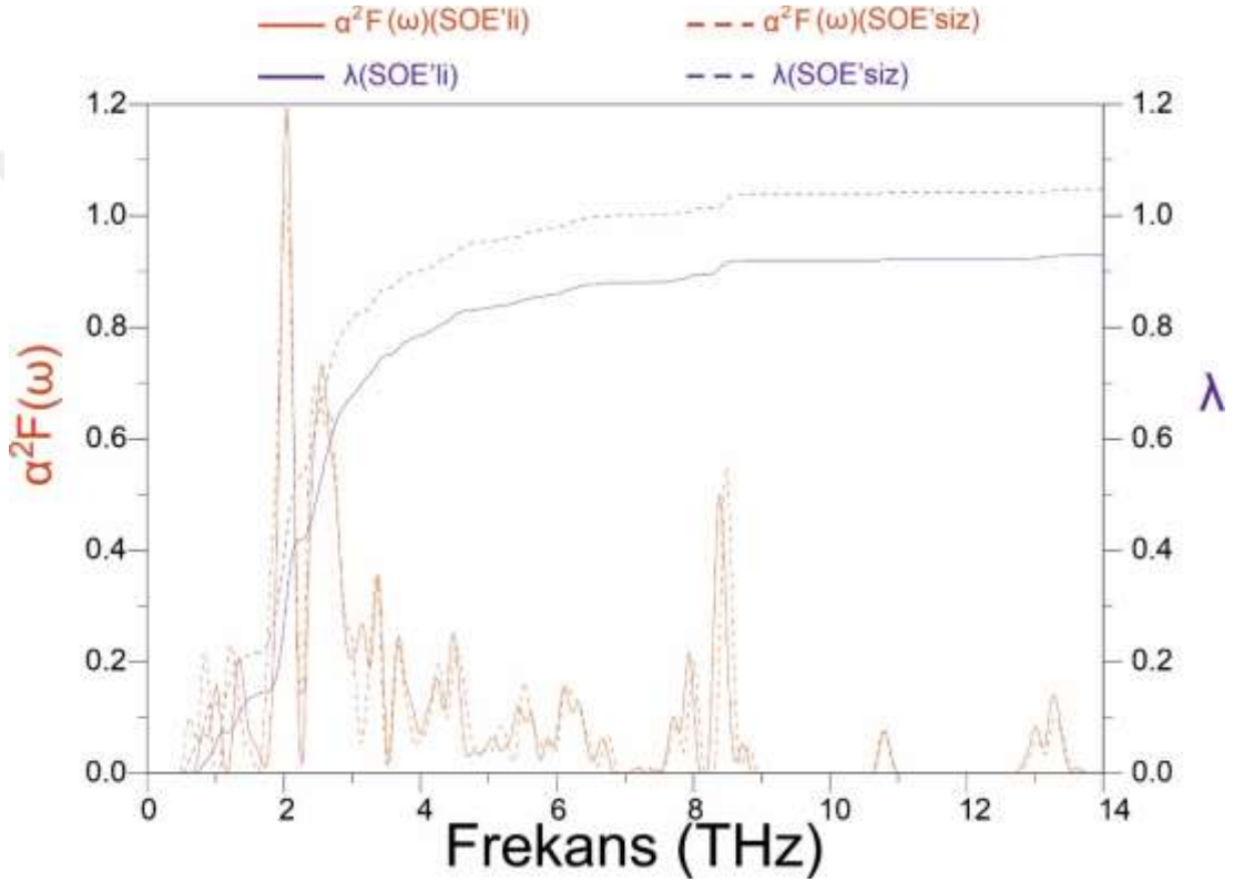
Şekil 3.7. Eliashberg spektral fonksiyonu \alpha^2 F(\omega) (kırmızı çizgi) ve frekans \text{Mg}_2\text{Ir}_3\text{Si} 'nin \text{Mg}_2\text{Cu}_3\text{Si} -tipi yapısı için ortalama elektron-fonon etkileşme parametresi \lambda 'nın (mavi çizgi) bağımlılığı. Spin-orbit etkisi (SOE) olmayan karşılık gelen sonuçlar kesikli çizgilerle gösterilmiştir.
