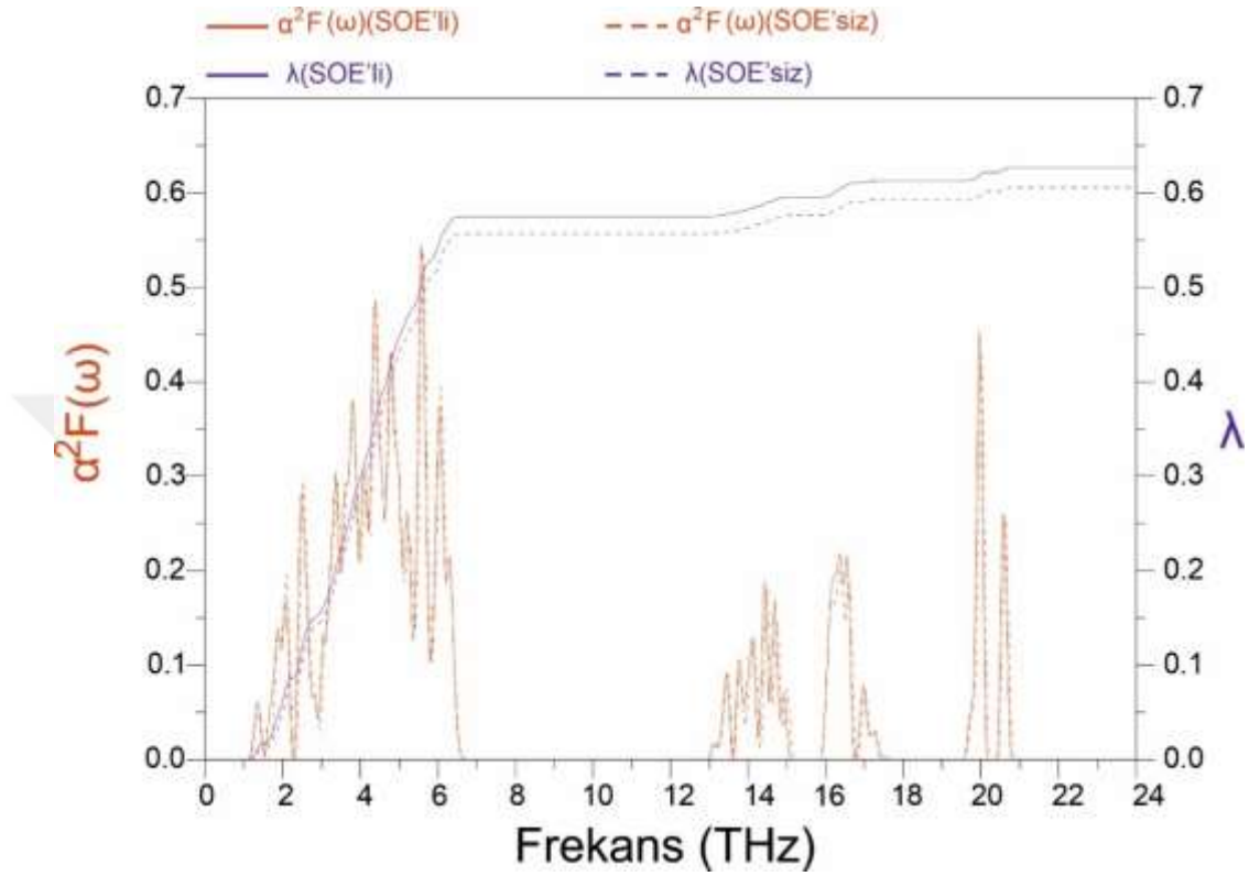
Şekil 4.11. \text{Re}_7\text{B}_3 malzemesi için hesaplanmış \alpha^2 F(\omega) - \lambda grafiğinin frekansla değişiminin gösterilmesi. SOE'siz sonuçlar kesikli çizgilerle gösterilir.
