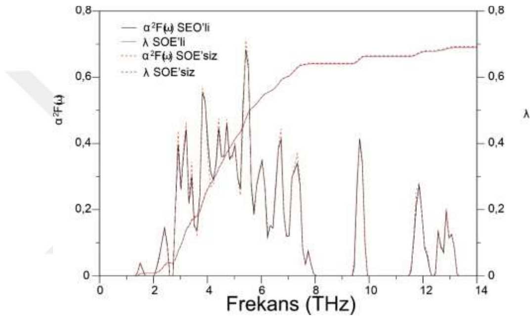
Şekil 5.6. Mo_3P malzemesi için hesaplanmış \alpha^2F(\omega) - \lambda grafiğinin frekansla değişiminin gösterilmesi
