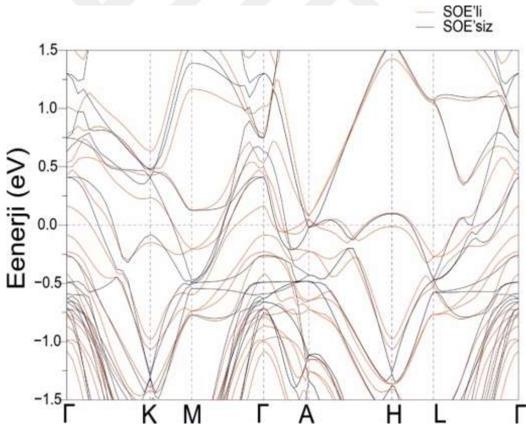
Şekil 3.2. \text{Mg}_2\text{Ir}_3\text{Si} için elektronik yapı.
