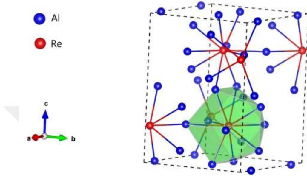
Şekil 6.1. Al 6 Re süperiletkeninin kristal yapısı.
