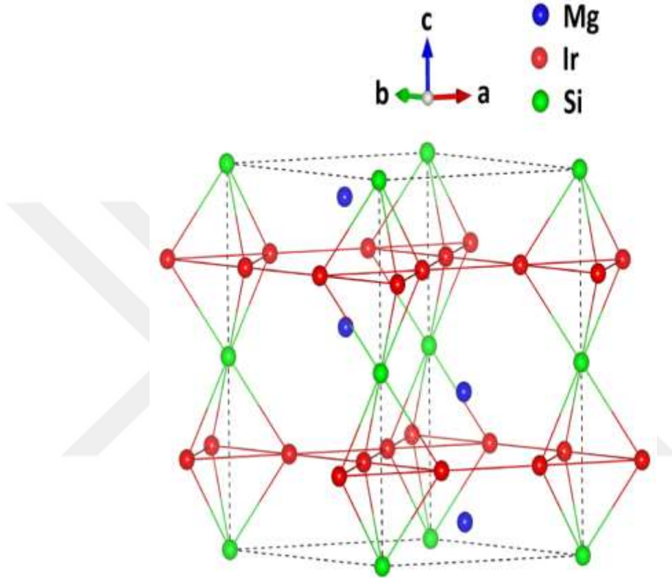
Şekil 3.1. \text{Mg}_2\text{Ir}_3\text{Si} malzemesi için kristal yapının gösterimi.
