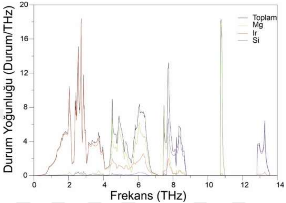
Şekil 3.6. Mg_2Ir_3Si bileşiği için fonon DOS grafiği.
