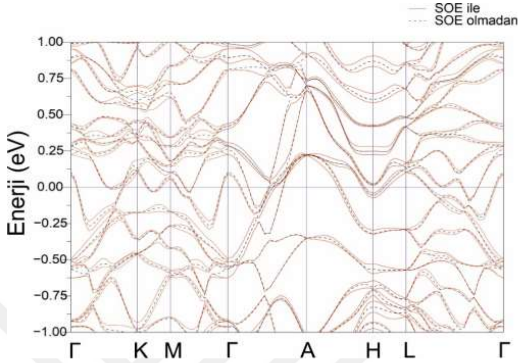
Şekil 4.2. Hekzagonal örgünün birinci Brillouin bölgesinde yüksek simetri yönleri boyunca spin-orbit etkileşim (SOE) olan ve olmayan Ru 7 B 3 'ün hesaplanan elektronik bant yapısı. Enerji ölçeği, Fermi düzeyi E_F = 0 'a göre tanımlanır.
