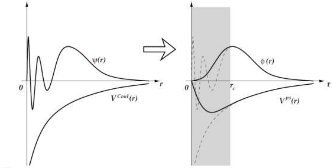
Şekil 2.1. Bir sistemin Coulomb potansiyeli ve dalga fonksiyonu ve pseudopotansiyel ve karşılık gelen sanal dalga fonksiyonu [15].
