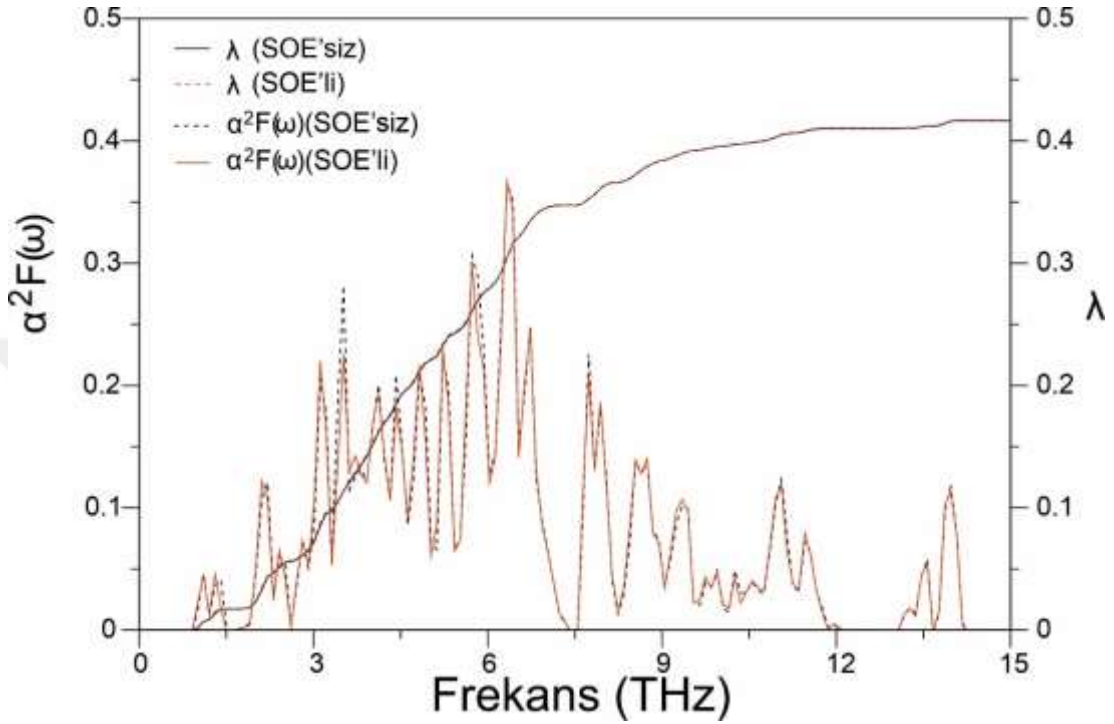
Şekil 6.6. \text{Al}_6\text{Re} malzemesi için hesaplanmış \alpha^2F(\omega) - \lambda grafiğinin frekansla değişiminin gösterilmesi.
