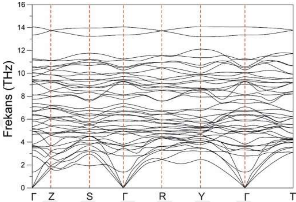
Şekil 6.4. \text{Al}_6\text{Re} için fonon dağılım eğrileri
