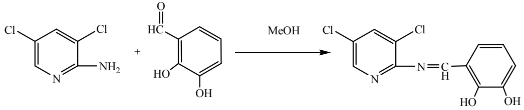
Şekil 3.3. (3) bileşiğinin sentezi
