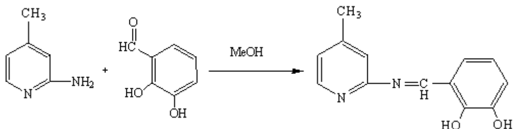
Şekil 3.5. (5) bileşiğinin sentezi
