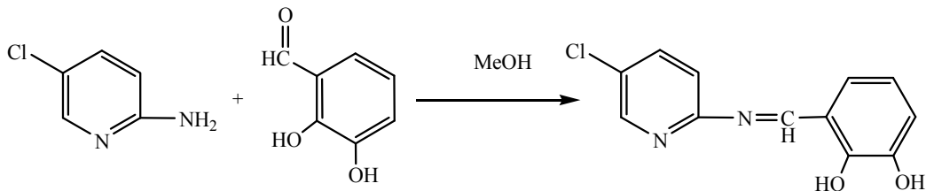
Şekil 3.1. (1) bileşiğinin sentezi
