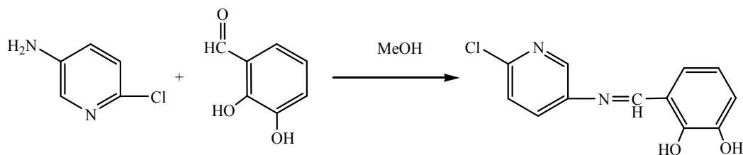
Şekil 3.2. (2) bileşiğinin sentezi
