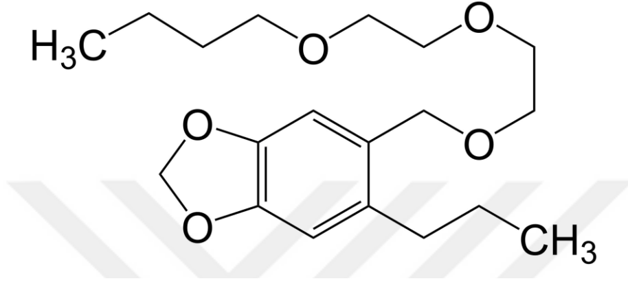
Şekil 2.14. Piperonyl butoxide sinerjist maddesinin kimyasal formülü (Anonymous 7)
