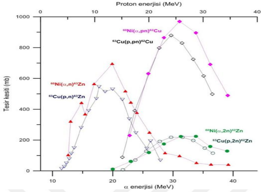
Şekil 1.5 ^{64}\text{Zn}^* Bileşik çekirdeğinin oluşum ve bozunum kanalları için tesis kesitleri (Gloshal 1950)
