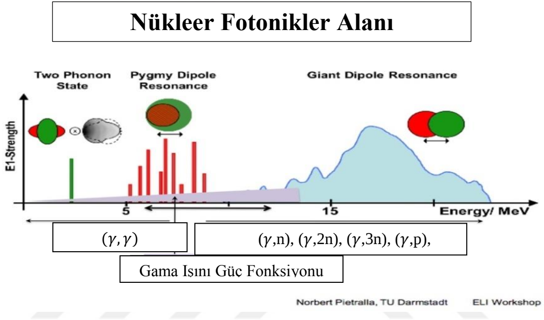
Şekil 3.5 Nükleer Fotonik Alanı (Utsunomiya 2003).
