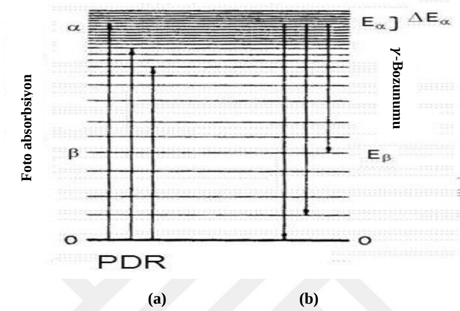
Şekil 3.6 Ortalama geçiş gücü (a) Yüksek uyarılmış durumlara fotoabsorbsiyon için (b) Aynı J^\pi seviyelerinin grubunun, düşük enerji seviyesi E_f 'e düşmesinden kaynaklanan gama bozunması için (Mamtimin 2014)
