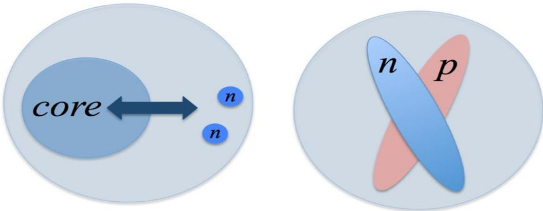
Şekil 3.8 Pygmy ve scissor rezonans parçacık salınım modları (Kgashne 2016)
