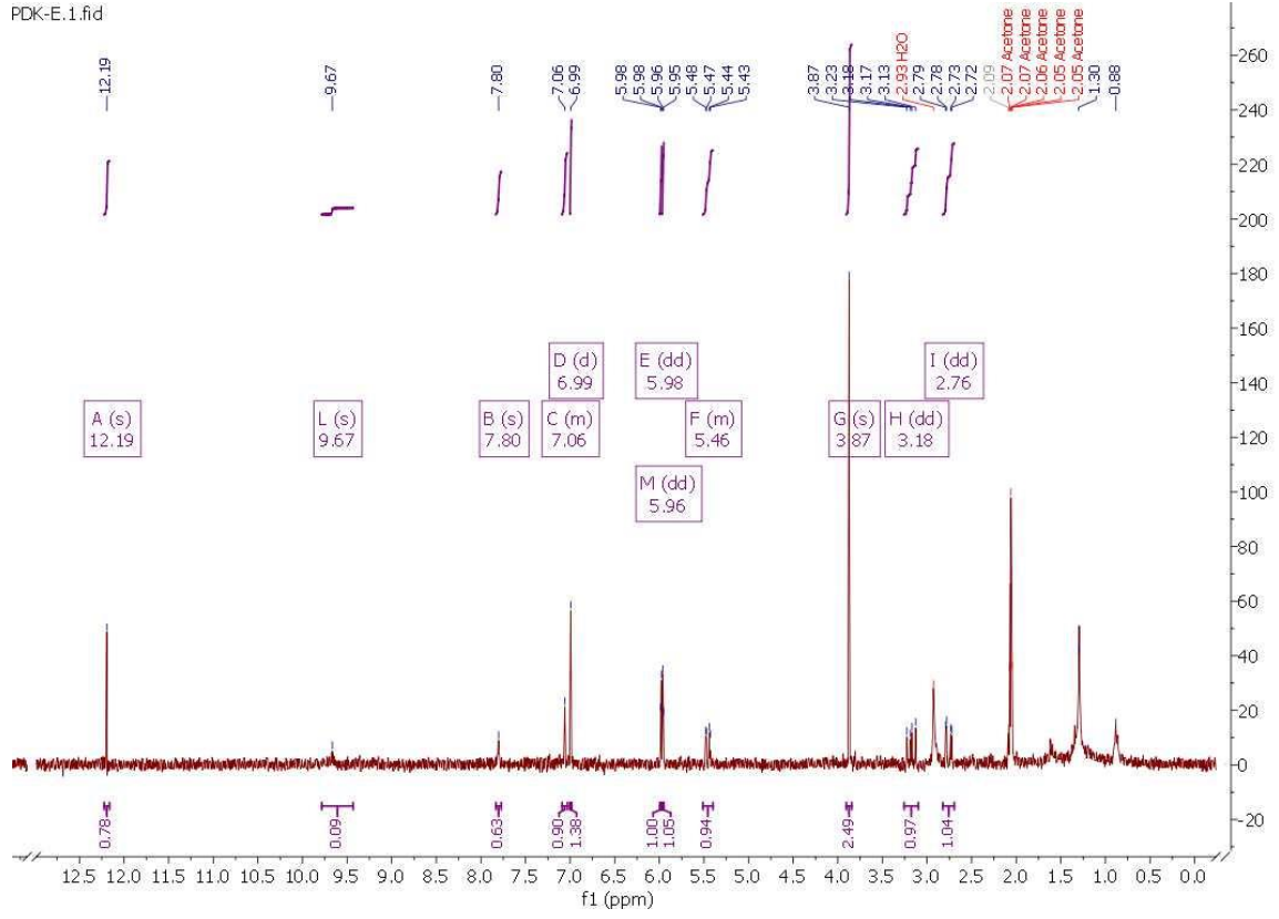
Şekil 4.36. M7 metaboliti ^1\text{H} -NMR spektrumu
