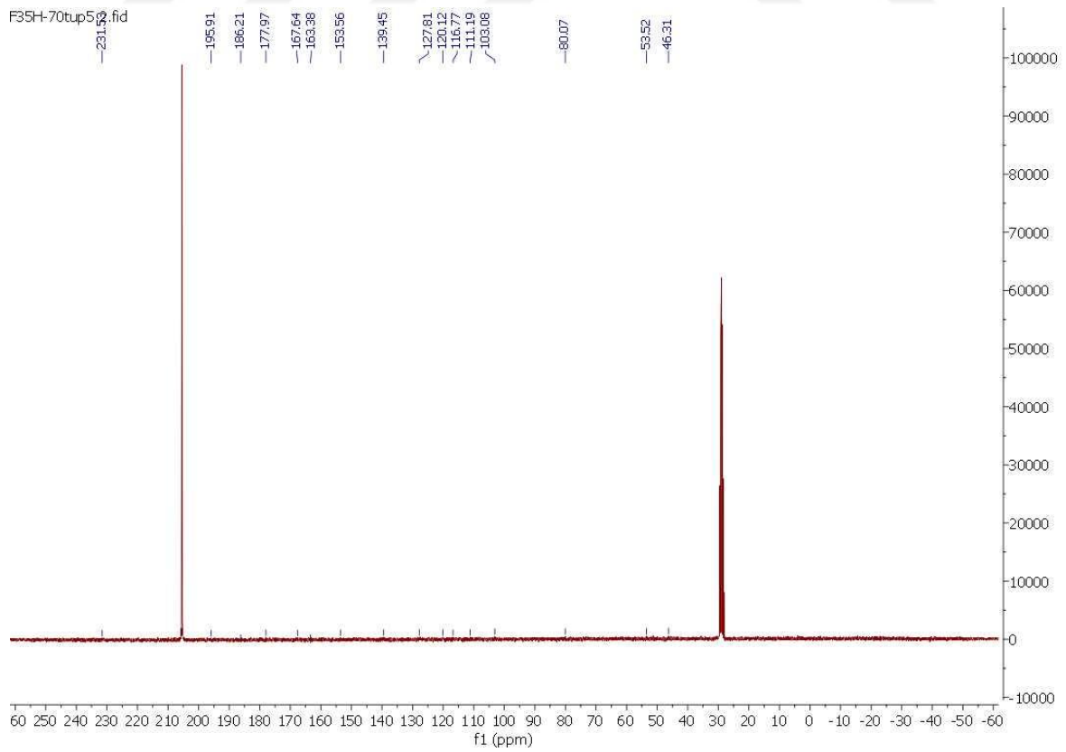
Şekil 4.53. M10 metaboliti ^{13}\text{C} -NMR spektrumu
