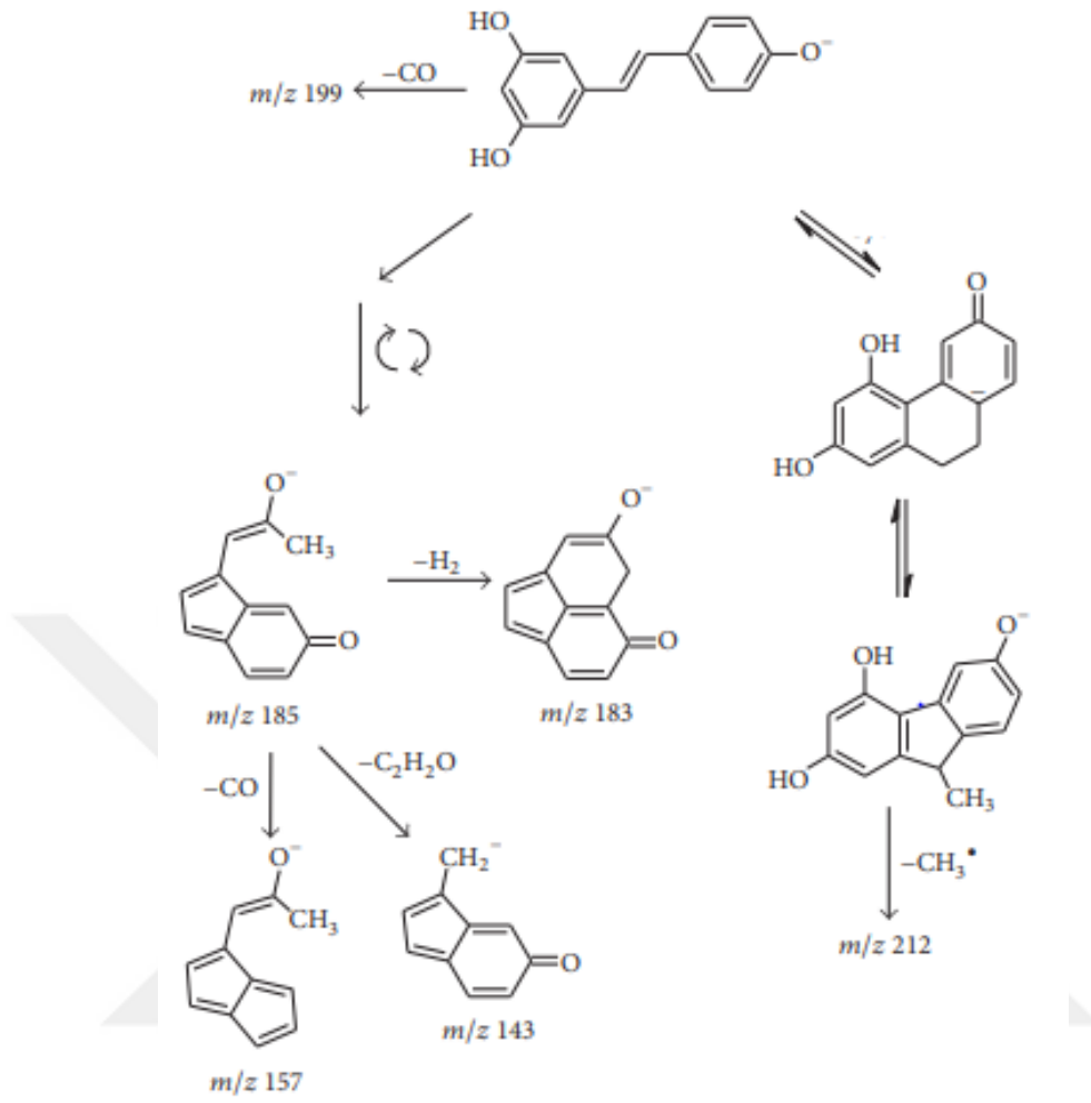
Şekil 4.5. Resveratrol'ün SK-SK spektrumunda parçalanma ürünleri ve m/z değerleri (Flamini, 2013)
