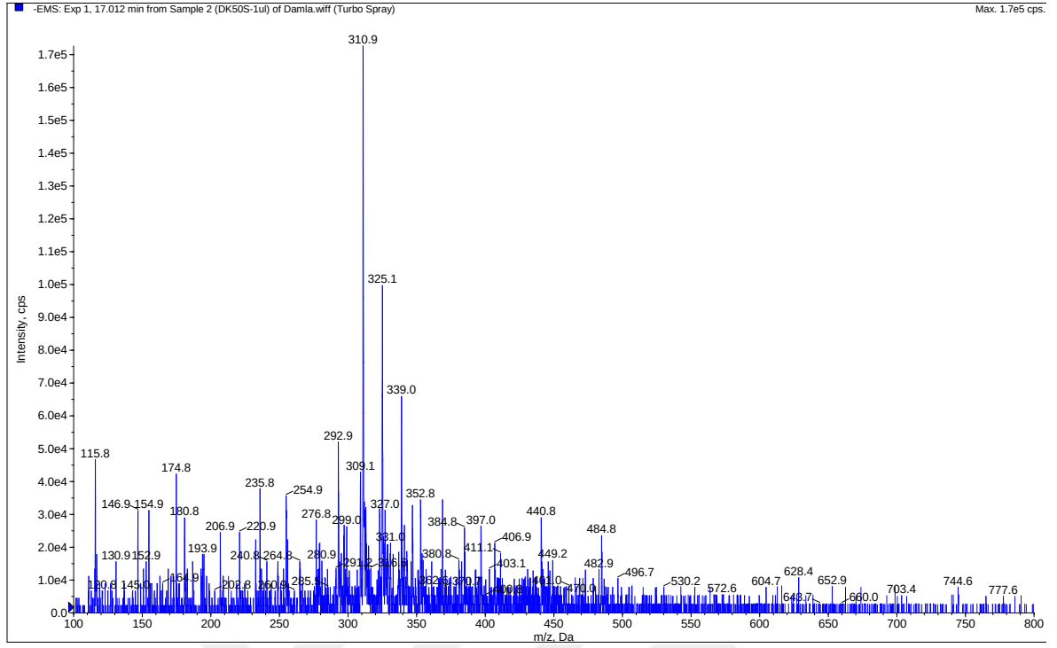
Şekil 4.57. M12 metaboliti kütle spektrumu
