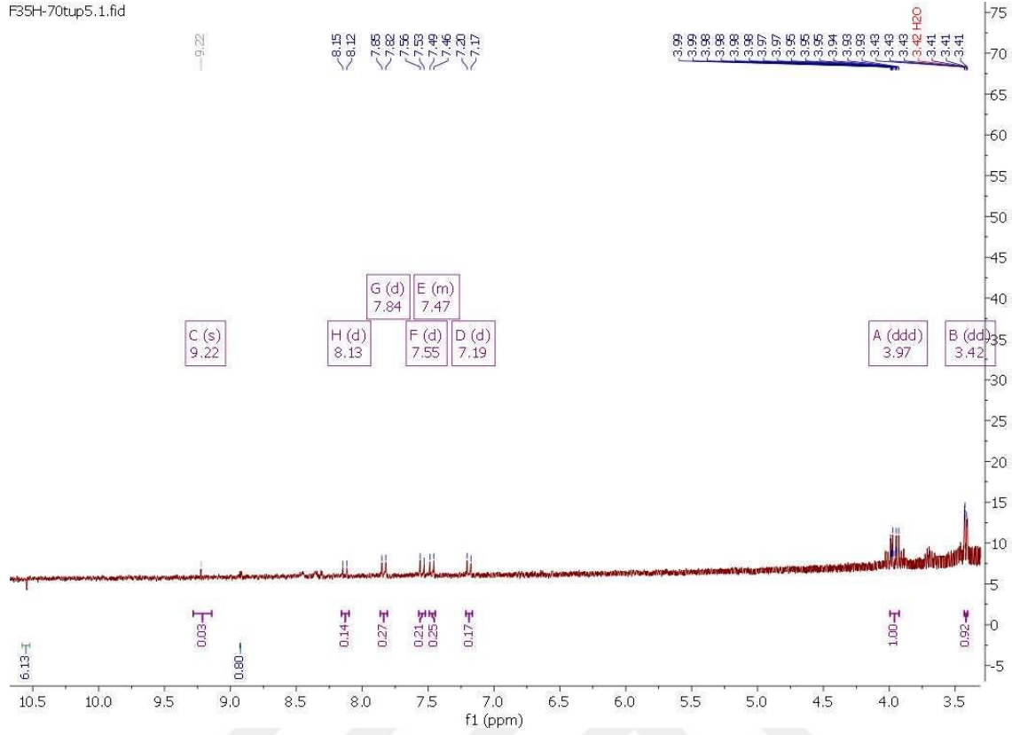
Şekil 4.52. M10 metaboliti ^1\text{H} -NMR spektrumunda 3-10.50 ppm aralığı
