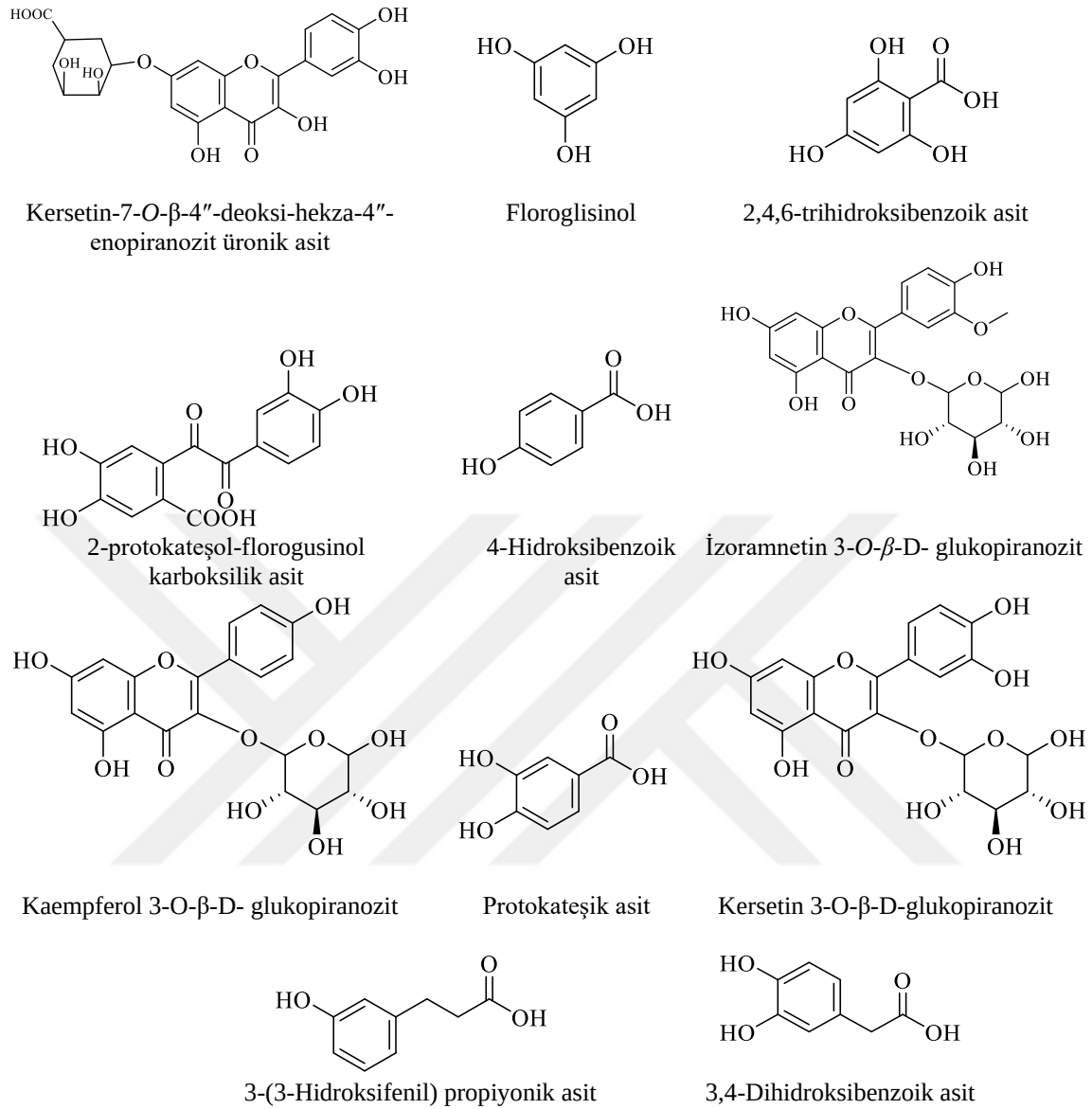
Şekil 2.5. Kersetin metabolitleri
