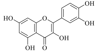
Kerşetin
