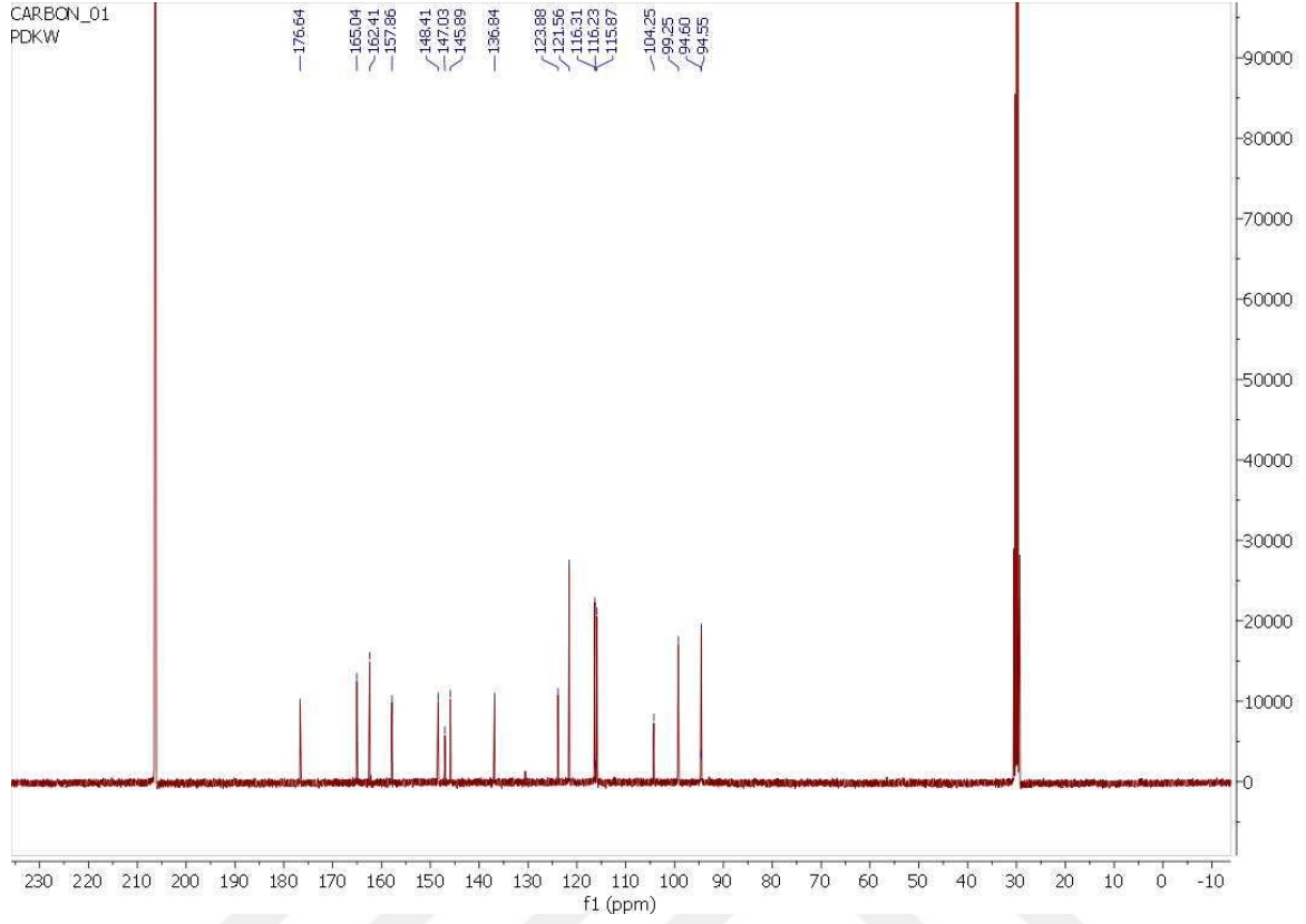
Şekil 4.27. Kersetin'in ^{13}\text{C} -NMR spektrumu
