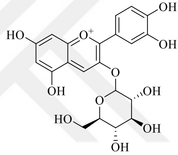
Siyanidin-3-O-glikozit
