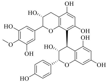
Proantosiyanidin
