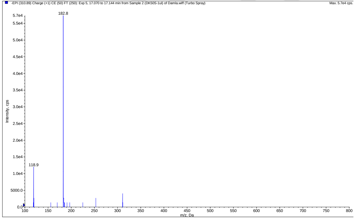
Şekil 4.58. M12 metaboliti SK/KS-KS analizi EPI spektrumu
