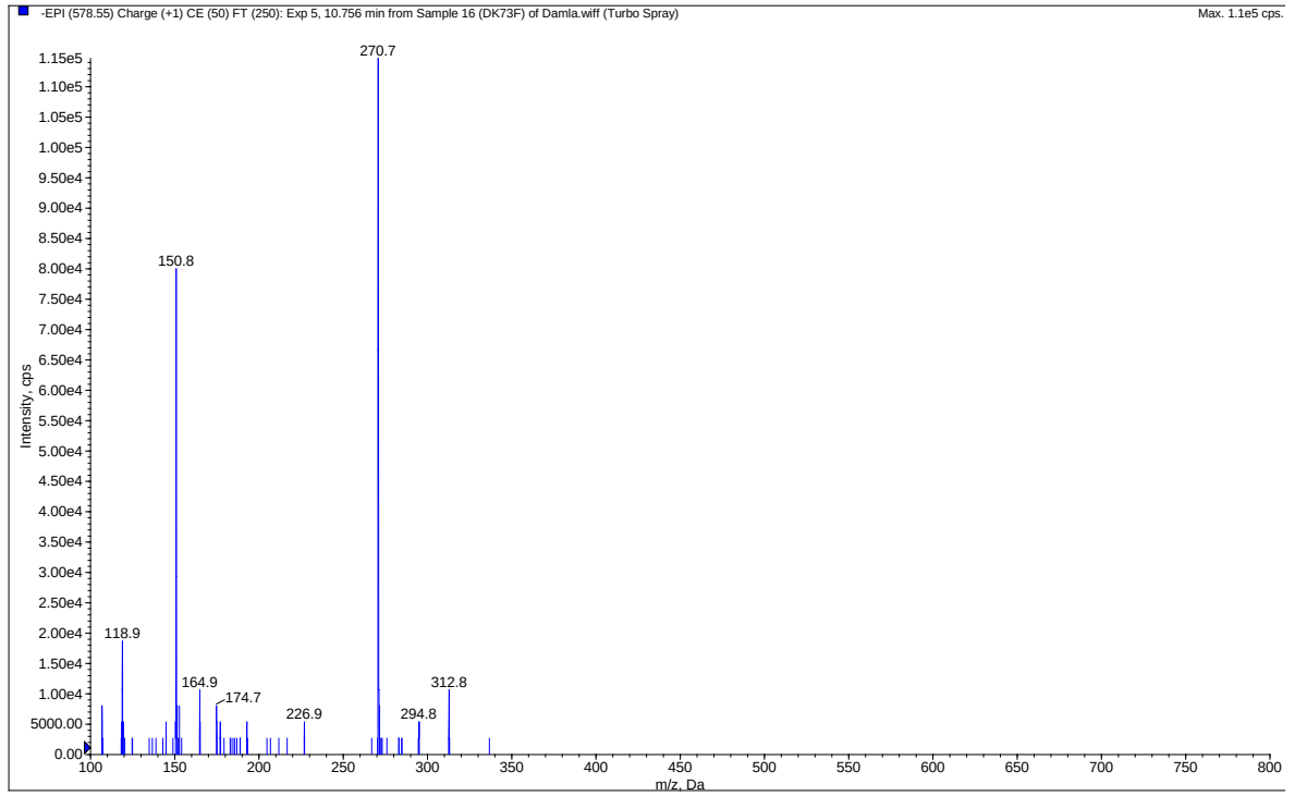
Şekil 4.65. M14 metaboliti EPI kütle spektrumu
