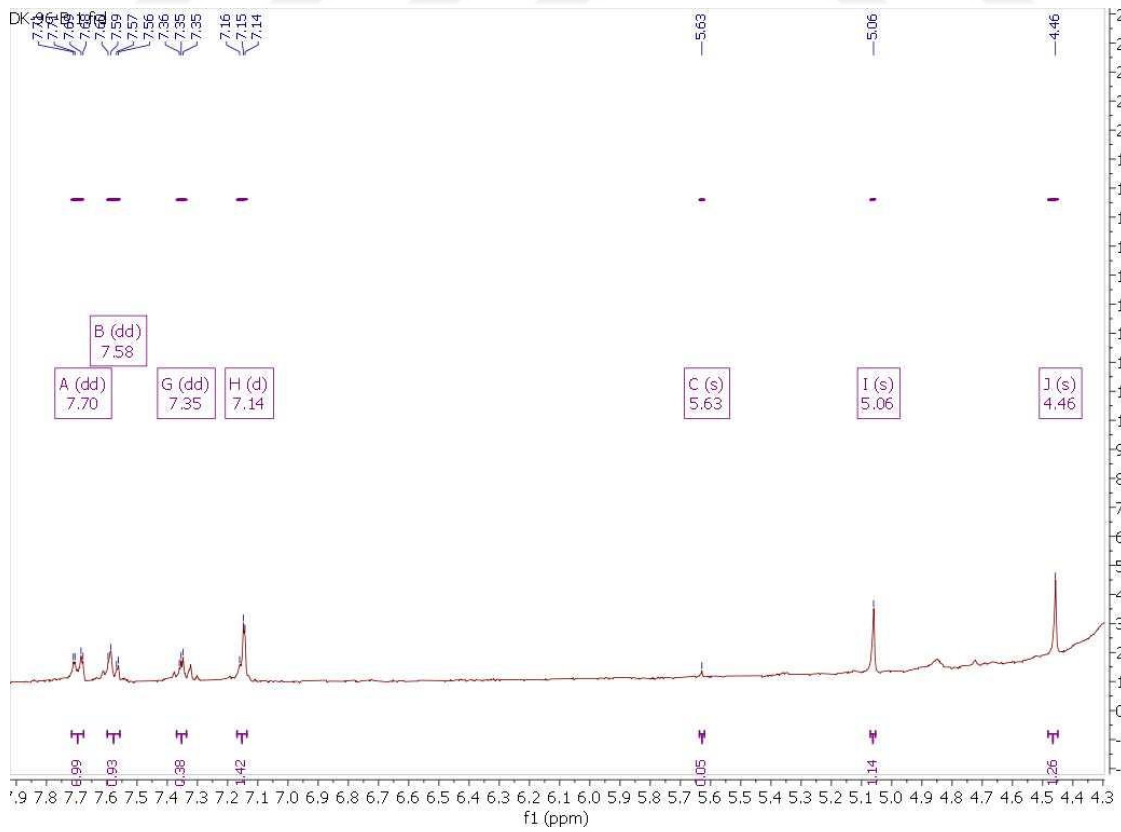
Şekil 4.26. M6 metaboliti ^1\text{H} -NMR spektrumu 4-8 ppm aralığı
