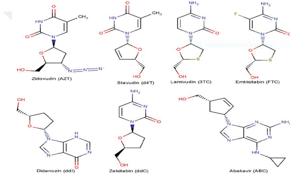
Şekil 6. NRTI'lerin Kimyasal Yapıları
