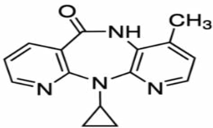
Nevirapine
