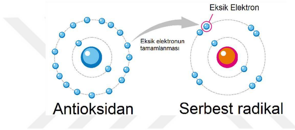
Şekil 11. Antioksidan ve serbest radikal (Başer, 2002)
