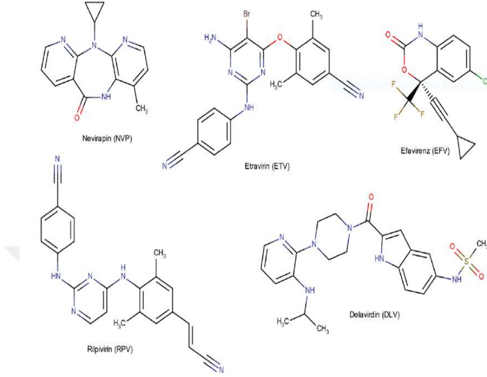
Şekil 8. NNRTI'lerin kimyasal yapıları.
