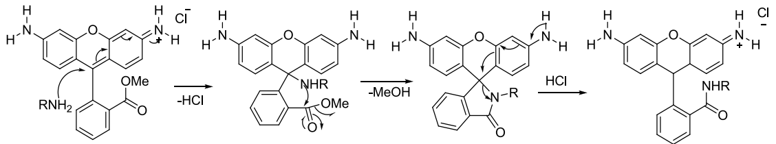
Şekil 1. 21. Alkil Grubu İçermeyen veya mono- N -alkil Rodamin Boyalar ile Primer Aminlerin Reaksiyonu
