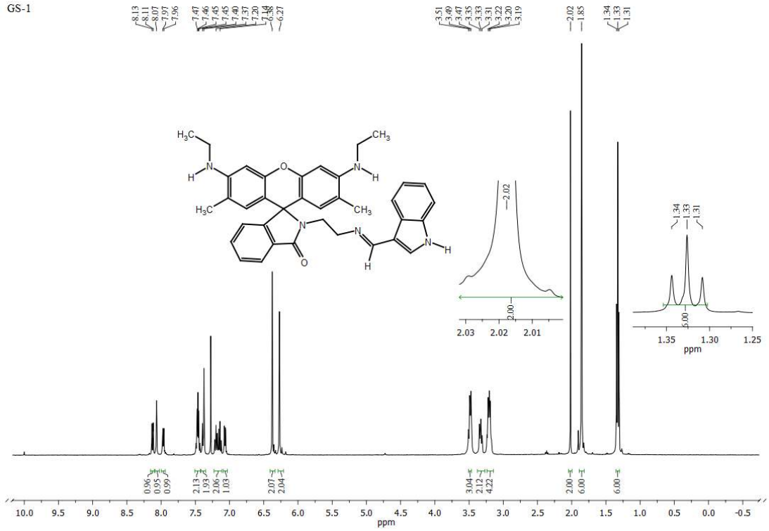
Şekil 3. 6. GS-1 Bileşiğinin ^1\text{H} -NMR Spektrumu
