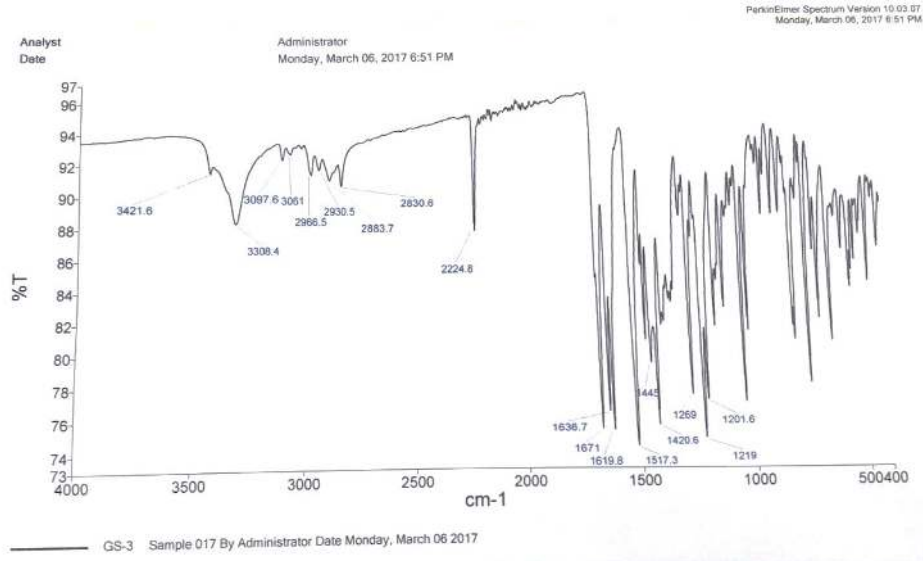
Şekil 3. 15. GŞ-3 Bileşiğinin IR Spektrumu
