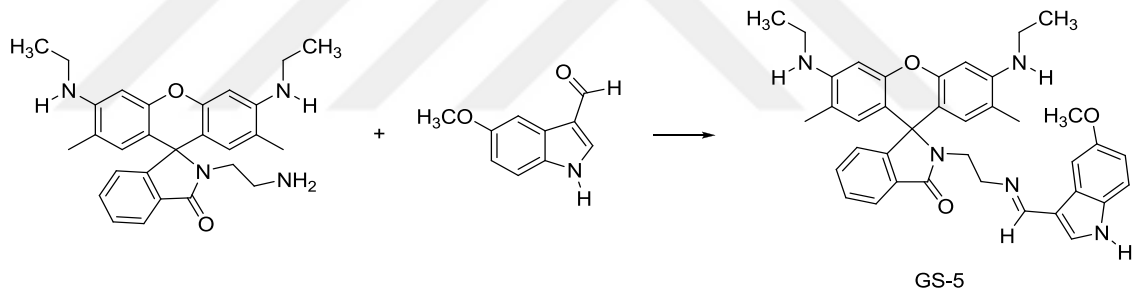
řekil 3. 24. Gř-5 Bileřiėinin Reaksiyon řeması
