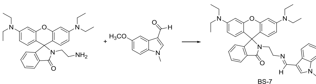
Şekil 3. 69. BS-7 Bileşiğinin Reaksiyon Şeması
