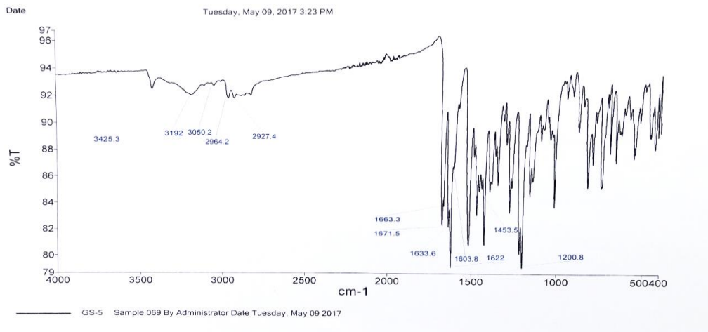
řekil 3. 25. Gř-5 Bileřiėinin IR Spektrumu
