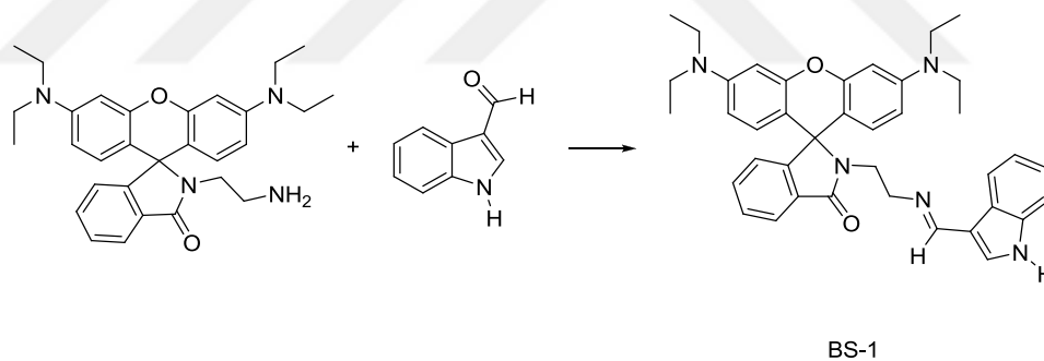
Şekil 3. 39. BS-1 Bileşiğinin Reaksiyon Şeması
