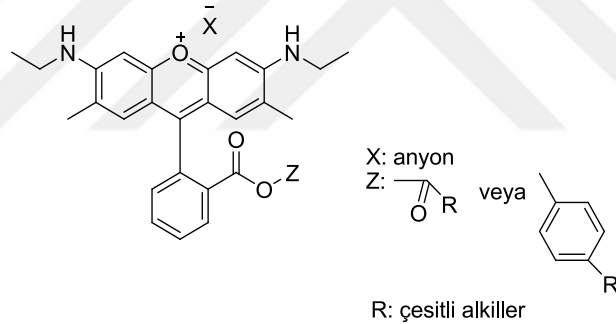
Şekil 1. 22. Rodamin 6G Bileşiğinin Alkil Halojenürlerle Reaksiyonu
