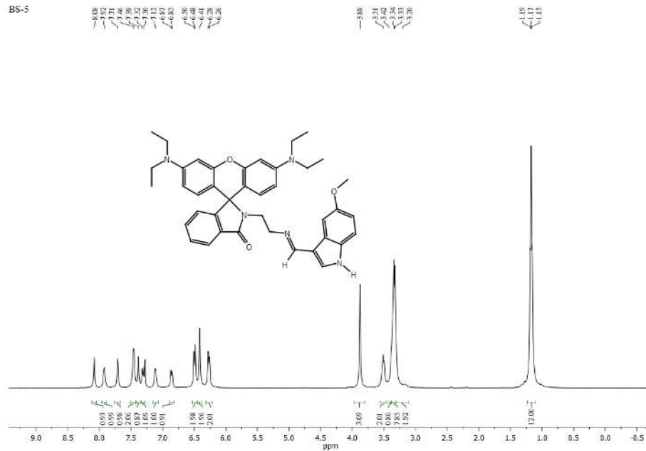
Şekil 3. 61. BS-5 Bileşiğinin ^1\text{H} -NMR Spektrumu
