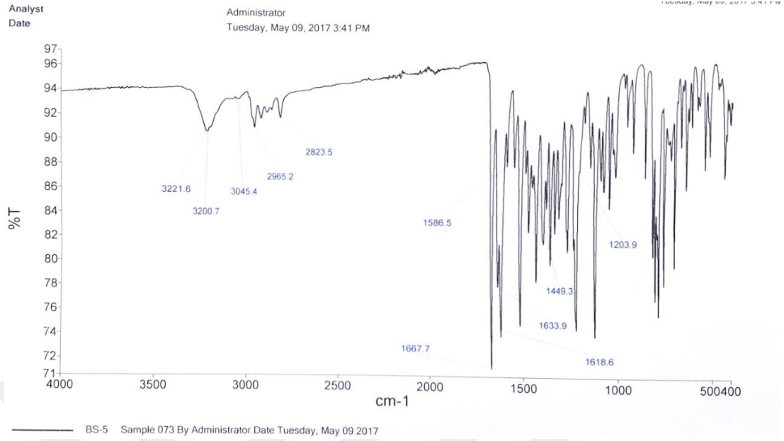
Şekil 3. 60. BS-5 Bileşiğinin IR Spektrumu
