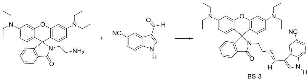
Şekil 3. 49. BS-3 Bileşiğinin Reaksiyon Şeması
