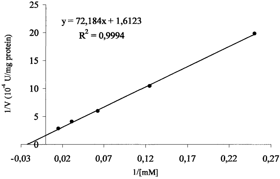
Şekil 70. K1 katalazının H_2O_2 varlığındaki Lineweaver-Burk grafiği
