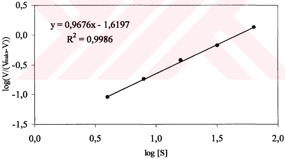
Şekil 71. K1 katalazının H_2O_2 varlığında elde edilen Hill grafiği
