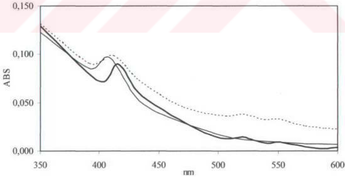
Şekil 18. A5 katalazının 350-600 nm arasındaki absorpsiyon spektrumu ( ____ 50 mM fosfat tamponu (pH 7,5) içindeki doğal katalaz, ____ 100 mM NaOH, 100 mM piridin ve 2 mM sodyum ditiyonit ile indirgenmiş katalaz, ..... 10 mM KCN ile muamele edilmiş katalaz)
