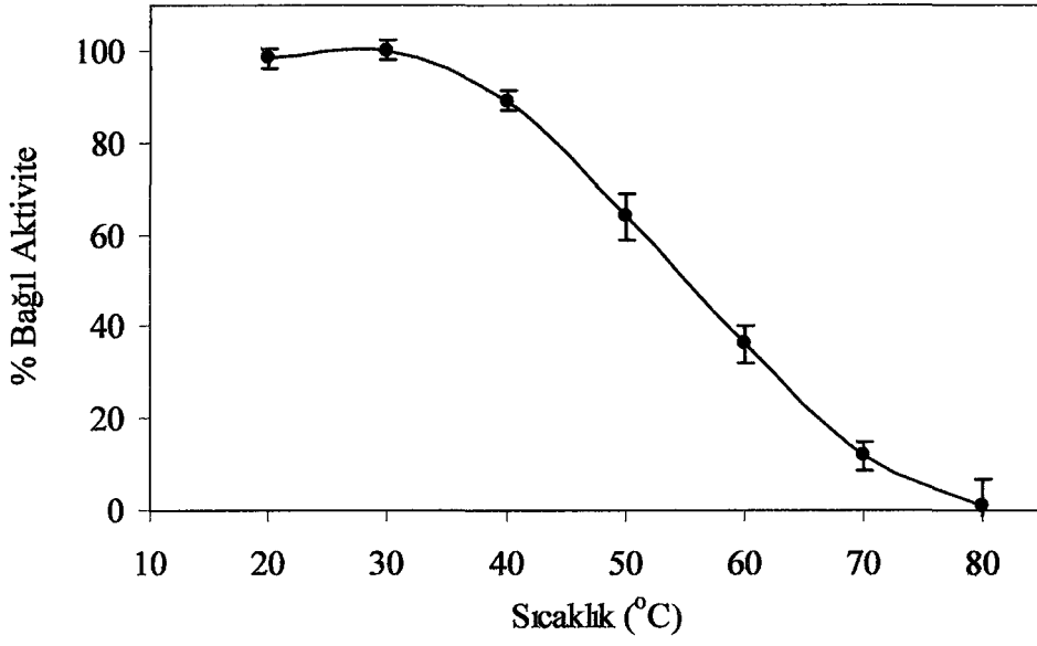
Şekil 24. TK4 suşundan elde edilen katalaz aktivitesinin sıcaklıkla ilişkisi
