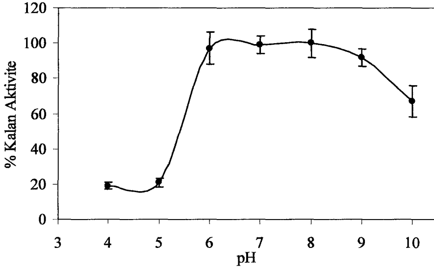
Şekil 34. TK4 suşundan elde edilen katalazın pH kararlılık grafiği
