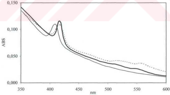
Şekil 13. TK4 katalazının 350-600 nm arasındaki absorpsiyon spektrumu ( — 50 mM fosfat tamponu (pH 7,5) içindeki doğal katalaz, - - - 100 mM NaOH, 100 mM piridin ve 2 mM sodyum ditiyonit ile indirgenmiş katalaz, ..... 10 mM KCN ile muamele edilmiş katalaz)
