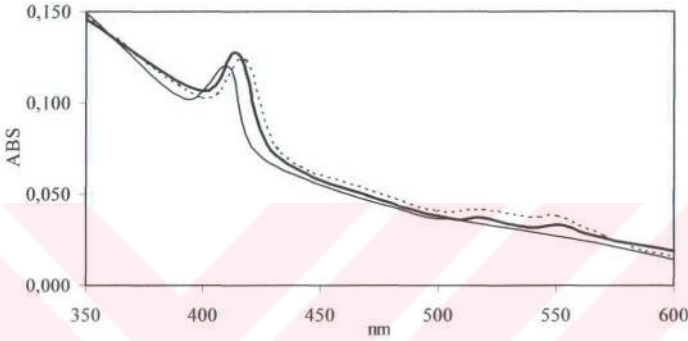
Şekil 14. A9 katalazının 350-600 nm arasındaki absorbsiyon spektrumu ( ____ 50 mM fosfat tamponu (pH 7,5) içindeki doğal katalaz, _____ 100 mM NaOH, 100 mM piridin ve 2 mM sodyum ditiyonit ile indirgenmiş katalaz, ..... 10 mM KCN ile muamele edilmiş katalaz)
