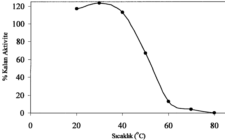
Şekil 55. K4 katalazının 60. dakikadaki termal kararlılık grafiği
