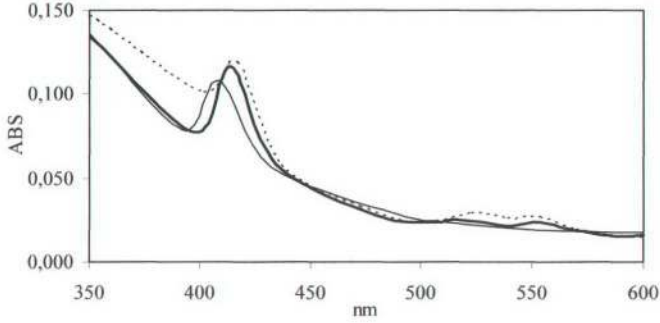
Şekil 12. Ay9 katalazının 350-600 nm arasındaki absorpsiyon spektrumu ( — 50 mM fosfat tamponu (pH 7,5) içindeki doğal katalaz, - - - 100 mM NaOH, 100 mM piridin ve 2 mM sodyum ditiyonit ile indirgenmiş katalaz, ..... 10 mM KCN ile muamele edilmiş katalaz)
