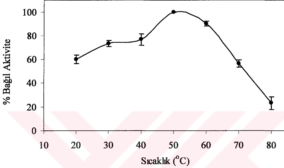
Şekil 28. K4 suşundan elde edilen katalaz aktivitesinin sıcaklıkla ilişkisi
