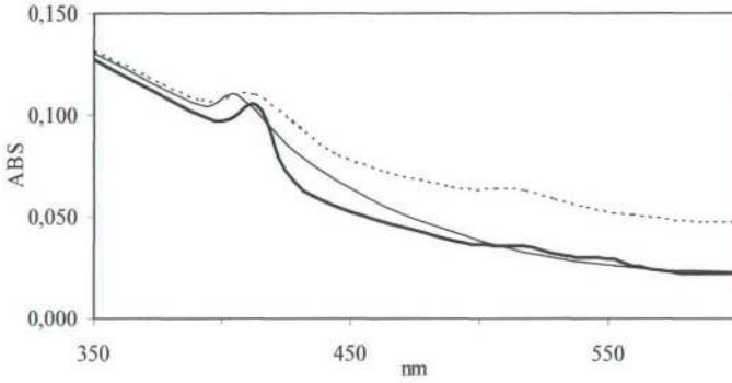
Şekil 17. K4 katalazının 350-600 nm arasındaki absorpsiyon spektrumu ( ____ 50 mM fosfat tamponu (pH 7,5) içindeki doğal katalaz, ____ 100 mM NaOH, 100 mM piridin ve 2 mM sodyum ditiyonit ile indirgenmiş katalaz, ..... 10 mM KCN ile muamele edilmiş katalaz)
