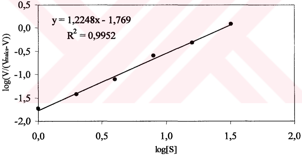
Şekil 75. K4 katalazının H_2O_2 varlığında elde edilen Hill grafiği
