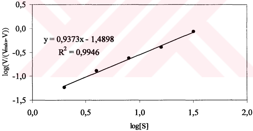
Şekil 77. A5 katalazının H_2O_2 varlığında elde edilen Hill grafiği
