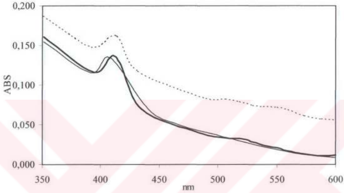
Şekil 19. A6 katalazının 350-600 nm arasındaki absorpsiyon spektrumu ( — 50 mM fosfat tamponu (pH 7,5) içindeki doğal katalaz, — 100 mM NaOH, 100 mM piridin ve 2 mM sodyum ditiyonit ile indirgenmiş katalaz, ..... 10 mM KCN ile muamele edilmiş katalaz)
