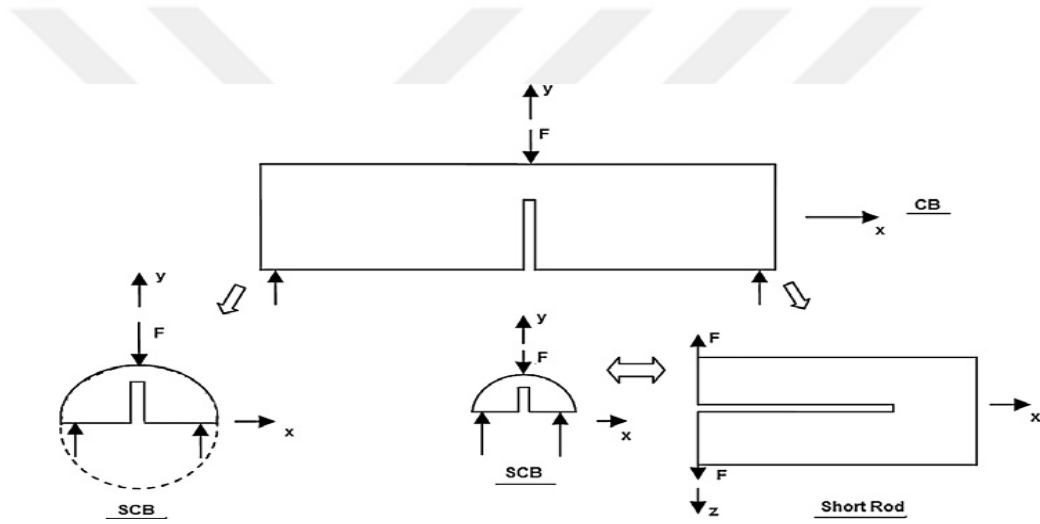
Şekil 3. 3 ISRM tarafından önerilmiş karot bazlı kırılma tokluğu numunelerinin bazılarının şematik görünümü [41]
