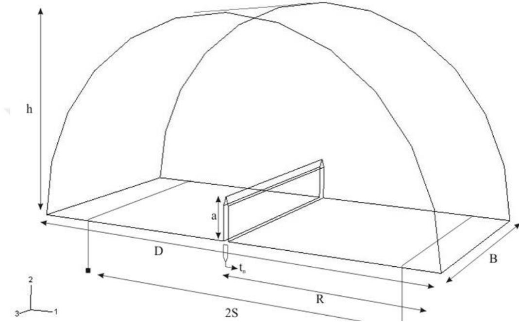
Şekil 4. 16 SCB numunesinin taslağı [49]
