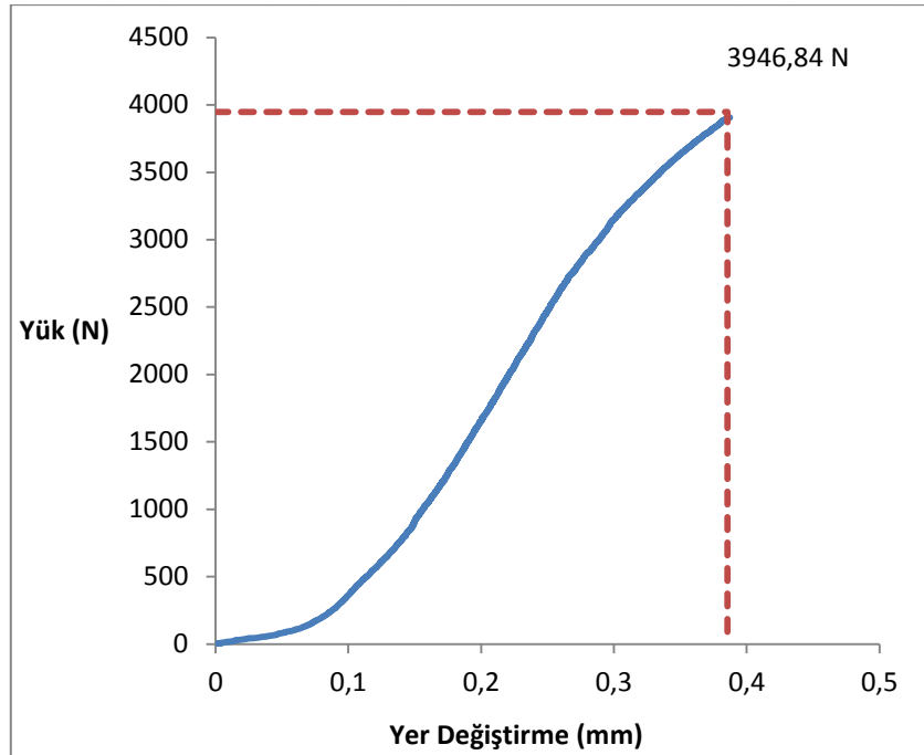
Ek 3.2. Burdur Koyu Bej kiretařına ait numunelerin örnek yük-yer deęiřtirme (deformasyon) eęrisi
