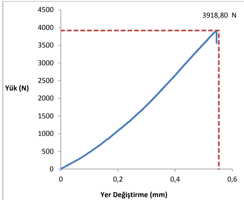
Ek 3.4. Kütahya Menekşe hakiki mermerine ait numunelerin örnek yük-yer değiştirme (deformasyon) eğrisi
