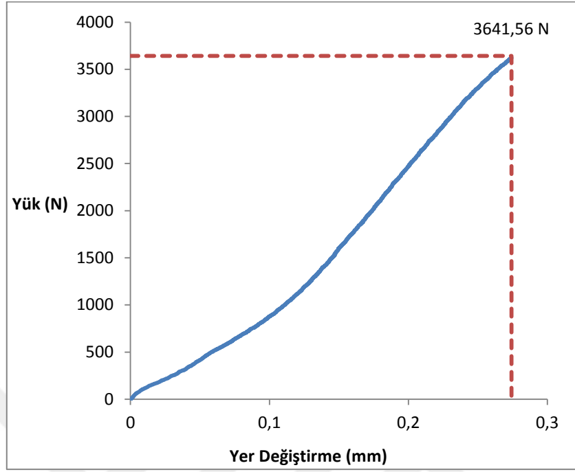
Ek 3.3. Burdur Açık Bej kireçtaşına ait numunelerin örnek yük-yer değiştirme (deformasyon) eğrisi
