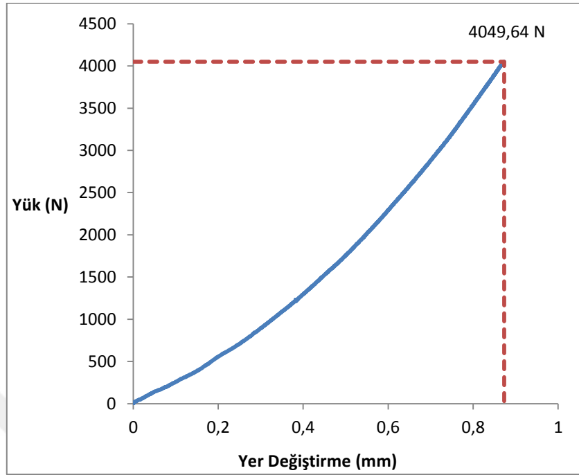
Ek 3.5. Afyon Şeker hakiki mermerine ait numunelerin örnek yük-yer değiştirme (deformasyon) eğrisi
