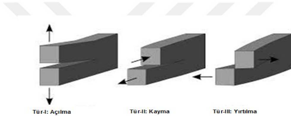
Şekil 3. 2 Kırılma türleri
