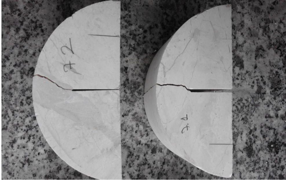
Şekil 4. 13 SCB numunesinin çentik boyunca kırıldıktan sonraki görünümü
