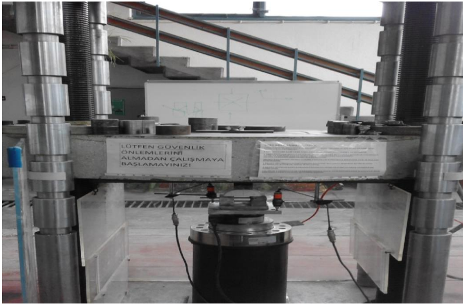
Şekil 4. 11 Hidrolik test cihazı (MTS)
