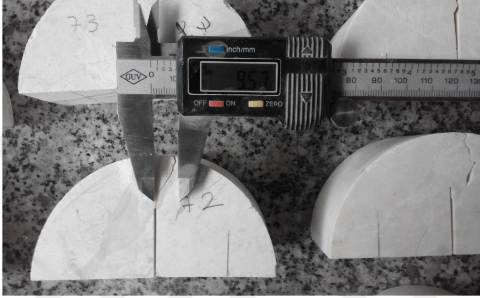
Şekil 4. 14 Çatlak düzleminin elektronik kumpas ile çentik düzlemi ile arasında olan mesafesinin ölçülmesi
