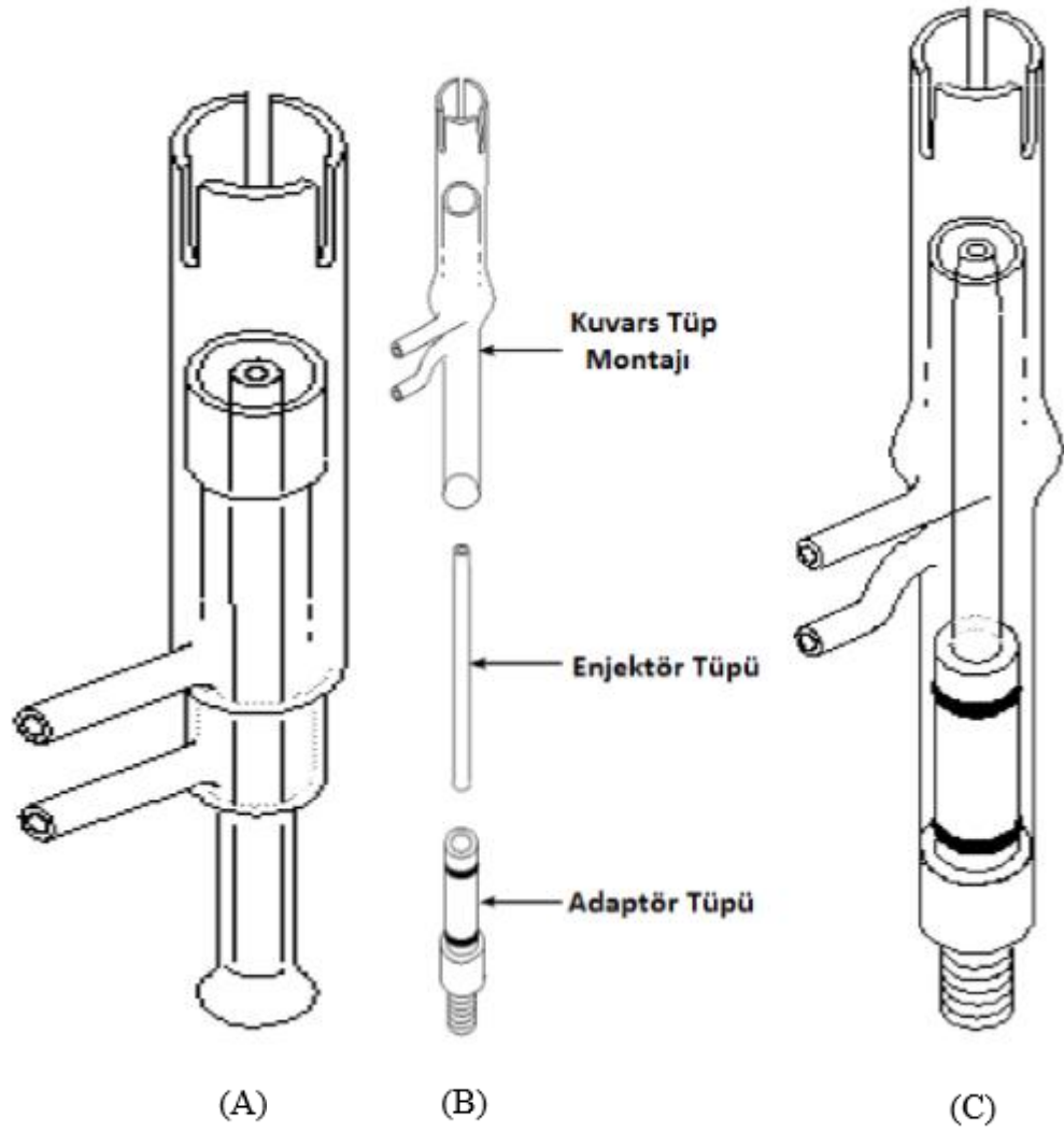
Şekil 2.5. ICP hamlaçları A - tek parça, B - sökülüş, C - monte edilmiş [Boss C.B. ve Fredeen K.J., 2004].
