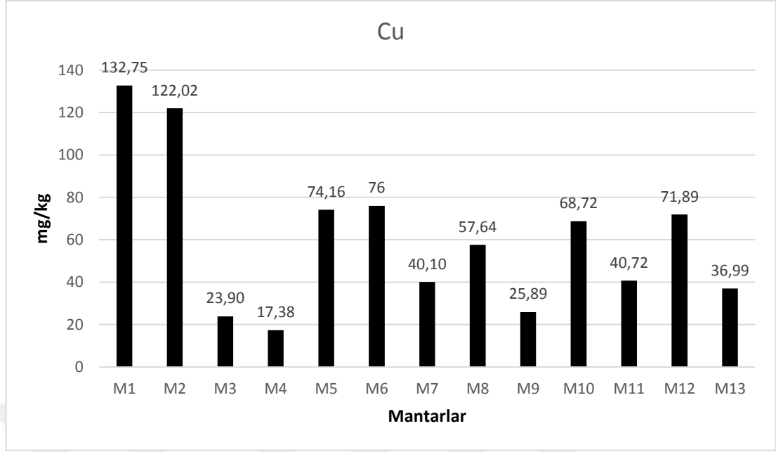
Şekil 4.5. Mantar örneklerinde Cu dağılımı (mg/kg)
