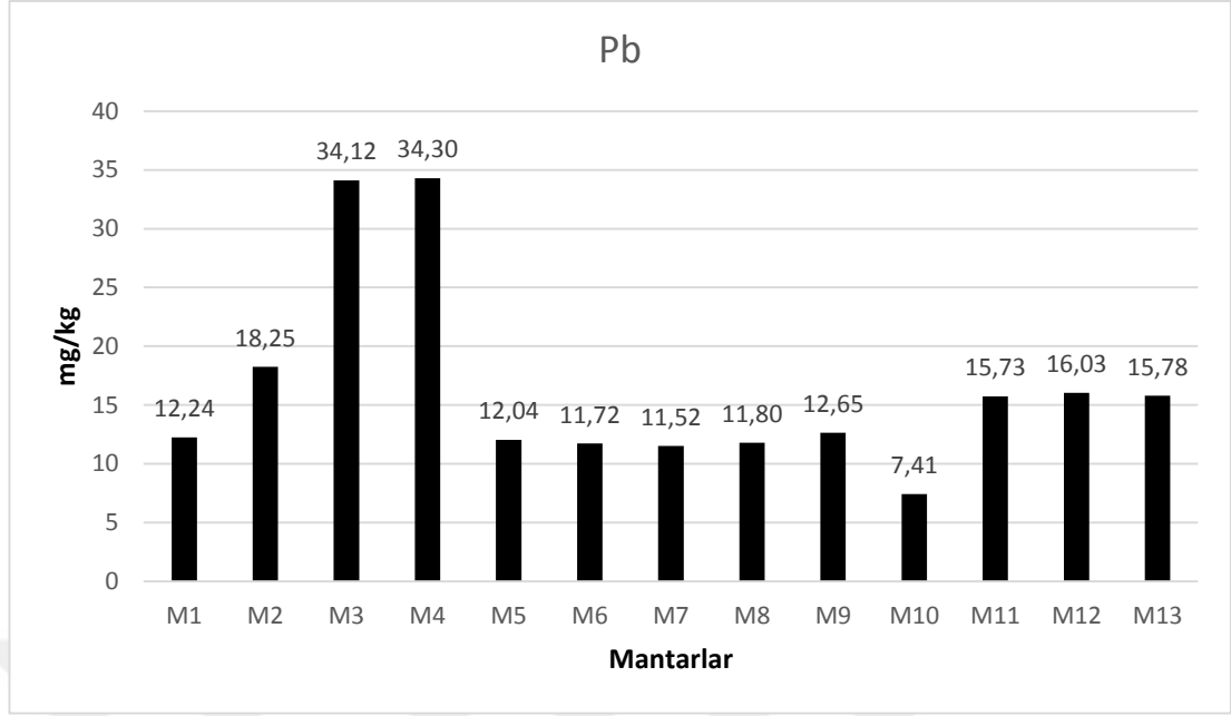
Şekil 4.9. Mantar örneklerinde Pb dağılımı (mg/kg)
