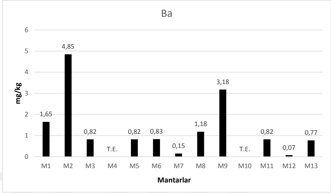
Şekil 4.1. Mantar örneklerinde Ba dağılımı (mg/kg)
