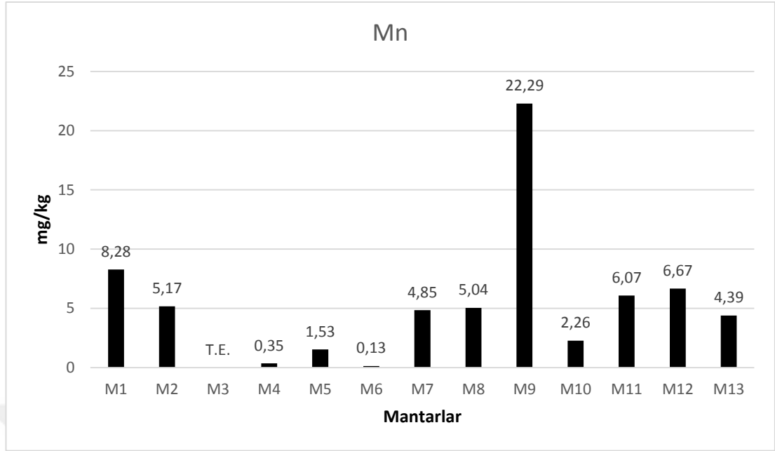
Şekil 4.7. Mantar örneklerinde Mn dağılımı (mg/kg)
