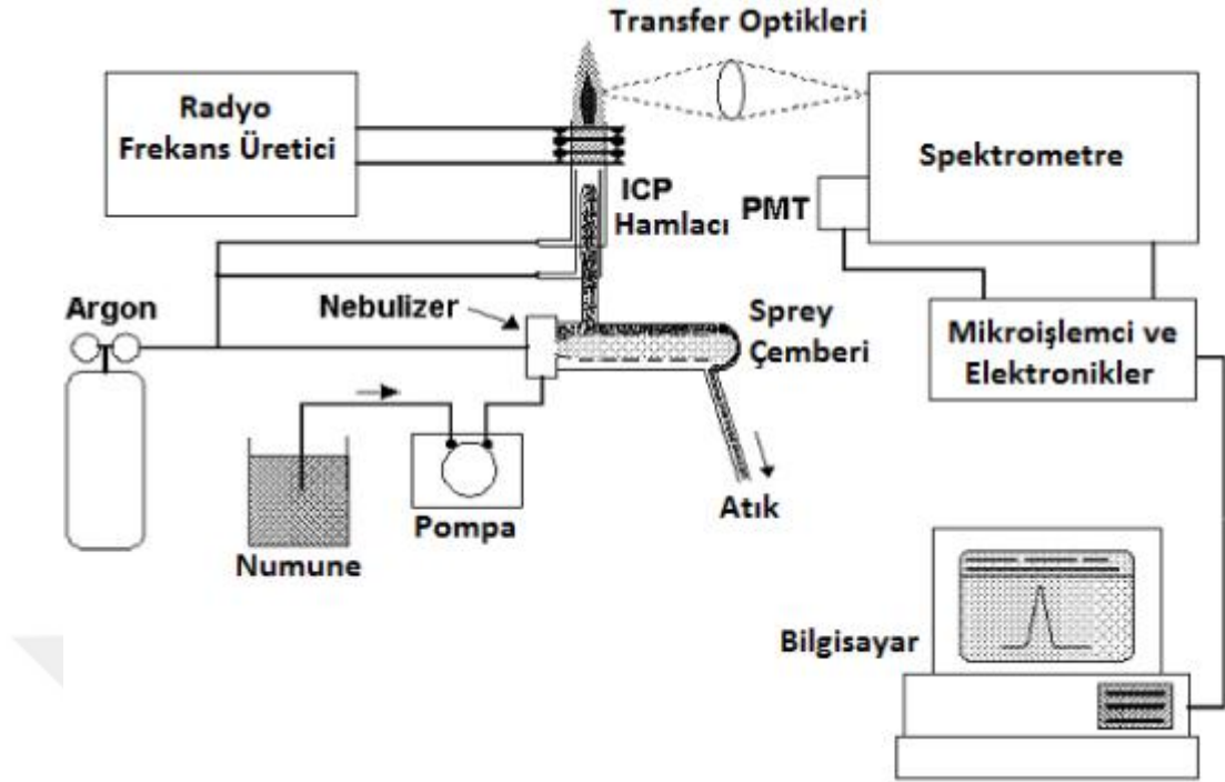
Şekil 2.2. Genel bir ICP-OES cihazının tasarımı ve bileşenleri [Boss C.B. ve Fredeen K.J., 2004].
