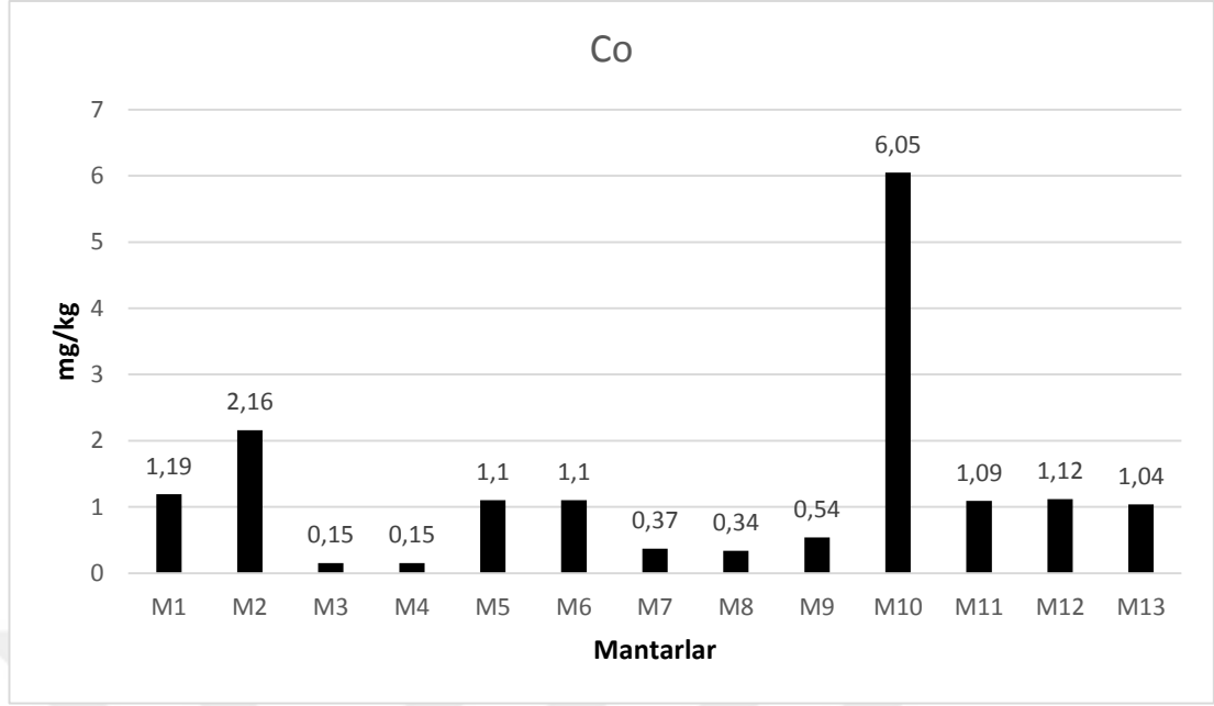
Şekil 4.3. Mantar örneklerinde Co dağılımı (mg/kg)
