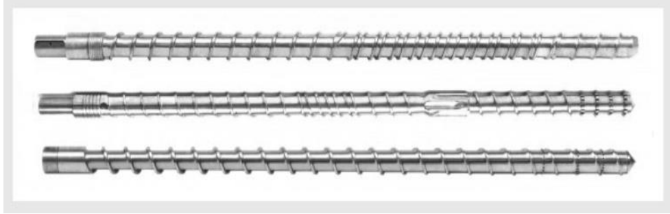
Şekil 8. Ekstrüderde kullanılan farklı vida tipleri [42]
