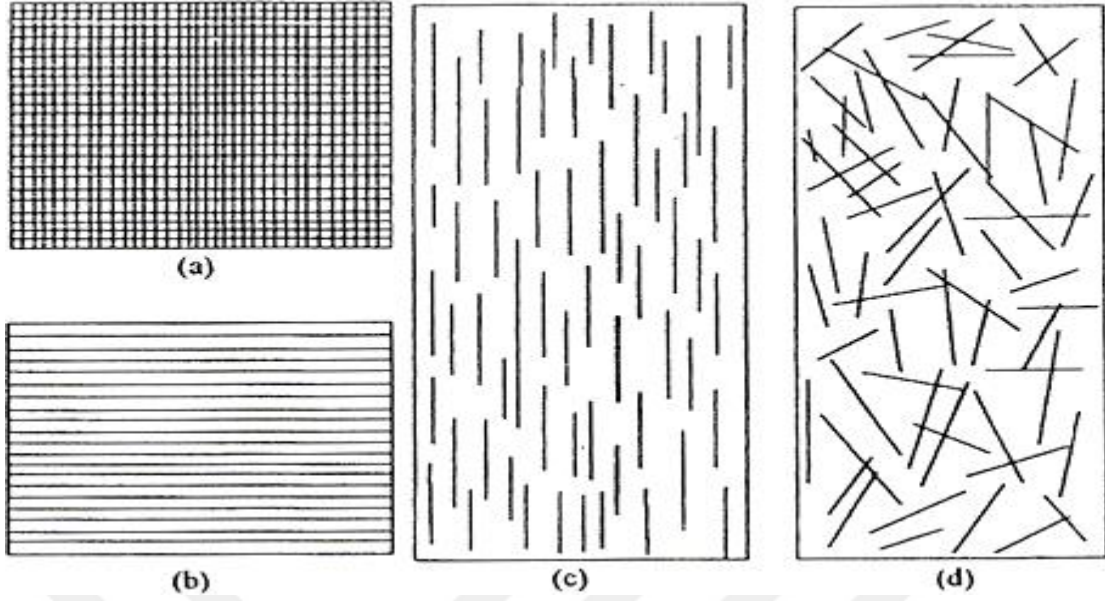
Şekil 1. Elyaf takviyeli kompozitlerde liflerin kompozit içerisindeki dizilişi; a) Örgülü elyaf takviyeli, b) Sürekli elyaf takviyeli, c) Yönlendirilmiş süreksiz elyaf takviyeli, d) Gelişigüzel dağılmış süreksiz elyaf takviyeli kompozitler [15]
