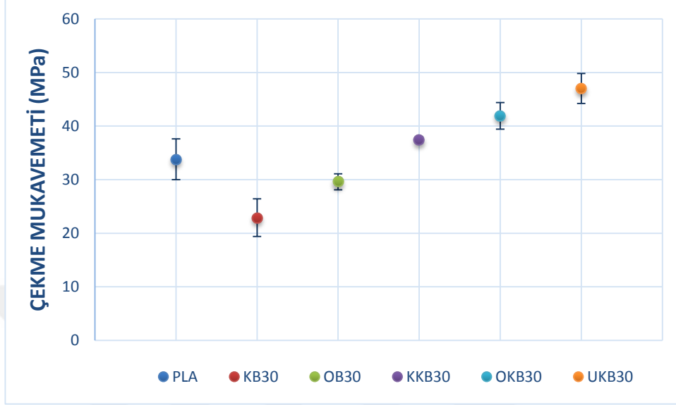
Şekil 34. Kısa ve orta elyaf boyutlu malzemelerin çekme mukavemeti grafiği
