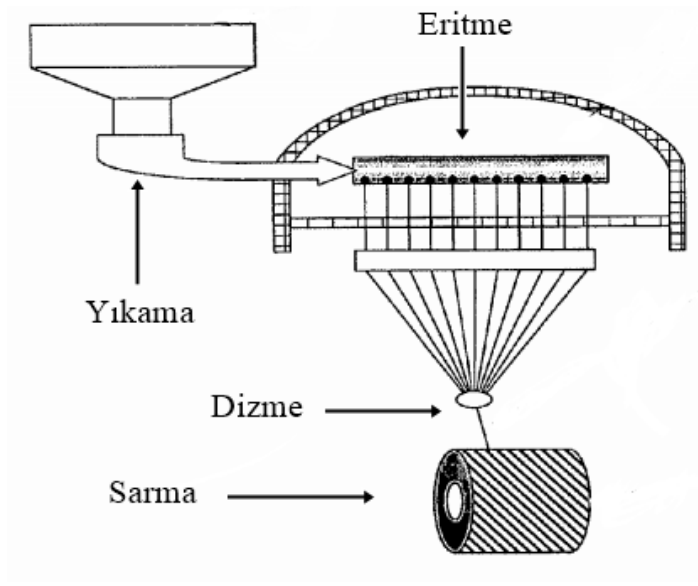
Şekil 3.1. Bazalt fiberin üretim şeması (Kamiya ve ark., 2013).
