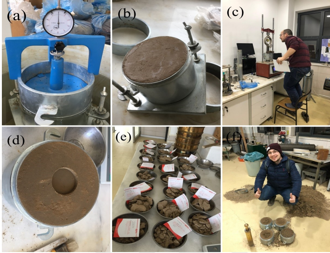
Şekil 4.23. Deney aşamaları, (a) Numunenin suda bekletilmesi, (b) Suda beklemiş numune, (c) Deneyin yapımı, (d) Deney sonrası numunenin görünümü, (e) Su muhtevası için alınmış örnekler, (f) Numune alınmış kalıplar.
