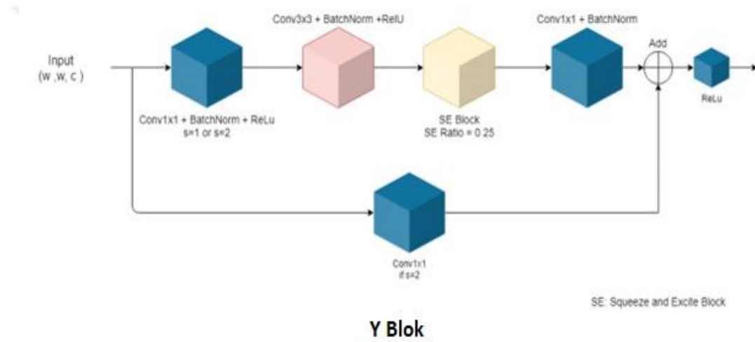
Şekil 3. 12. RegNetY mimarisi (Radosavovic vd., 2020)
