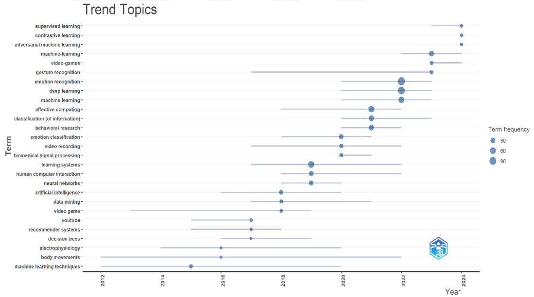
Şekil 2. 3. Yıllara göre trend topic anahtar kelimeler (frekans \geq 4 )
