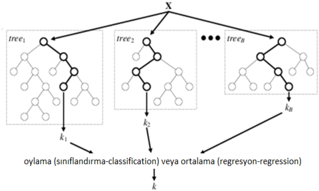
Şekil 3. 6. RF algoritması
