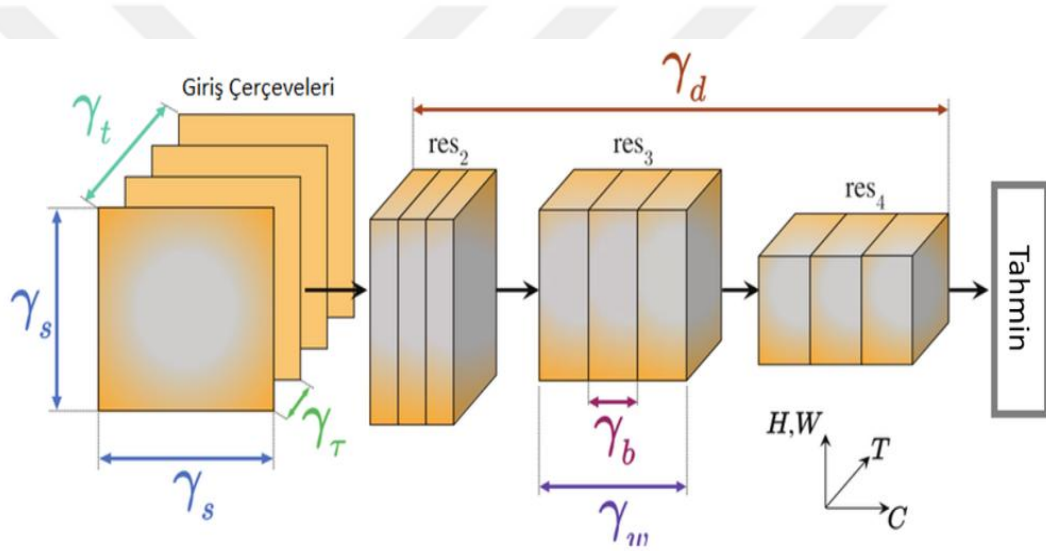
Şekil 3. 15. X3D-medium ağlarının çerçevesi (Feichtenhofer vd., 2020)
