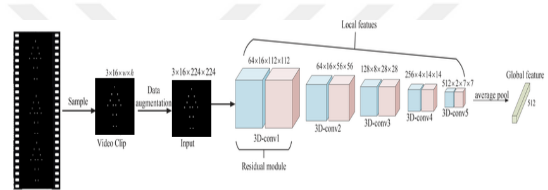
Şekil 3. 14. 3D-ResNet-18 ağ mimarisi (Xue vd., 2020)
