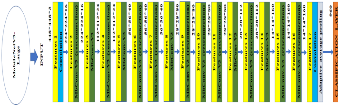
Şekil 3. 11. MobileNetV3 mimarisi
