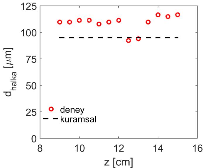
Şekil 3.10. Bessel-Vortex hüzmeleri spot çapı-uzaklık grafiği (kuramsal olarak hesaplanan çap değeri yaklaşık 95 μm, deneysel olarak elde edilen ortalama çap değeri 108 μm' dir)
