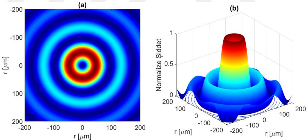
Şekil 1.6. Kuramsal olarak hesaplanan (a) 2 ve (b) 3 boyutlu Bessel-Vortex hüzmesi elektrik Alan profilleri. Hesaplamalarda dalga boyu 633 nm, Konik Mercek Taban açısı 0.5^\circ alınmıştır
