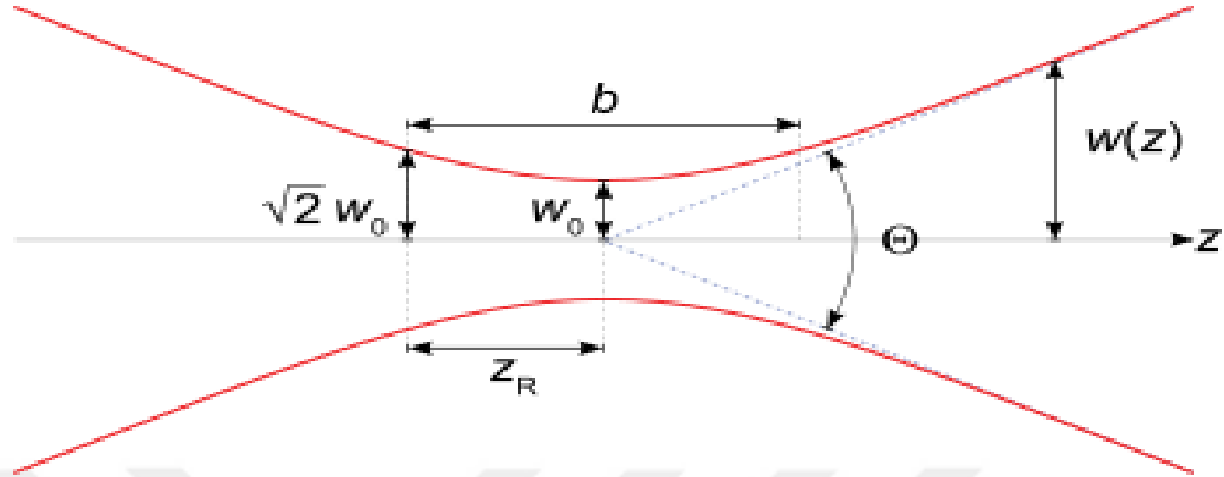
Şekil 1.3. Gauss hüzmeleri şeması (Anonim 1)
