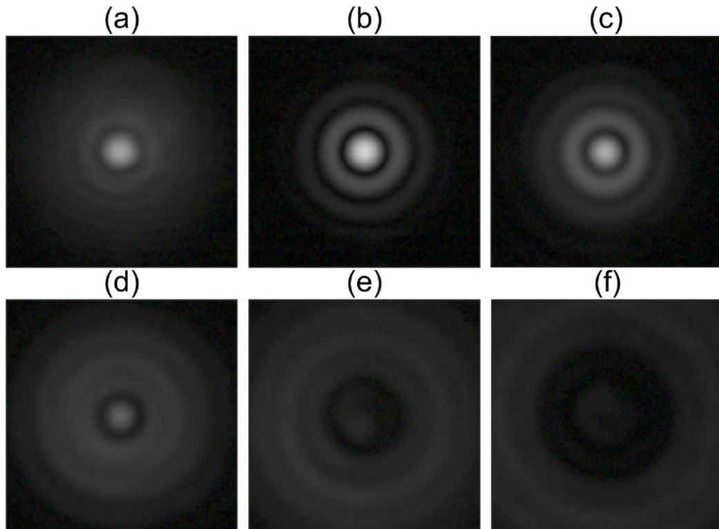
Şekil 3.5. CCD kamera ile kaydedilen kamera ile Axicon arasındaki uzaklığa göre a) 5 cm b) 10 cm c) 15 cm d) 20 cm e) 25 cm f) 30 cm Bessel hüzmesi şiddet profilleri
