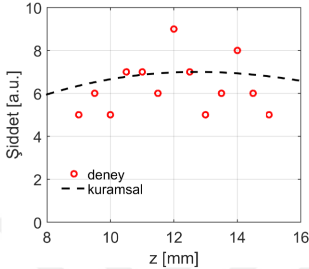
Şekil 3.9. Bessel-vortex hüzmeleri şiddet-uzaklık grafiği
