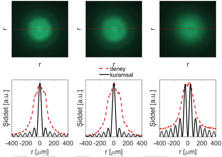
Şekil 3.15. Yeşil LED ile yapılan Bessel ve Bessel-Vortex hüzme şekillendirme çalışmaları (Bessel hüzmeleri farklı iki uzaklıkta elde edilmiştir ve renkli CCD kamera kullanılmıştır)
