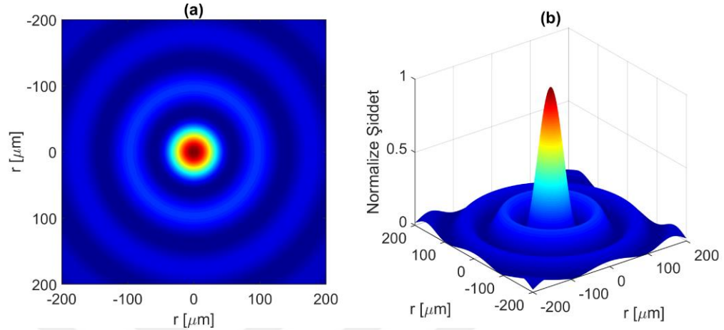
Şekil 1.5. Kuramsal olarak hesaplanan (a) 2 ve (b) 3 boyutlu Bessel hüzmesi elektrik Alan profilleri. Hesaplamalarda dalga boyu 633 nm, Konik Mercek Taban açısı 0.5^\circ alınmıştır
