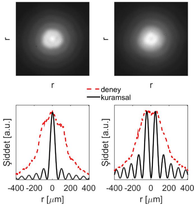
Şekil 3.16. Kırmızı LED ile yapılan Bessel ve Bessel-Vortex hüzme şekillendirme çalışmaları (siyah-beyaz CCD kamera kullanılmıştır)
