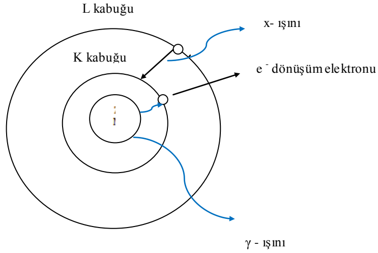
Şekil 4: İç dönüşüm olayı. Nükleer uyarılma enerjisi, yayınlanan K kabuğu elektronuna aktarılır ve boşluk L kabuğundan gelen bir elektronun geçişi ile doldurulur. K kabuğu ve L kabuğu arasındaki enerji farkı karakteristik K_x ışını olarak ortaya çıkar. 8
