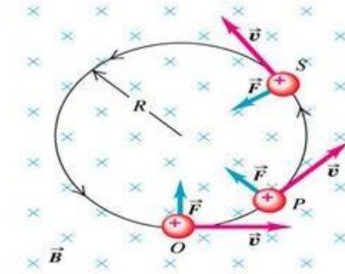
Şekil 8: Düzgün manyetik alan içerisindeki yüklü bir parçacığın hareketi (13)
