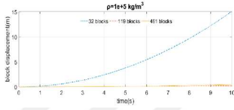
f) p=1e+5 \text{ kg/m}^3
