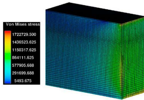
d) t=2s (Von Mises stress)
