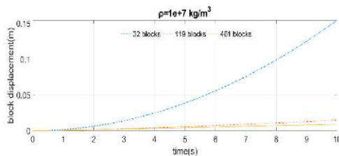
a) p=1e+7 \text{ kg/m}^3
