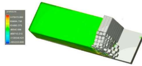
f) t\sim 12s (semi-gradual failure)
