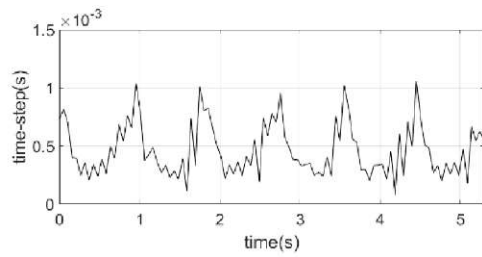
b) 2mm grid size
