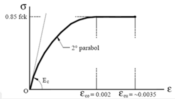
Şekil 3.6. Betonarme çubuğun eğilmesinde dış basınç lifindeki \sigma - \varepsilon diyagramı (Özer 2006)
