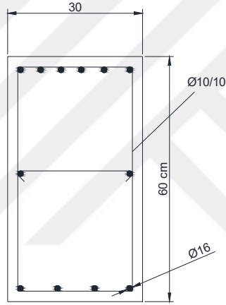
Şekil 3.18. 30/ 60 olan kirişin enine ve boyuna donatıları
