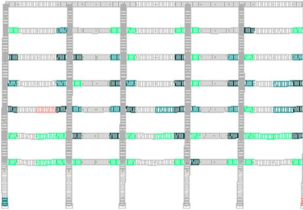
Şekil 4.44. 0.2g'ye göre ölçeklenen Kobe deprem kaydından elde edilen hasarlar
