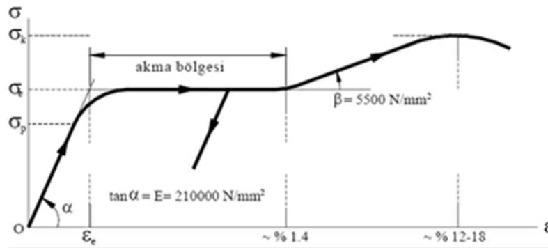
Şekil 3.3. Yapı çeliğinin gerilme-şekil değiştirme diyagramı
