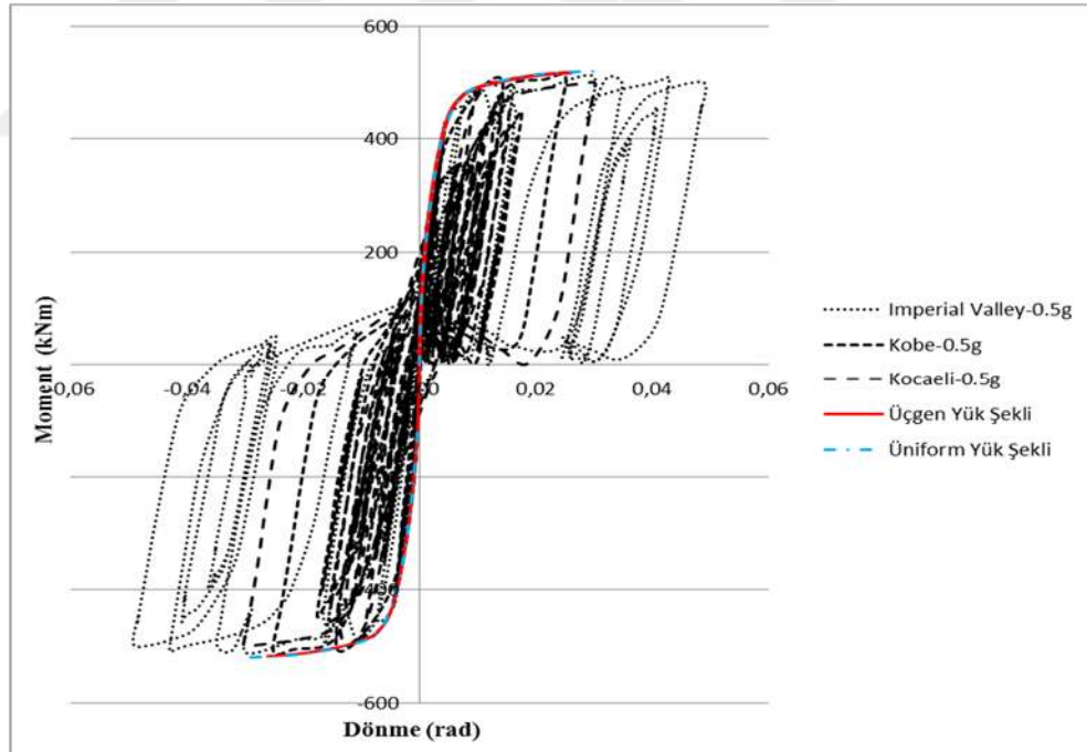
Şekil 4.12. Doğrusal olmayan statik ve 0.5g'lik dinamik yükler altında C111a kolonunun alt ucunda oluşan moment dönme eğrileri
