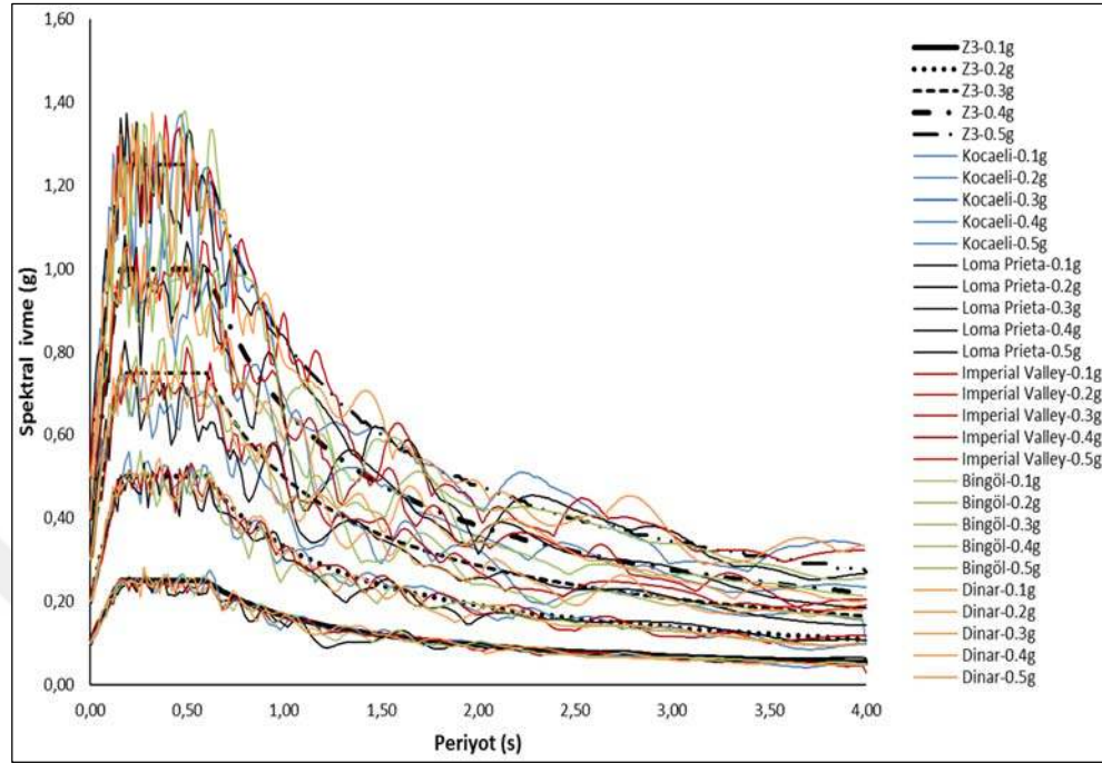
Şekil 3.19. Z3 zemin sınıfı ve farklı yer ivmeleri için tasarım spektrumuna göre ölçeklendirilmiş deprem ivme kayıtlarının tepki spektrumu
