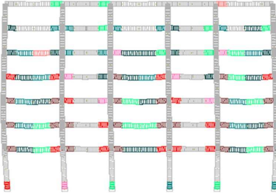
Şekil 4.41. 0.4 g'ye göre ölçeklenen Imperial Valley deprem kaydından elde edilen hasarlar
