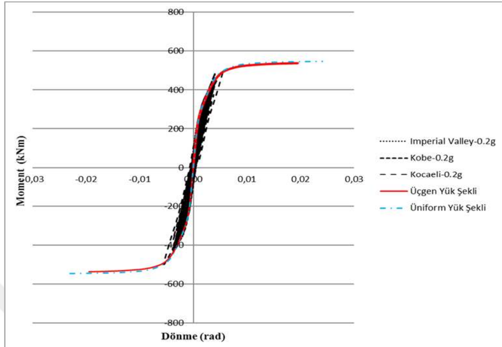
Şekil 4.19. Doğrusal olmayan statik ve 0.2g'lik dinamik yükler altında C31 la kolonunun alt ucunda oluşan moment dönme eğrileri
