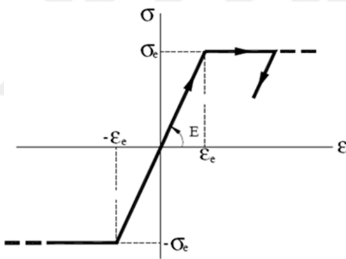
Şekil 3.5. Çeliğin ideal elasto-plastik malzeme davranış modeli
