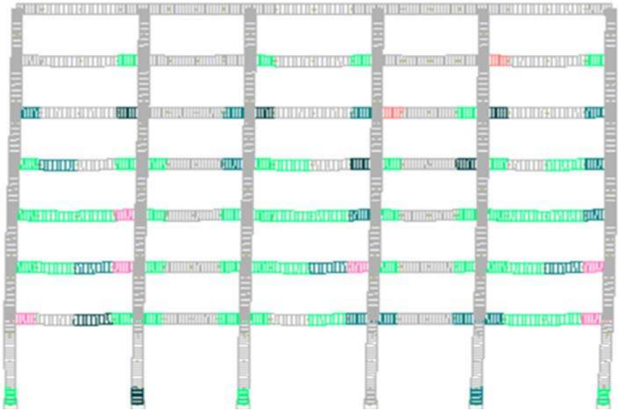
Şekil 4.49. 0.2g'ye göre ölçeklenen Kocaeli deprem kaydından elde edilen hasarlar
