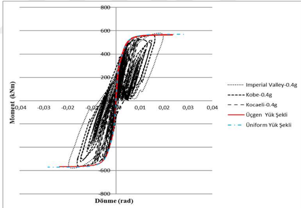
Şekil 4.16. Doğrusal olmayan statik ve 0.4g'lik dinamik yükler altında C211a kolonunun alt ucunda oluşan moment dönme eğrileri
