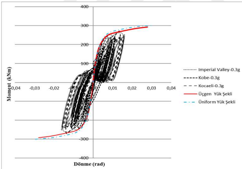
Şekil 4.30. Doğrusal olmayan statik ve 0.3g'lık dinamik yükler altında B212a kirişin sol ucunda oluşan moment dönme eğrileri
