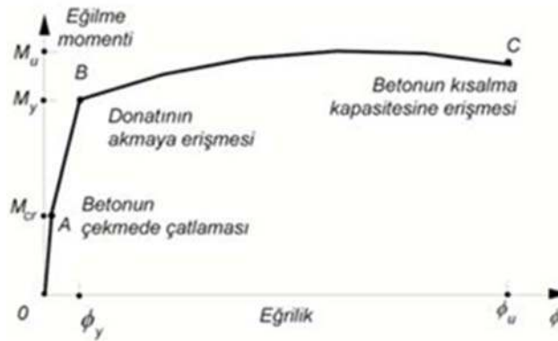
Şekil 3.7. Moment- eğrilik ilişkisi (Celep 2008)
