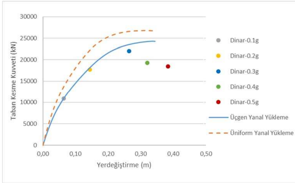
Şekil 4.60. Y yönü için Dinar deprem kayıtlarından elde edilen maksimum deplasmana karşılık gelen taban kesme kuvveti
