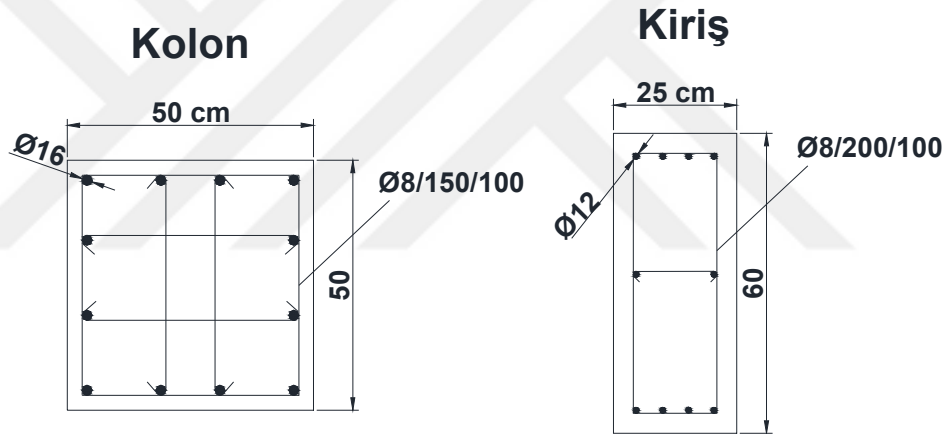
Şekil 3.13. Binanın düzlemsel görünüşü ve yapısal eleman detayları
