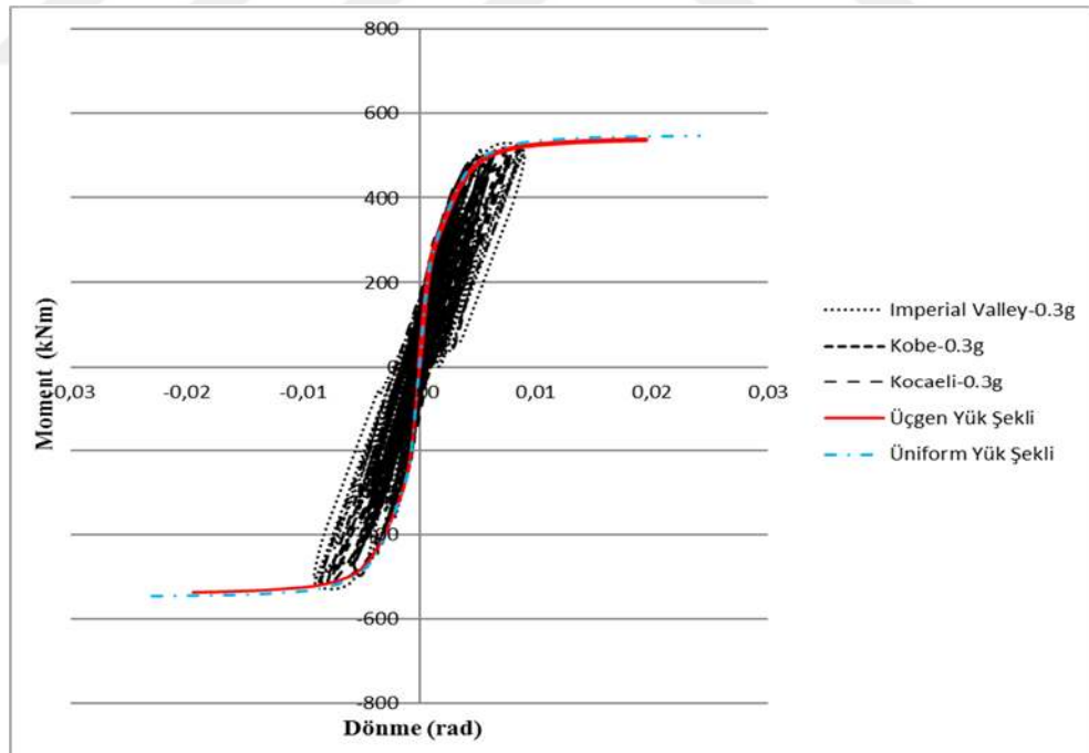
Şekil 4.20. Doğrusal olmayan statik ve 0.3g'lik dinamik yükler altında C31 la kolonunun alt ucunda oluşan moment dönme eğrileri
