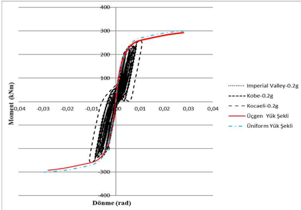
Şekil 4.29. Doğrusal olmayan statik ve 0.2g'lık dinamik yükler altında B212a kirişin sol ucunda oluşan moment dönme eğrileri
