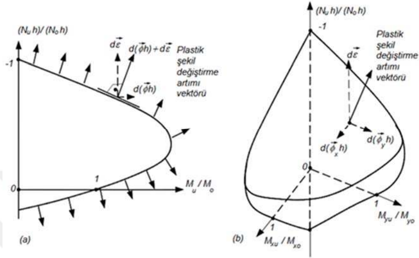
Şekil 3.9. Betonarme kesitlerde karşılıklı etki diyagramı (akma eğrisi) ve plastik şekil değiştirmeler (Celep 2008)
