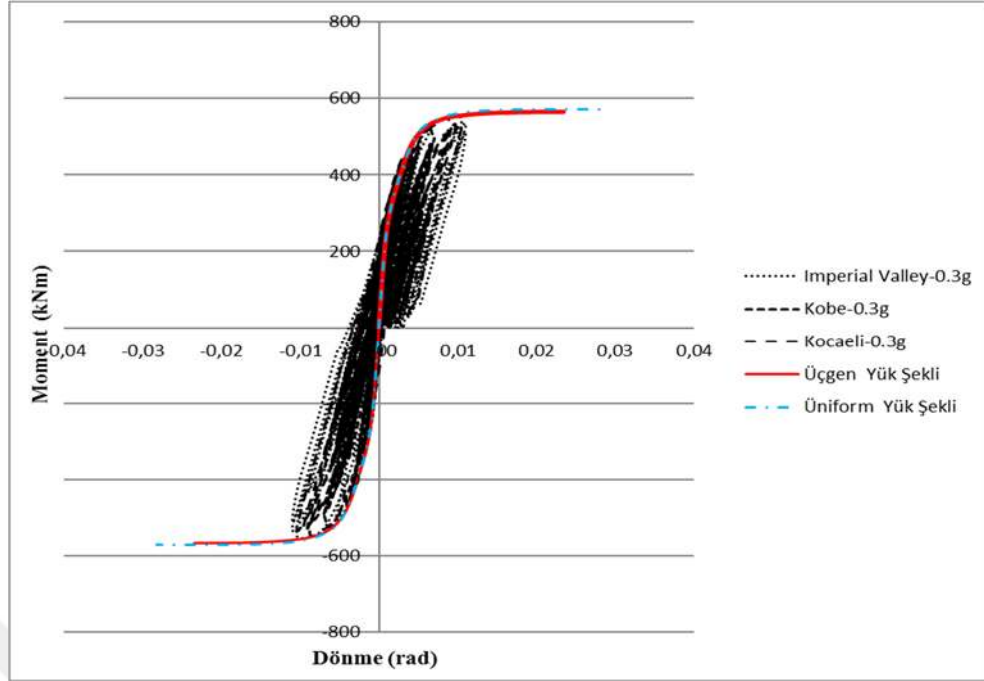
Şekil 4.15. Doğrusal olmayan statik ve 0.3g'lik dinamik yükler altında C211a kolonunun alt ucunda oluşan moment dönme eğrileri
