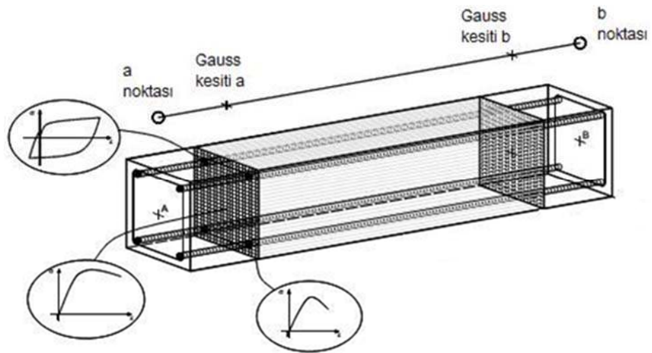
Şekil 3.10. Betonarme bir kirişin fiber elemanlara ayrılması ve malzeme davranışları (Seismostruct’den adapte edilmiştir)
