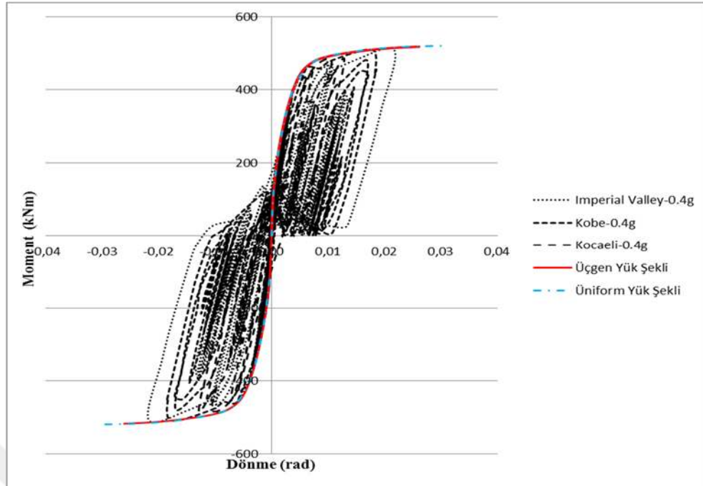
Şekil 4.11. Doğrusal olmayan statik ve 0.4g'lik dinamik yükler altında C111a kolonunun alt ucunda oluşan moment dönme eğrileri
