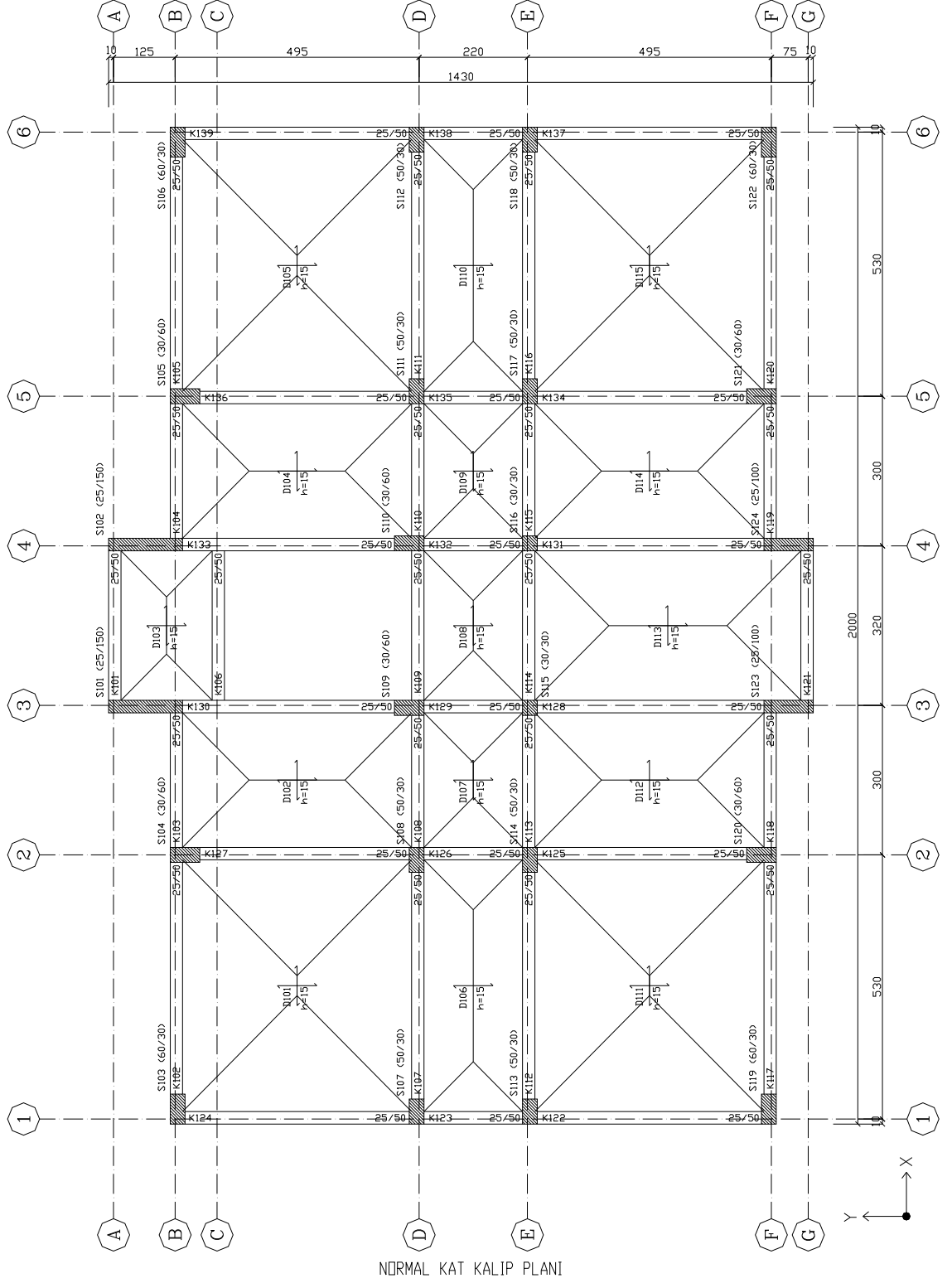
Ek-2: Örnek Binaın Kalıp Planları ve Donatı Detayları
