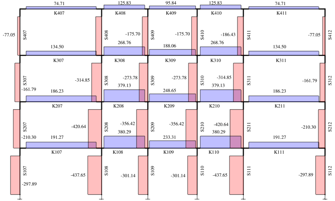
Şekil 4.14. +X yönü deprem yüklemesinden dolayı D-D aksında elde edilen kesme kuvveti ( V_E ) diyagramı (Probina)
