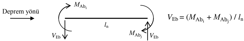
Şekil 4.22. Kirişlerde artık moment kapasitelerini dengeleyen kesme kuvvetleri
