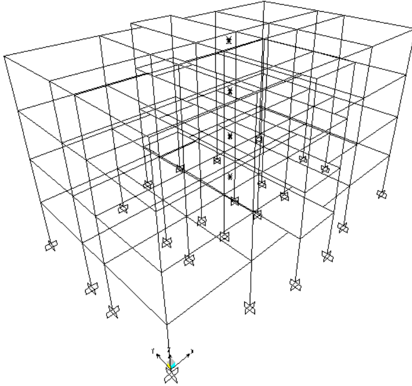
Şekil 4.3. Yapının üç boyutlu bilgisayar modeli (SAP2000)
