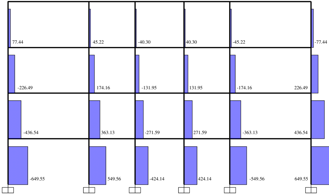
Şekil 4.13. +X yönü deprem yüklemesinden dolayı D-D aksında elde edilen eksenel kuvveti ( N_E ) diyagramı (SAP2000)
