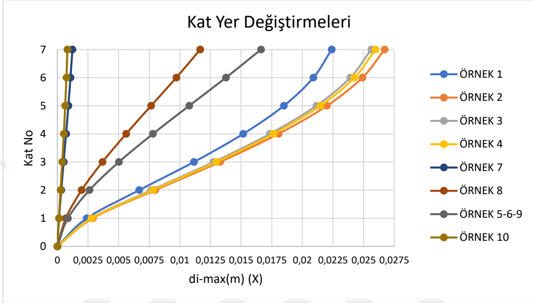
řekil 28. X Doğrultusundaki Maksimum Kat Yer Deęiřtirmeleri
