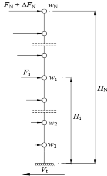
Şekil 12. Kat Seviyelerine Etkiyen Deprem Yükleri
