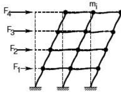
Şekil 2. Yatay Yük Altında Çerçevenin Deformasyonu
