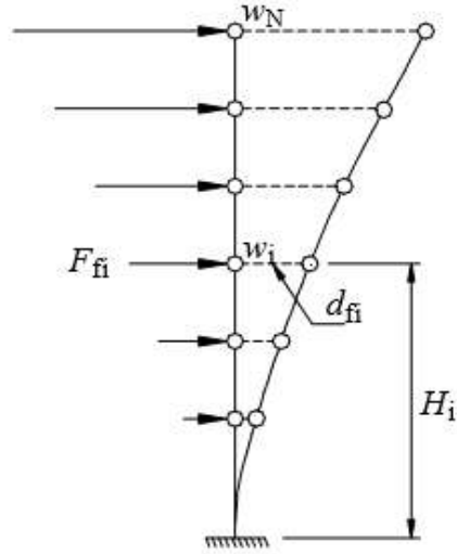
Şekil 9. Fiktif Yükler ve Yer Değiştirmeler
