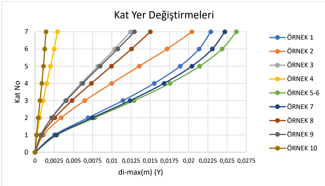
řekil 29. Y Doğrultusundaki Maksimum Kat Yer Deęiřtirmeleri
