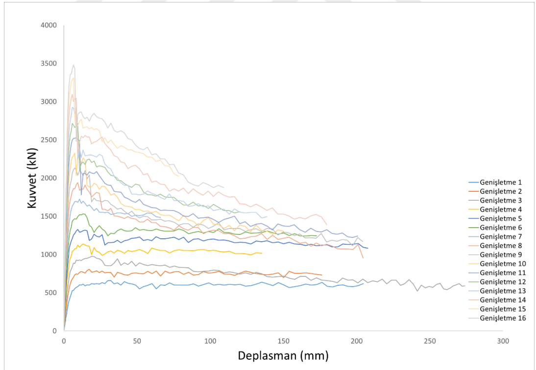
Şekil 5.50. Tüm genişletme modellerinin kuvvet deplasman grafikleri
