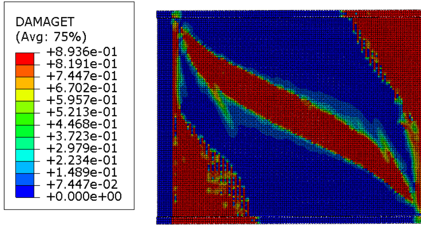
Şekil 5.71. Genişletme 11 modeli beton çekme hasarı
