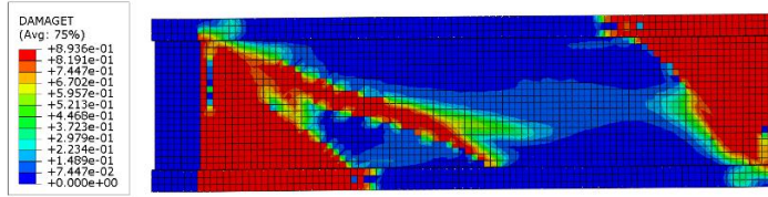
Şekil 5.41. Kısaltma 7 modeli beton çekme hasarı
