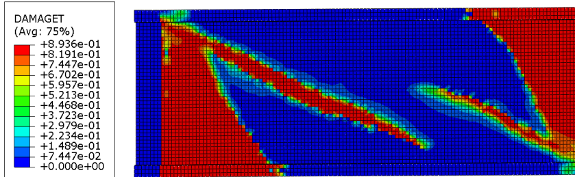
Şekil 5.63. Genişletme 3 modeli beton çekme hasarı
