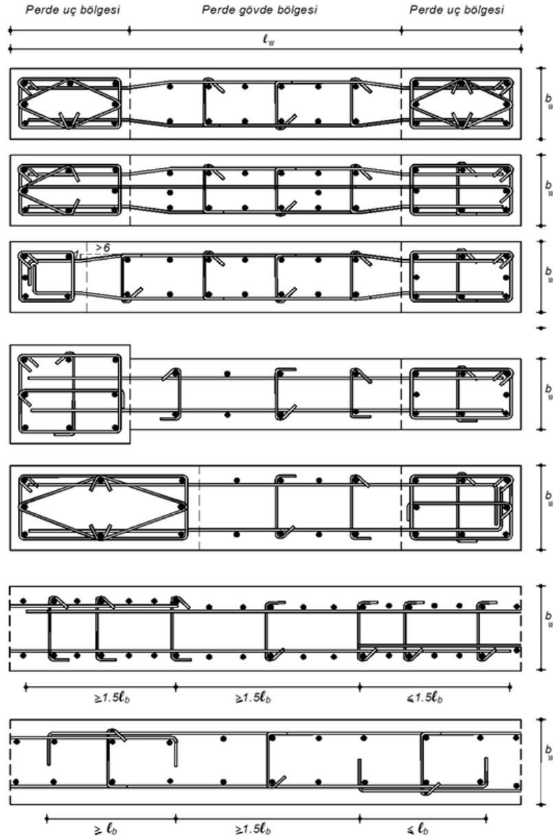
Şekil 3.9. TBDY 2018'e göre uygulanabilecek örnek perde donatı düzenleri
