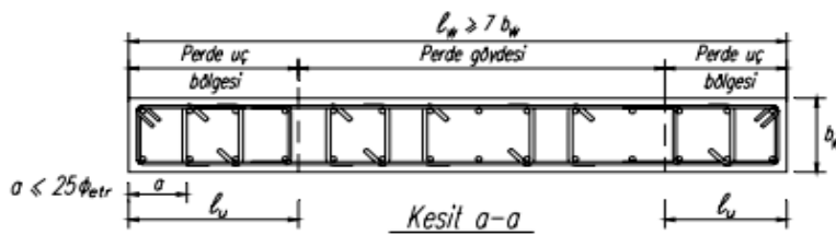
Şekil 3.11. TDY 2007 donatı düzeni
