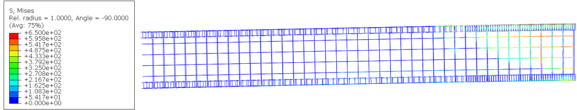
Şekil 5.11. Donatı düzeni-2'ye ait modelde donatılar için Von Mises gerilme dağılımı
