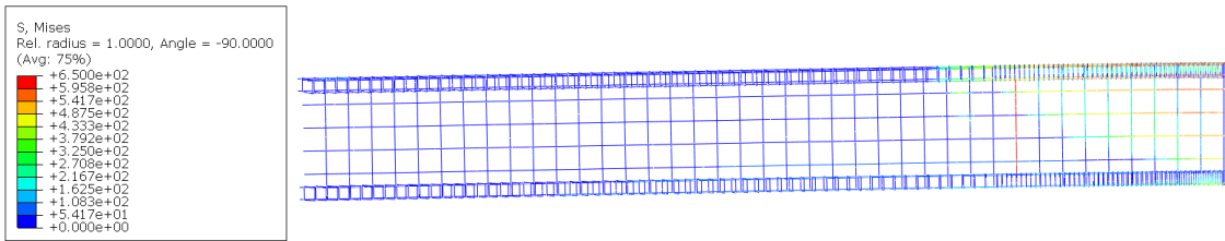
Şekil 5.8. Deneysel duruma ait modelde donatılar için Von Mises gerilme dağılımı
