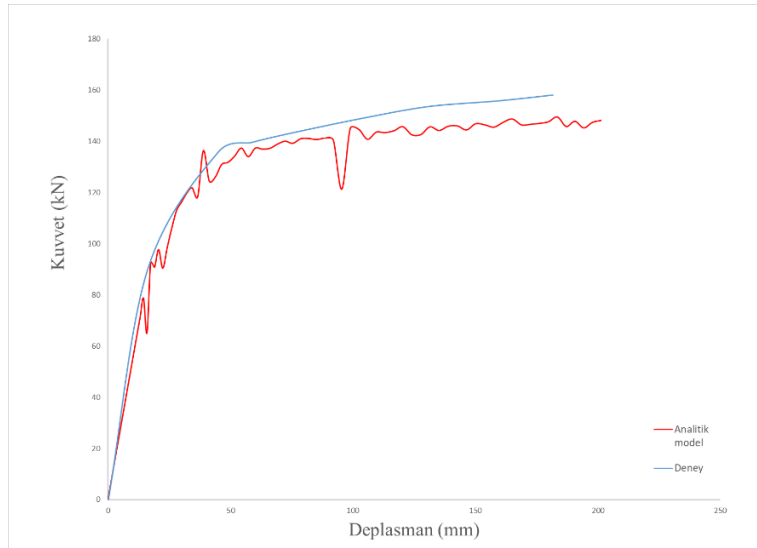
Şekil 5.5. Yük-deplasman eğrilerinin karşılaştırılması
