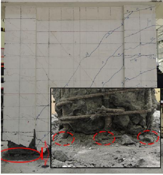
Şekil 3.6. Beton ezilmesi örneği (Yang vd. 2017)
