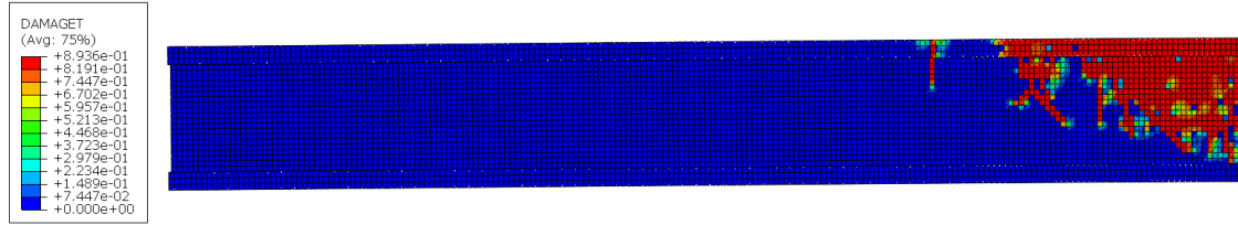
Şekil 5.7. Deneysel duruma ait model için beton çekme hasar dağılımı
