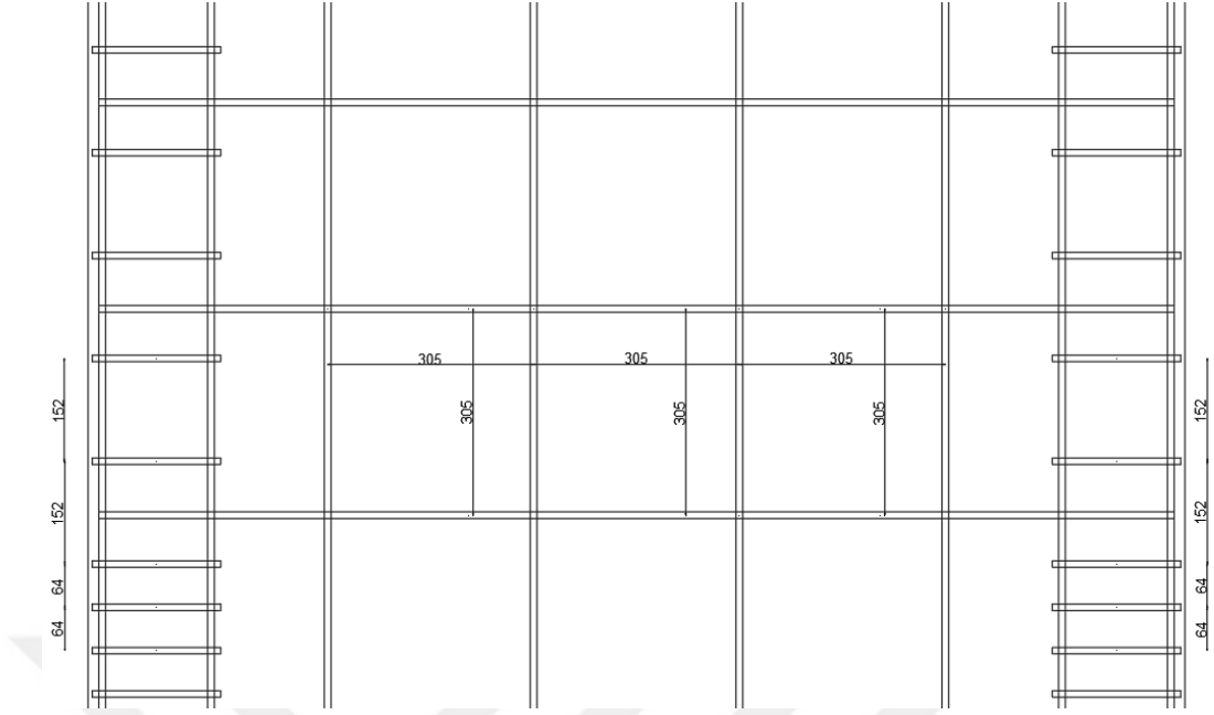
Şekil 4.24. Deney modelindeki perdenin yatay donatı şeması
