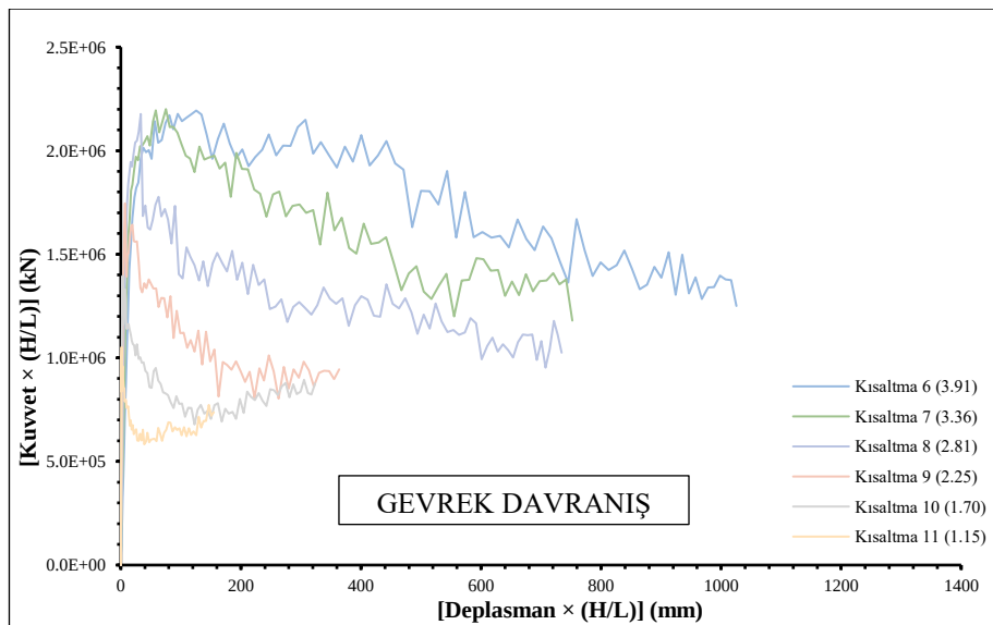
Şekil 5.78. Kısaltma 6-11 modelleri için [Kuvvet \times (H/L)] – [Deplasman \times (H/L)]
