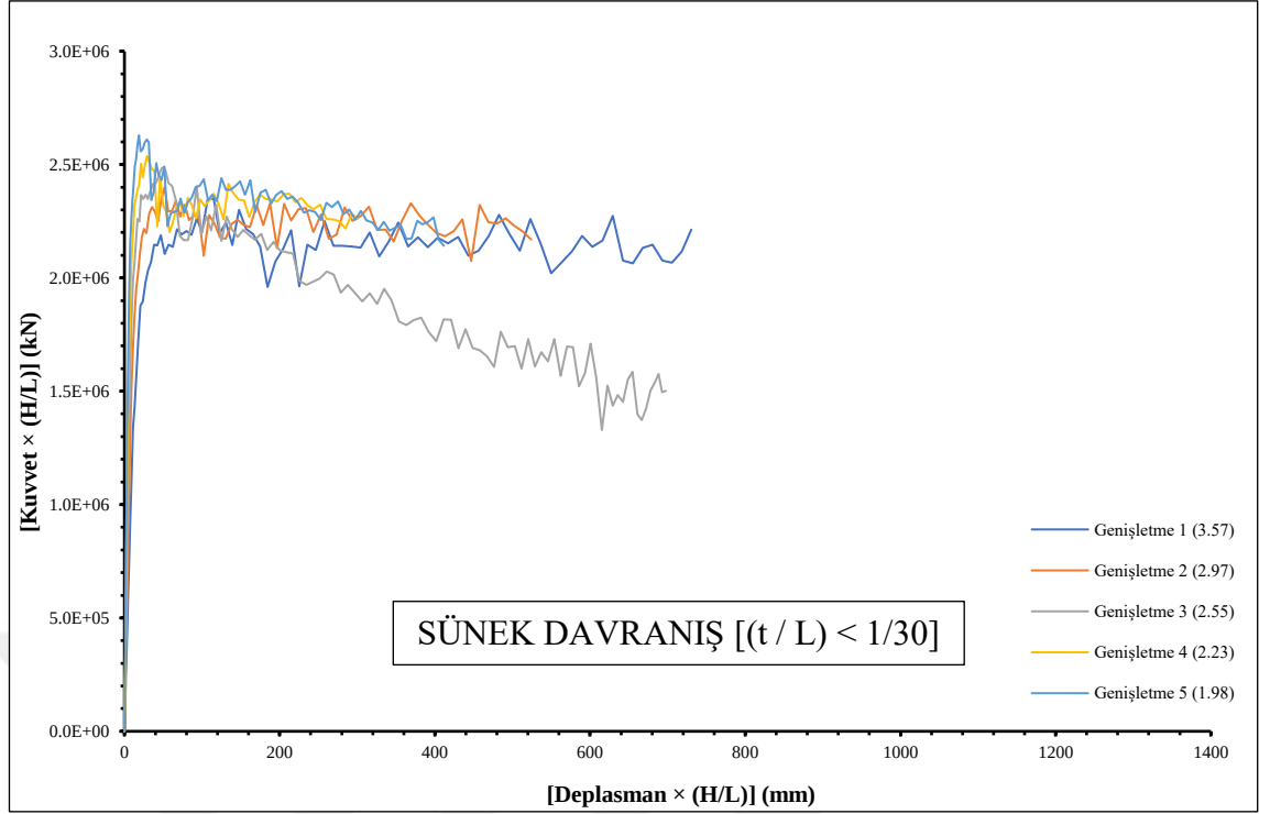
Şekil 5.79. Genişletme 1-5 modelleri için [Kuvvet \times (H/L)] - [Deplasman \times (H/L)]
