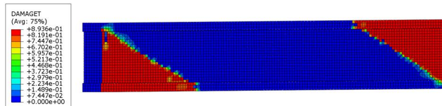
Şekil 5.38. Kısaltma 4 modeli beton çekme hasarı
