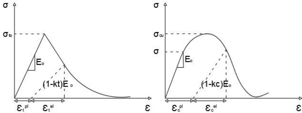
Şekil 3.14. Tek eksenli yük altındaki betonun davranışı a) çekme; b) basınç (Kaya 2023)
