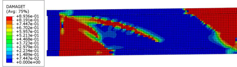
Şekil 5.40. Kısaltma 6 modeli beton çekme hasarı
