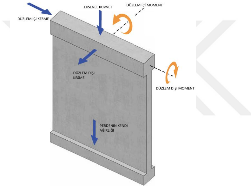
Şekil 3.1. Perdeye etkiyen temel kuvvetler (ACI 318-9)
