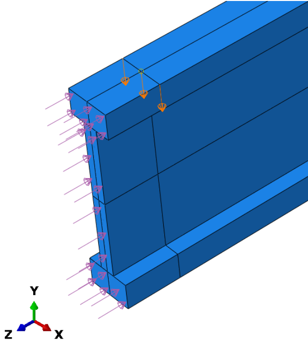
Şekil 4.16. Yatay ve düşey yükleme durumları
