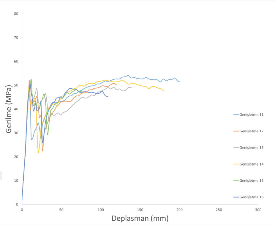
Şekil 5.59. Genişletme 11-14 ve Genişletme 16 modellerinin basınç-deplasman grafikleri
