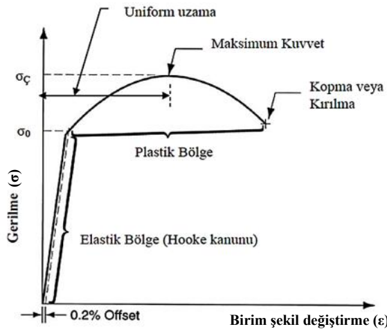
Şekil 3.13. Gerilme birim şekil değiştirme diyagramı (Kaya 2023)
