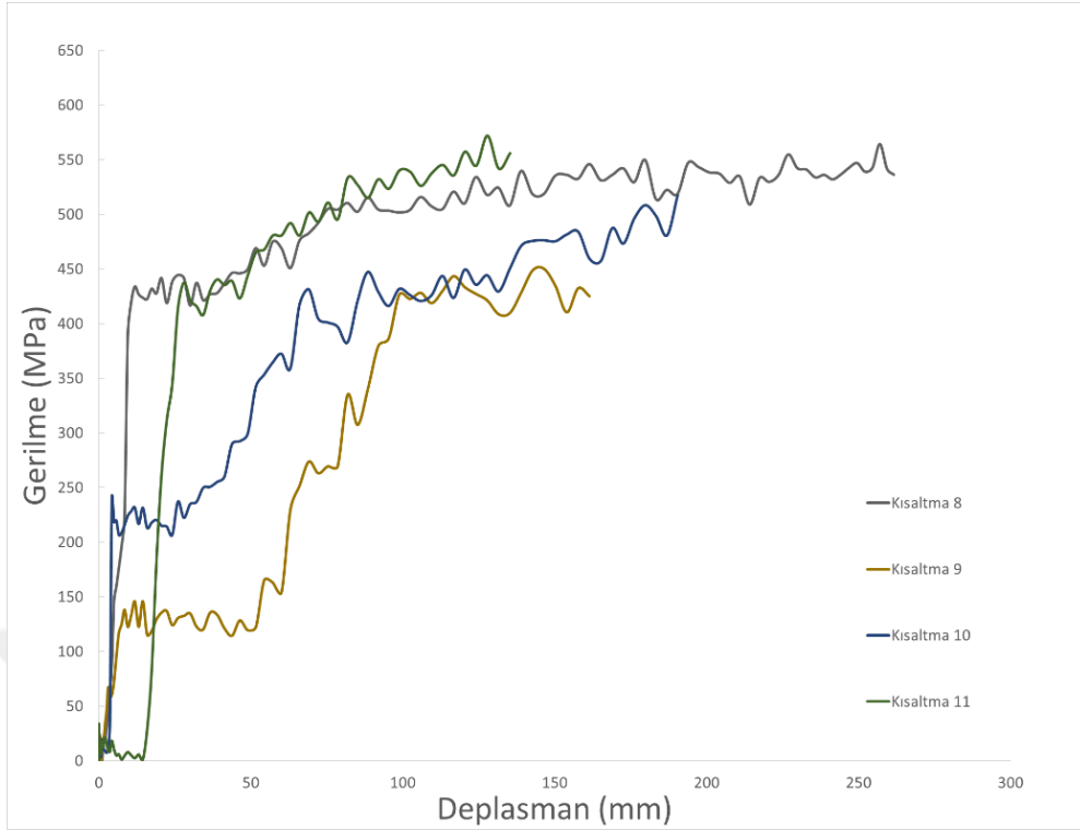
Şekil 5.28. Kısaltma 8-11 modellerinin çekme gerilmesi-deplasman grafikleri
