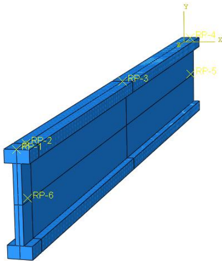
Şekil 4.10. Referans noktalarının oluşturulması
