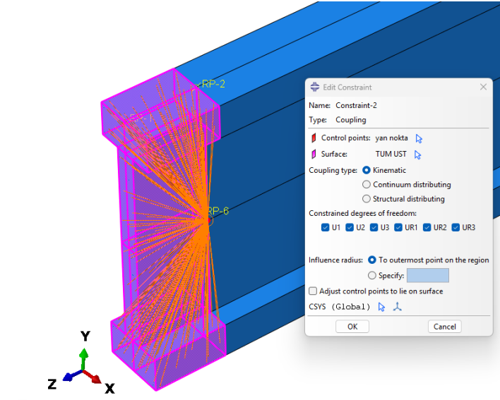
Şekil 4.18. Kısıtlama “Constraint” uygulanması
