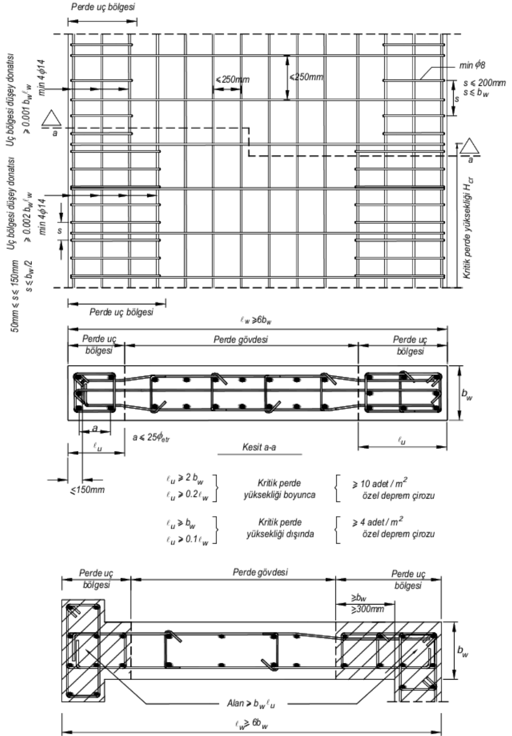
Şekil 3.8. TBODY 2018'e göre perde donatı düzeni
