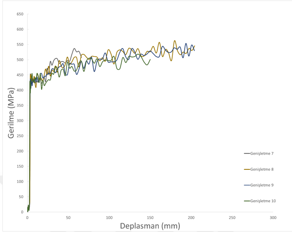
Şekil 5.53. Genişletme 7-10 modellerinin çekme gerilmesi-deplasman grafikleri
