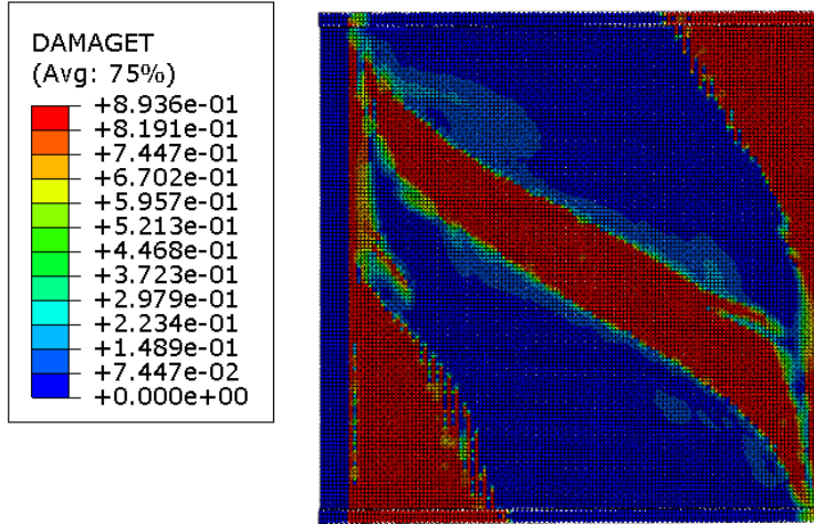
Şekil 5.74. Genişletme 14 modeli beton çekme hasarı
