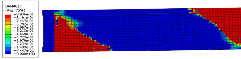
Şekil 5.39. Kısaltma 5 modeli beton çekme hasarı
