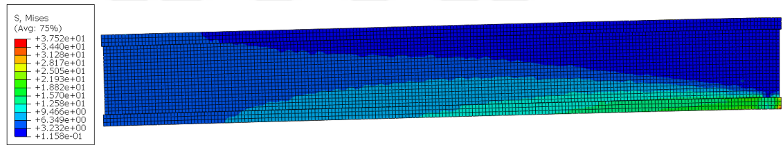
Şekil 5.18. Donatı düzeni-4 C25 modeli için Von Mises gerilme dağılımı
