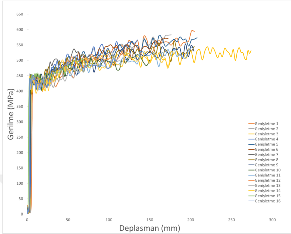
Şekil 5.55. Tüm genişletme modellerinin çekme gerilmesi-deplasman grafikleri
