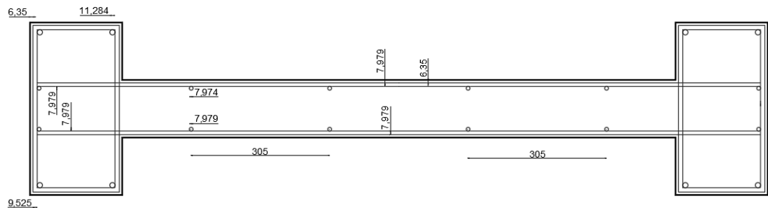
Şekil 4.21. Çift sıralı dışarıdan donatılı model (Donatı düzeni-2)
