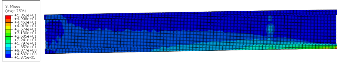
Şekil 5.6. Deneysel duruma ait model için Von Mises gerilme dağılımı
