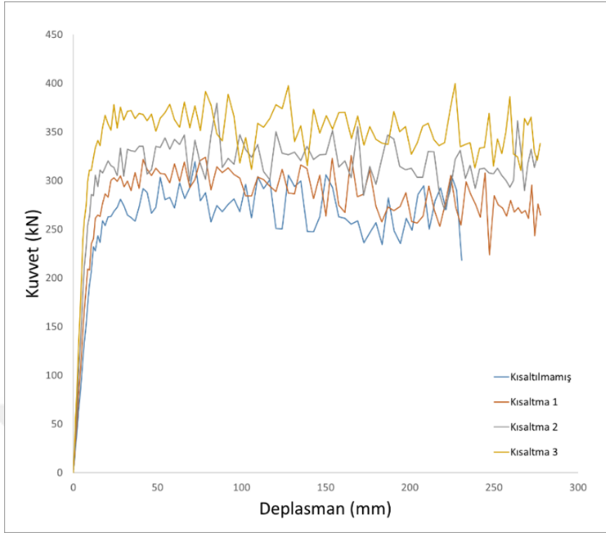
Şekil 5.22. Kısaltılmamış, Kısaltma 1-3 modellerinin kuvvet deplasman grafikleri
