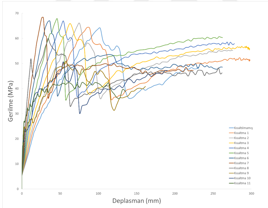
Şekil 5.33. Tüm modellerin basınç gerilmesi-deplasman grafikleri
