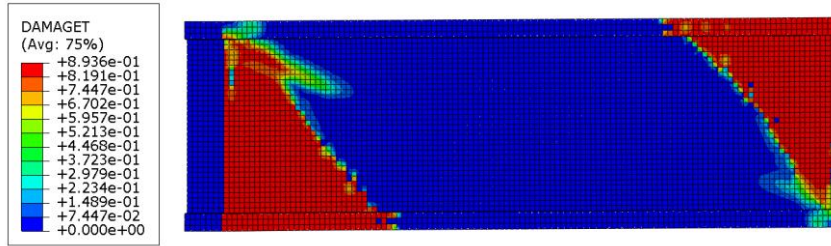
Şekil 5.62. Genişletme 2 modeli beton çekme hasarı
