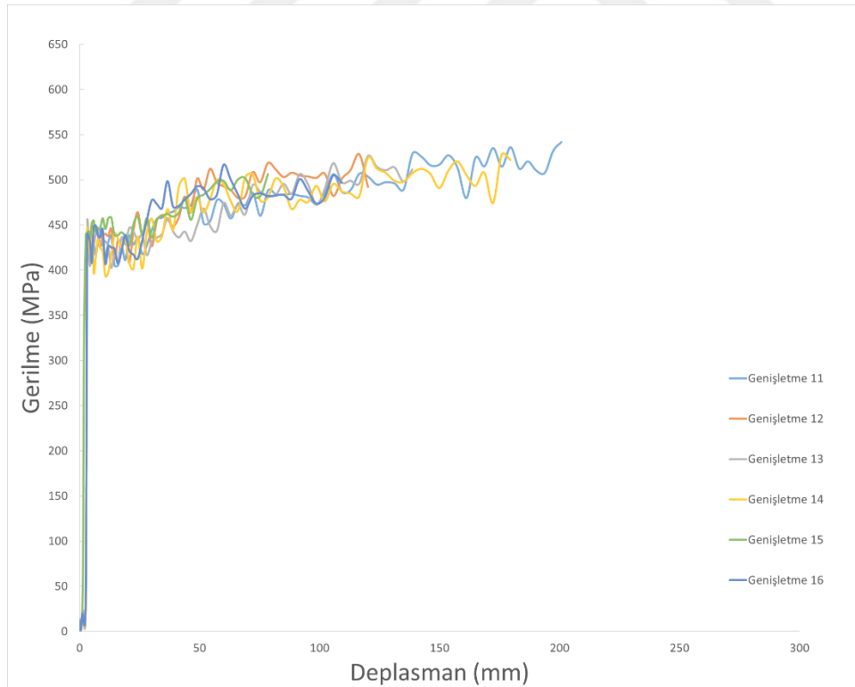
Şekil 5.54. Genişletme 11-16 modellerinin çekme gerilmesi-deplasman grafikleri
