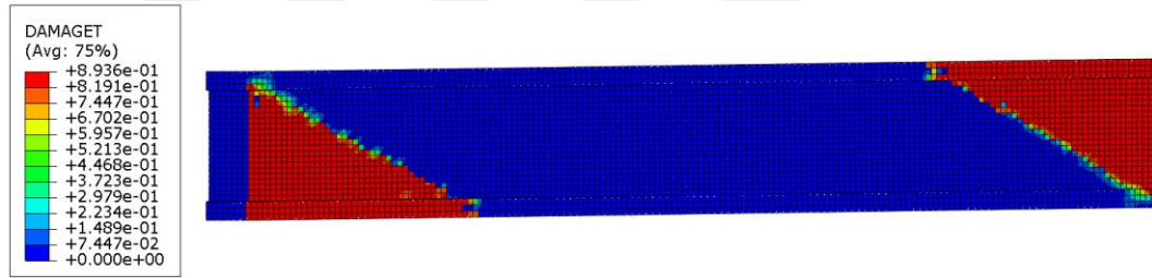
Şekil 5.36. Kısaltma 2 modeli beton çekme hasarı
