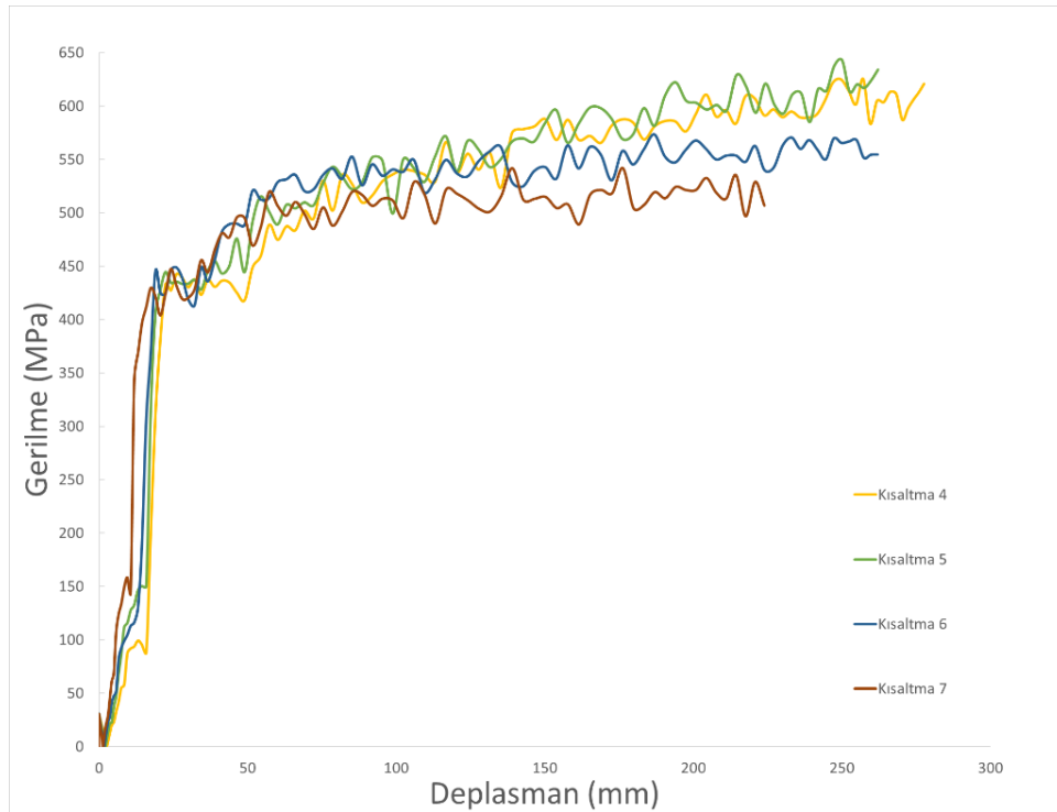
Şekil 5.27. Kısıltma 4-7 modellerinin çekme gerilmesi-deplasman grafikleri
