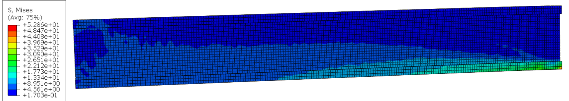
Şekil 5.15. Donatı düzeni-4'e ait model için Von Mises gerilme dağılımı
