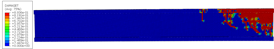
Şekil 5.10. Donatı düzeni-2'ye ait model için beton çekme hasar dağılımı
