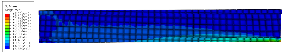
Şekil 5.12. Donatı düzeni-3'e ait model için Von Mises gerilme dağılımı
