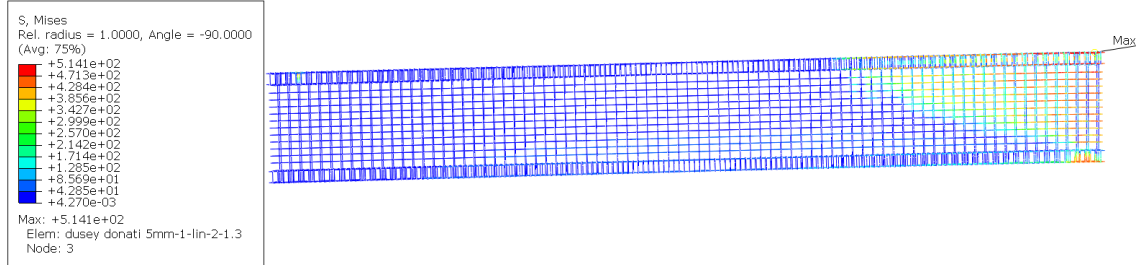
Şekil 5.17. Donatı düzeni-4’e ait modelde donatılar için Von Mises gerilme dağılımı
