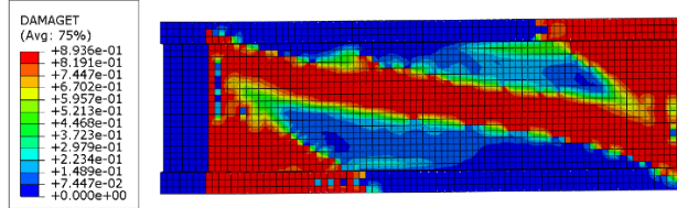
Şekil 5.42. Kısaltma 8 modeli beton çekme hasarı
