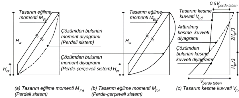
Şekil 3.10. Tasarım eğilme momenti ve tasarım kesme kuvveti diyagramları (TBDY)
