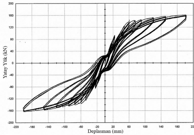
Şekil 5.3. Yük-deplasman eğrisi (İbrahim, 2000)
