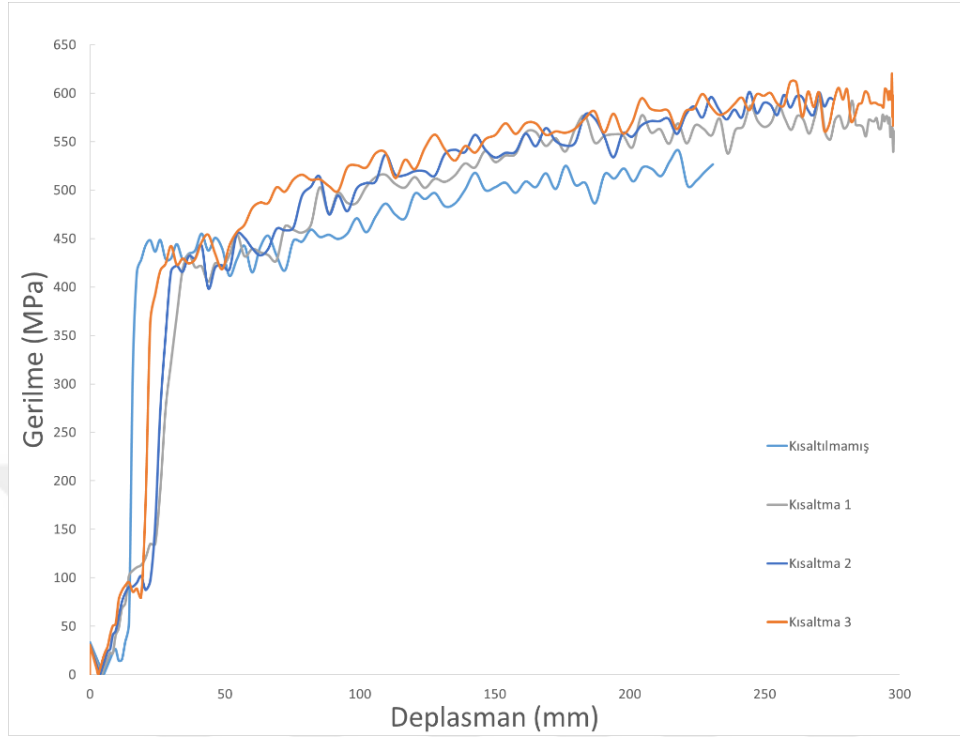
Şekil 5.26. Kısıtılmamış, Kısıltma 1-3 modellerinin çekme gerilmesi-deplasman grafikleri
