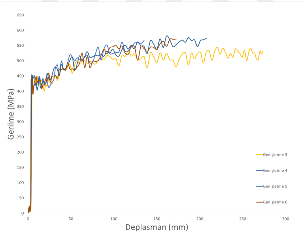
Şekil 5.52. Genişletme 3-6 modellerinin çekme gerilmesi-deplasman grafikleri
