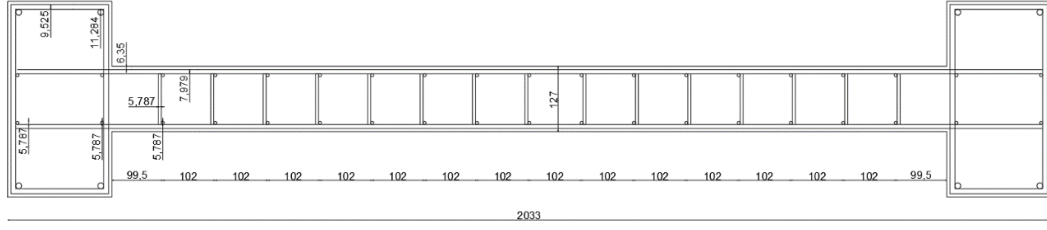
Şekil 4.27. Genişletme 1 modeli donatı düzeni
