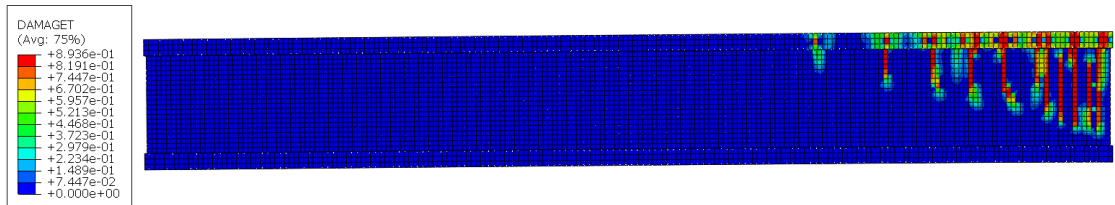
Şekil 5.19. Donatı düzeni-4 C25 modeli için beton çekme hasar dağılımı
