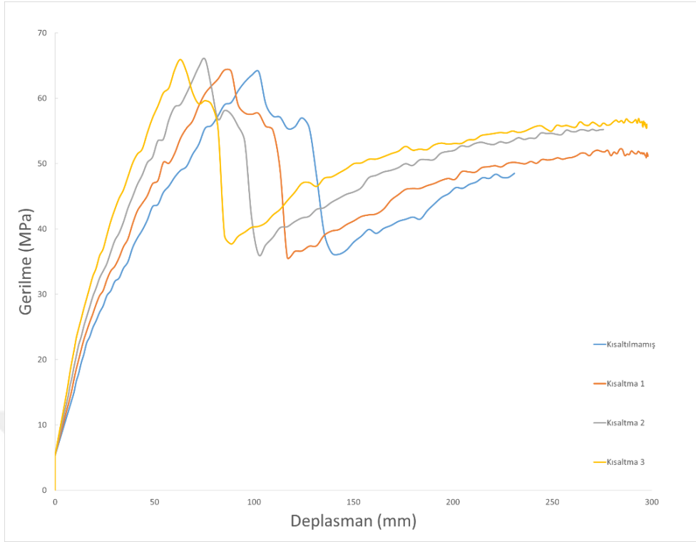
Şekil 5.30. Kısaltılmamış, Kısaltma 1-3 modellerinin basınç gerilmesi-deplasman grafikleri
