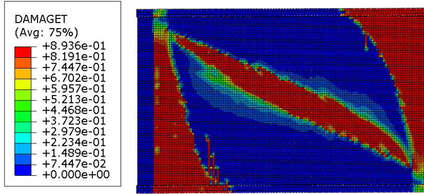
Şekil 5.68. Genişletme 8 modeli beton çekme hasarı
