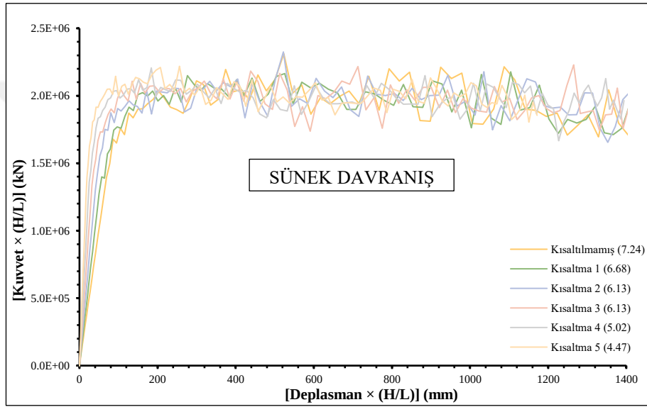
Şekil 5.77. Kısaltma 1-5 modelleri için [Kuvvet \times (H/L)] – [Deplasman \times (H/L)]
