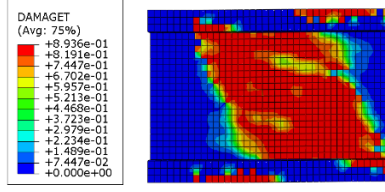
Şekil 5.45. Kısaltma 11 modeli beton çekme hasarı
