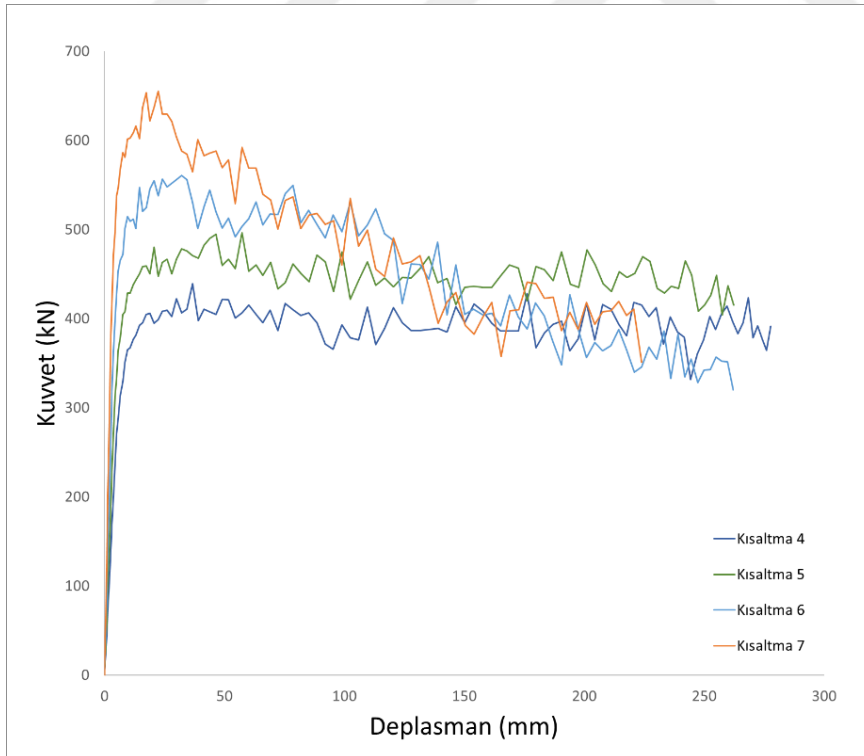
Şekil 5.23. Kısaltma 4-7 modellerinin kuvvet deplasman grafikleri
