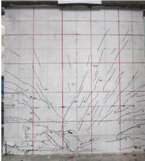
Şekil 3.7. Sünek kırılma örneği (Tong vd. 2019)
