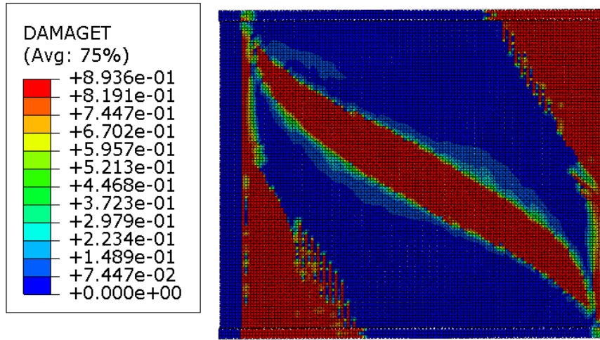
Şekil 5.72. Genişletme 12 modeli beton çekme hasarı
