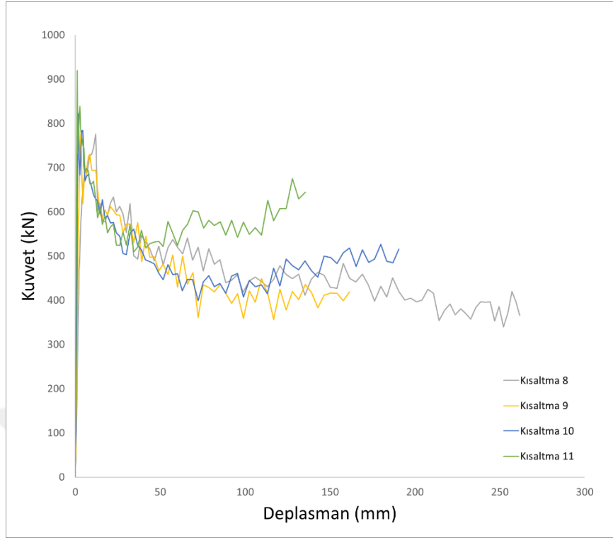
Şekil 5.24. Kısaltma 8-11 modellerinin kuvvet deplasman grafikleri
