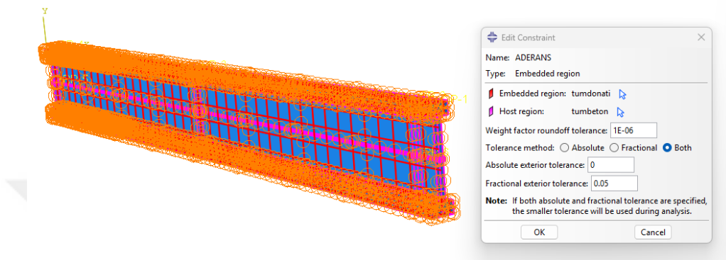
Şekil 4.11. Aderansın tanımlanması
