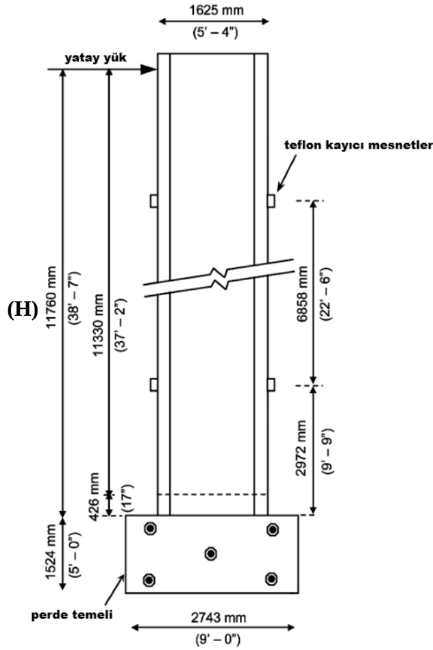
Şekil 4.4. Perde düşey kesiti (Adebar vd. 2007)
