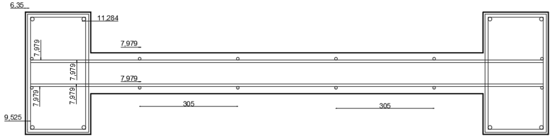
Şekil 4.22. Çift sıralı içeriden donatılı model (Donatı düzeni-3)
