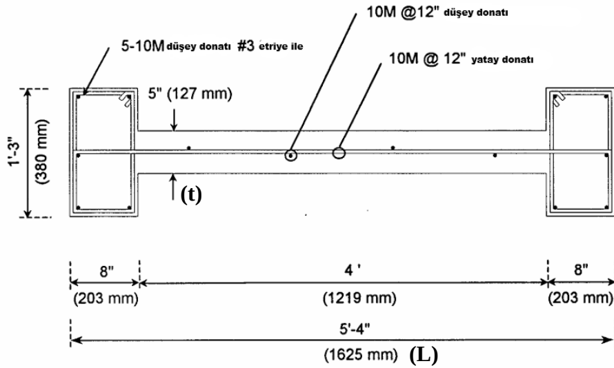
Şekil 4.3. Perde yatay kesiti
