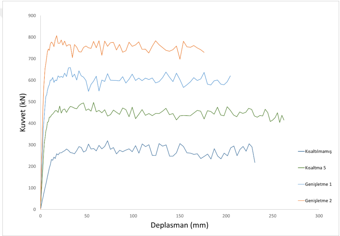
Şekil 5.46. Kısaltılmamış, Kısaltma 5, Genişletme 1 ve Genişletme 2 modellerinin kuvvet deplasman grafikleri
