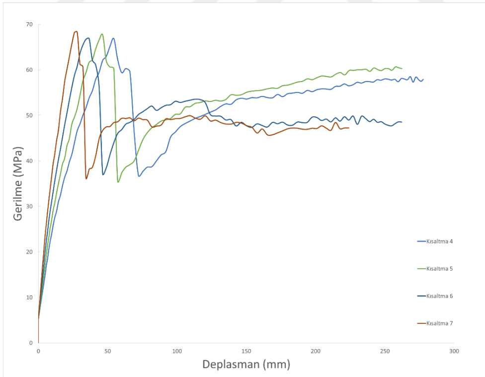
Şekil 5.31. Kısaltma 4-7 modellerinin basınç gerilmesi-deplasman grafikleri
