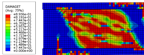
Şekil 5.44. Kısaltma 10 modeli beton çekme hasarı
