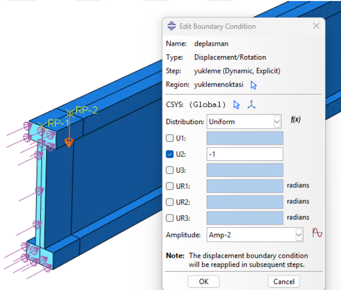
Şekil 4.12. Yüklemenin tanımlanması
