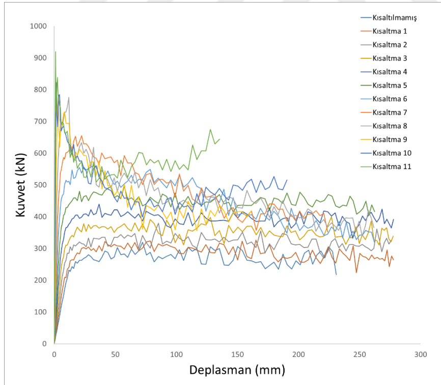
Şekil 5.25. Tüm modellerin kuvvet-deplasman grafikleri
