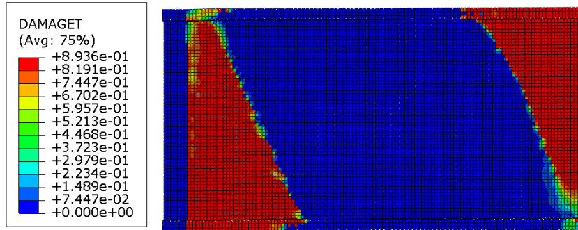
Şekil 5.65. Genişletme 5 modeli beton çekme hasarı
