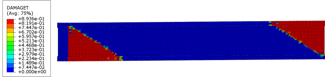
Şekil 5.35. Kısaltma 1 modeli beton çekme hasarı
