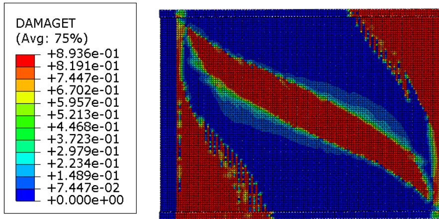
Şekil 5.70. Genişletme 10 modeli beton çekme hasarı
