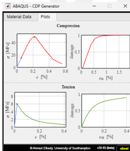
Şekil 4.8. ABAQUS CDP Generator (Elkady 2023)
