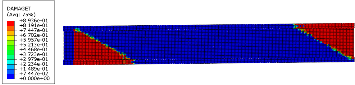
Şekil 5.34. Kısaltılmamış model beton çekme hasarı
