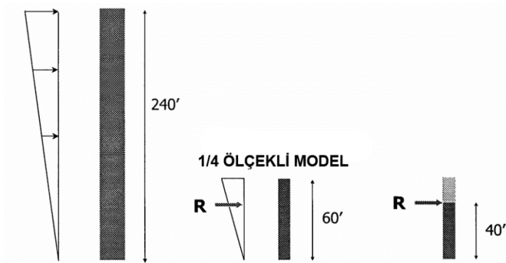
Şekil 4.2. Üretilen perde modeli ölçeği
