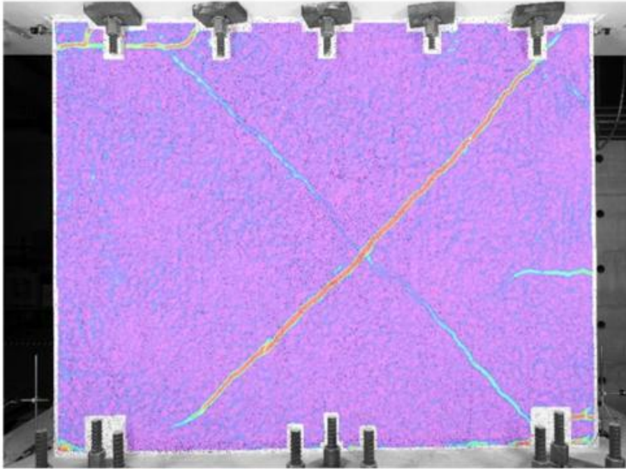
Şekil 3.3. Kesme kırılması örneği (Pohl vd. 2022)
