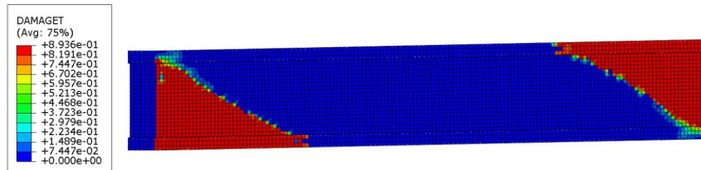
Şekil 5.37. Kısaltma 3 modeli beton çekme hasarı
