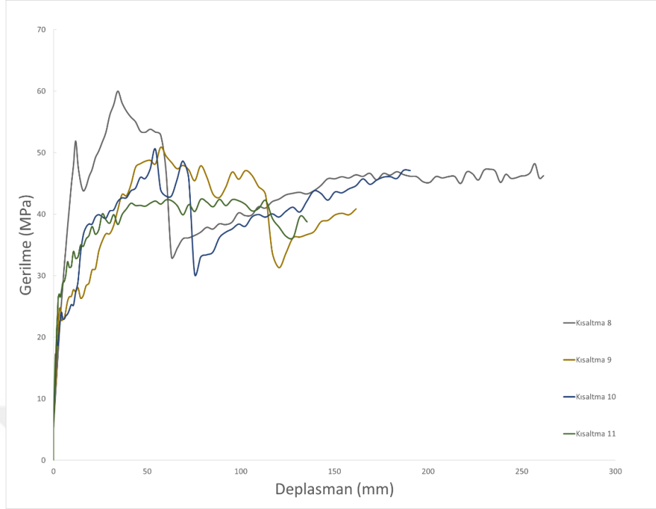
Şekil 5.32. Kısaltma 8-11 modellerinin basınç gerilmesi-deplasman grafikleri
