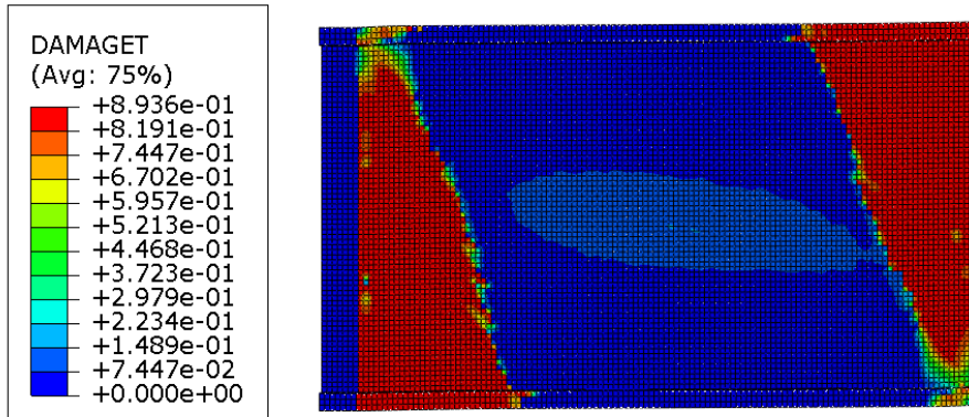
Şekil 5.67. Genişletme 7 modeli beton çekme hasarı
