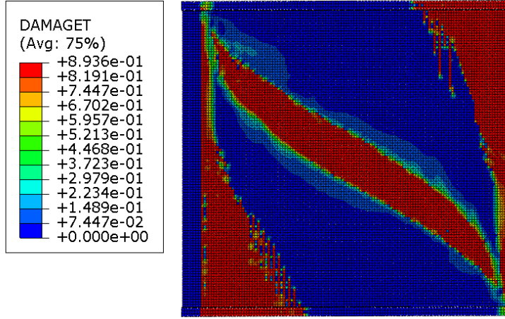
Şekil 5.74. Genişletme 14 modeli beton çekme hasarı
