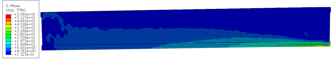
Şekil 5.9. Donatı düzeni-2'ye ait model için Von Mises gerilme dağılımı
