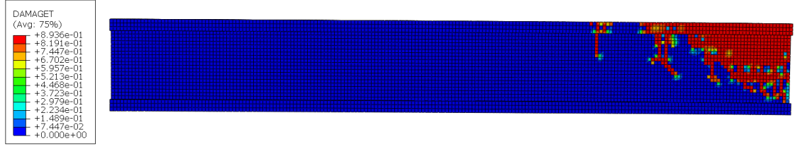
Şekil 5.13. Donatı düzeni-3'e ait model için beton çekme hasar dağılımı
