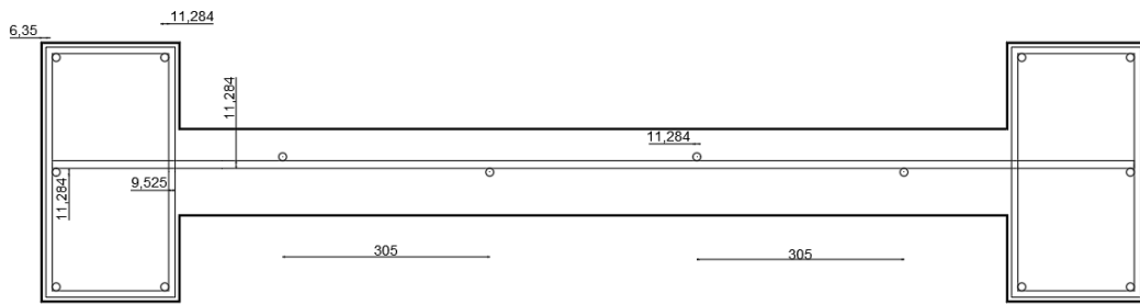
Şekil 4.20. Deneyde kullanılan perde modelinin donatı şeması (Donatı düzeni-1)
