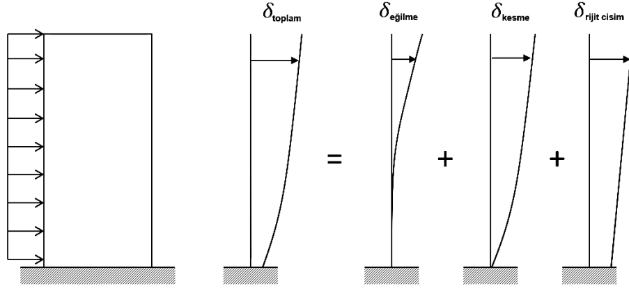
Şekil 3.2. Perde deformasyon şekilleri
