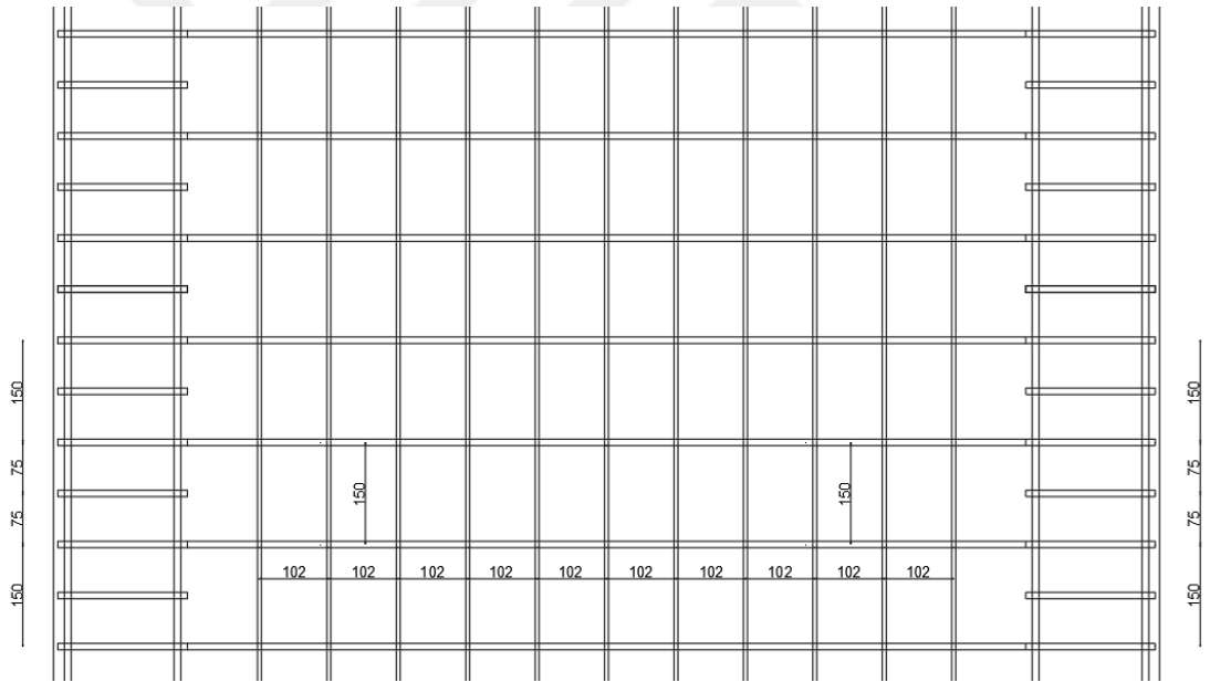
Şekil 4.25. TBDY 2018'e göre oluşturulan perdenin yatay donatı şeması
