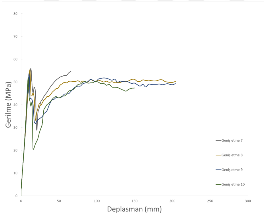
Şekil 5.58. Genişletme 7-10 modellerinin çekme gerilmesi-deplasman grafikleri
