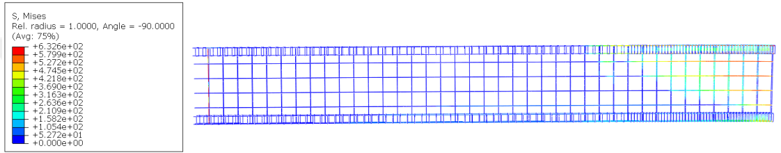
Şekil 5.14. Donatı düzeni-3'e ait modelde donatılar için Von Mises gerilme dağılımı
