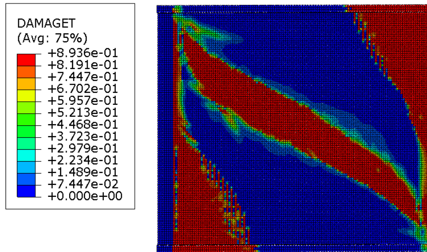
Şekil 5.73. Genişletme 13 modeli beton çekme hasarı
