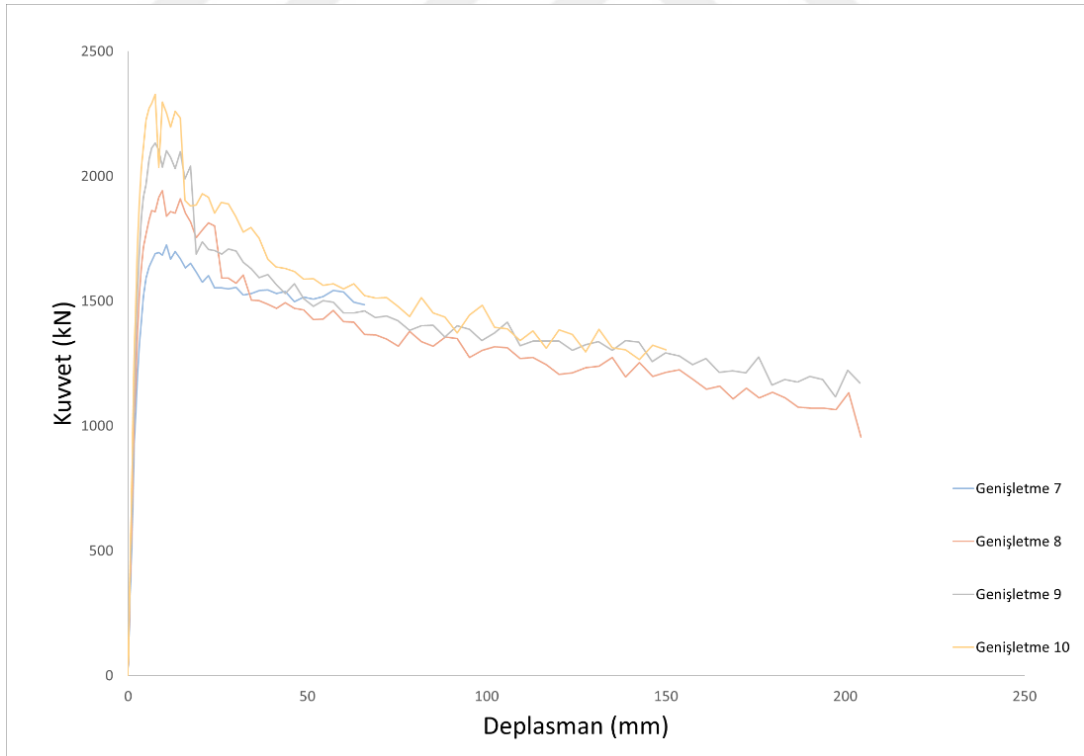
Şekil 5.48. Genişletme 7-10 modellerinin kuvvet deplasman grafikleri
