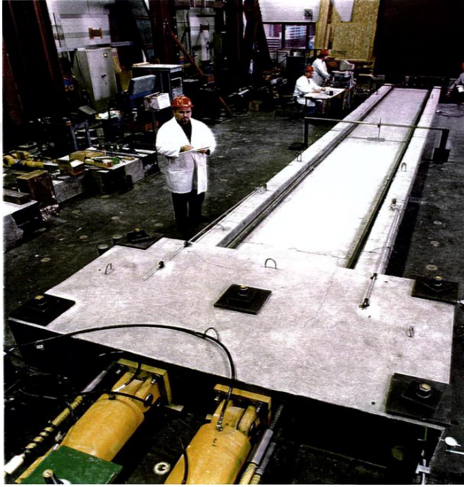
Şekil 4.1. Üretilen perde modeli (İbrahim 2000)
