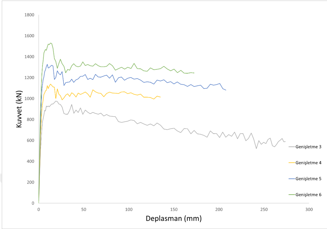
Şekil 5.47. Genişletme 3-6 modellerinin kuvvet deplasman grafikleri
