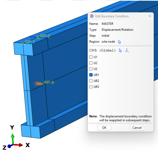
Şekil 4.18. Kısıtlama “Constraint” uygulanması
