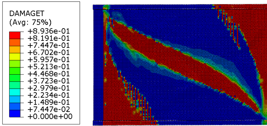
Şekil 5.69. Genişletme 9 modeli beton çekme hasarı
