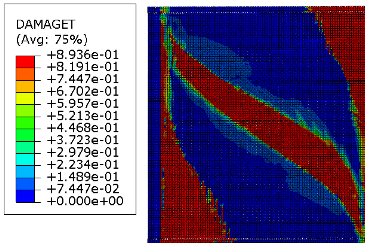
Şekil 5.76. Genişletme 16 modeli beton çekme hasarı
