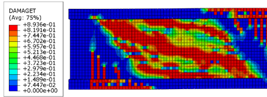
Şekil 5.43. Kısaltma 9 modeli beton çekme hasarı
