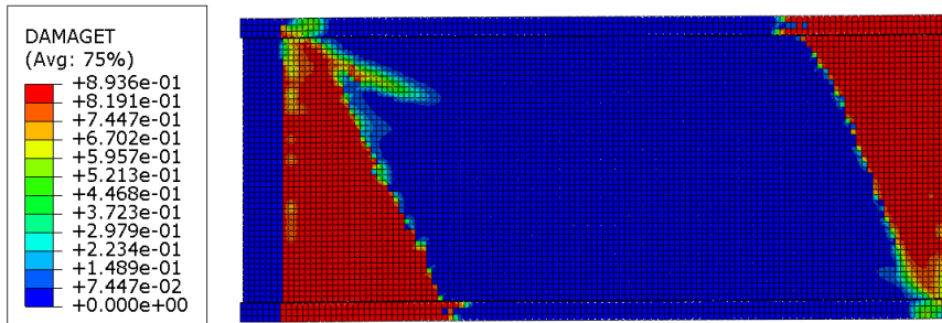
Şekil 5.64. Genişletme 4 modeli beton çekme hasarı
