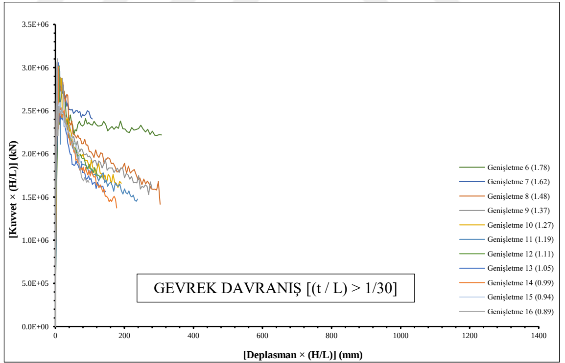
Şekil 5.80. Genişletme 6-16 modelleri için [Kuvvet \times (H/L)] - [Deplasman \times (H/L)]
