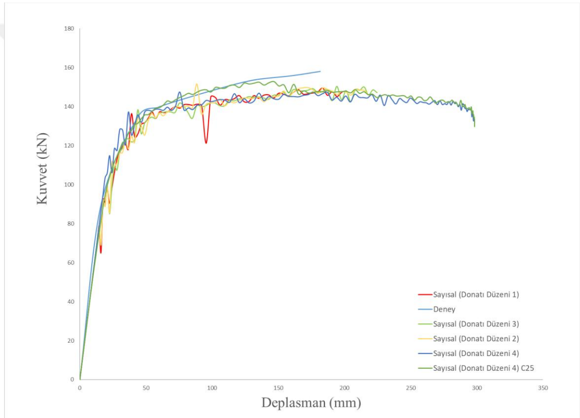
Şekil 5.21. Donatı düzeni farklı modellerin yük-deplasman eğrisi karşılaştırmaları
