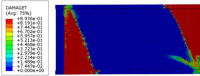
Şekil 5.65. Genişletme 5 modeli beton çekme hasarı
