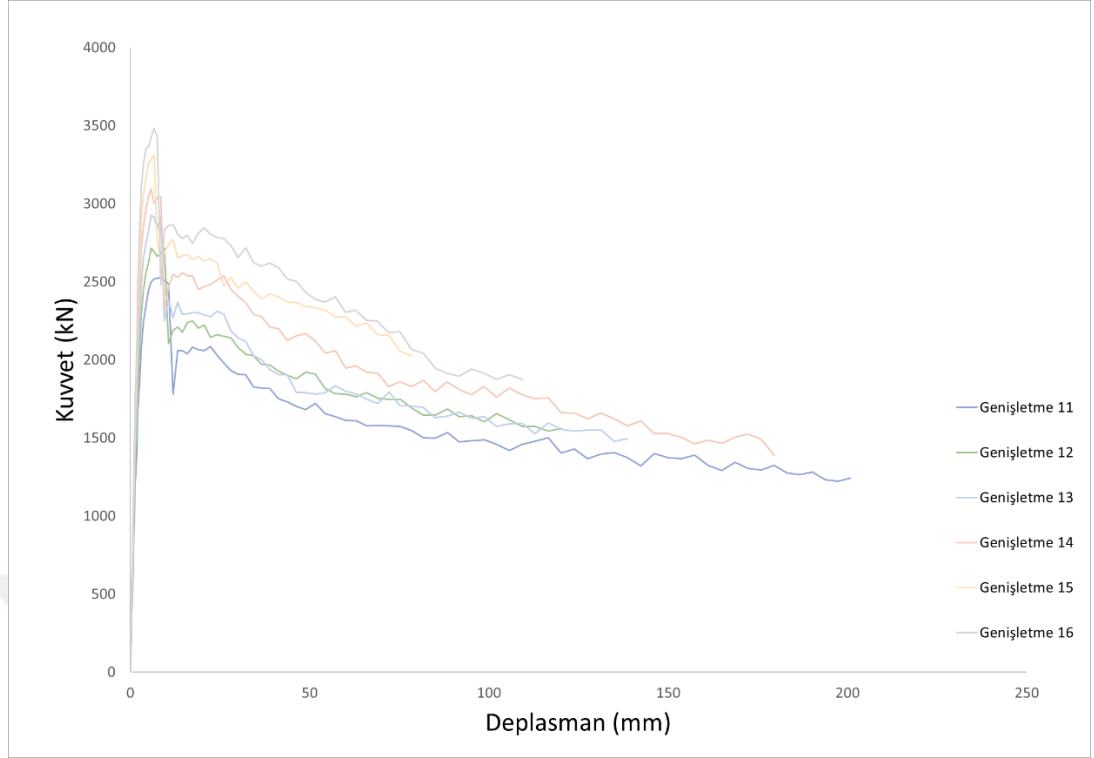
Şekil 5.49. Genişletme 11-16 modellerinin kuvvet deplasman grafikleri
