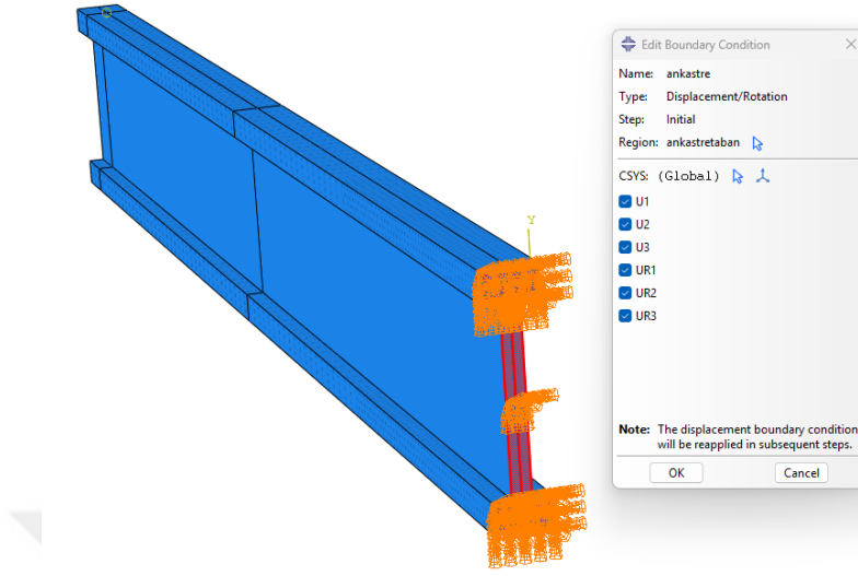
Şekil 4.13. Ankastreliğin tanımlanması
