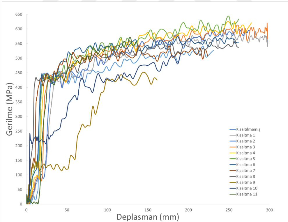
Şekil 5.29. Tüm modellerin çekme gerilmesi-deplasman grafikleri
