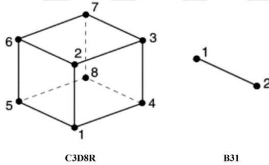
Şekil 4.14. Sonlu eleman tipleri
