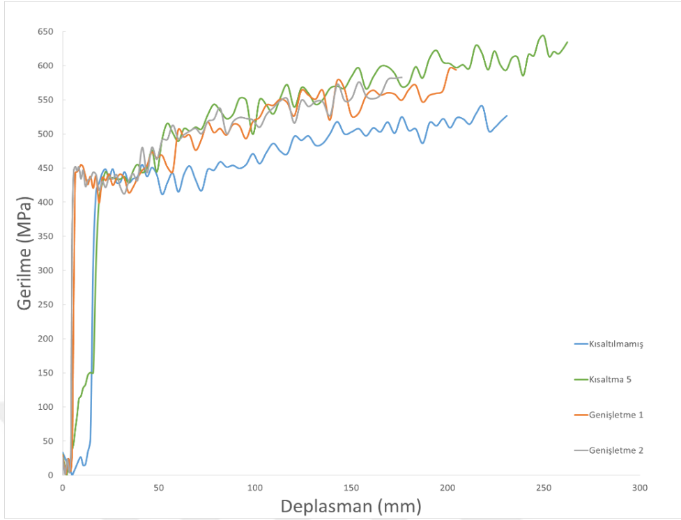
Şekil 5.51. Kısaltılmamış, Kısaltma 5, Genişletme 1 ve Genişletme 2 modellerinin çekme gerilmesi-deplasman grafikleri
