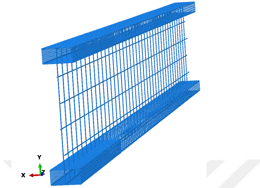
Şekil 4.9. Assembly modülünde tüm donatıların oluşturulması
