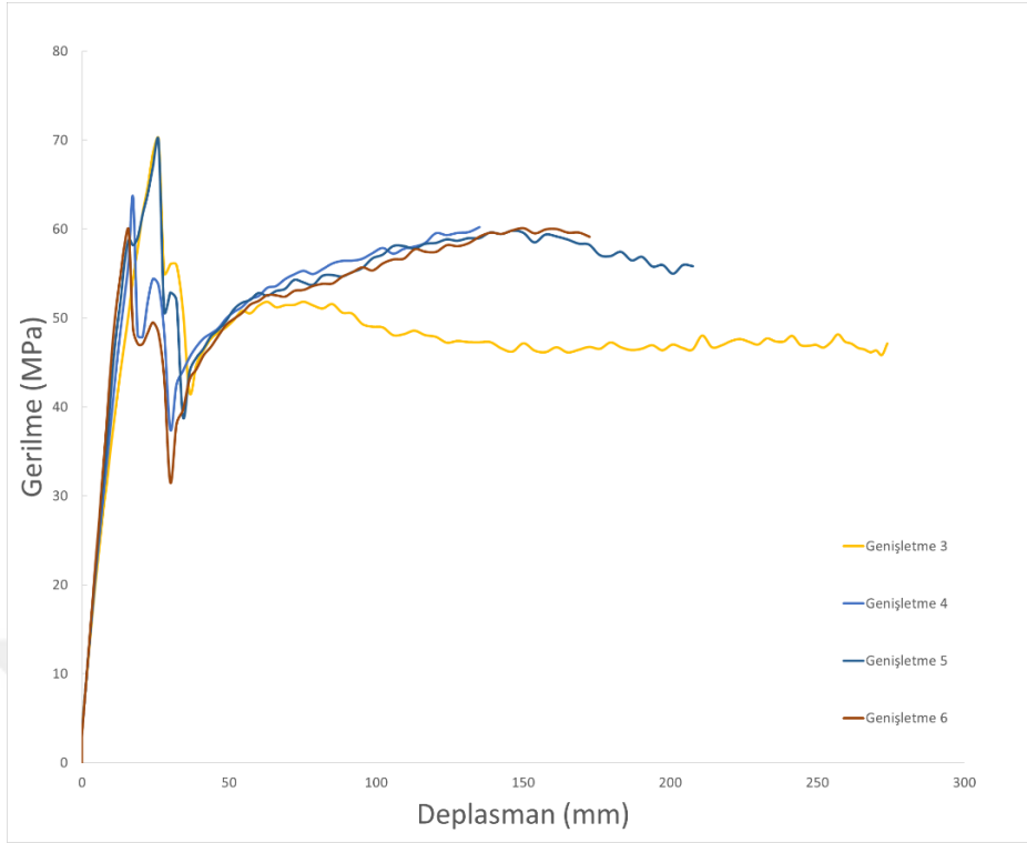
Şekil 5.57. Genişletme 3-6 modellerinin basınç gerilmesi-deplasman grafikleri
