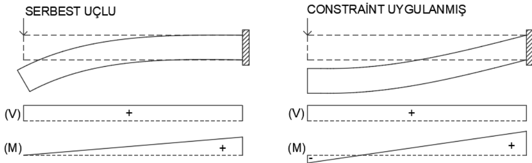
Şekil 4.17. “Constraint” tanımıyla kısıtlanan perde uç dönmesi
