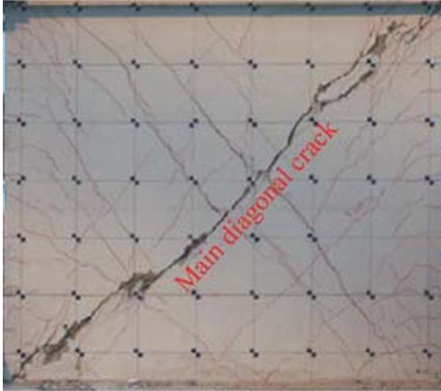
Şekil 3.5. Diyagonal çatlama örneği (Wenlong vd. 2019)
