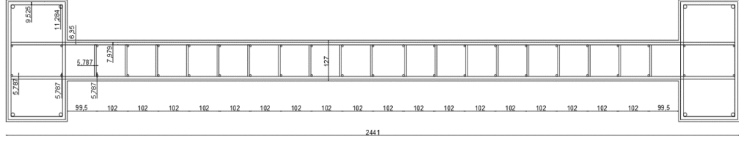
Şekil 4.28. Genişletme 2 modeli donatı düzeni
