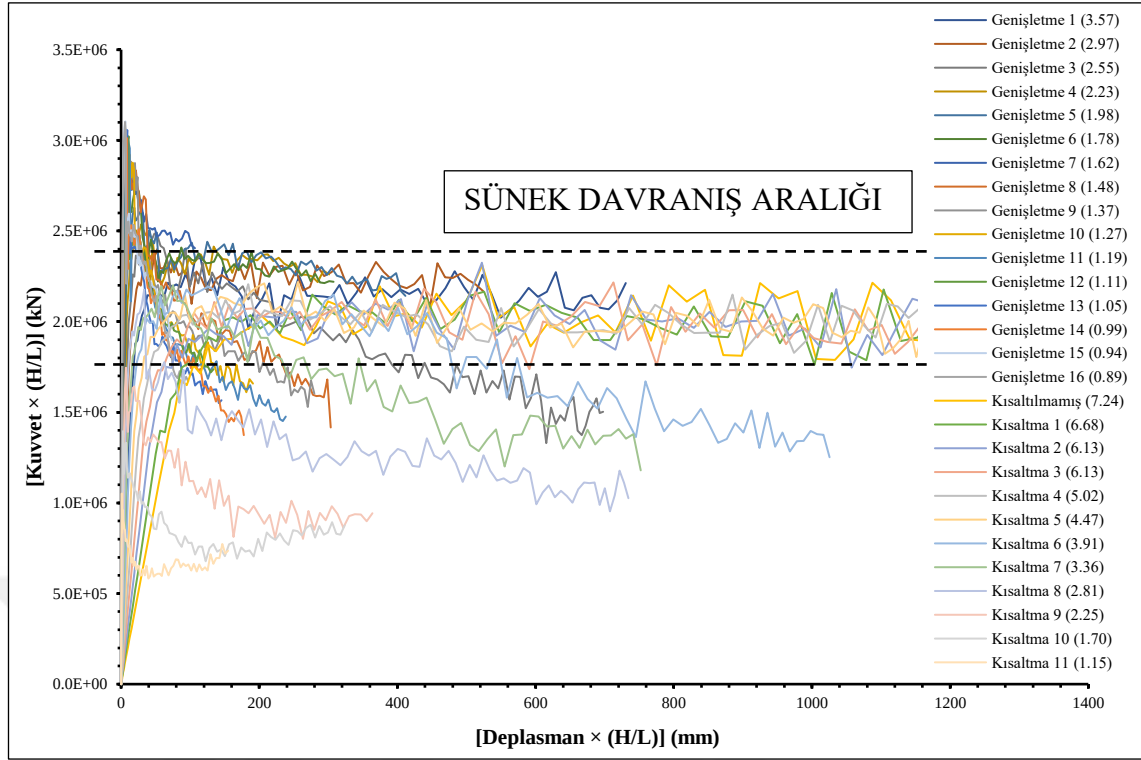
Şekil 5.81. Tüm sayısal modeller için [Kuvvet×(H/L)]–[Deplasman×(H/L)]
