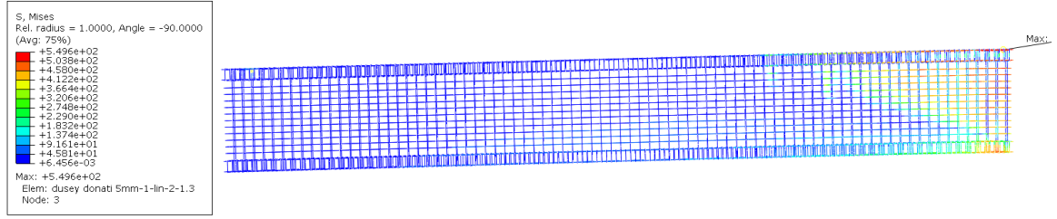
Şekil 5.20. Donatı düzeni-4 C25 modelinde donatılar için Von Mises gerilme dağılımı
