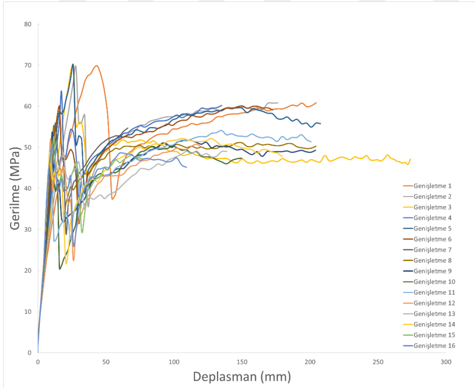
Şekil 5.60. Tüm genişletme modellerinin basınç gerilmesi-deplasman grafikleri
