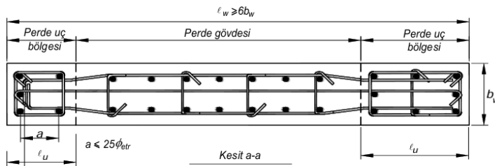
Şekil 3.12. TBDY 2018 donatı düzeni
