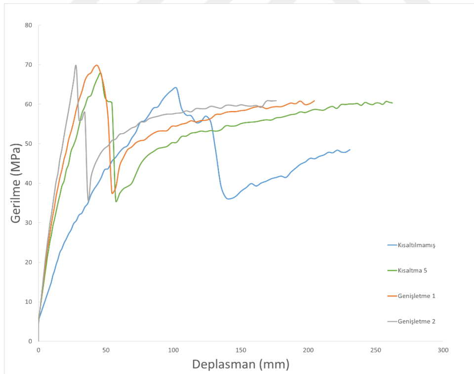
Şekil 5.56. Kısıltılmamış, Kısıltma 5, Genişletme 1 ve Genişletme 2 modellerinin basınç gerilmesi-deplasman grafikleri
