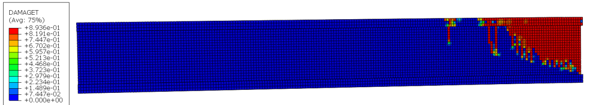
Şekil 5.16. Donatı düzeni-4'e ait model için beton çekme hasar dağılımı
